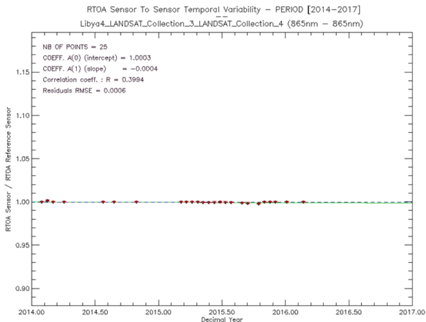
Figure 5-Temporal variability of the ratio RTOA OLI ESA / RTOA OLI USGS (NIR band)
