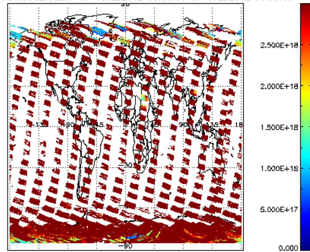
SCIOL2P_NADIR3CO_vcd_Lerr for 18FEB2012 00:00:00 to 19FEB2012 00:00:00
