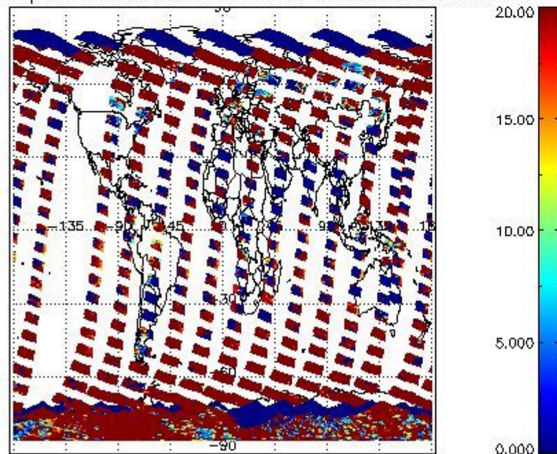
cL_opt_depth for 12FEB2012 00:00:00 to 13FEB2012 00:00:00
