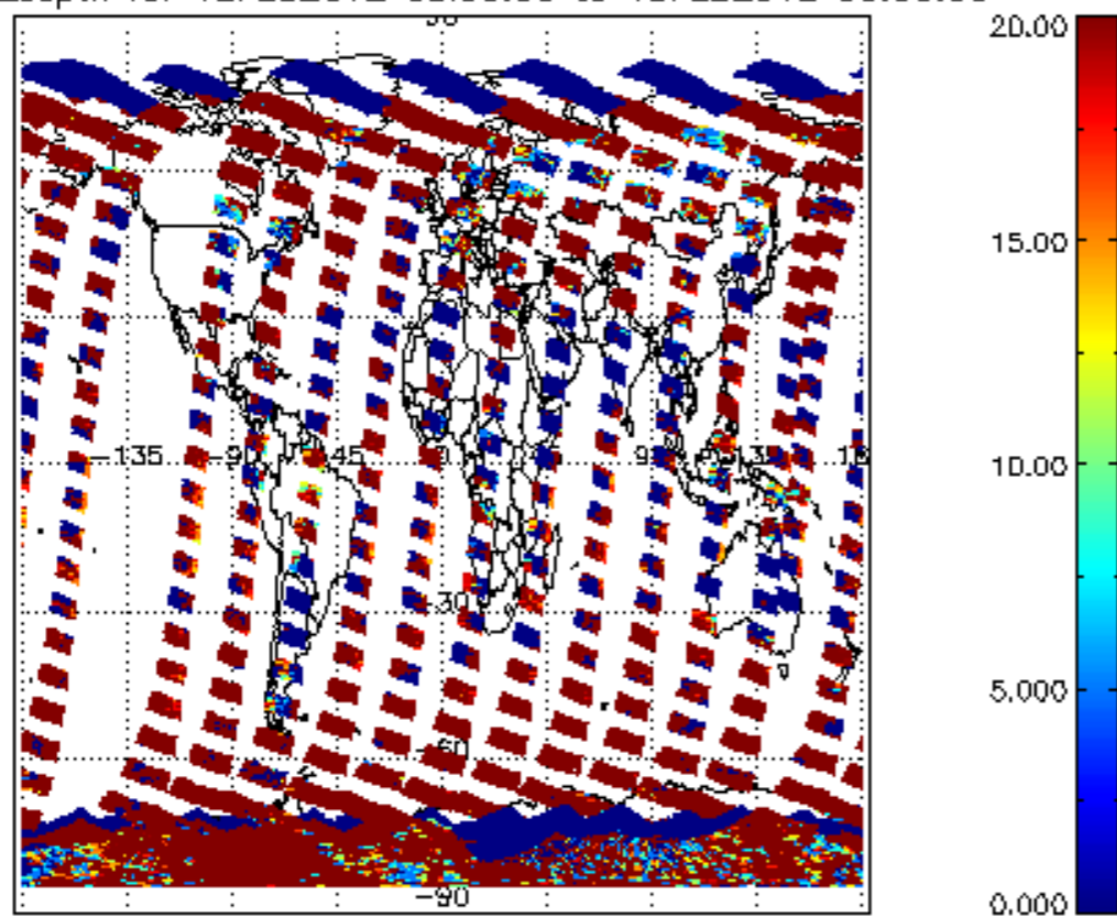
cl_opt_depth for 12FEB2012 00:00:00 to 13FEB2012 00:00:00
