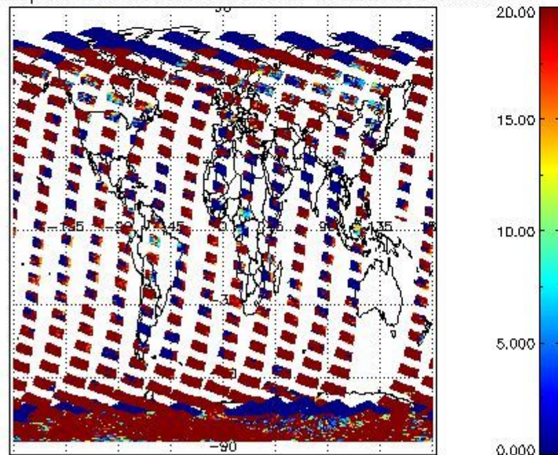
cL_opt_depth for 09FEB2012 00:00:00 to 10FEB2012 00:00:00
