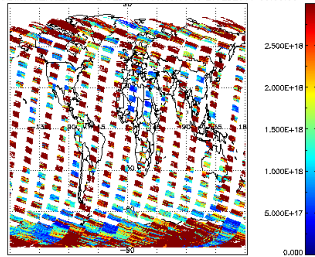
SCIOL2P_NADIR3CO_vcd_Lerr for 26FEB2011 00:00:00 to 27FEB2011 00:00:00
