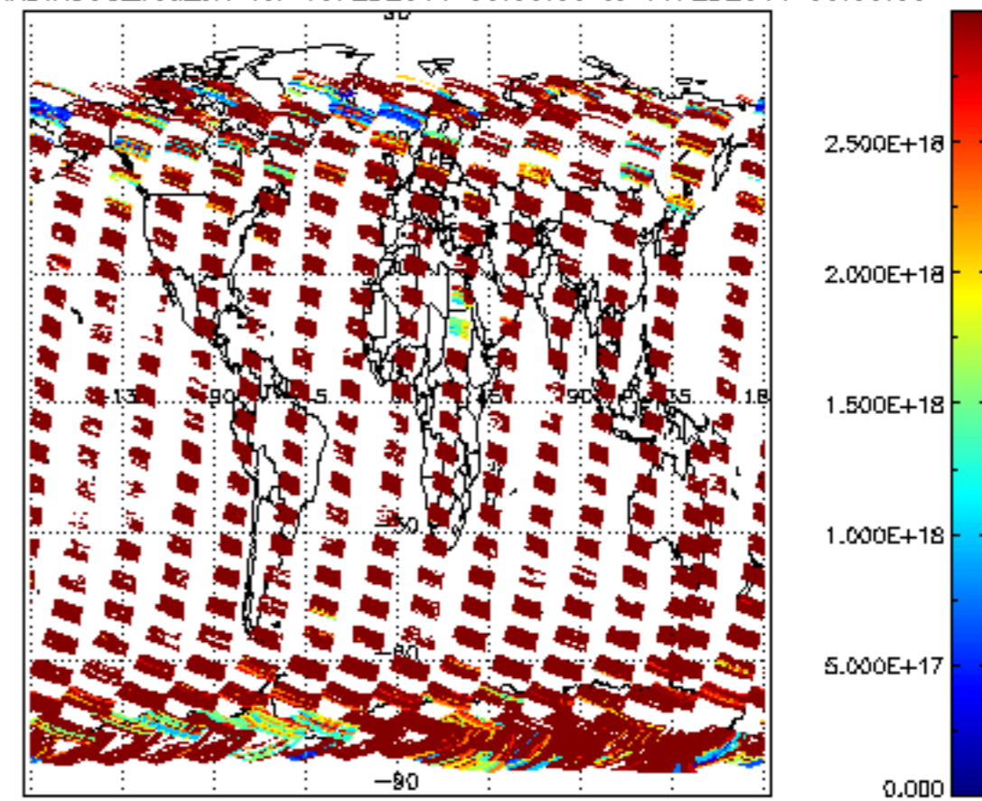
SCIOL2P_NADIR3CO_vcd_Lerr for 15FEB2011 00:00:00 to 16FEB2011 00:00:00
