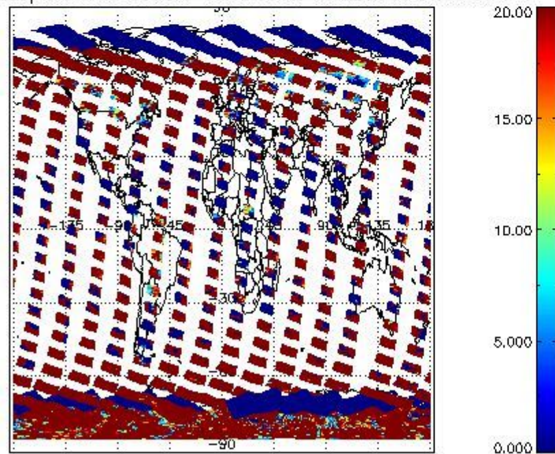
cL_opt_depth for 09FEB2011 00:00:00 to 10FEB2011 00:00:00
