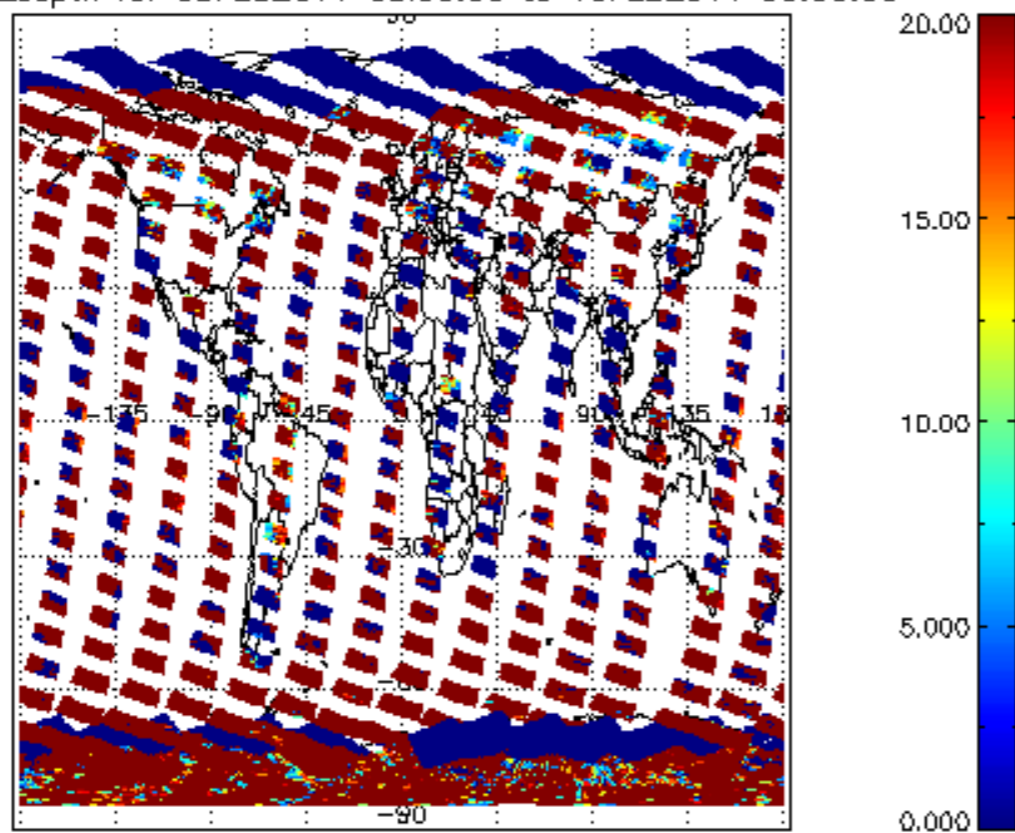
cL_opt_depth for 09FEB2011 00:00:00 to 10FEB2011 00:00:00
