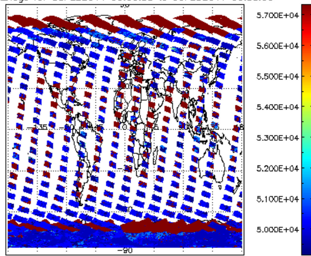
cloud_flags for 08FEB2011 00:00:00 to 09FEB2011 00:00:00
