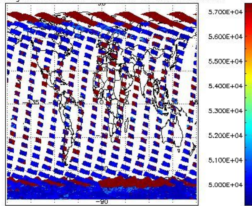
cloud_flags for 08FEB2011 00:00:00 to 09FEB2011 00:00:00
