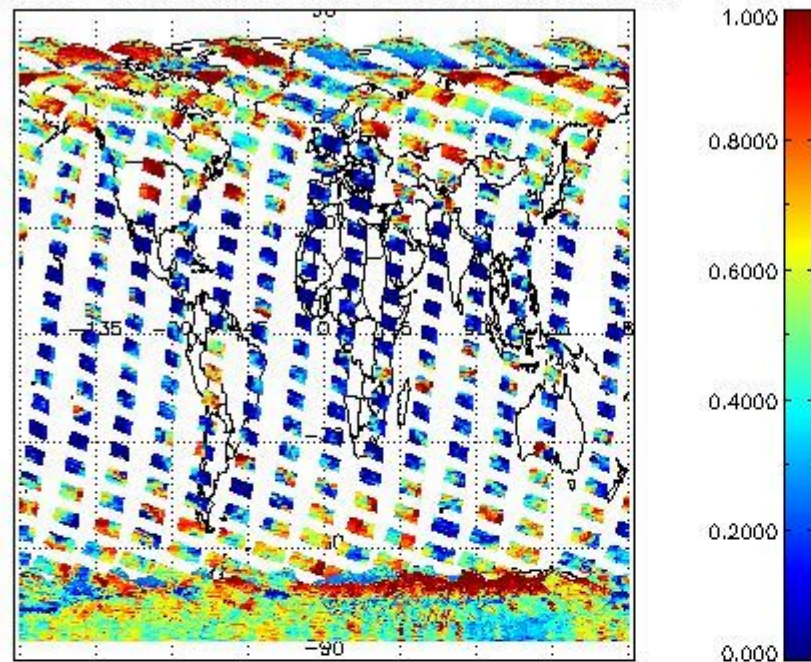
cL_frae for 08FEB2011 00:00:00 to 09FEB2011 00:00:00
