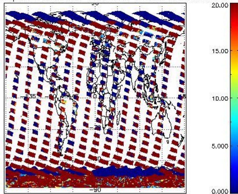
cL_opt_depth for 08FEB2011 00:00:00 to 09FEB2011 00:00:00
