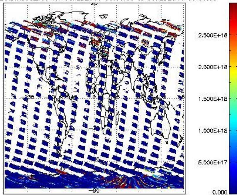
SCIDL2P_NADIR3CO_vcd for 08FEB2011 00:00:00 to 09FEB2011 00:00:00
