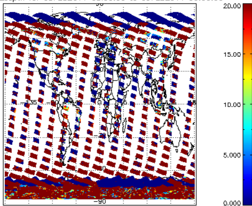
cL_opt_depth for 08FEB2011 00:00:00 to 09FEB2011 00:00:00
