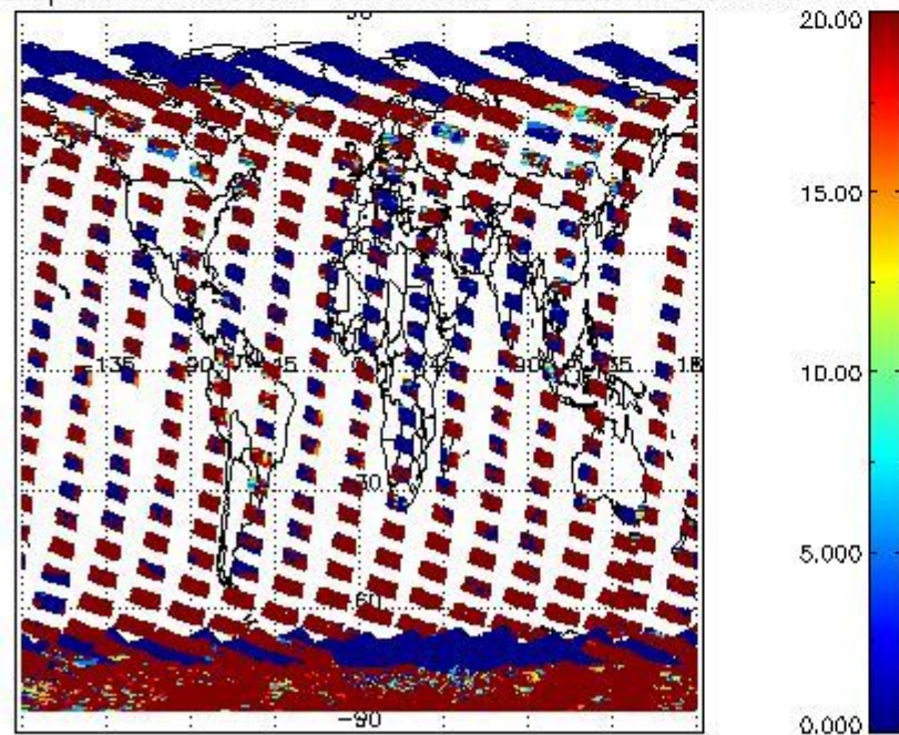
cL_opt_depth for 07FEB2011 00:00:00 to 08FEB2011 00:00:00
