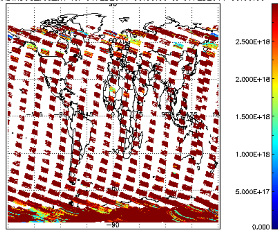
SCIOL2P_NADIR3CO_vcd_Lerr for 06FEB2011 00:00:00 to 07FEB2011 00:00:00
