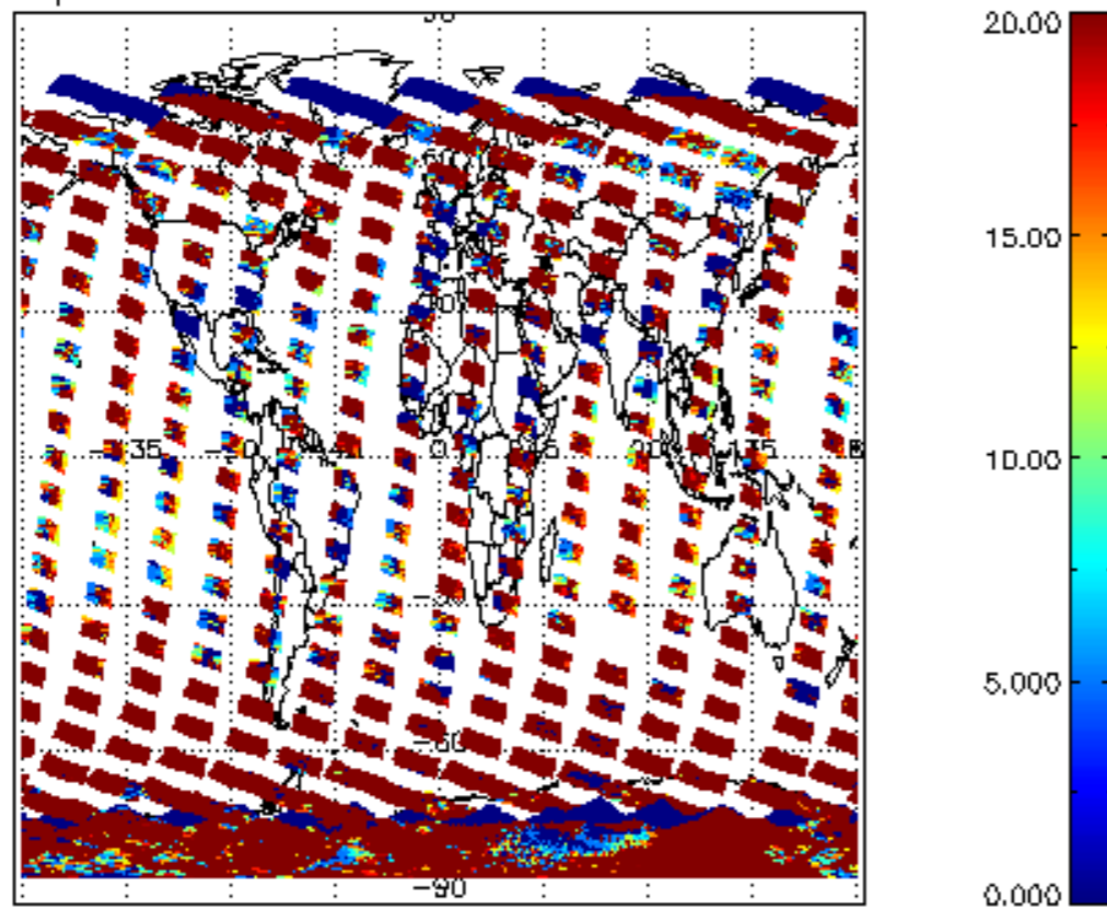
cl_opt_depth for 08FEB2008 00:00:00 to 09FEB2008 00:00:00
