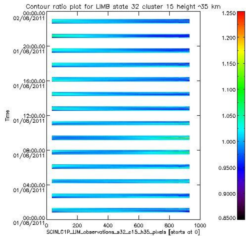
sciamachy_i1b_source_packet_report_SCIA_7_04_U_20110801_21.PNG
