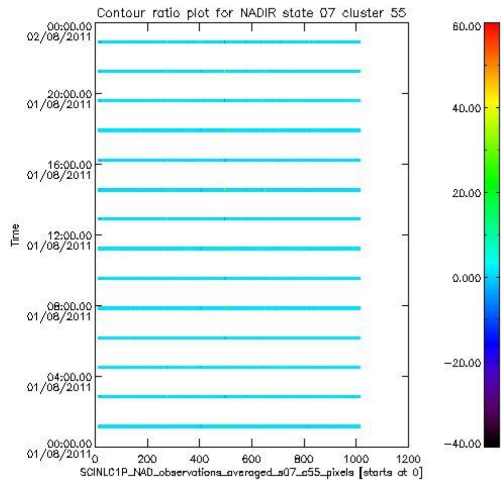
sciamachy_l1b_source_packet_report_SCIA_7_04_U_20110801_9.PNG
