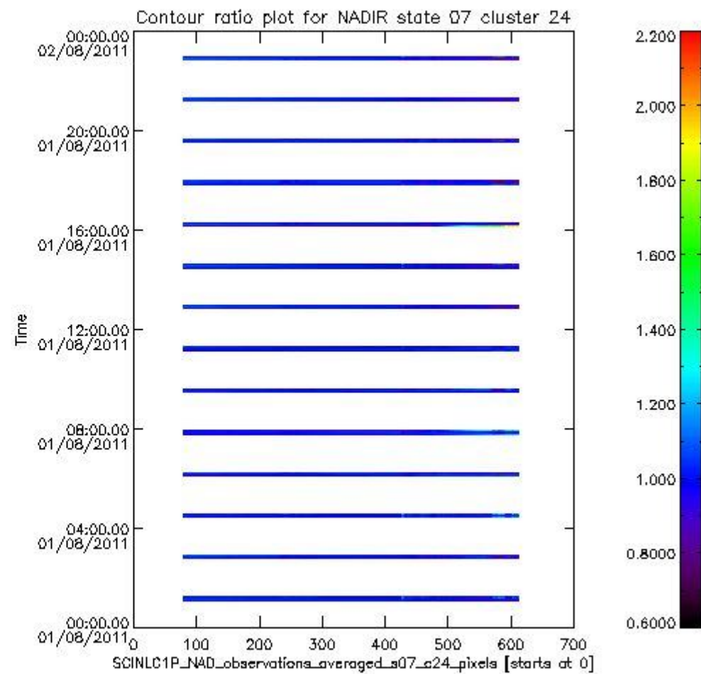
sciamachy_l1b_source_packet_report_SCIA_7_04_U_20110801_7.PNG
