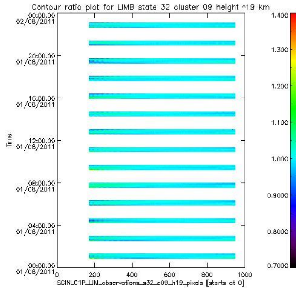
sciamachy_l1b_source_packet_report_SCIA_7_04_U_20110801_11.PNG
