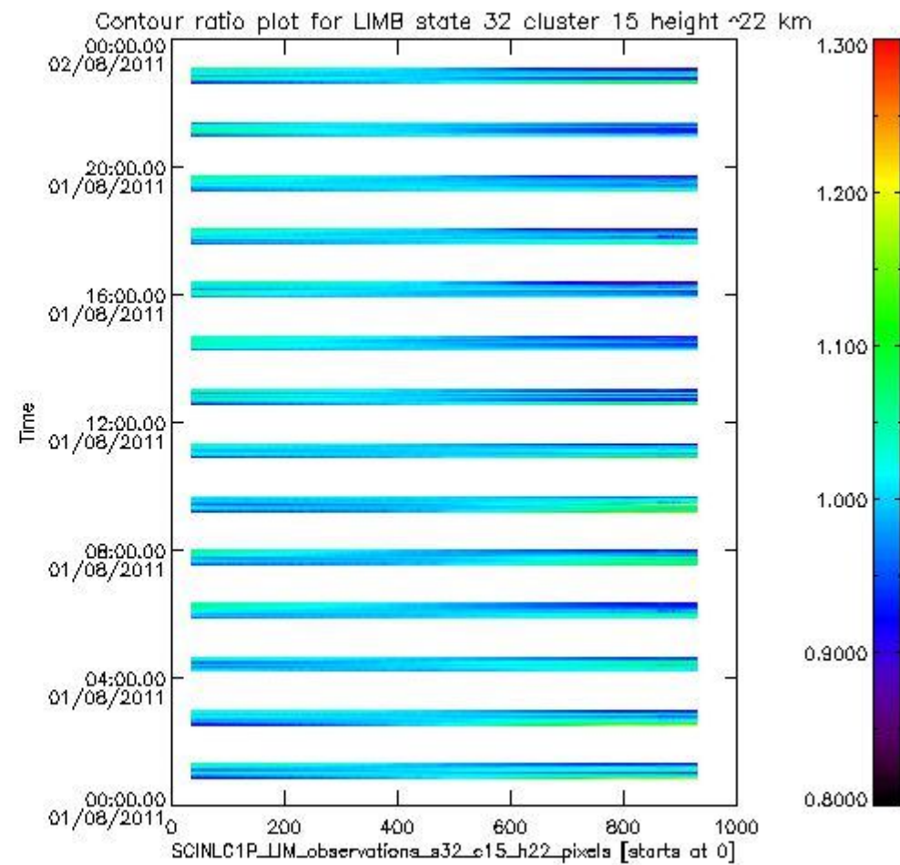
sciamachy_11b_source_packet_report_SCIA_7_04_U_20110801_17.PNG
