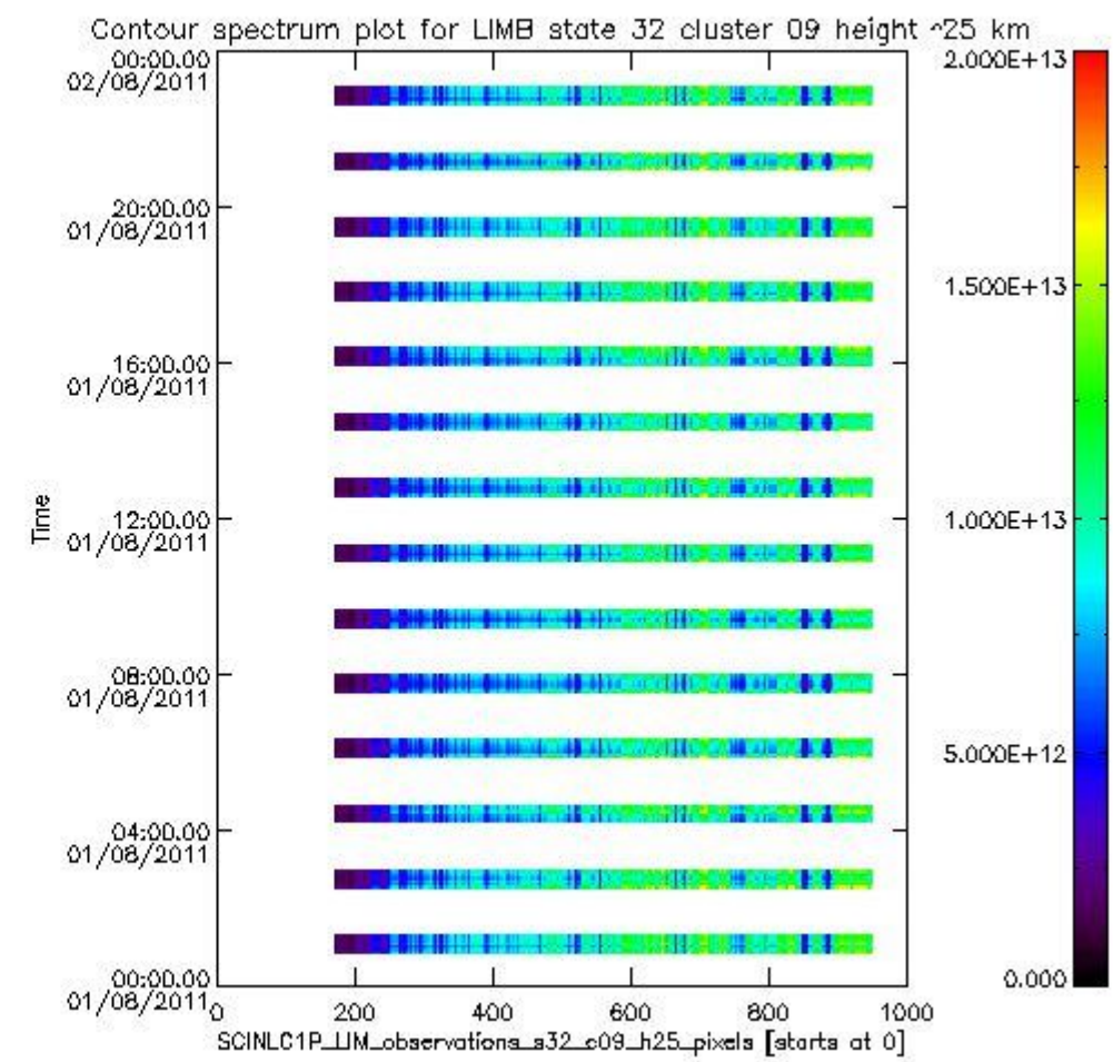
sciamachy_l1b_source_packet_report_SCIA_7_04_U_20110801_14.PNG
