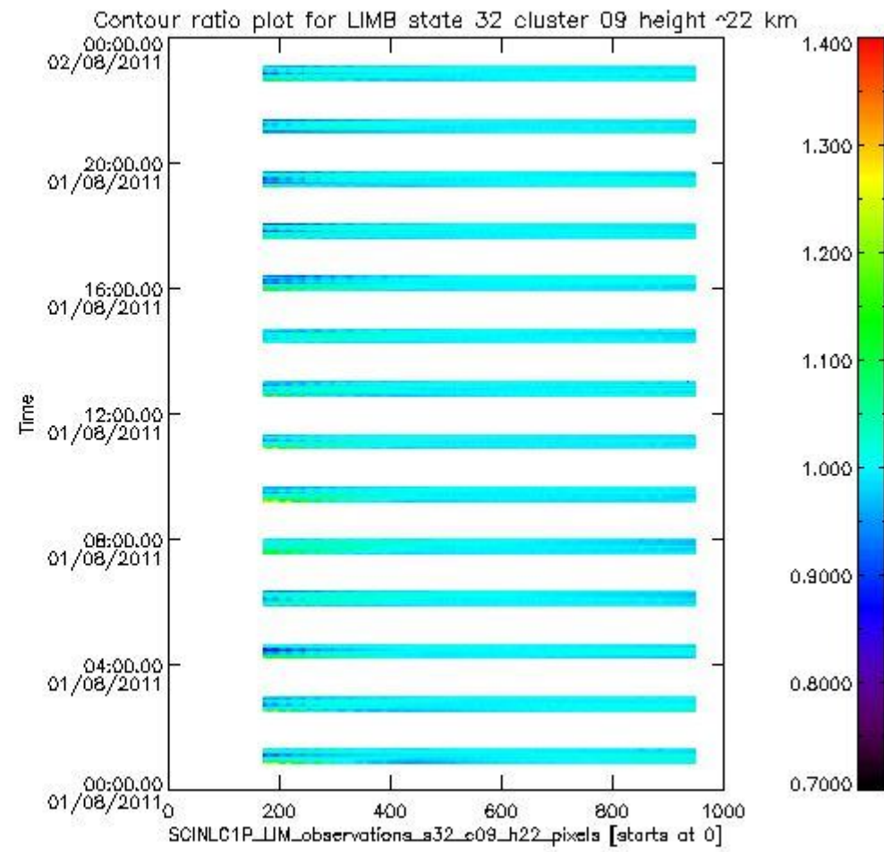
sciamachy_l1b_source_packet_report_SCIA_7_04_U_20110801_13.PNG
