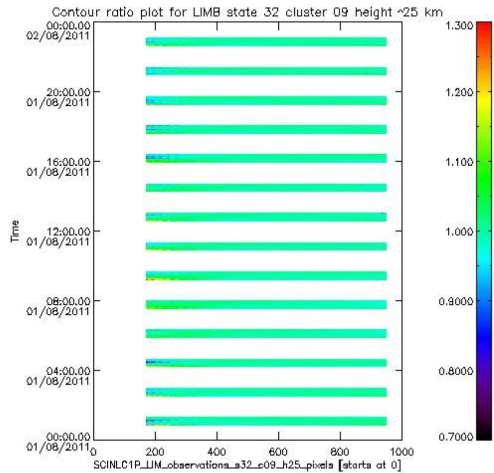
sciamachy_l1b_source_packet_report_SCIA_7_04_U_20110801_15.PNG
