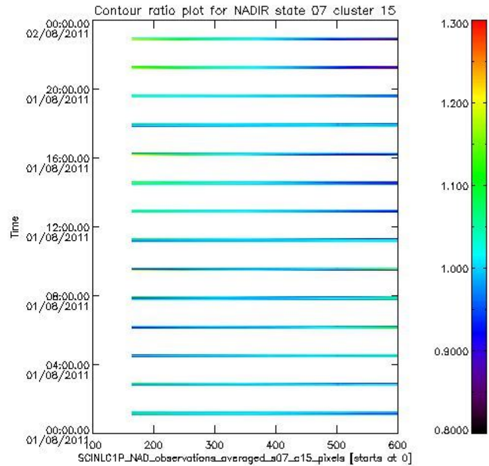
sciamachy_l1b_source_packet_report_SCIA_7_04_U_20110801_5.PNG
