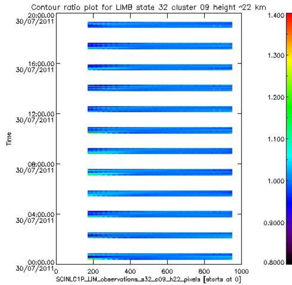
sciamachy_l1b_source_packet_report_SCIA_7_04_U_20110730_13.PNG
