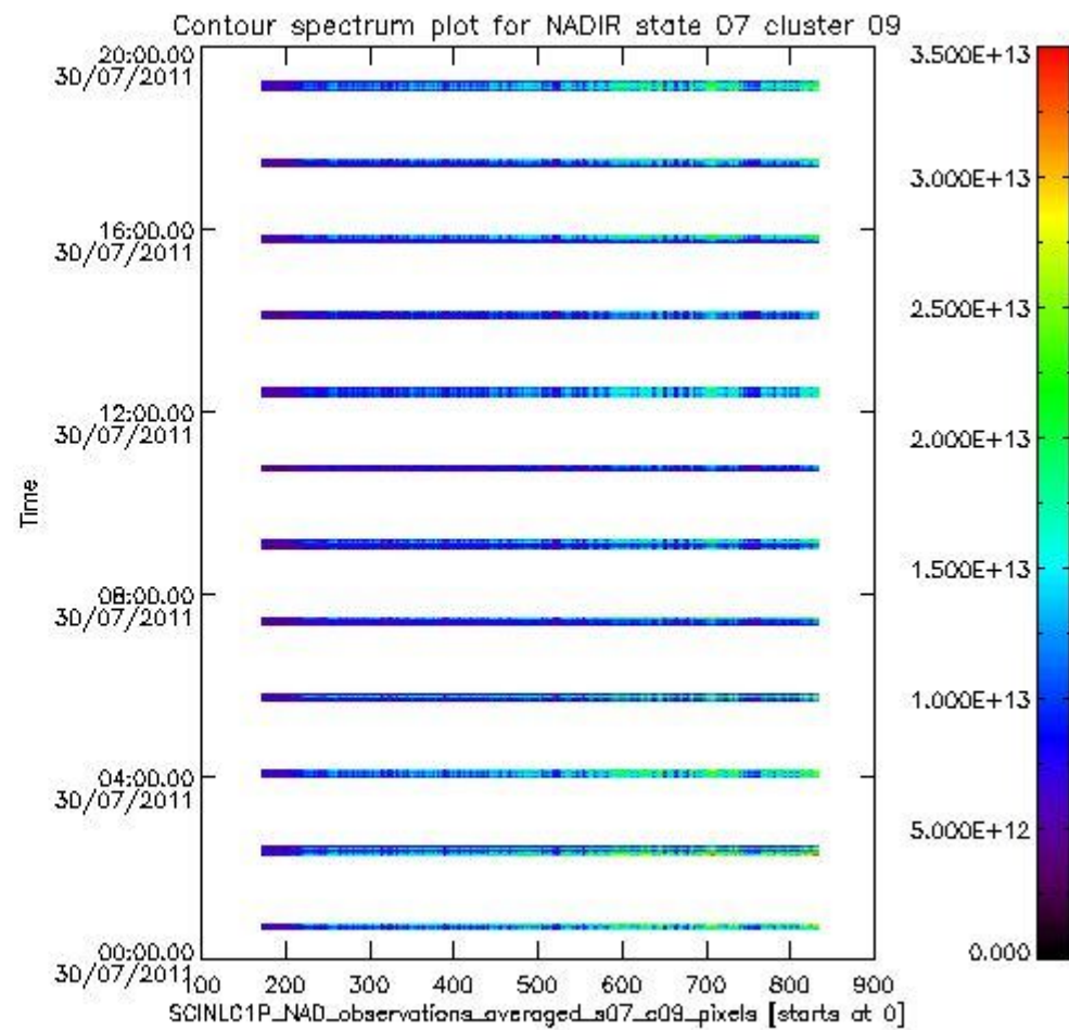
sciamachy_i1b_source_packet_report_SCIA_7_04_U_20110730_2.PNG
