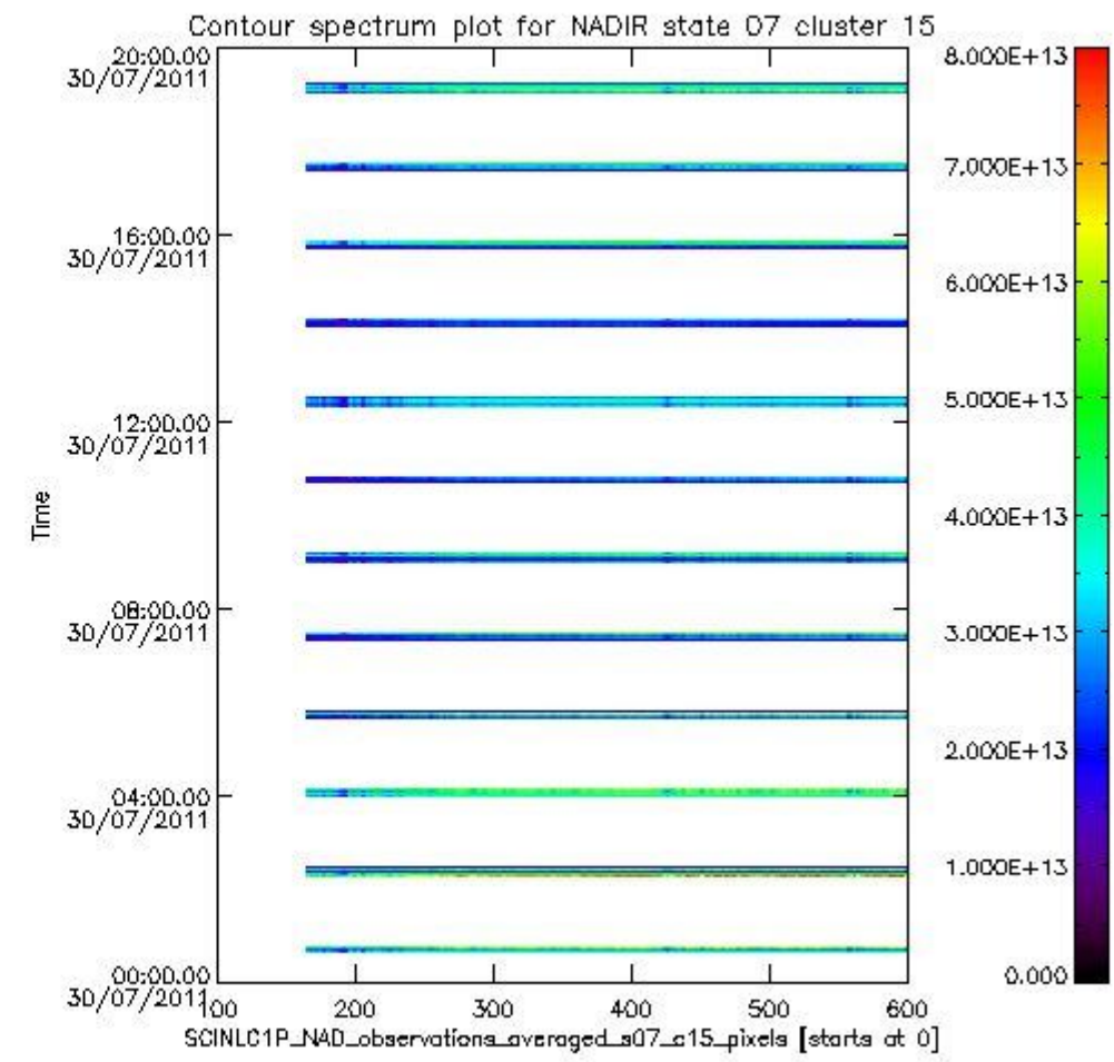
sciamachy_i1b_source_packet_report_SCIA_7_04_U_20110730_4.PNG
