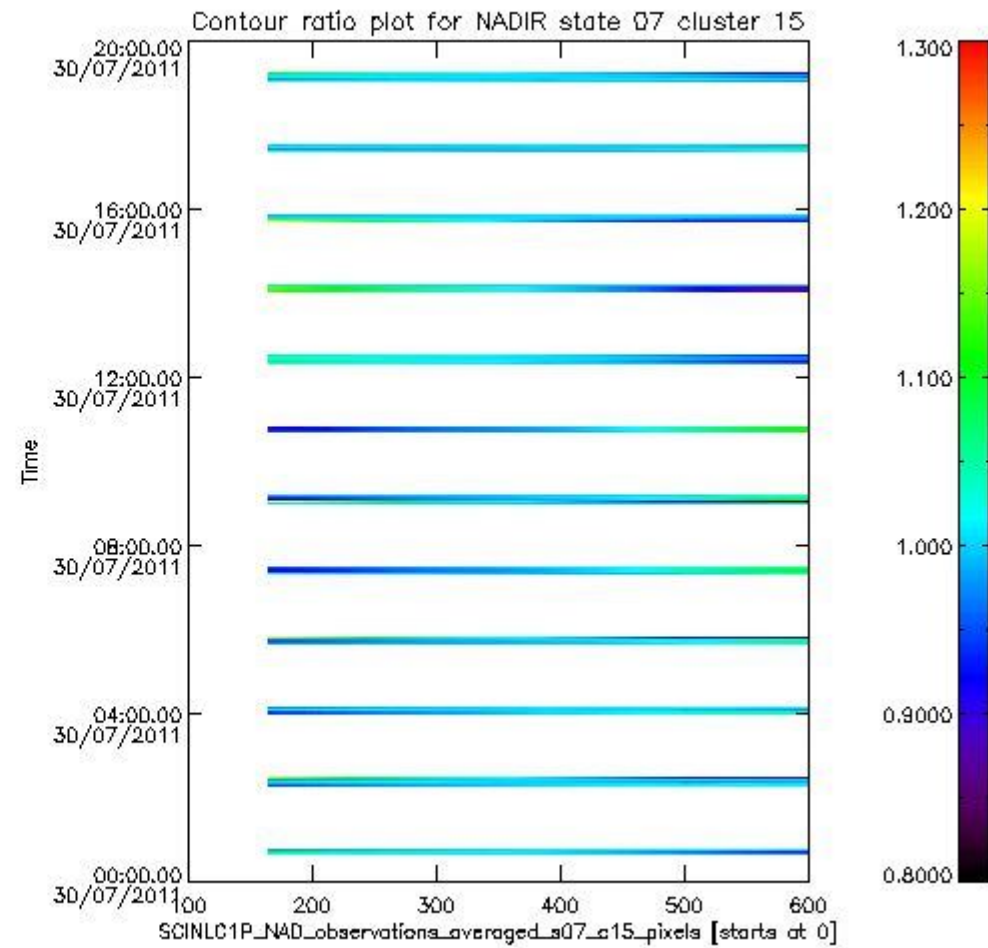
sciamachy_l1b_source_packet_report_SCIA_7_04_U_20110730_5.PNG
