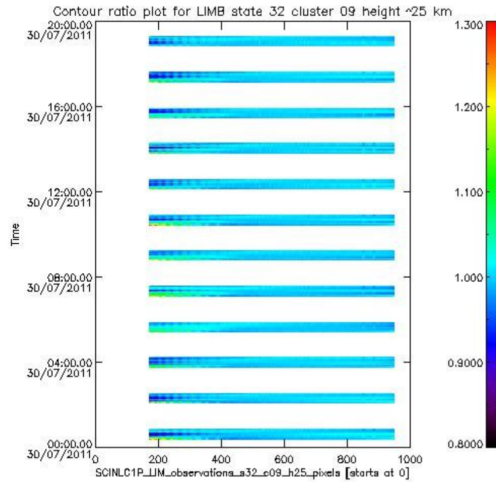
sciamachy_l1b_source_packet_report_SCIA_7_04_U_20110730_15.PNG
