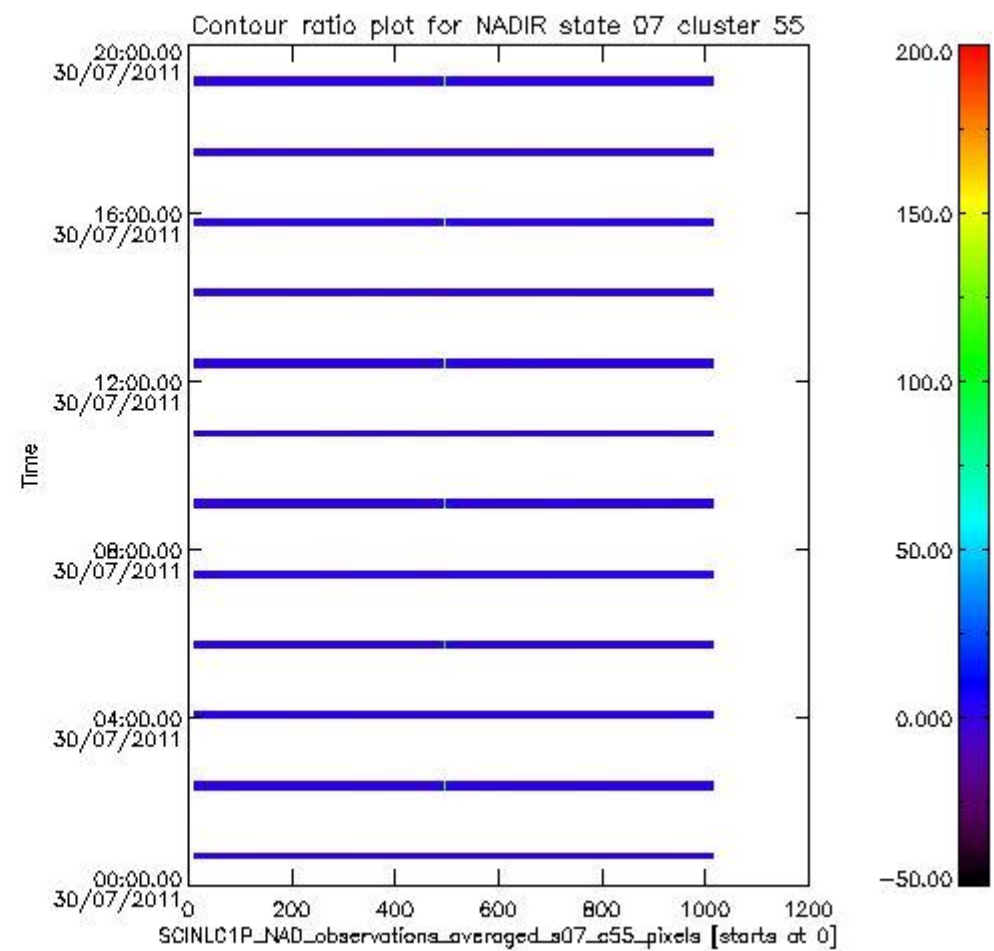
sciamachy_l1b_source_packet_report_SCIA_7_04_U_20110730_9.PNG
