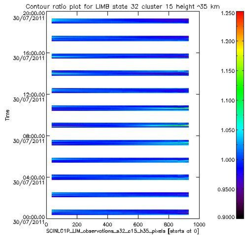
sciamachy_i1b_source_packet_report_SCIA_7_04_U_20110730_21.PNG
