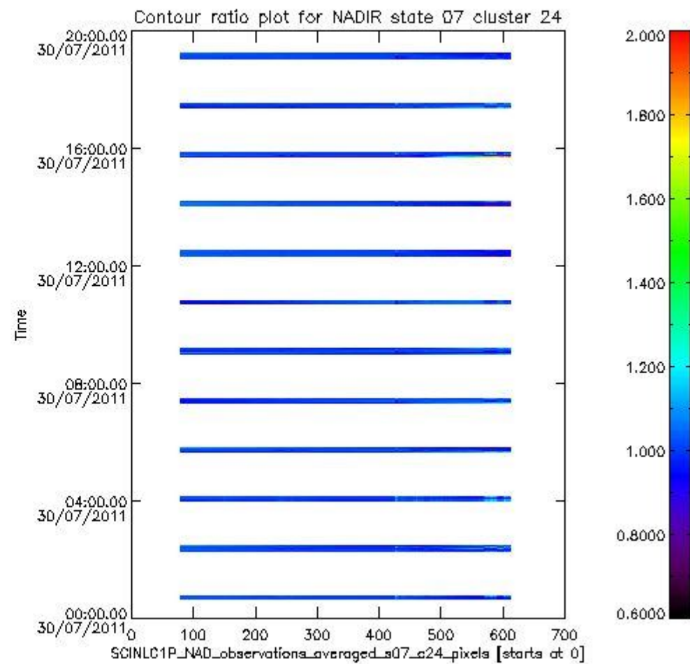
sciamachy_l1b_source_packet_report_SCIA_7_04_U_20110730_7.PNG
