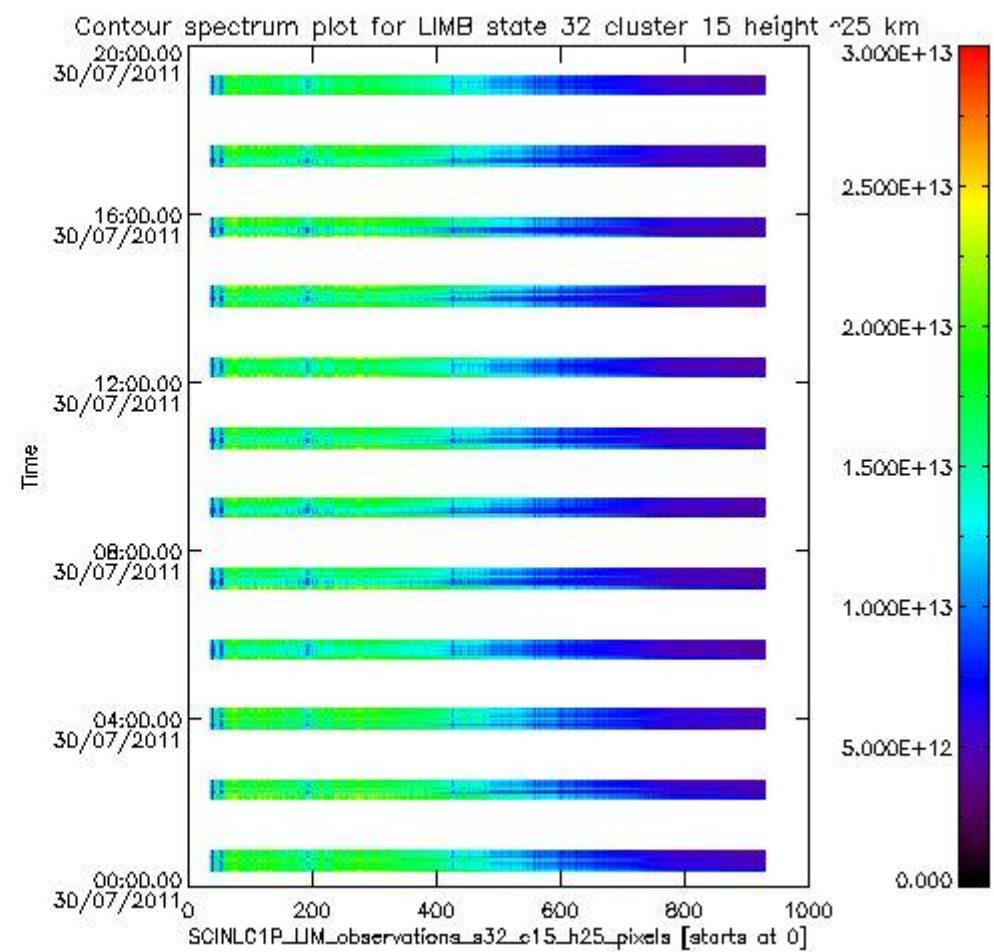
sciamachy_l1b_source_packet_report_SCIA_7_04_U_20110730_18.PNG
