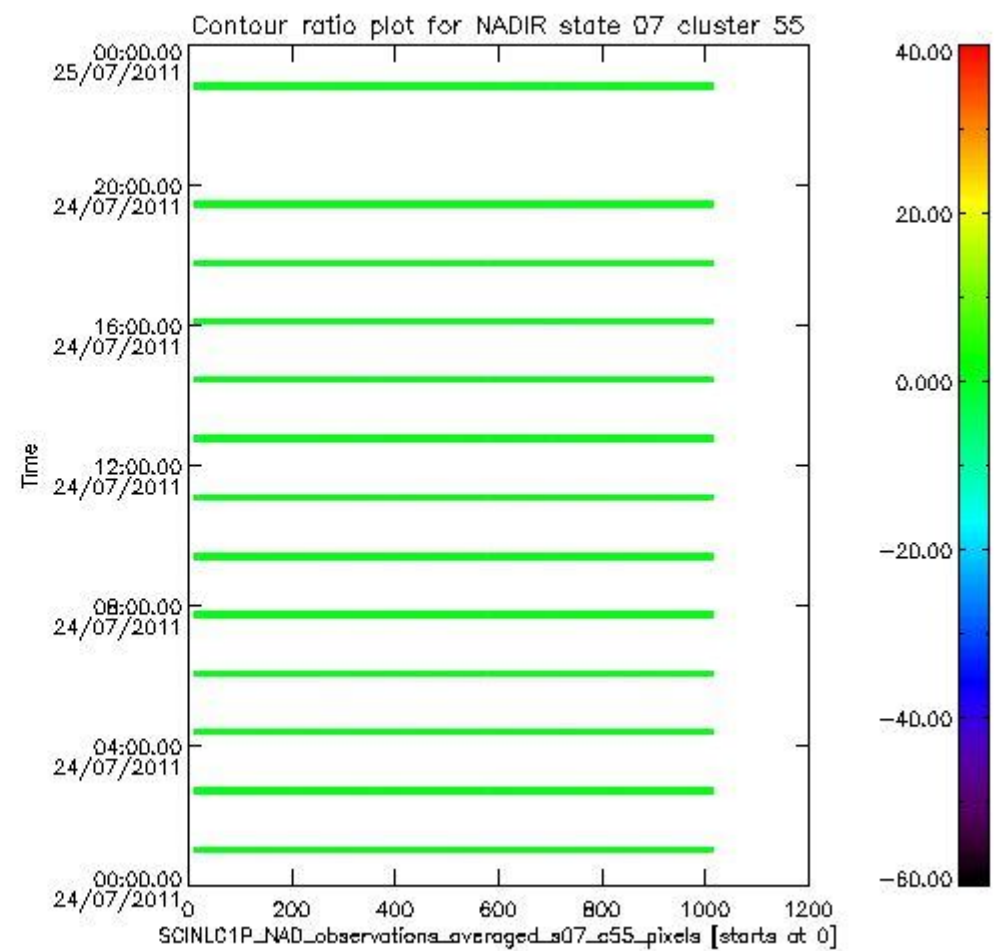
sciamachy_l1b_source_packet_report_SCIA_7_04_U_20110724_9.PNG
