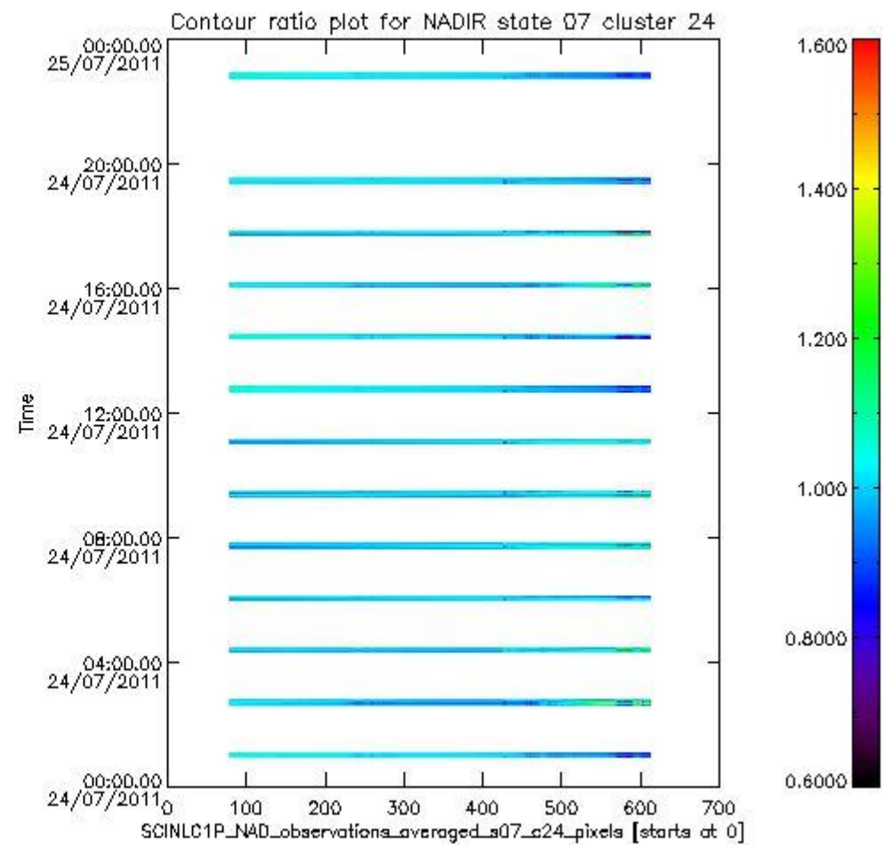
sciamachy_l1b_source_packet_report_SCIA_7_04_U_20110724_7.PNG
