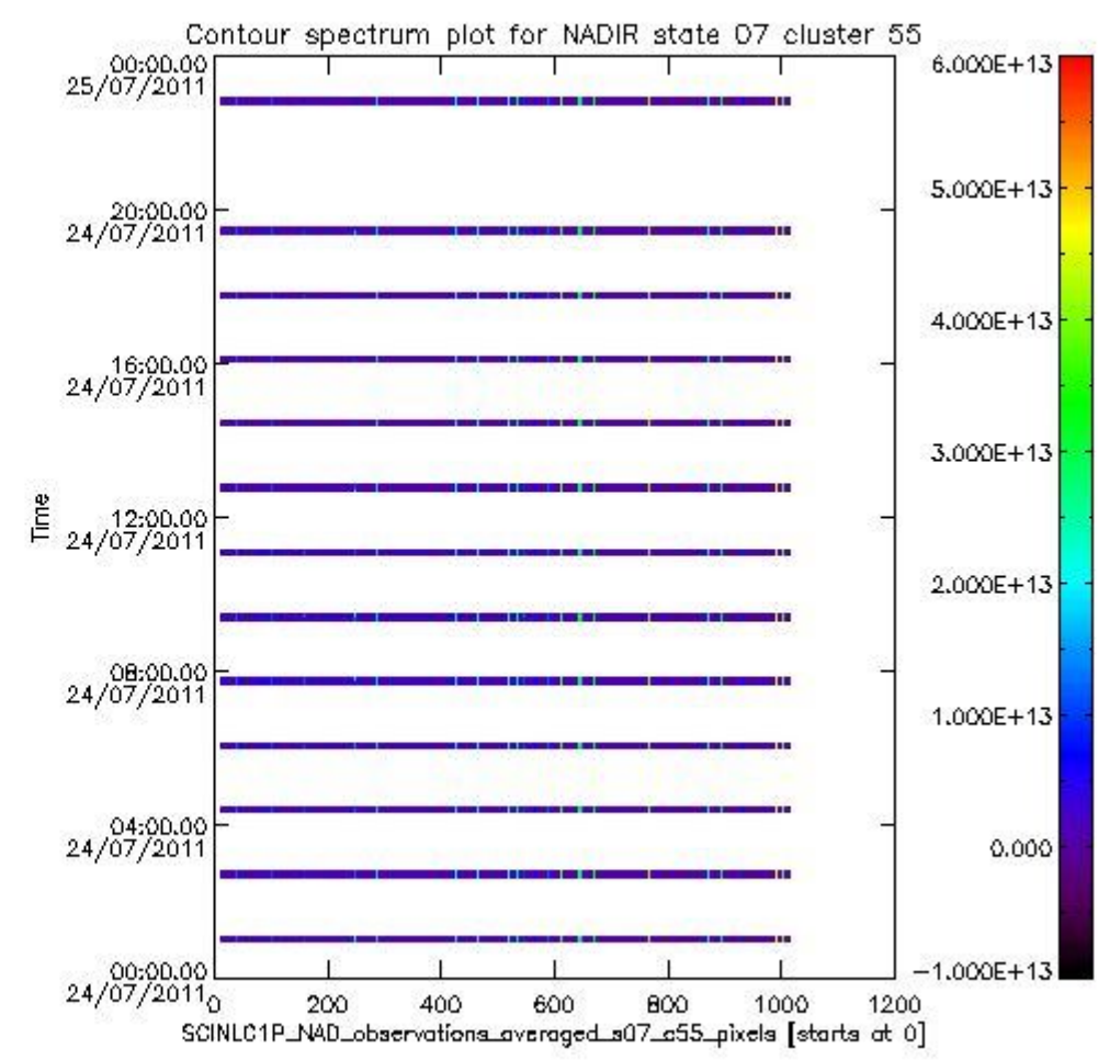
sciamachy_i1b_source_packet_report_SCIA_7_04_U_20110724_8.PNG
