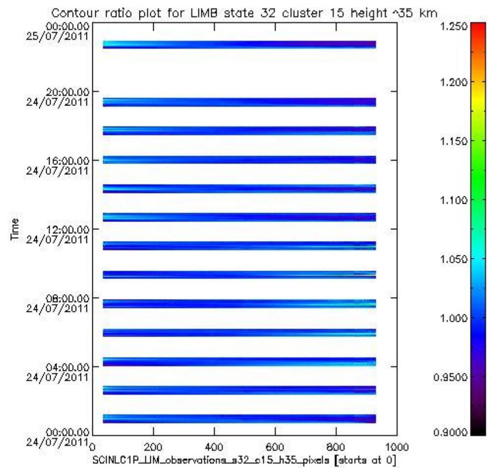
sciamachy_i1b_source_packet_report_SCIA_7_04_U_20110724_21.PNG
