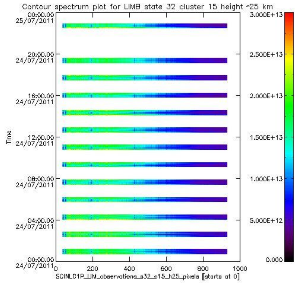
sciamachy_l1b_source_packet_report_SCIA_7_04_U_20110724_18.PNG
