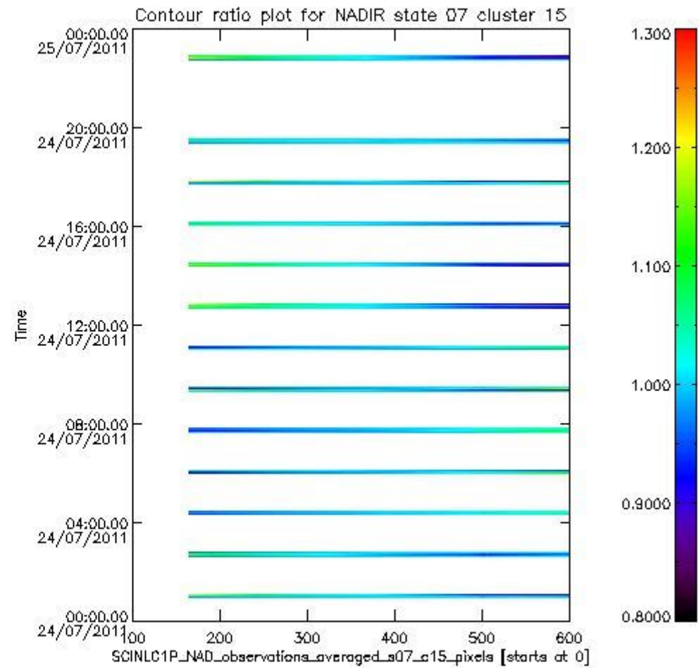
sciamachy_l1b_source_packet_report_SCIA_7_04_U_20110724_5.PNG
