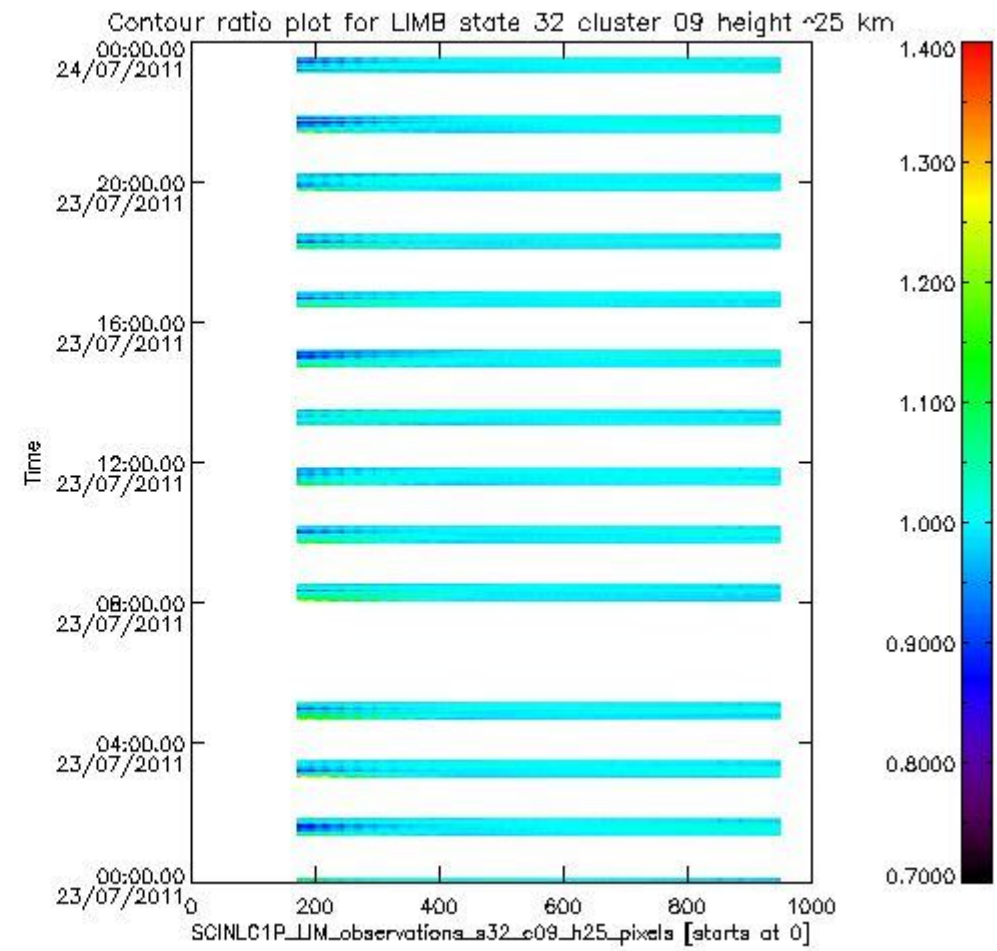
sciamachy_l1b_source_packet_report_SCIA_7_04_U_20110723_15.PNG
