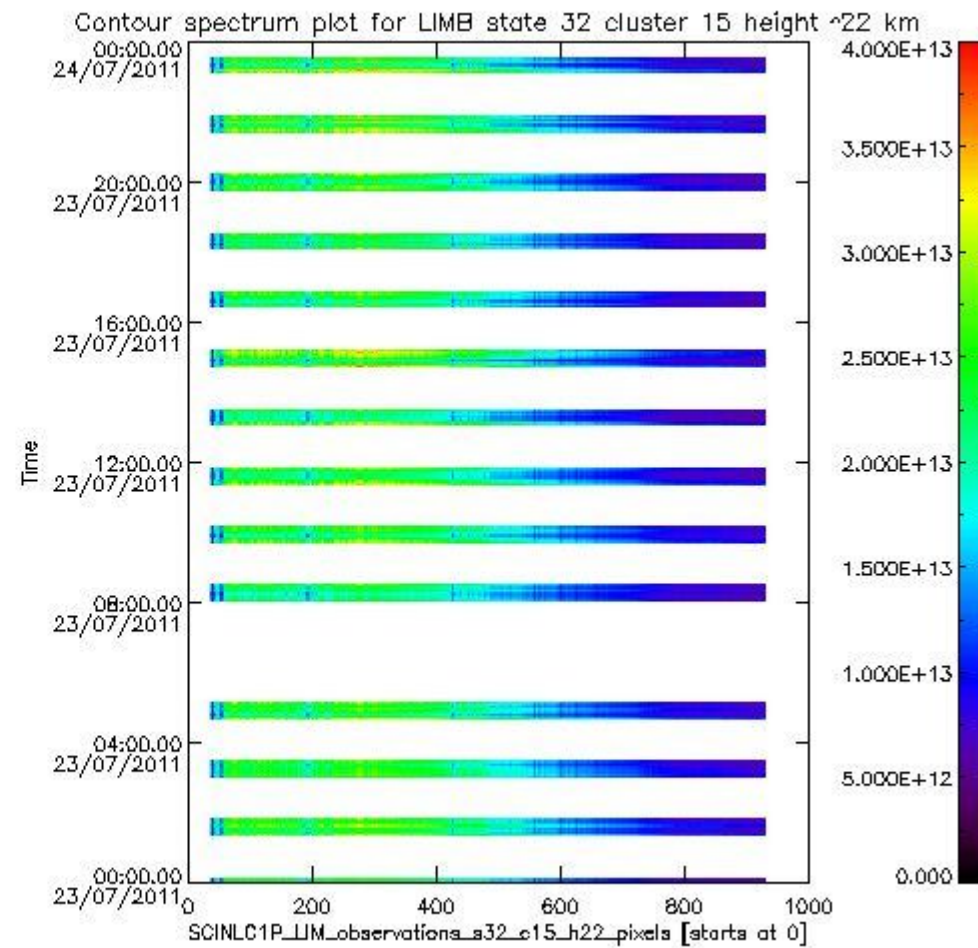
sciamachy_l1b_source_packet_report_SCIA_7_04_U_20110723_16.PNG
