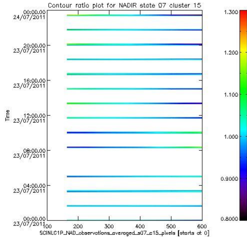
sciamachy_l1b_source_packet_report_SCIA_7_04_U_20110723_5.PNG
