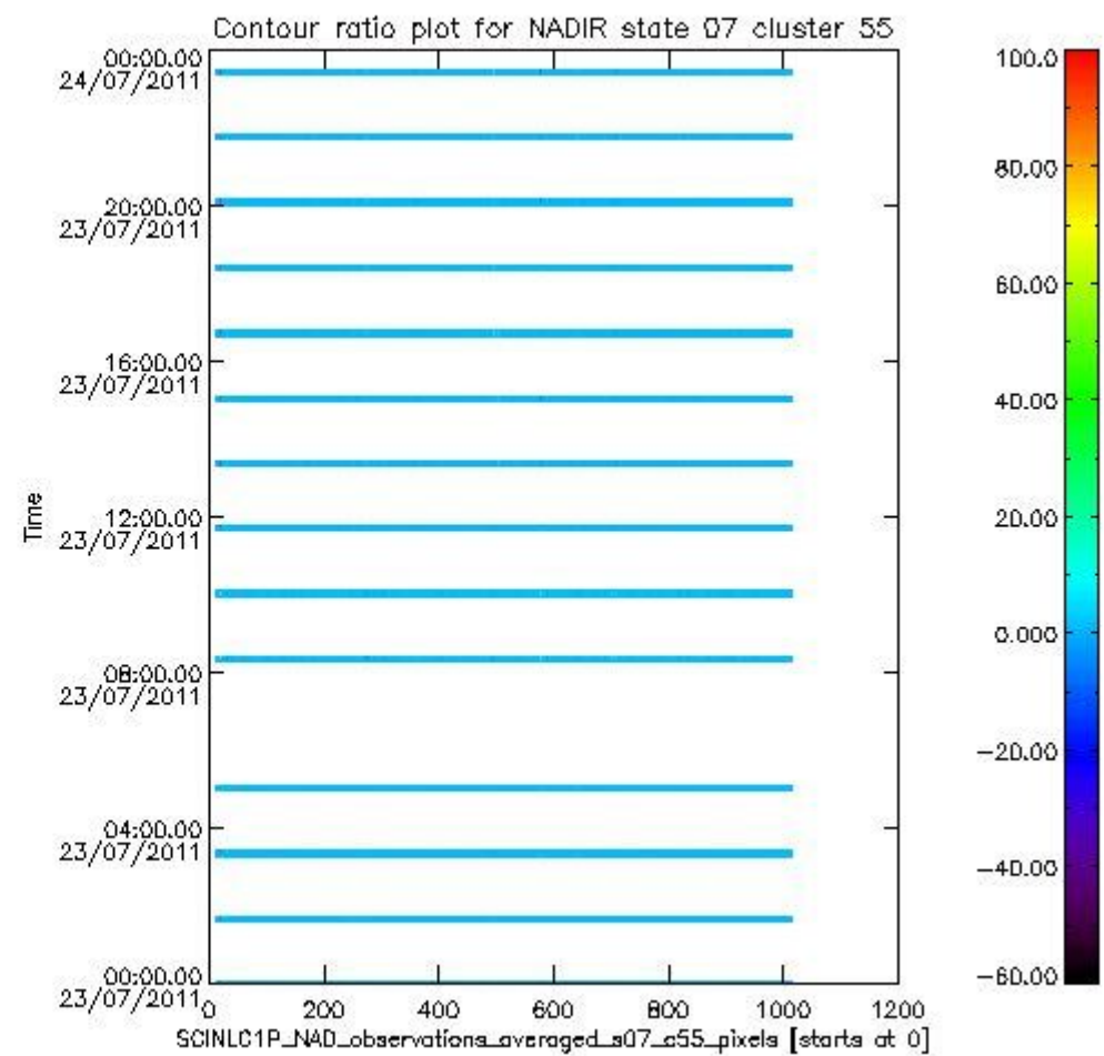
sciamachy_l1b_source_packet_report_SCIA_7_04_U_20110723_9.PNG
