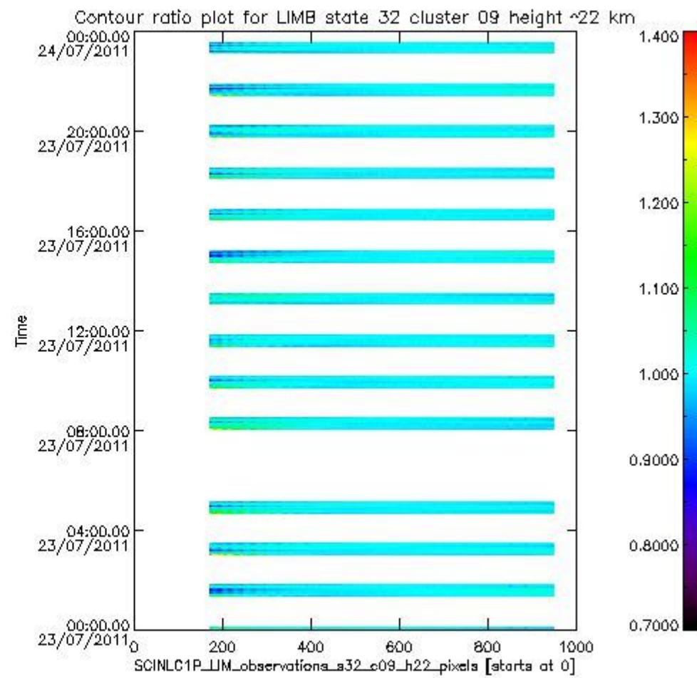
sciamachy_l1b_source_packet_report_SCIA_7_04_U_20110723_13.PNG
