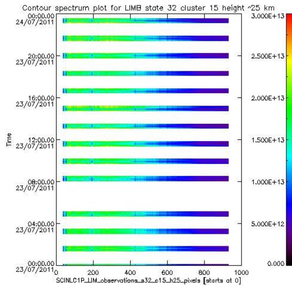
sciamachy_l1b_source_packet_report_SCIA_7_04_U_20110723_18.PNG
