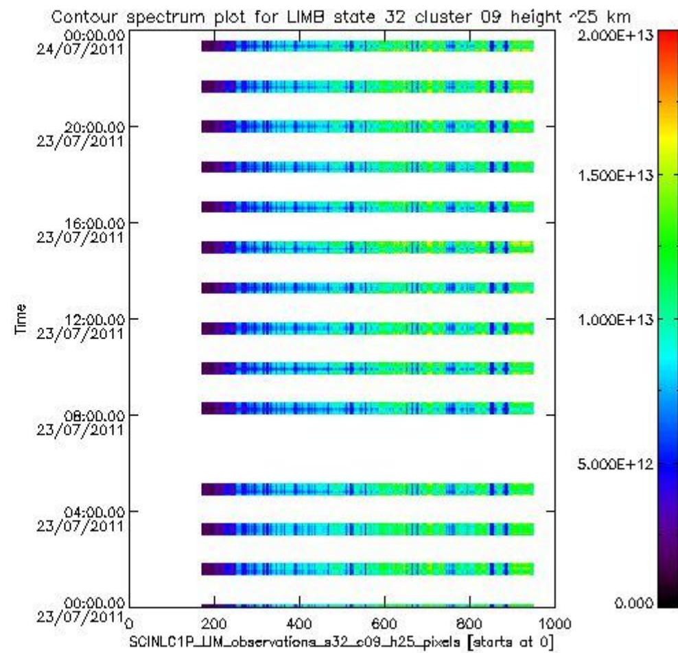
sciamachy_l1b_source_packet_report_SCIA_7_04_U_20110723_14.PNG
