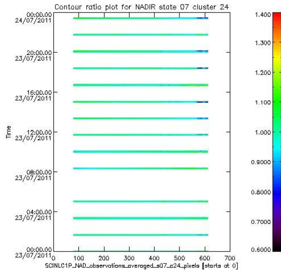
sciamachy_l1b_source_packet_report_SCIA_7_04_U_20110723_7.PNG
