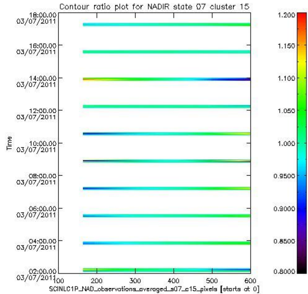
sciamachy_l1b_source_packet_report_SCIA_7_04_U_20110703_5.PNG
