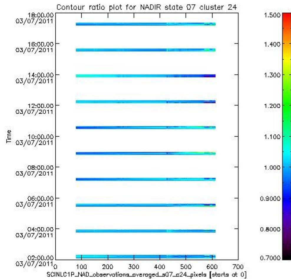
sciamachy_l1b_source_packet_report_SCIA_7_04_U_20110703_7.PNG
