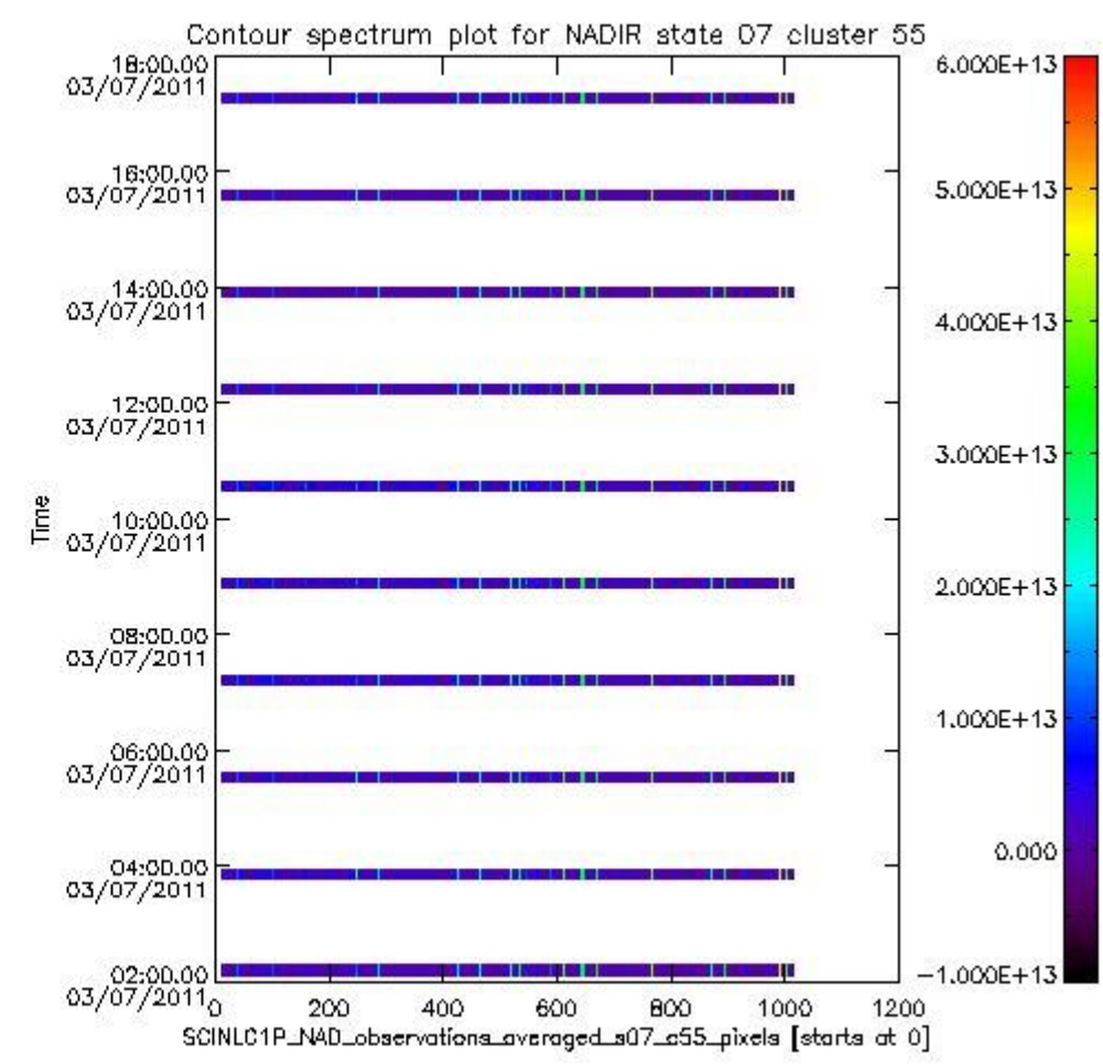
sciamachy_i1b_source_packet_report_SCIA_7_04_U_20110703_8.PNG
