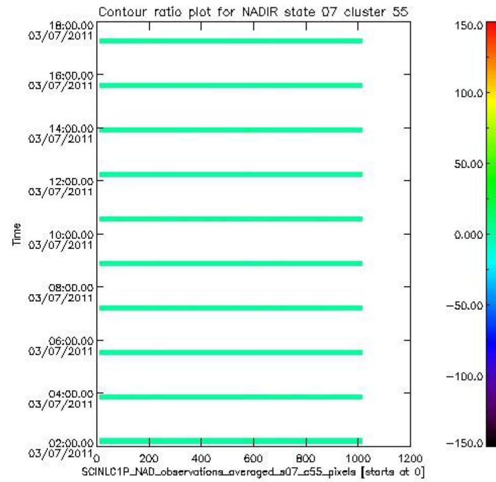
sciamachy_l1b_source_packet_report_SCIA_7_04_U_20110703_9.PNG
