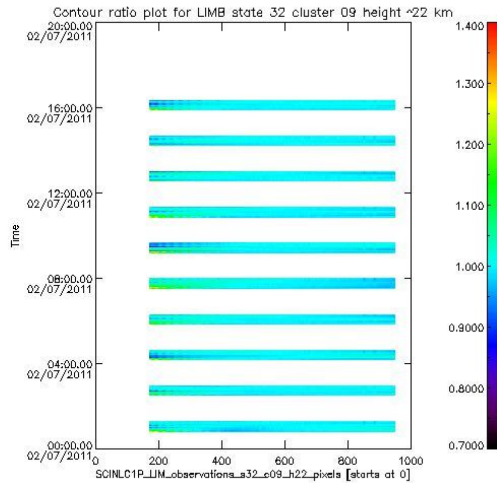
sciamachy_l1b_source_packet_report_SCIA_7_04_U_20110702_13.PNG
