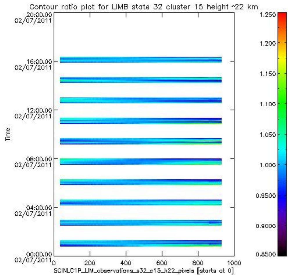
sciamachy_11b_source_packet_report_SCIA_7_04_U_20110702_17.PNG
