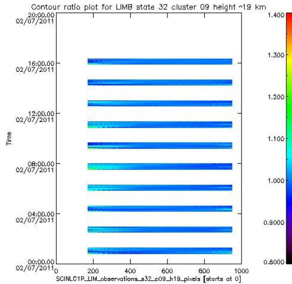
sciamachy_i1b_source_packet_report_SCIA_7_04_U_20110702_11.PNG
