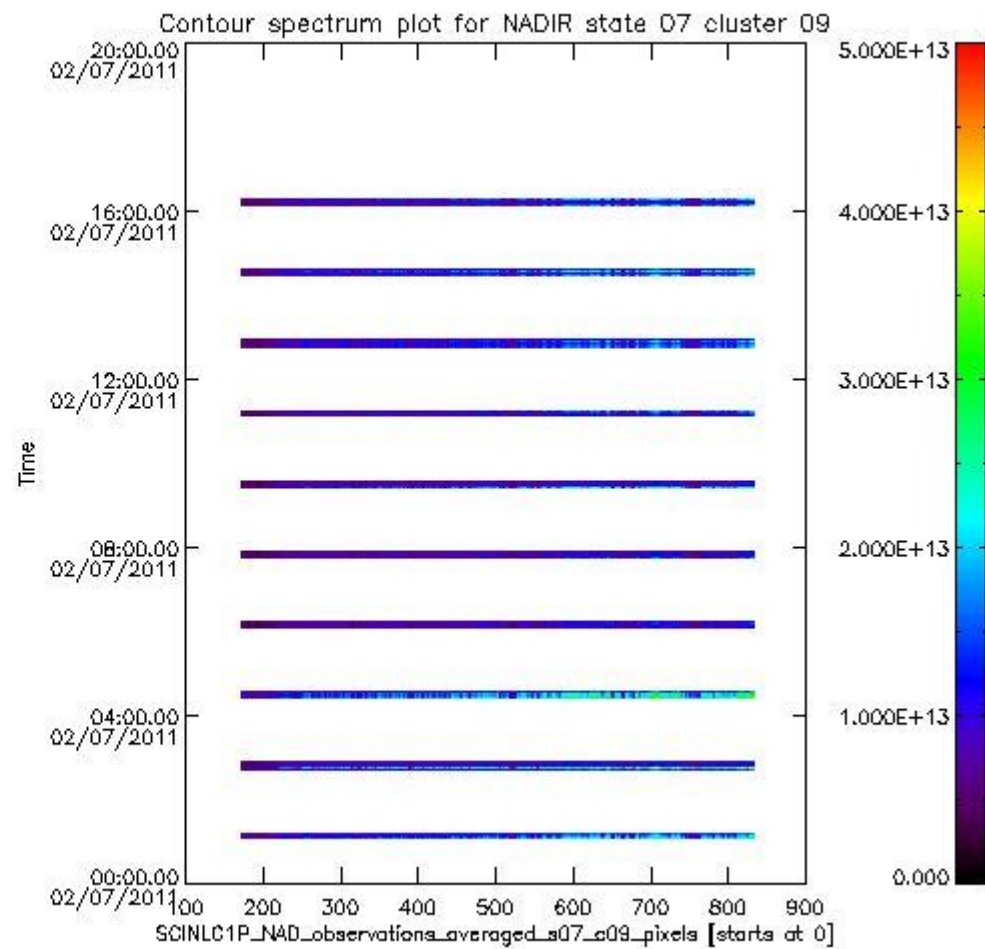
sciamachy_i1b_source_packet_report_SCIA_7_04_U_20110702_2.PNG
