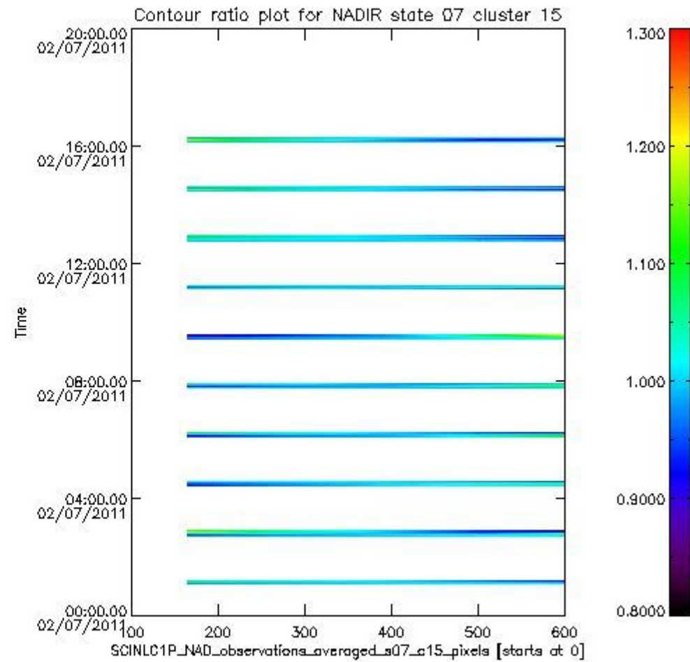
sciamachy_l1b_source_packet_report_SCIA_7_04_U_20110702_5.PNG
