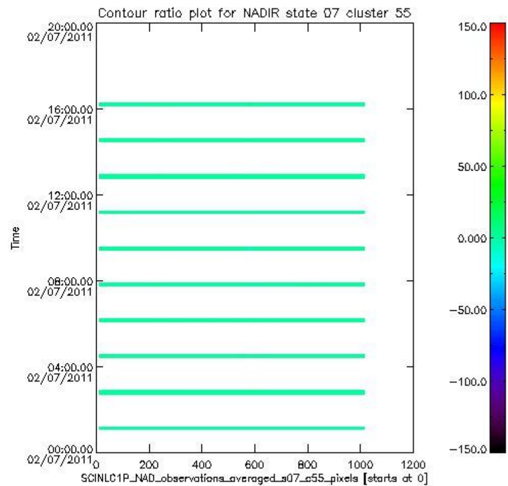
sciamachy_l1b_source_packet_report_SCIA_7_04_U_20110702_9.PNG
