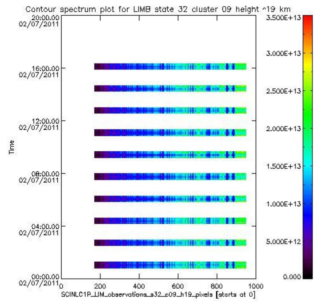
sciamachy_i1b_source_packet_report_SCIA_7_04_U_20110702_10.PNG
