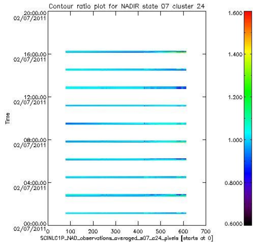
sciamachy_l1b_source_packet_report_SCIA_7_04_U_20110702_7.PNG
