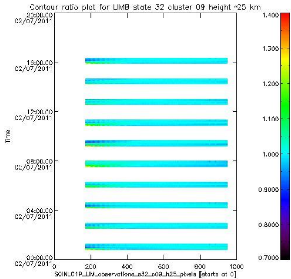
sciamachy_l1b_source_packet_report_SCIA_7_04_U_20110702_15.PNG
