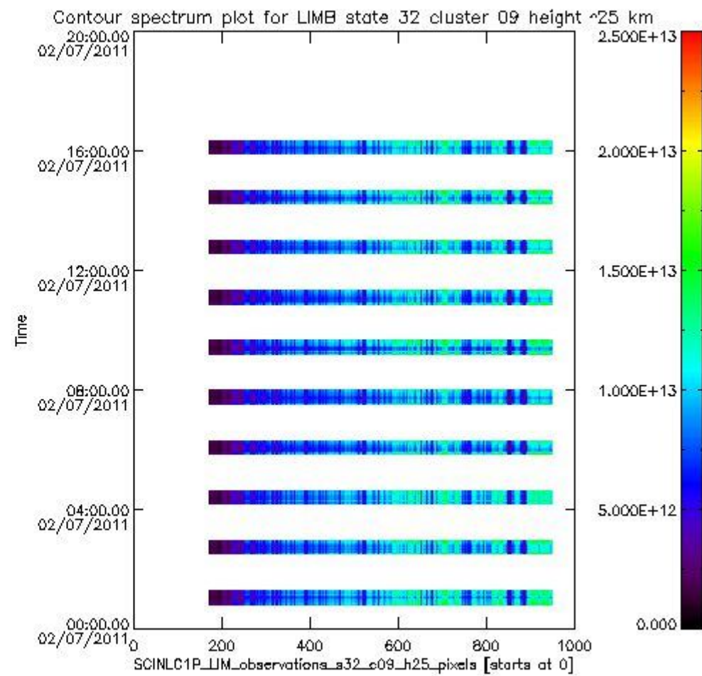
sciamachy_l1b_source_packet_report_SCIA_7_04_U_20110702_14.PNG
