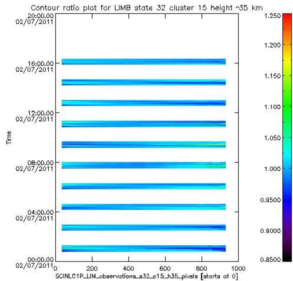
sciamachy_i1b_source_packet_report_SCIA_7_04_U_20110702_21.PNG
