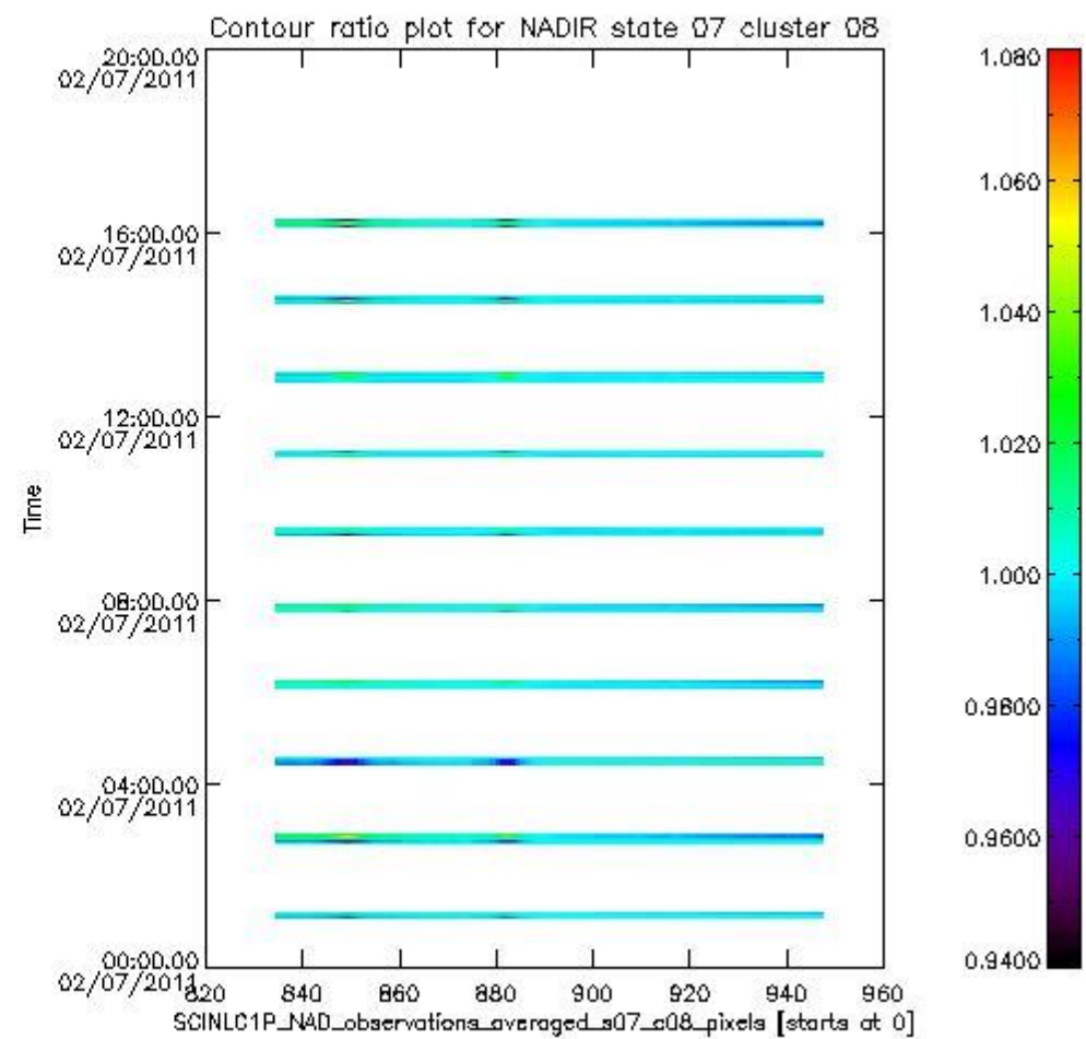
sciamachy_i1b_source_packet_report_SCIA_7_04_U_20110702_1.PNG
