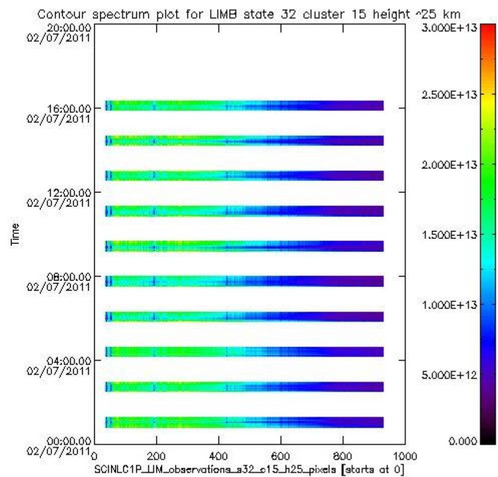
sciamachy_l1b_source_packet_report_SCIA_7_04_U_20110702_18.PNG
