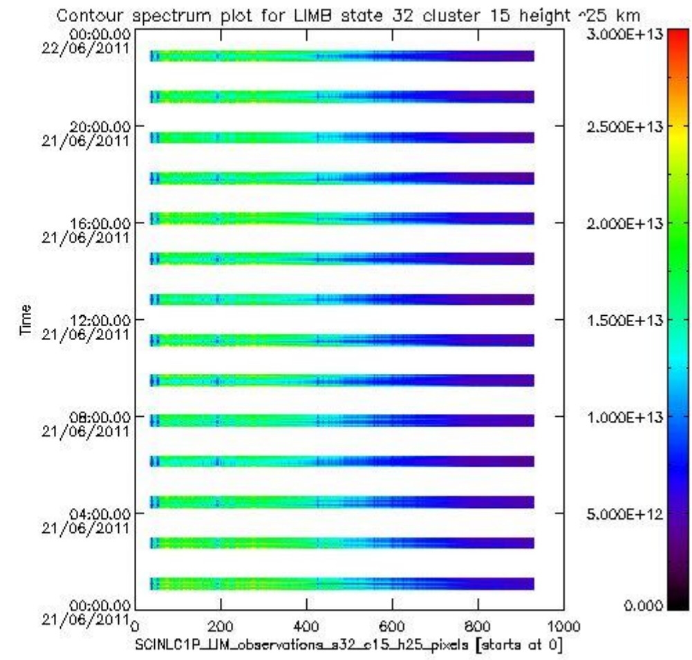
sciamachy_l1b_source_packet_report_SCIA_7_04_U_20110621_18.PNG
