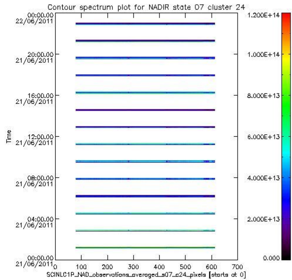
sciamachy_i1b_source_packet_report_SCIA_7_04_U_20110621_6.PNG
