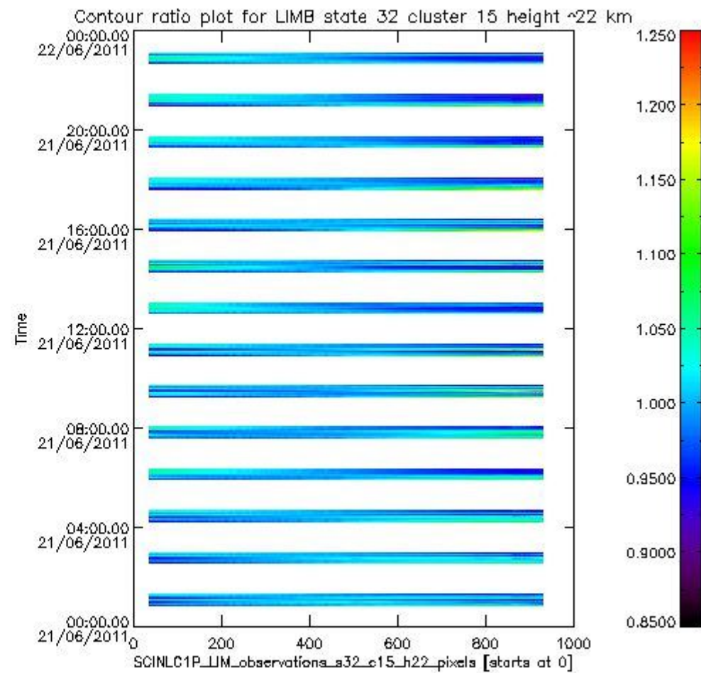
sciamachy_11b_source_packet_report_SCIA_7_04_U_20110621_17.PNG
