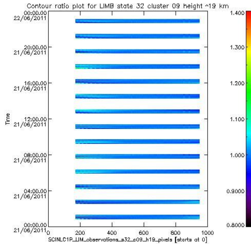
sciamachy_i1b_source_packet_report_SCIA_7_04_U_20110621_11.PNG
