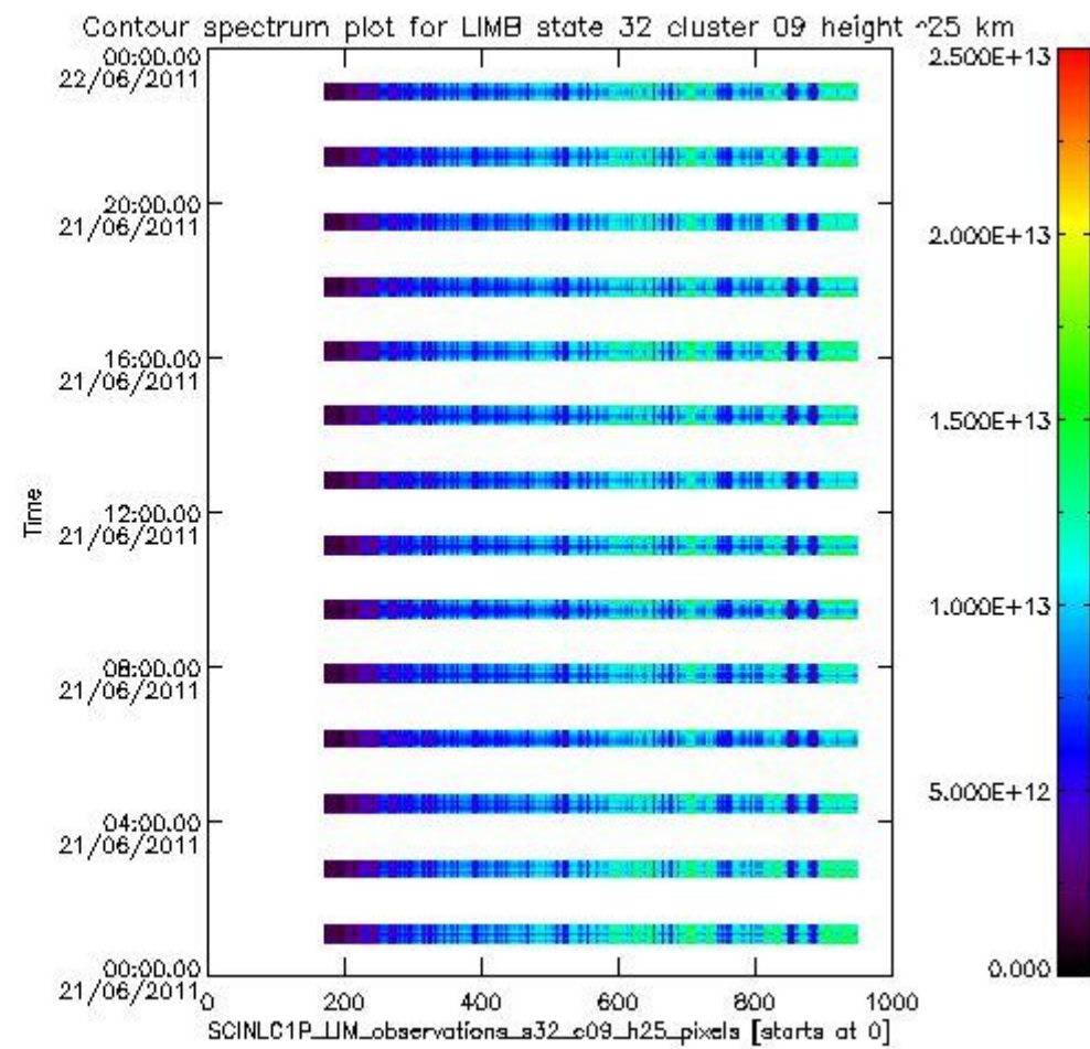
sciamachy_l1b_source_packet_report_SCIA_7_04_U_20110621_14.PNG
