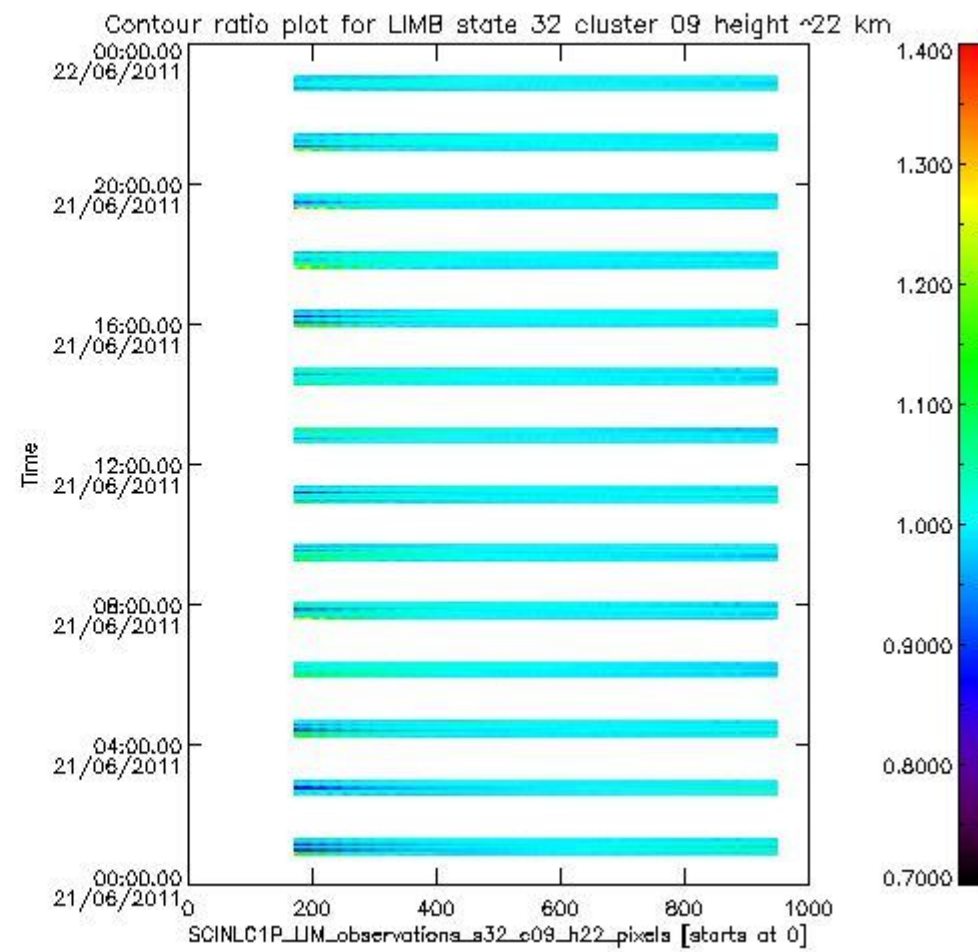
sciamachy_l1b_source_packet_report_SCIA_7_04_U_20110621_13.PNG
