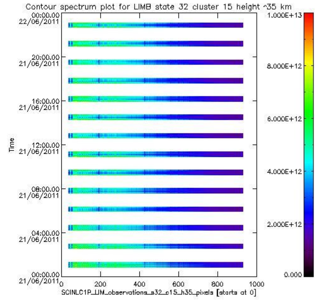
sciamachy_11b_source_packet_report_SCIA_7_04_U_20110621_20.PNG
