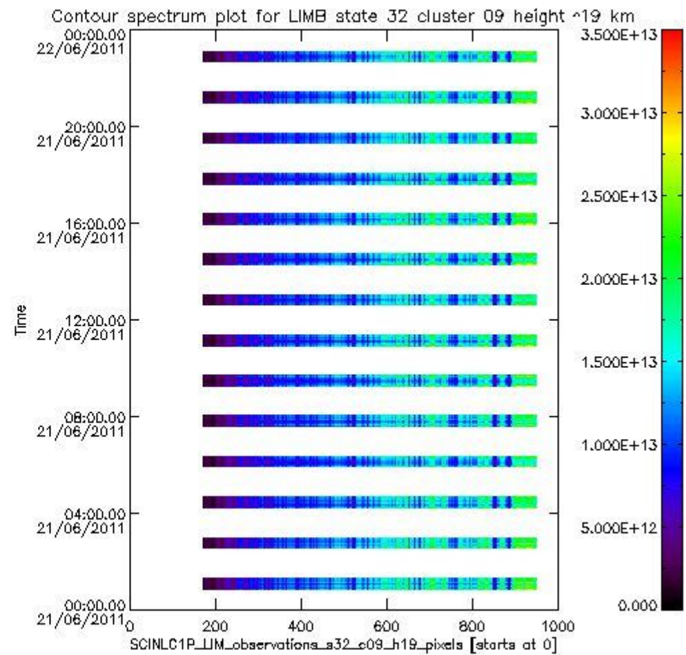
sciamachy_l1b_source_packet_report_SCIA_7_04_U_20110621_10.PNG
