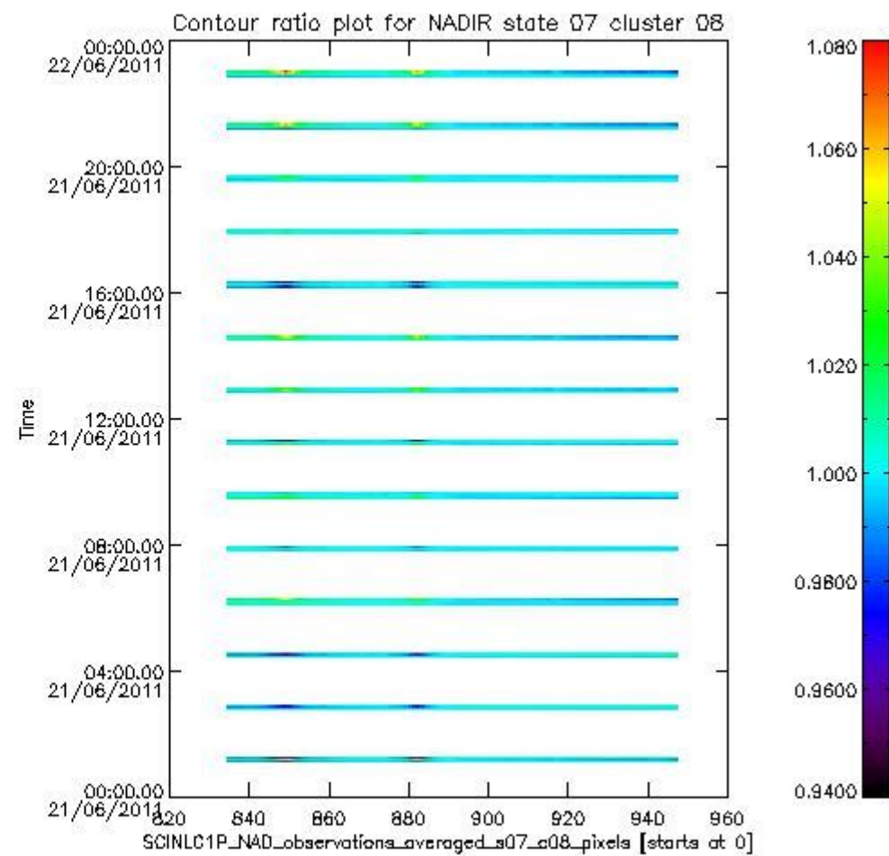
sciamachy_l1b_source_packet_report_SCIA_7_04_U_20110621_1.PNG
