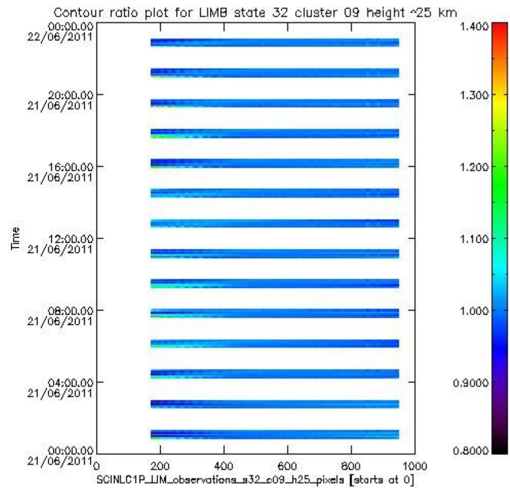
sciamachy_l1b_source_packet_report_SCIA_7_04_U_20110621_15.PNG
