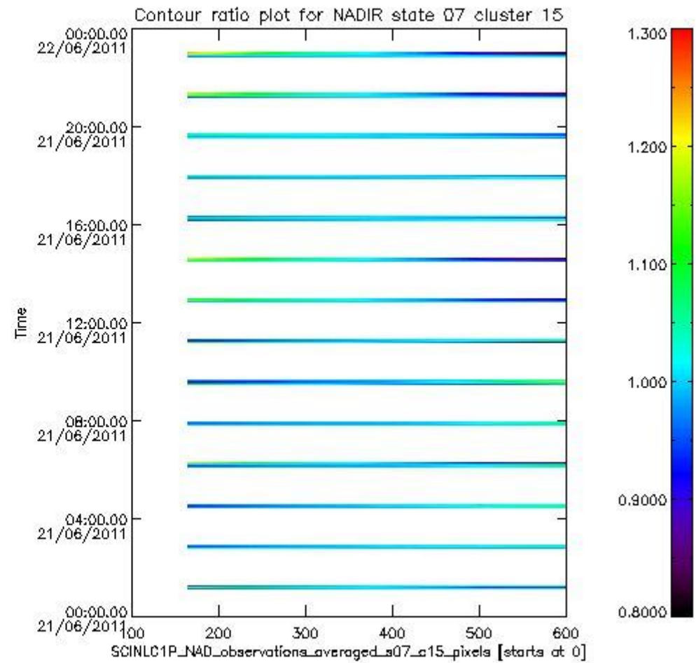
sciamachy_l1b_source_packet_report_SCIA_7_04_U_20110621_5.PNG
