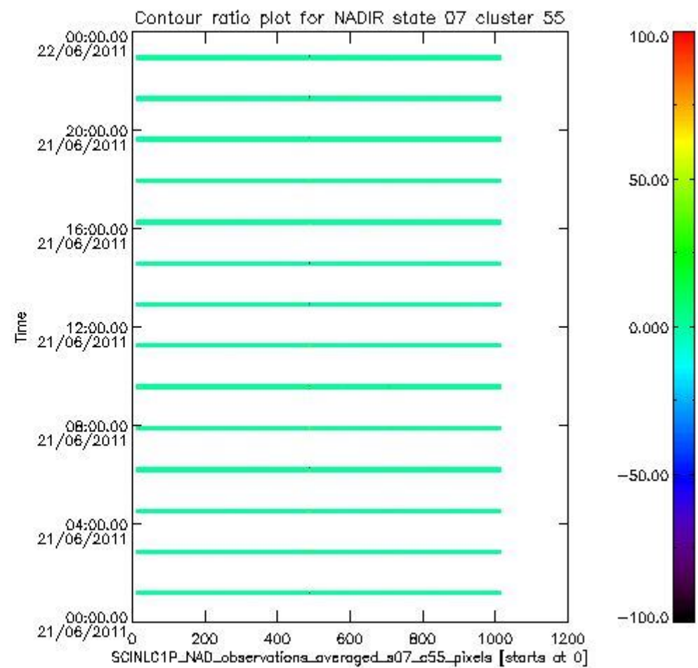
sciamachy_l1b_source_packet_report_SCIA_7_04_U_20110621_9.PNG
