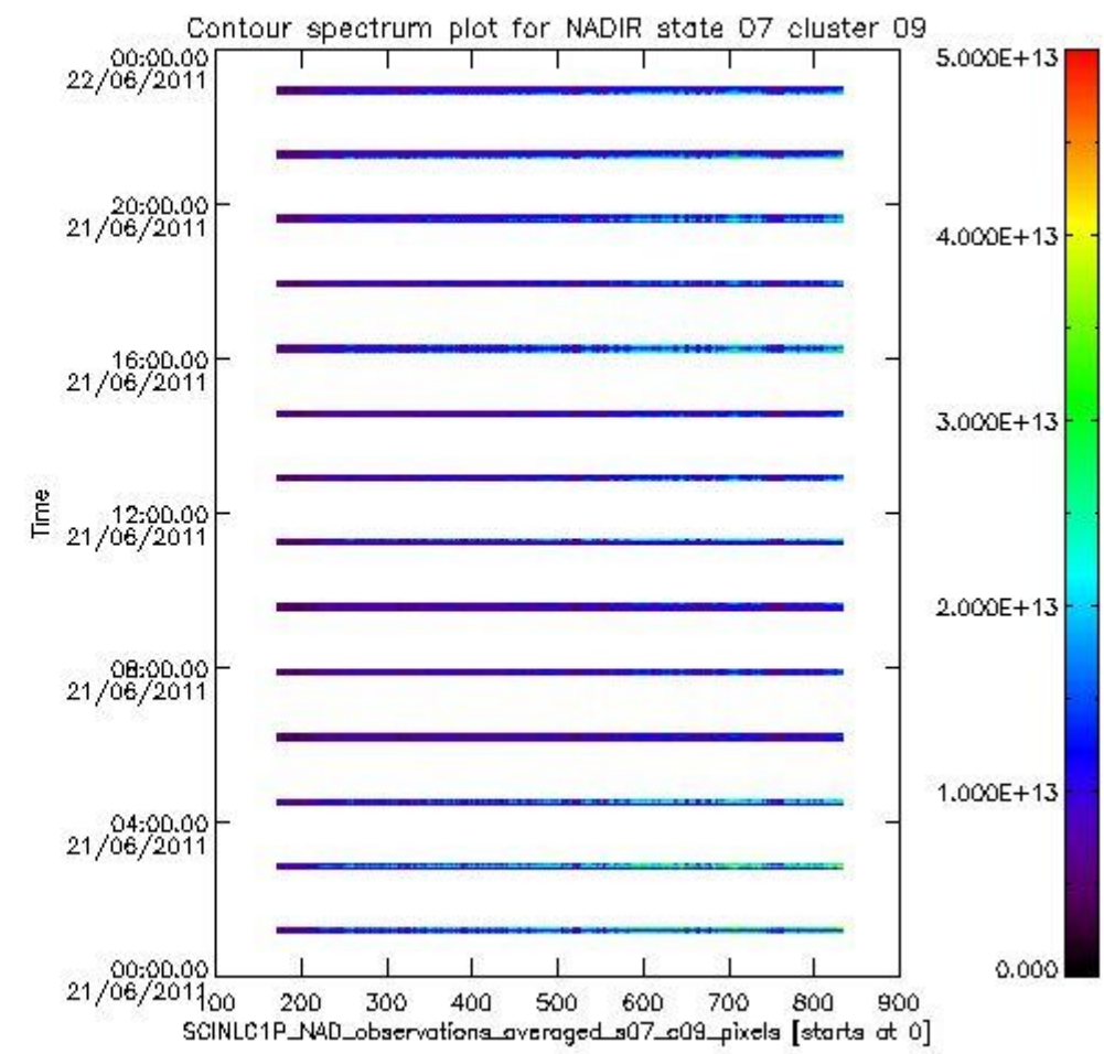
sciamachy_i1b_source_packet_report_SCIA_7_04_U_20110621_2.PNG
