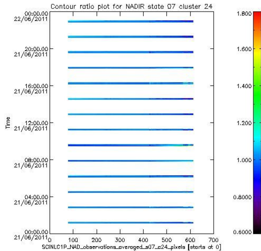
sciamachy_l1b_source_packet_report_SCIA_7_04_U_20110621_7.PNG
