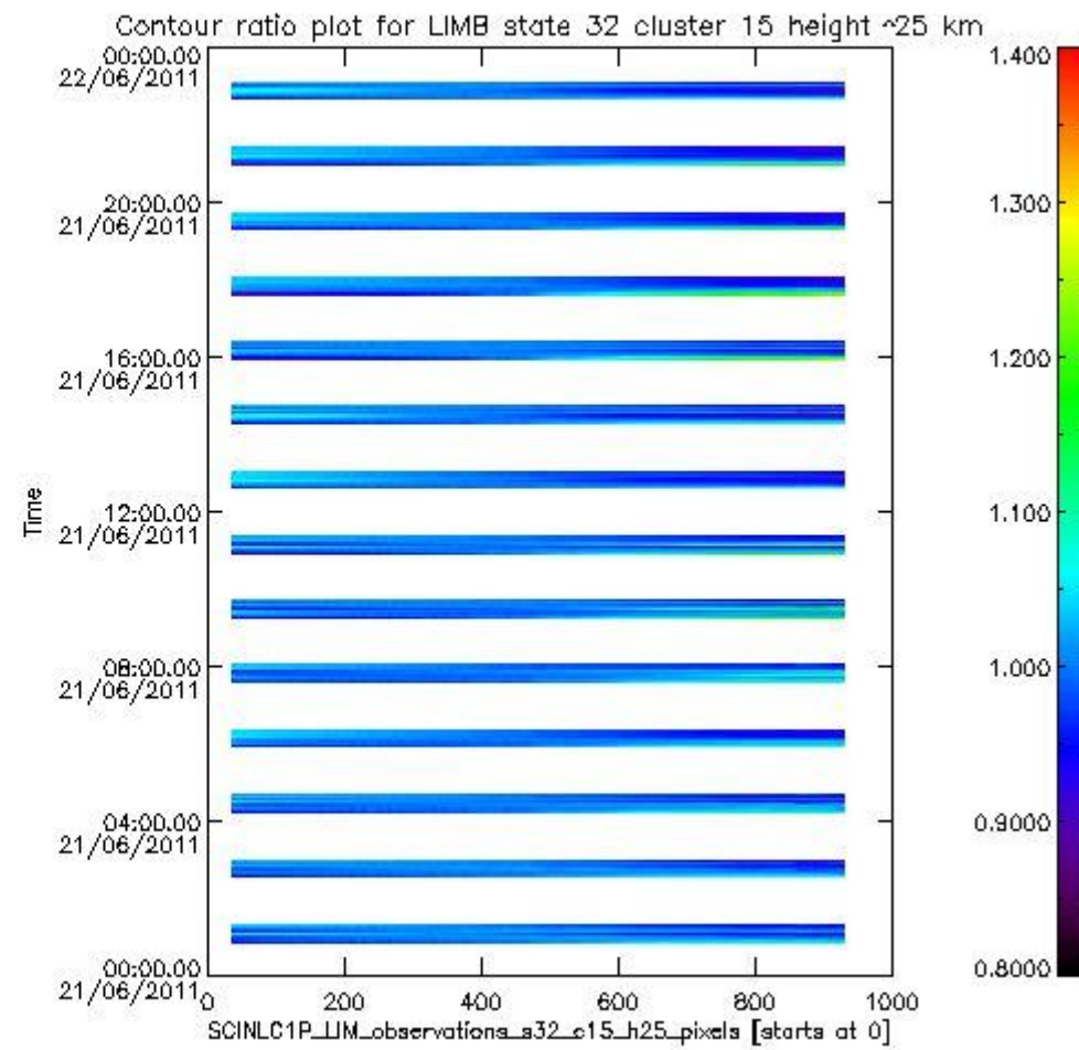
sciamachy_11b_source_packet_report_SCIA_7_04_U_20110621_19.PNG
