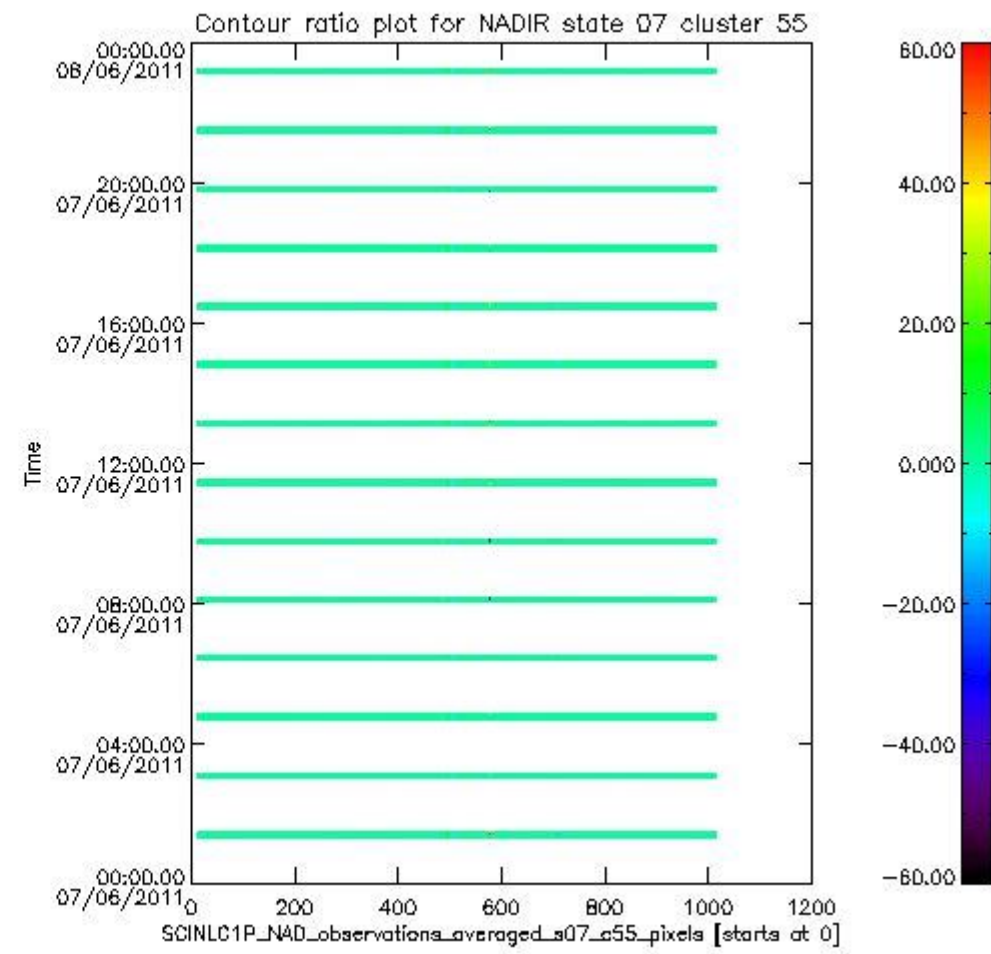
sciamachy_l1b_source_packet_report_SCIA_7_04_U_20110607_9.PNG
