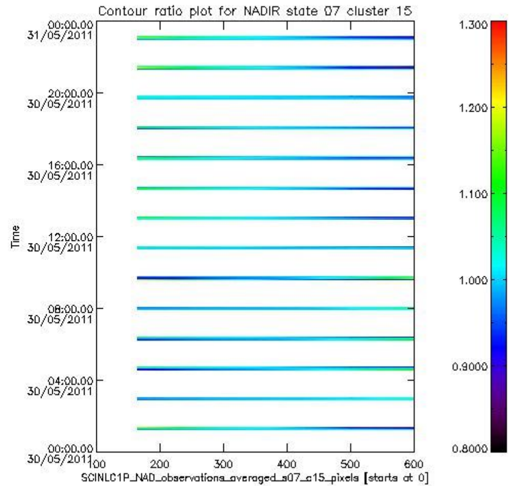
sciamachy_l1b_source_packet_report_SCIA_7_04_U_20110530_5.PNG
