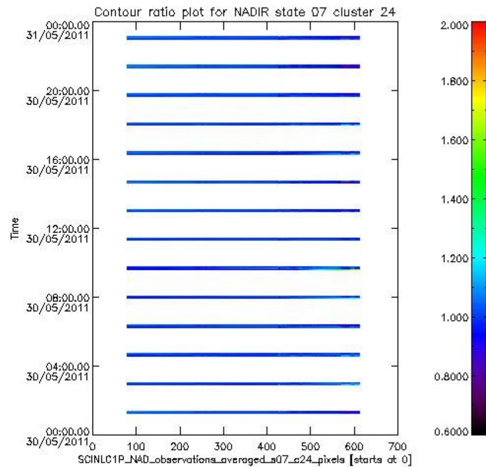
sciamachy_l1b_source_packet_report_SCIA_7_04_U_20110530_7.PNG
