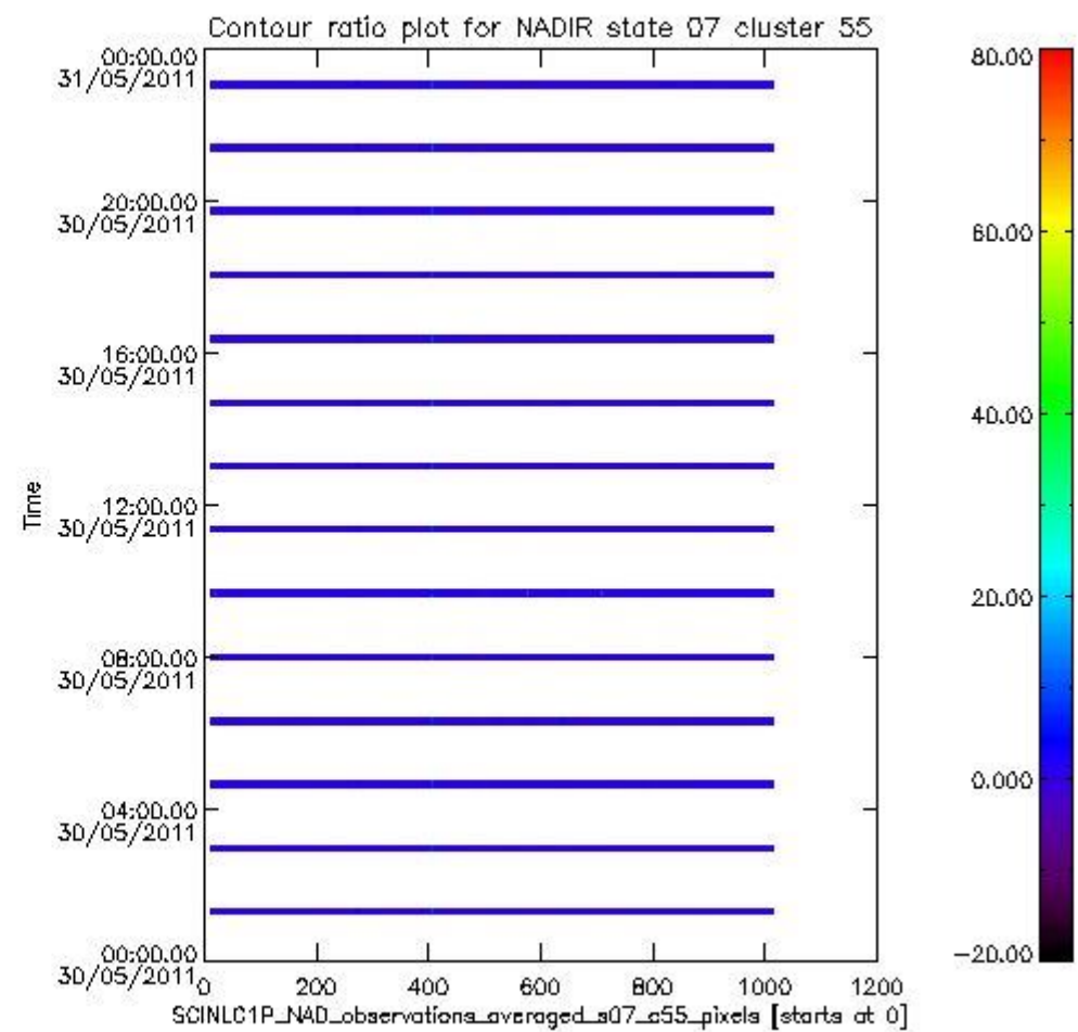
sciamachy_l1b_source_packet_report_SCIA_7_04_U_20110530_9.PNG
