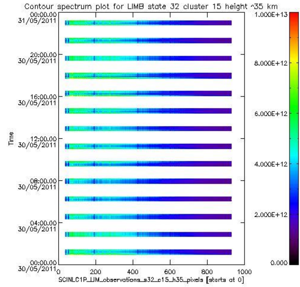
sciamachy_11b_source_packet_report_SCIA_7_04_U_20110530_20.PNG
