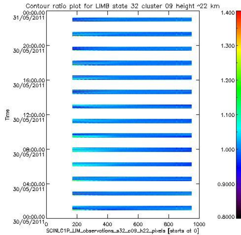
sciamachy_l1b_source_packet_report_SCIA_7_04_U_20110530_13.PNG
