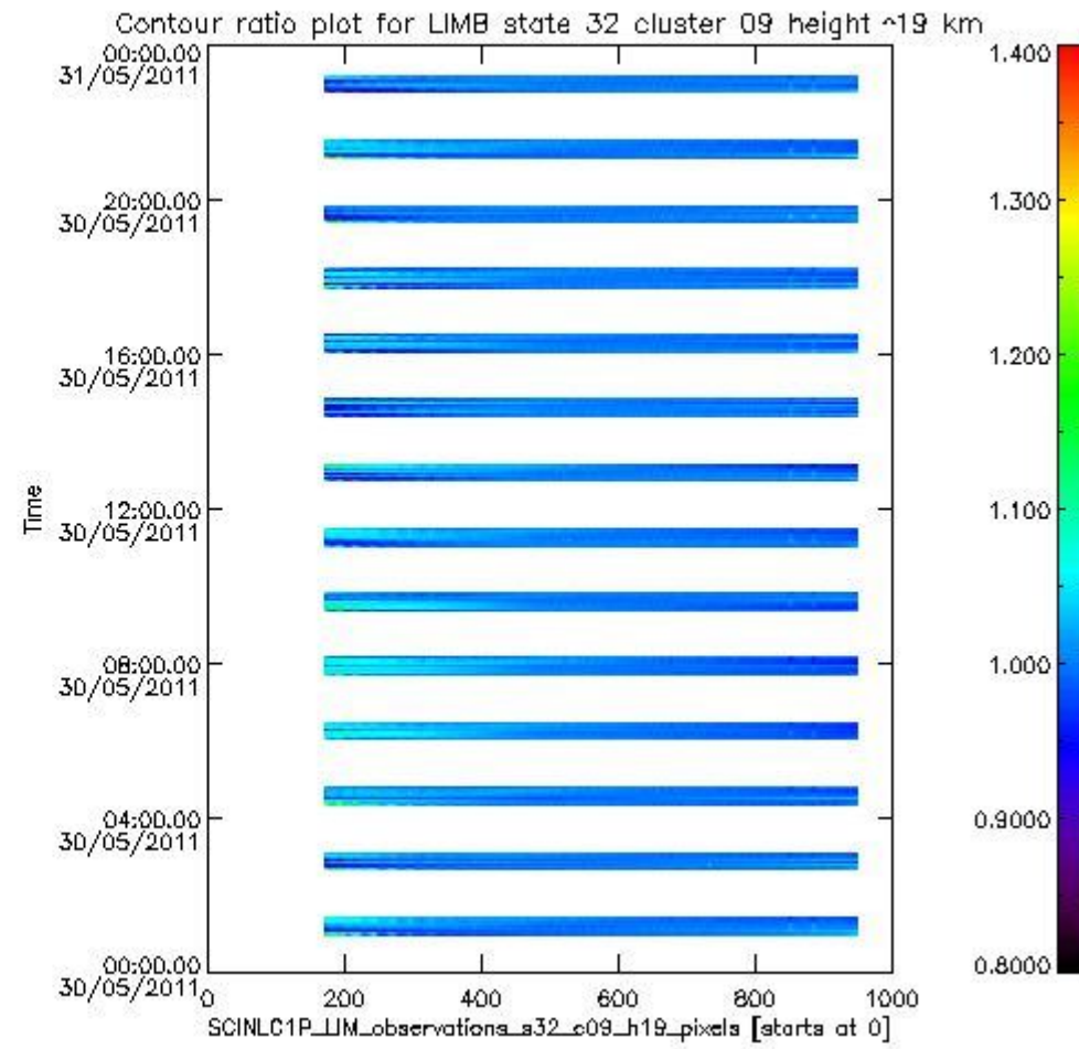
sciamachy_l1b_source_packet_report_SCIA_7_04_U_20110530_11.PNG
