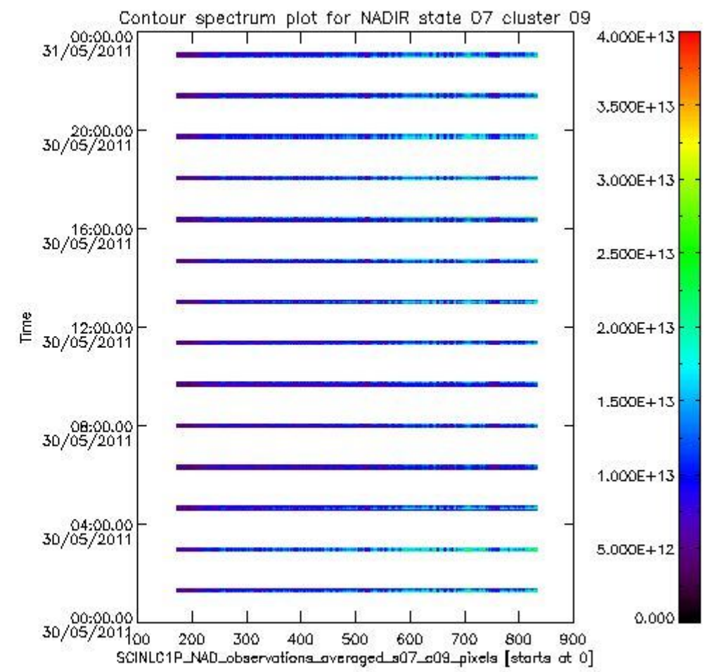
sciamachy_i1b_source_packet_report_SCIA_7_04_U_20110530_2.PNG
