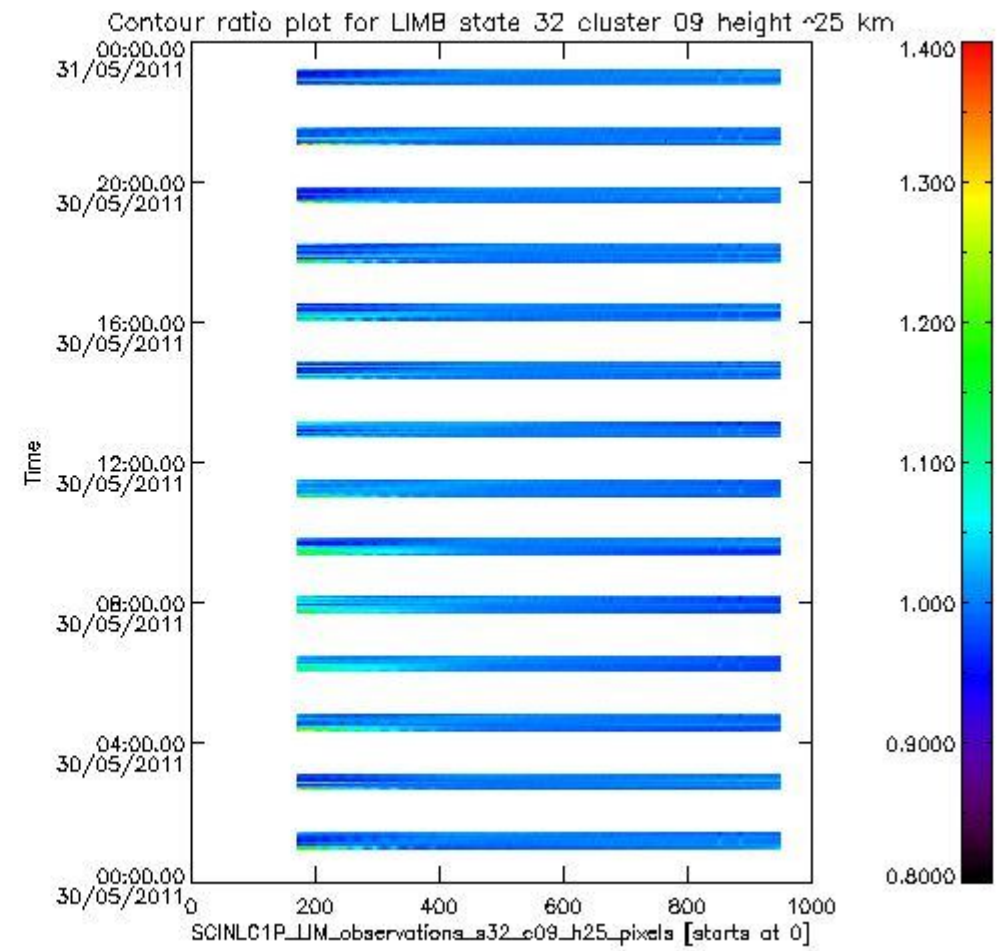
sciamachy_l1b_source_packet_report_SCIA_7_04_U_20110530_15.PNG
