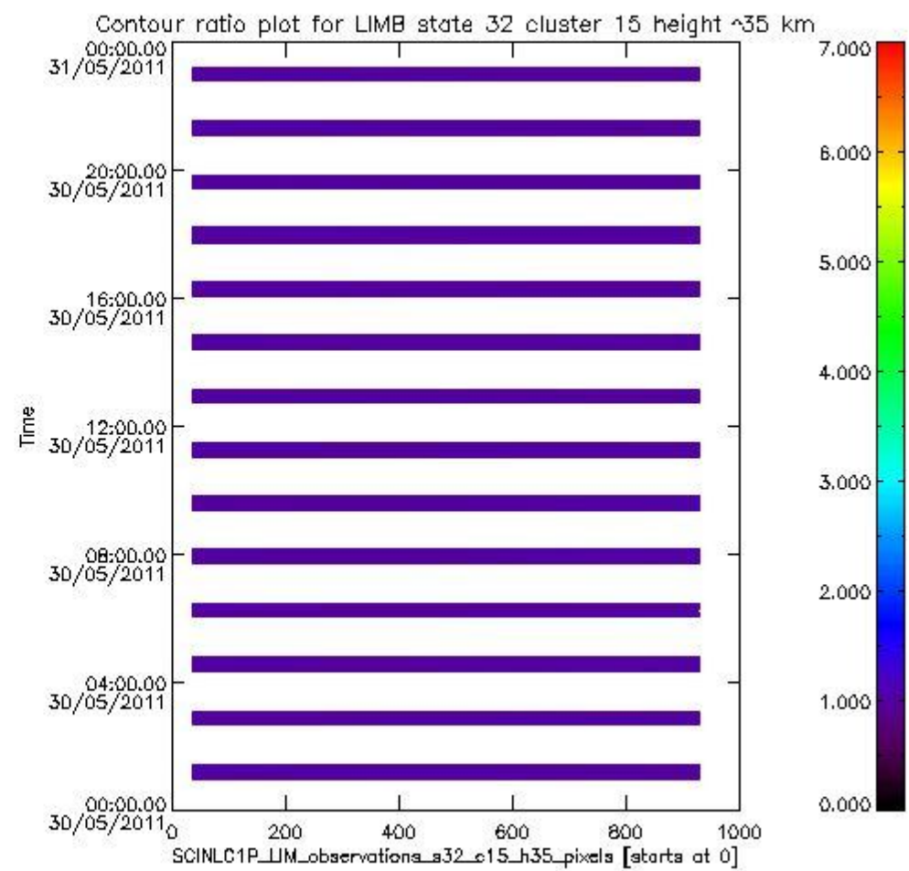
sciamachy_11b_source_packet_report_SCIA_7_04_U_20110530_21.PNG
