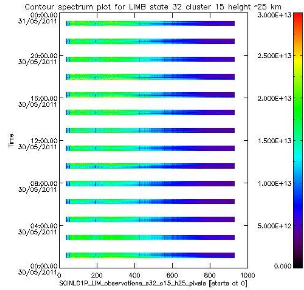
sciamachy_l1b_source_packet_report_SCIA_7_04_U_20110530_18.PNG
