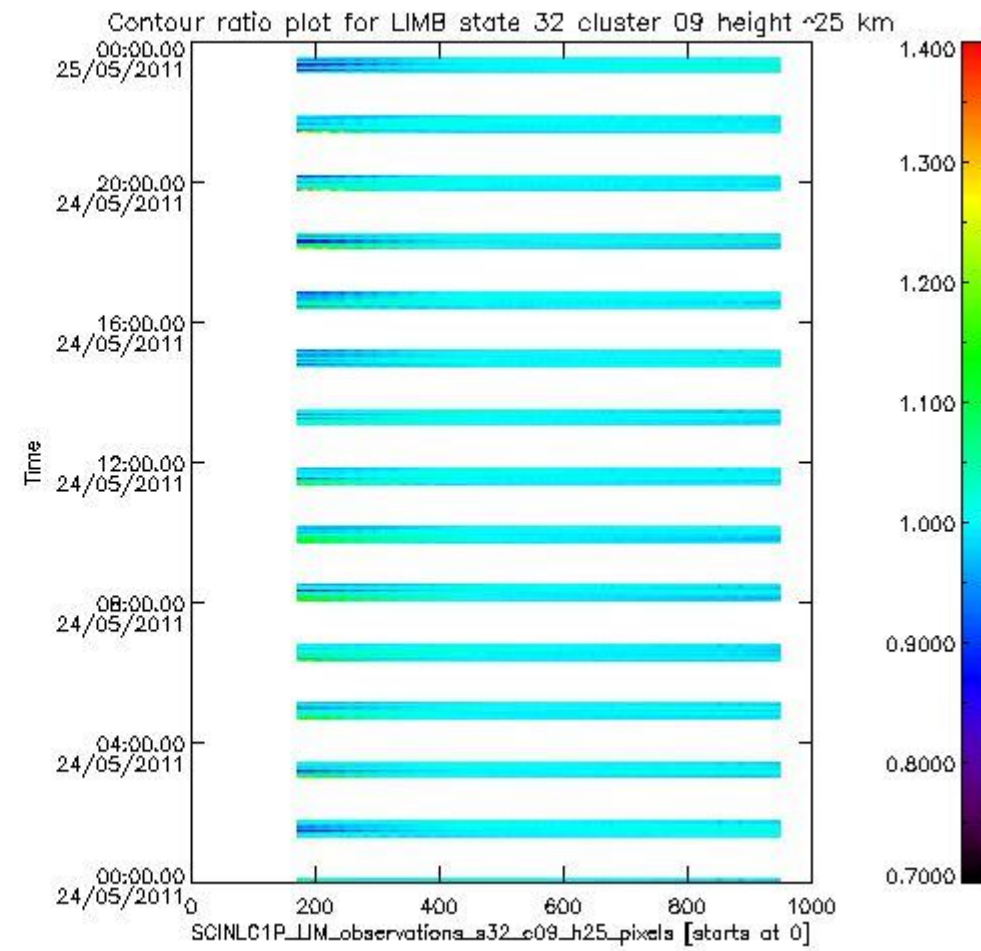
sciamachy_l1b_source_packet_report_SCIA_7_04_U_20110524_15.PNG
