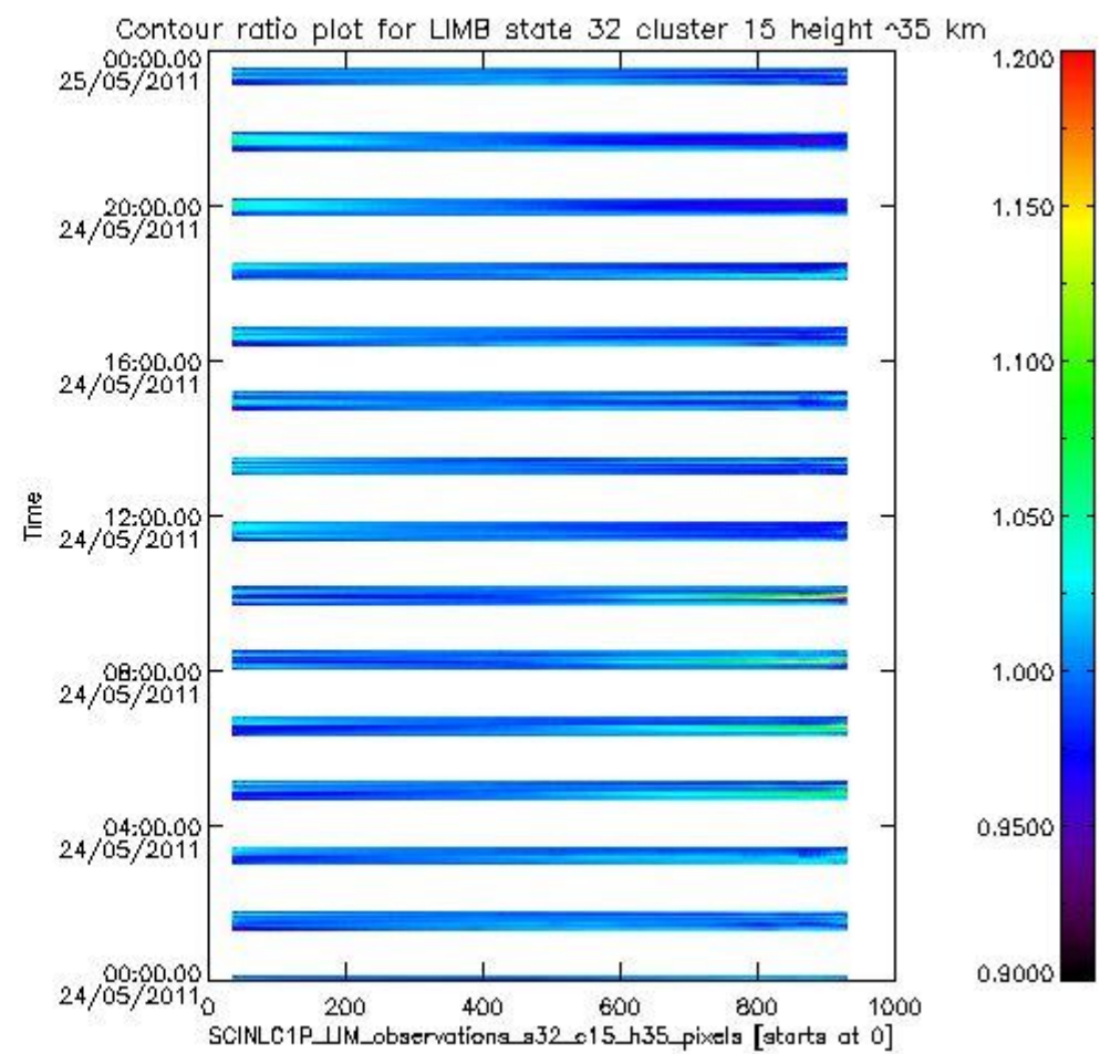
sciamachy_i1b_source_packet_report_SCIA_7_04_U_20110524_21.PNG
