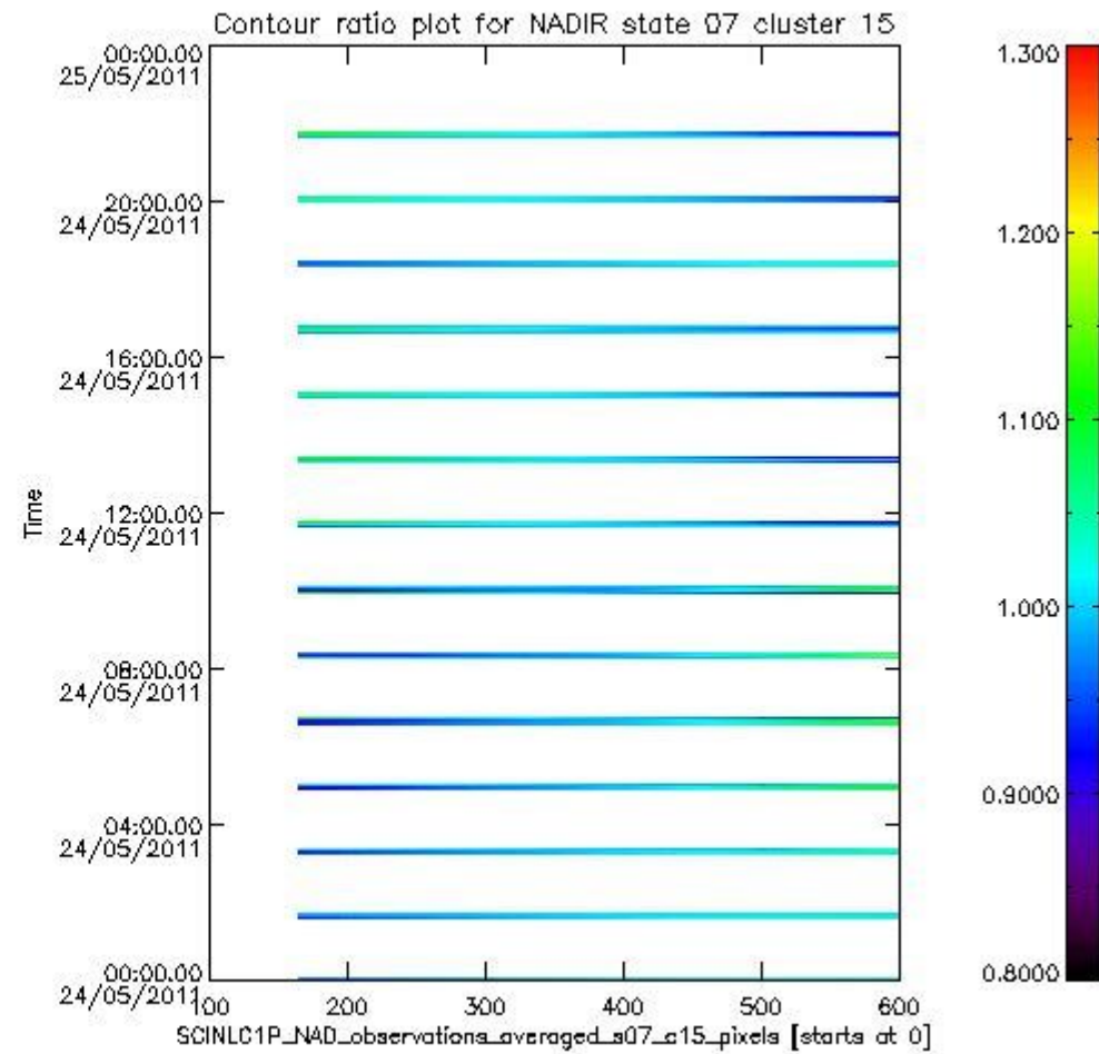
sciamachy_l1b_source_packet_report_SCIA_7_04_U_20110524_5.PNG
