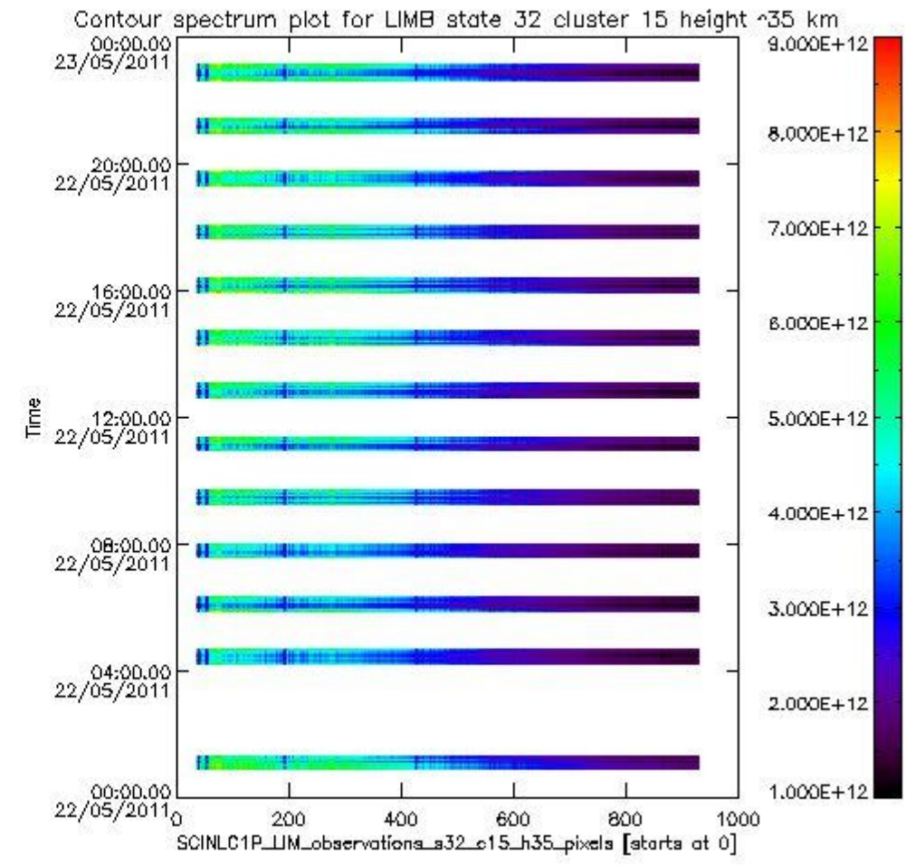
sciamachy_11b_source_packet_report_SCIA_7_04_U_20110522_20.PNG
