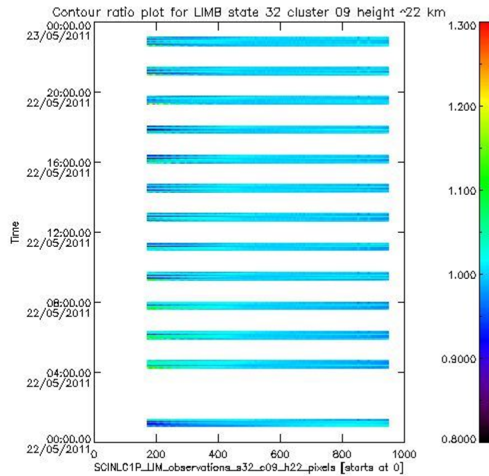
sciamachy_l1b_source_packet_report_SCIA_7_04_U_20110522_13.PNG
