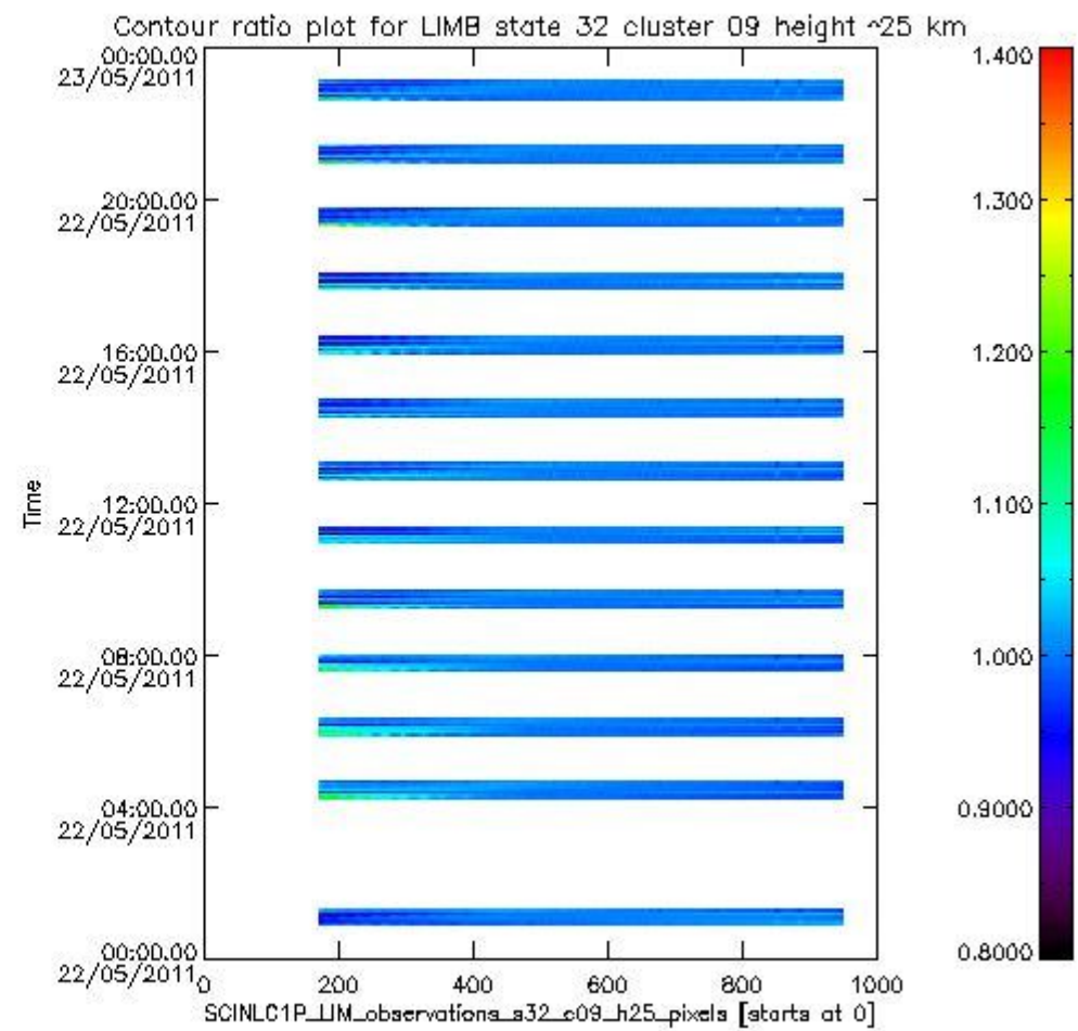
sciamachy_l1b_source_packet_report_SCIA_7_04_U_20110522_15.PNG
