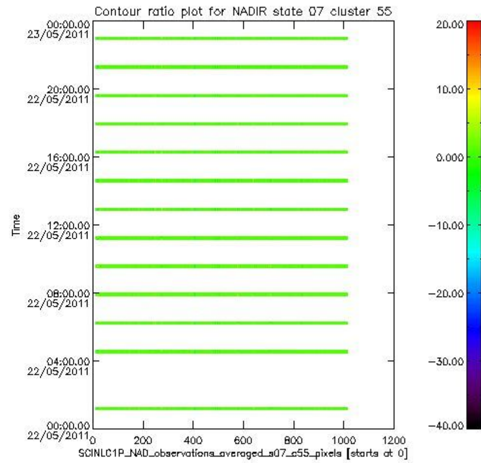
sciamachy_l1b_source_packet_report_SCIA_7_04_U_20110522_9.PNG
