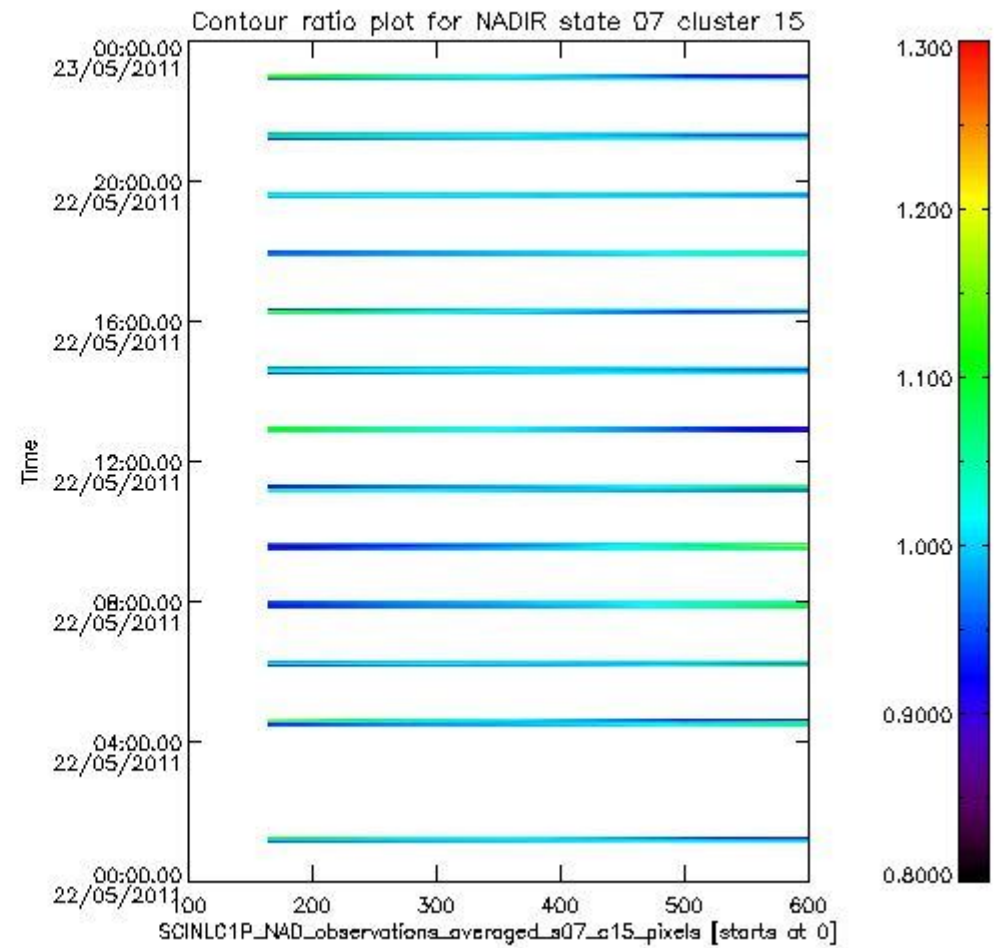
sciamachy_l1b_source_packet_report_SCIA_7_04_U_20110522_5.PNG
