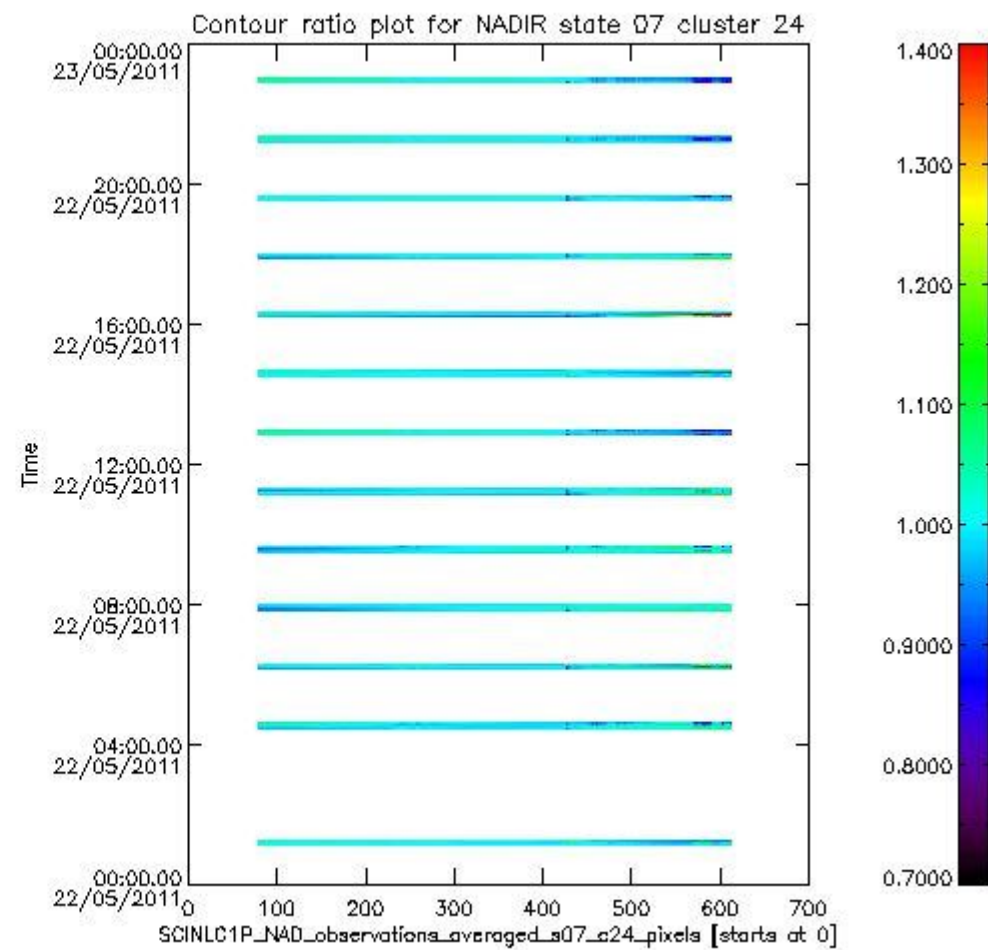
sciamachy_l1b_source_packet_report_SCIA_7_04_U_20110522_7.PNG
