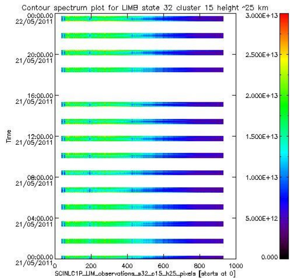
sciamachy_l1b_source_packet_report_SCIA_7_04_U_20110521_18.PNG
