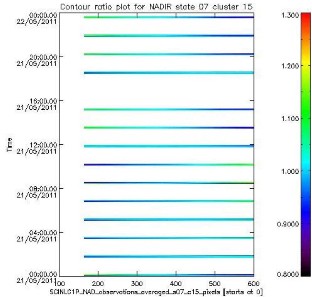
sciamachy_l1b_source_packet_report_SCIA_7_04_U_20110521_5.PNG
