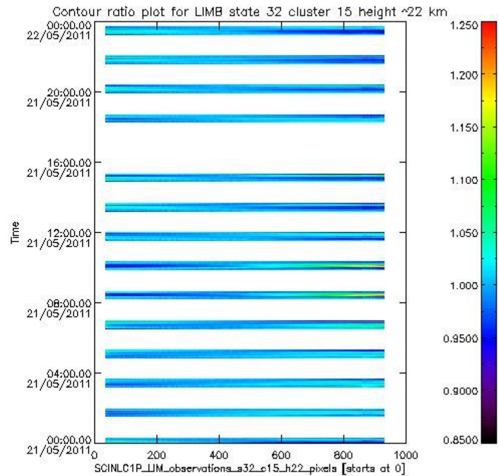
sciamachy_11b_source_packet_report_SCIA_7_04_U_20110521_17.PNG
