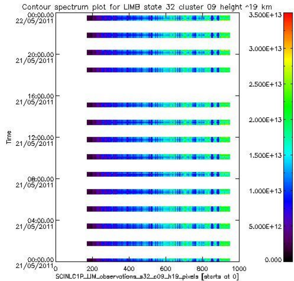
sciamachy_l1b_source_packet_report_SCIA_7_04_U_20110521_10.PNG
