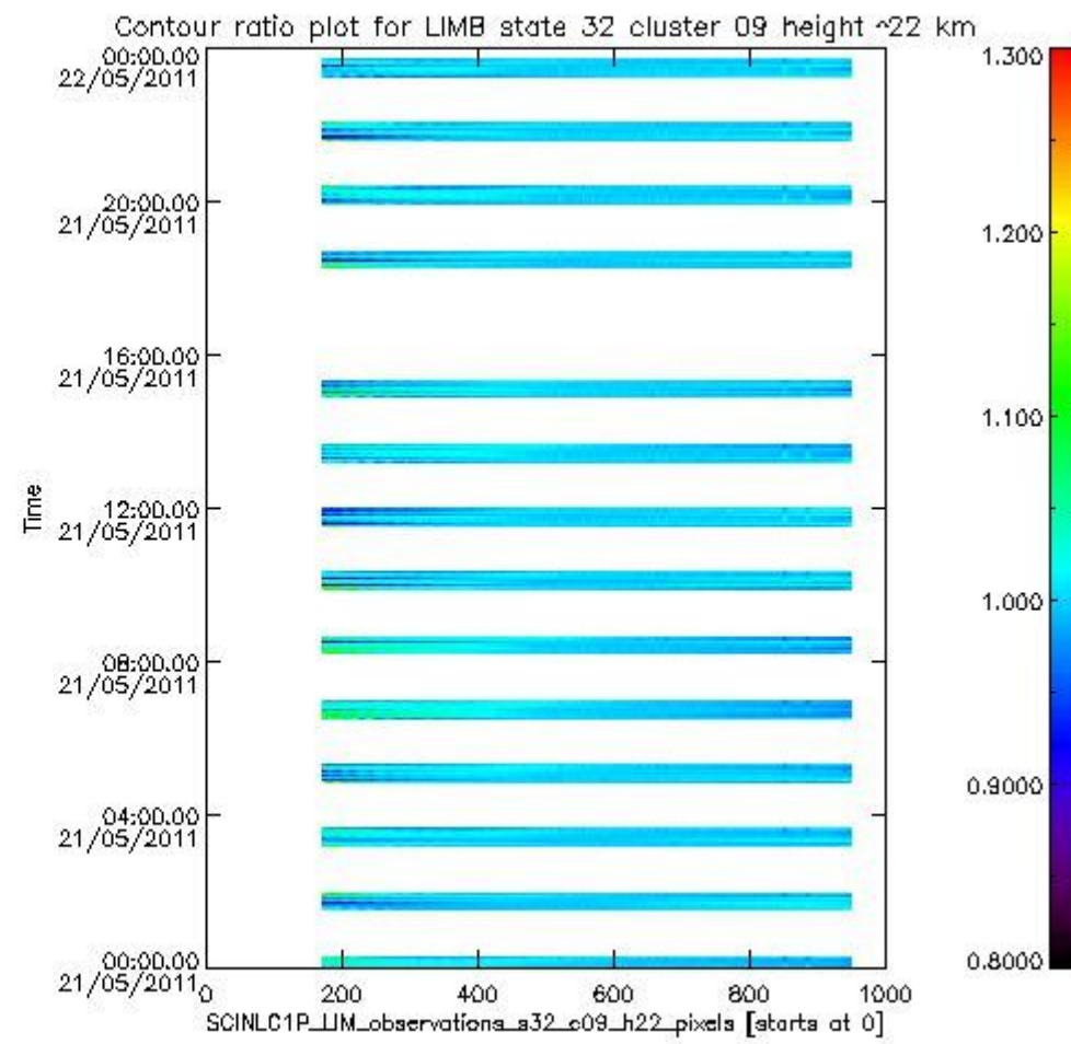
sciamachy_l1b_source_packet_report_SCIA_7_04_U_20110521_13.PNG
