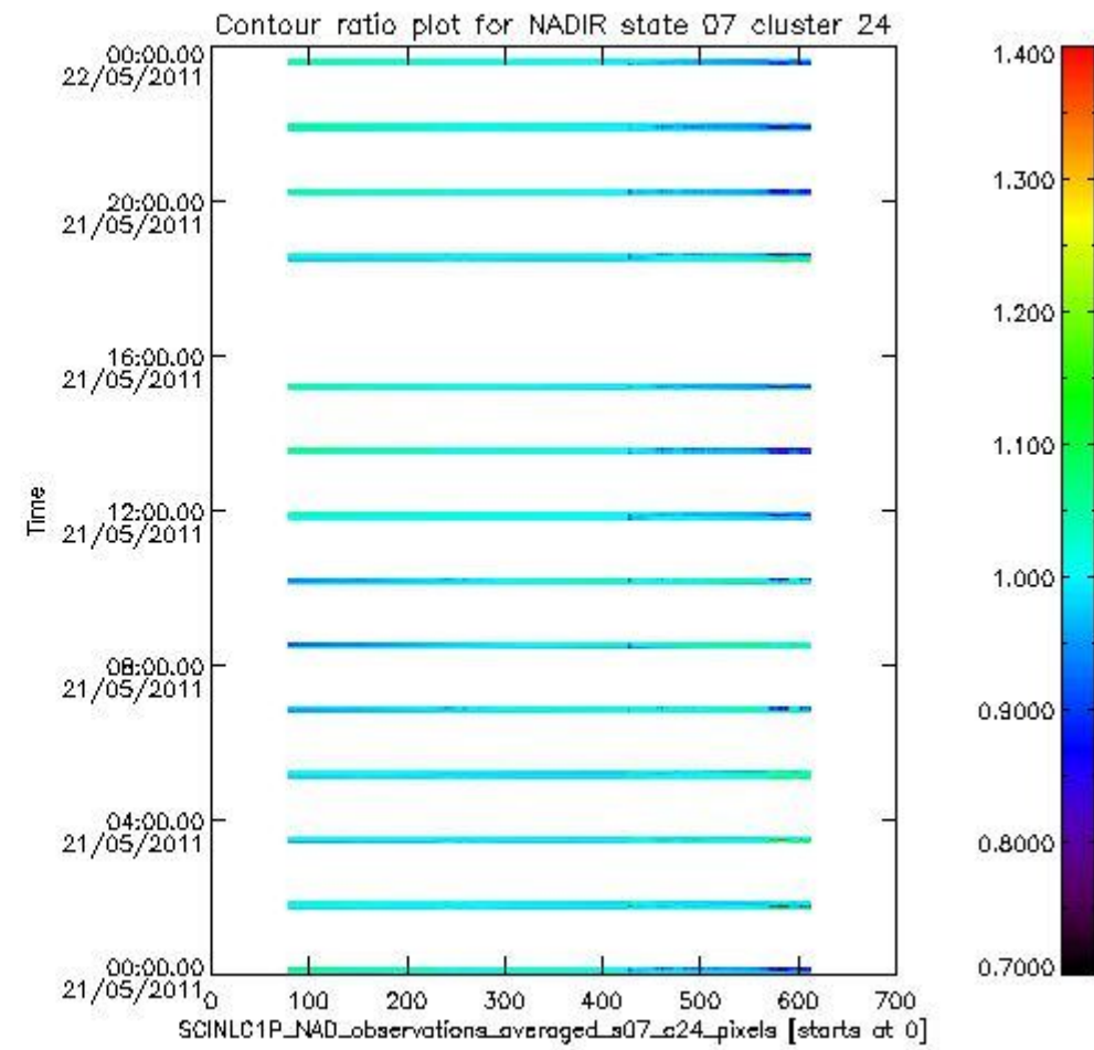
sciamachy_l1b_source_packet_report_SCIA_7_04_U_20110521_7.PNG
