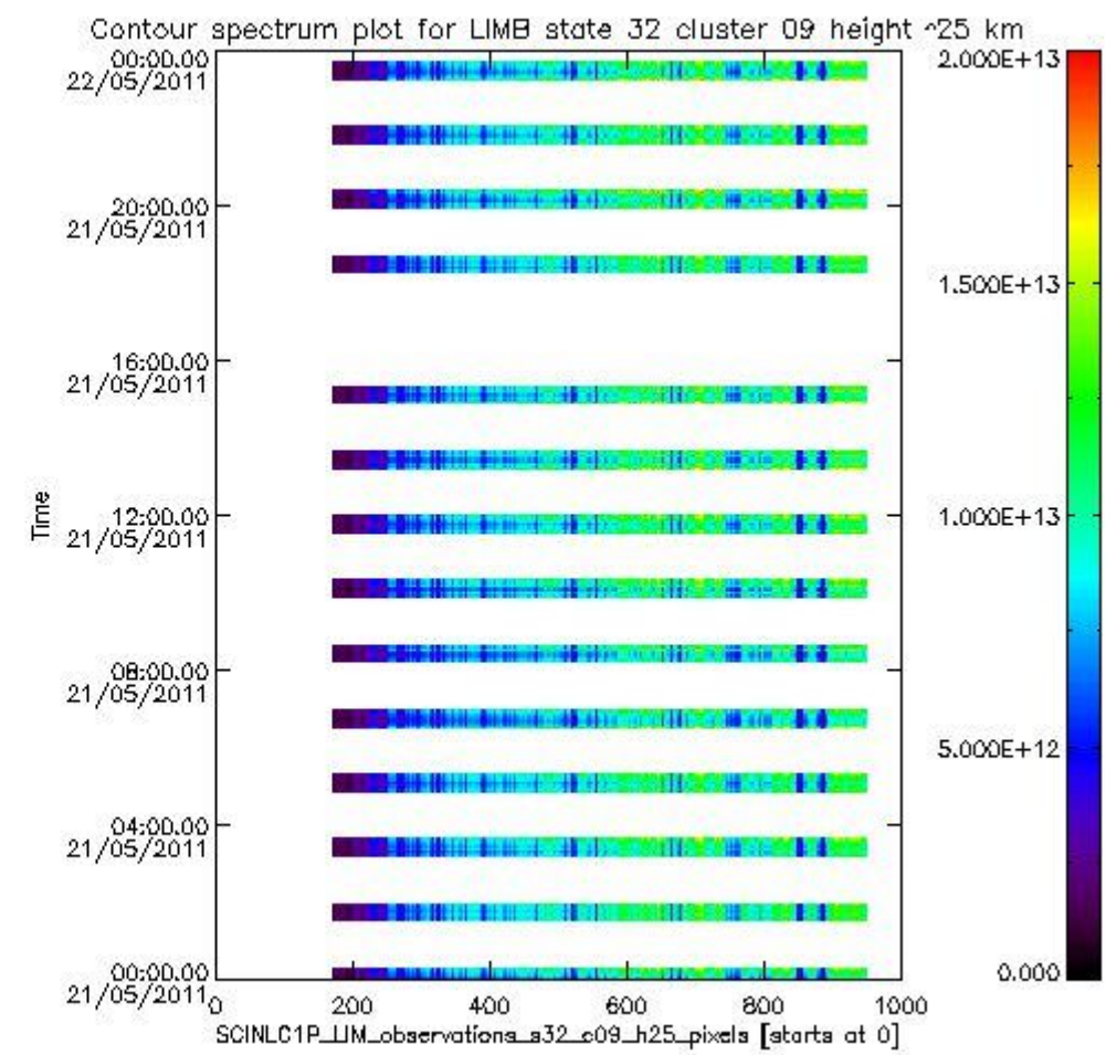
sciamachy_l1b_source_packet_report_SCIA_7_04_U_20110521_14.PNG
