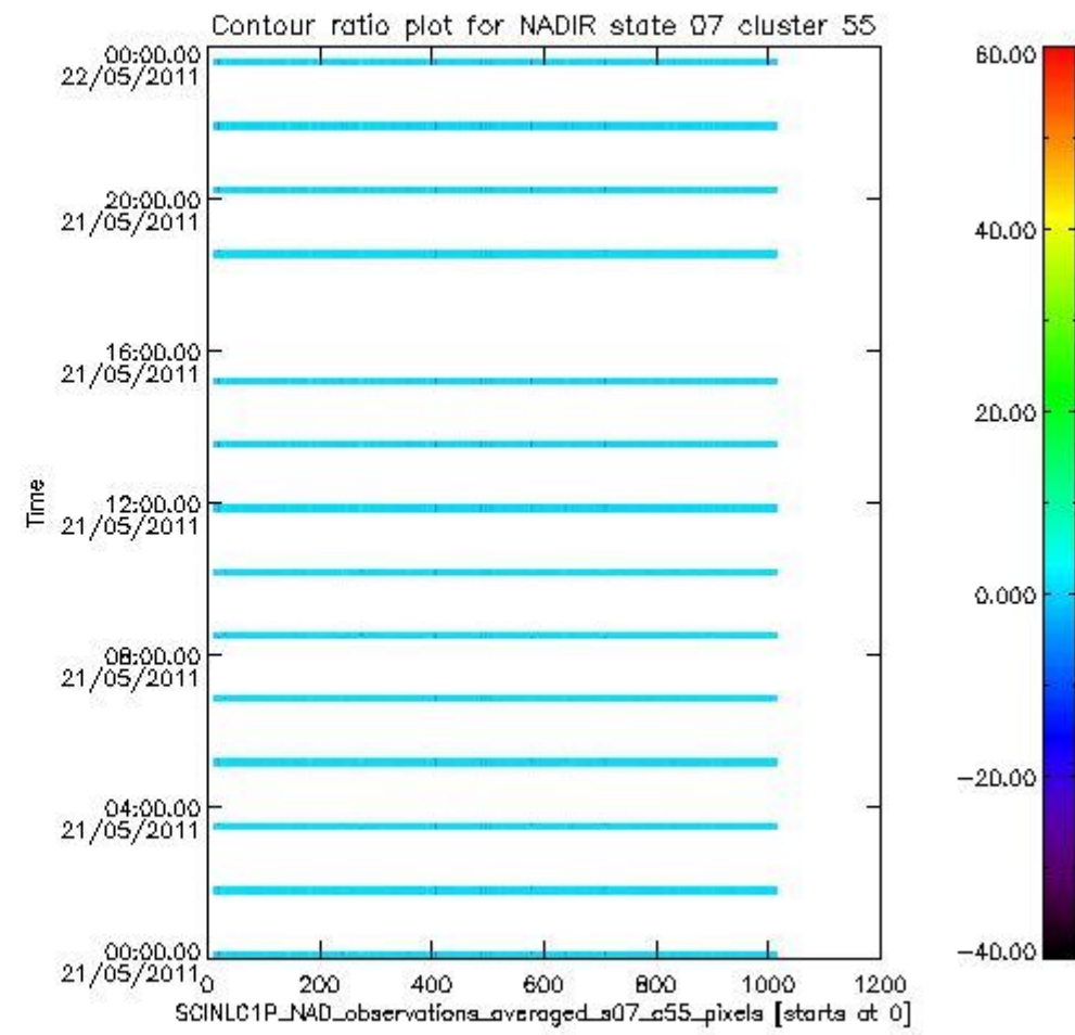
sciamachy_l1b_source_packet_report_SCIA_7_04_U_20110521_9.PNG
