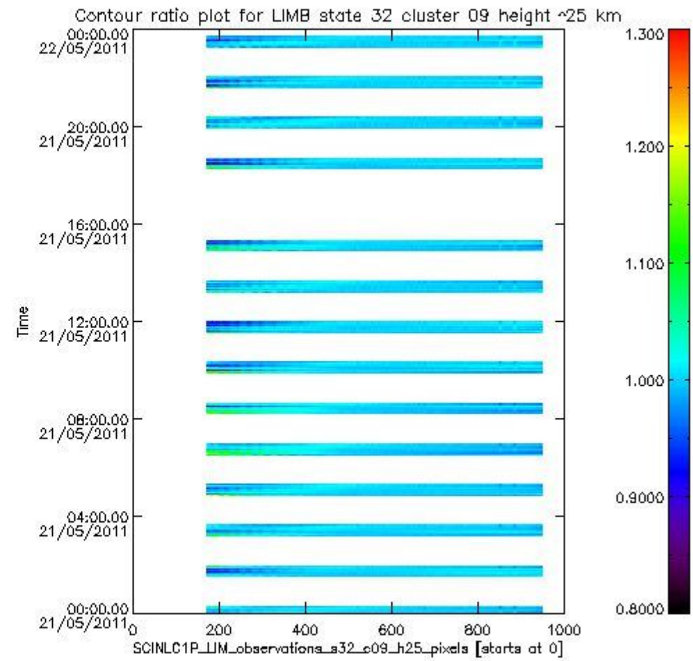
sciamachy_l1b_source_packet_report_SCIA_7_04_U_20110521_15.PNG
