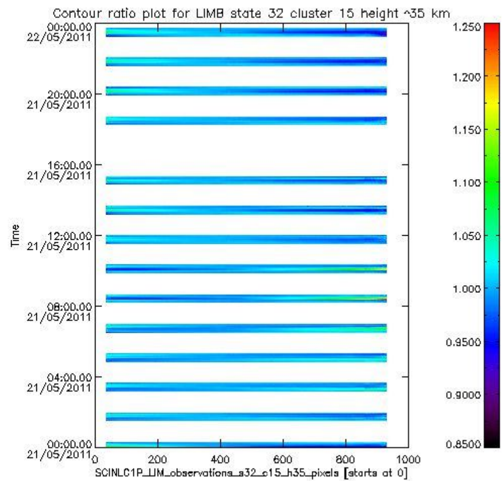
sciamachy_i1b_source_packet_report_SCIA_7_04_U_20110521_21.PNG
