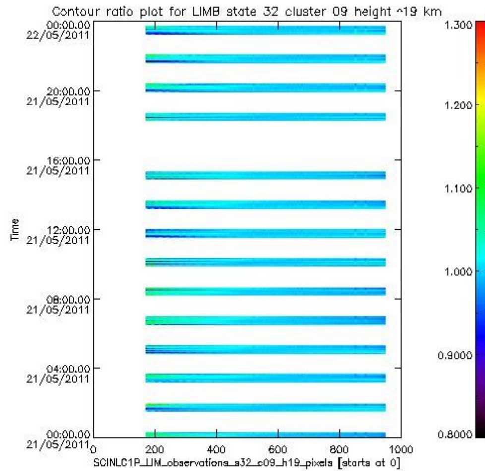
sciamachy_l1b_source_packet_report_SCIA_7_04_U_20110521_11.PNG
