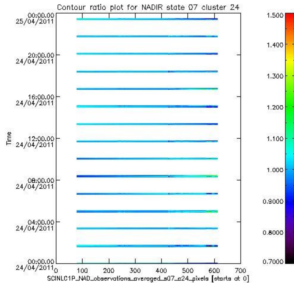
sciamachy_l1b_source_packet_report_SCIA_7_04_U_20110424_7.PNG
