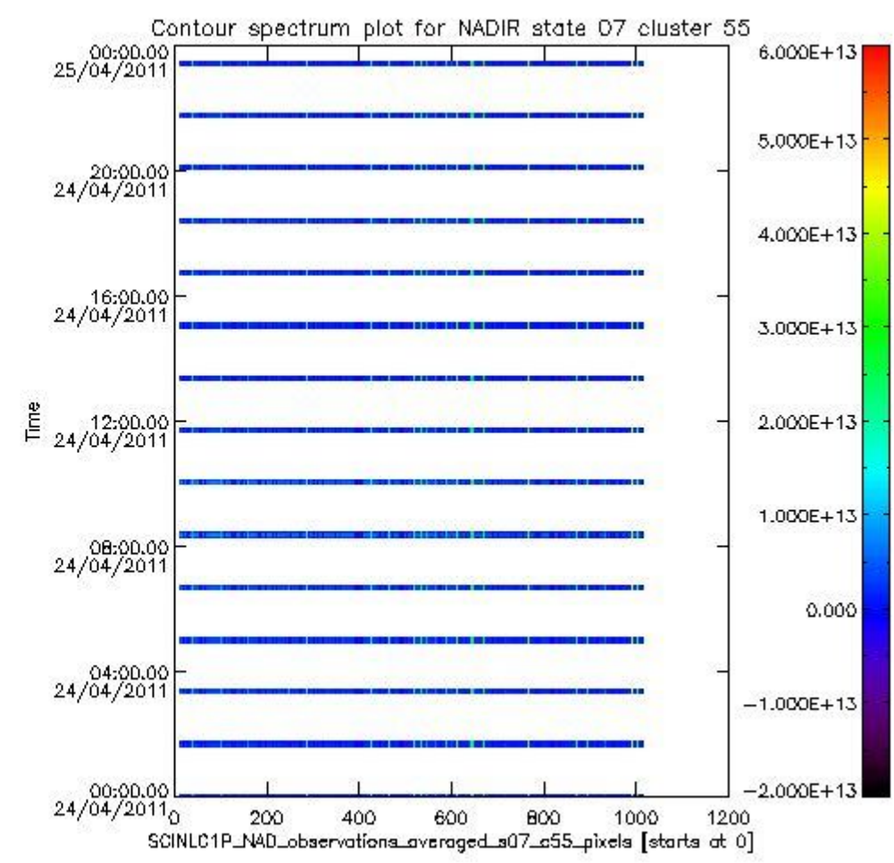
sciamachy_l1b_source_packet_report_SCIA_7_04_U_20110424_8.PNG
