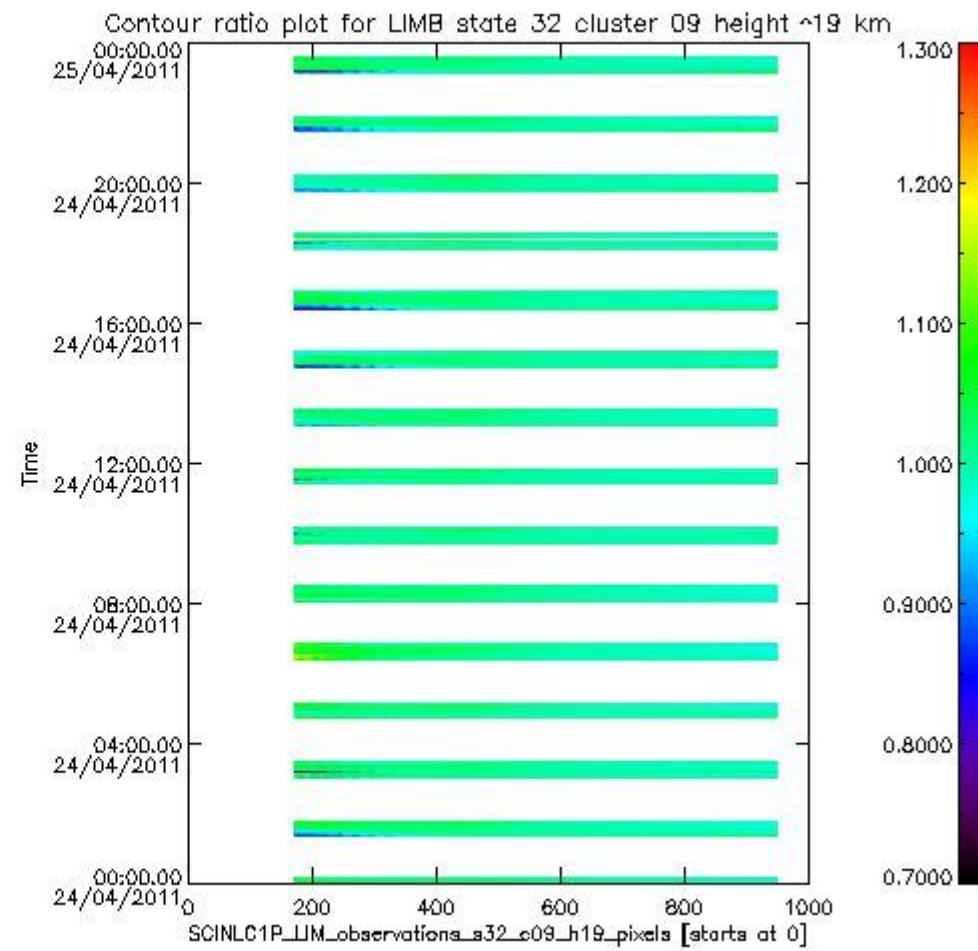
sciamachy_l1b_source_packet_report_SCIA_7_04_U_20110424_11.PNG
