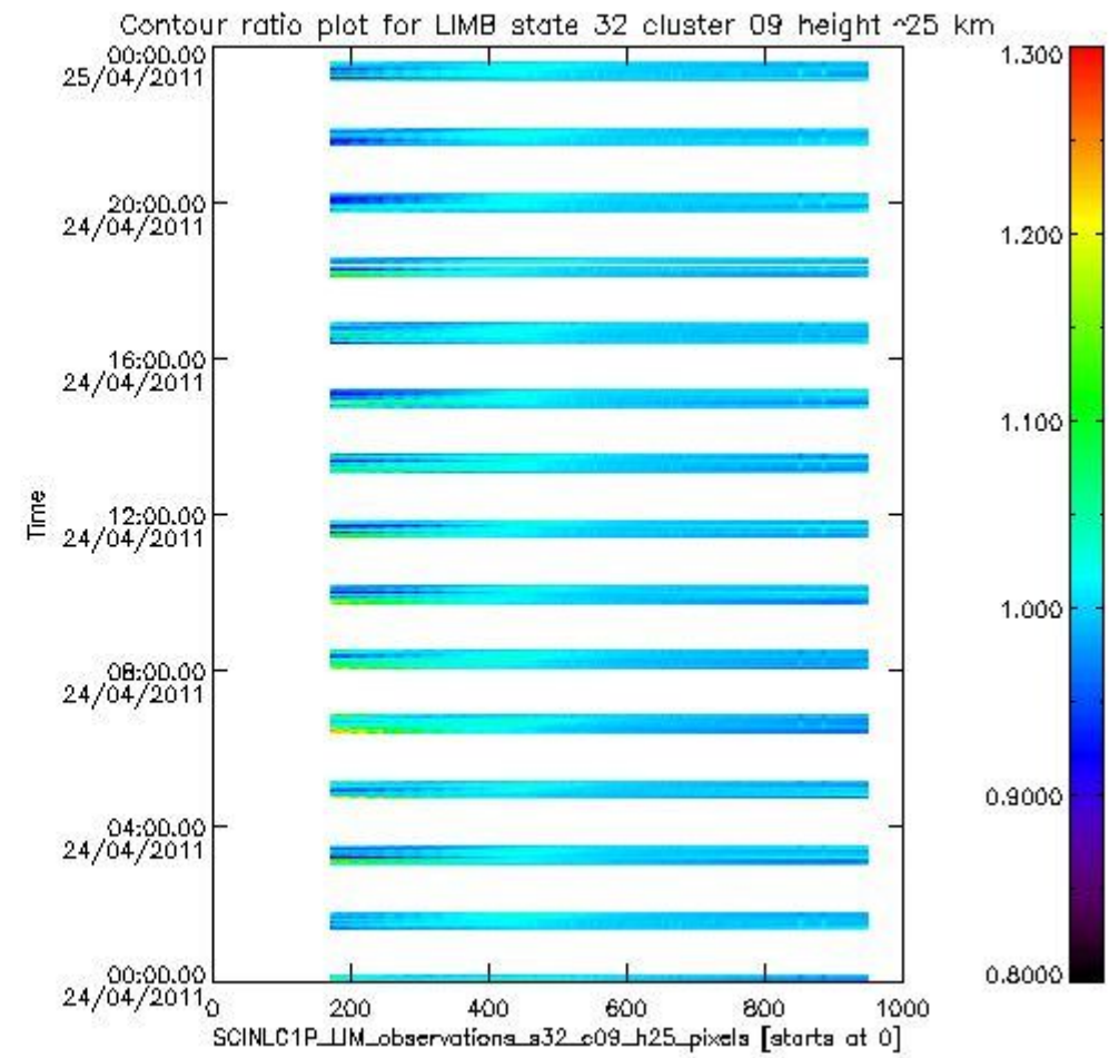
sciamachy_l1b_source_packet_report_SCIA_7_04_U_20110424_15.PNG
