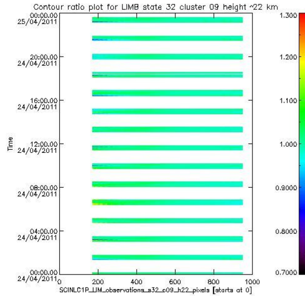
sciamachy_l1b_source_packet_report_SCIA_7_04_U_20110424_13.PNG
