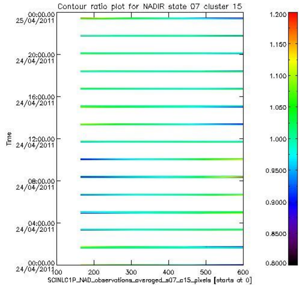
sciamachy_l1b_source_packet_report_SCIA_7_04_U_20110424_5.PNG
