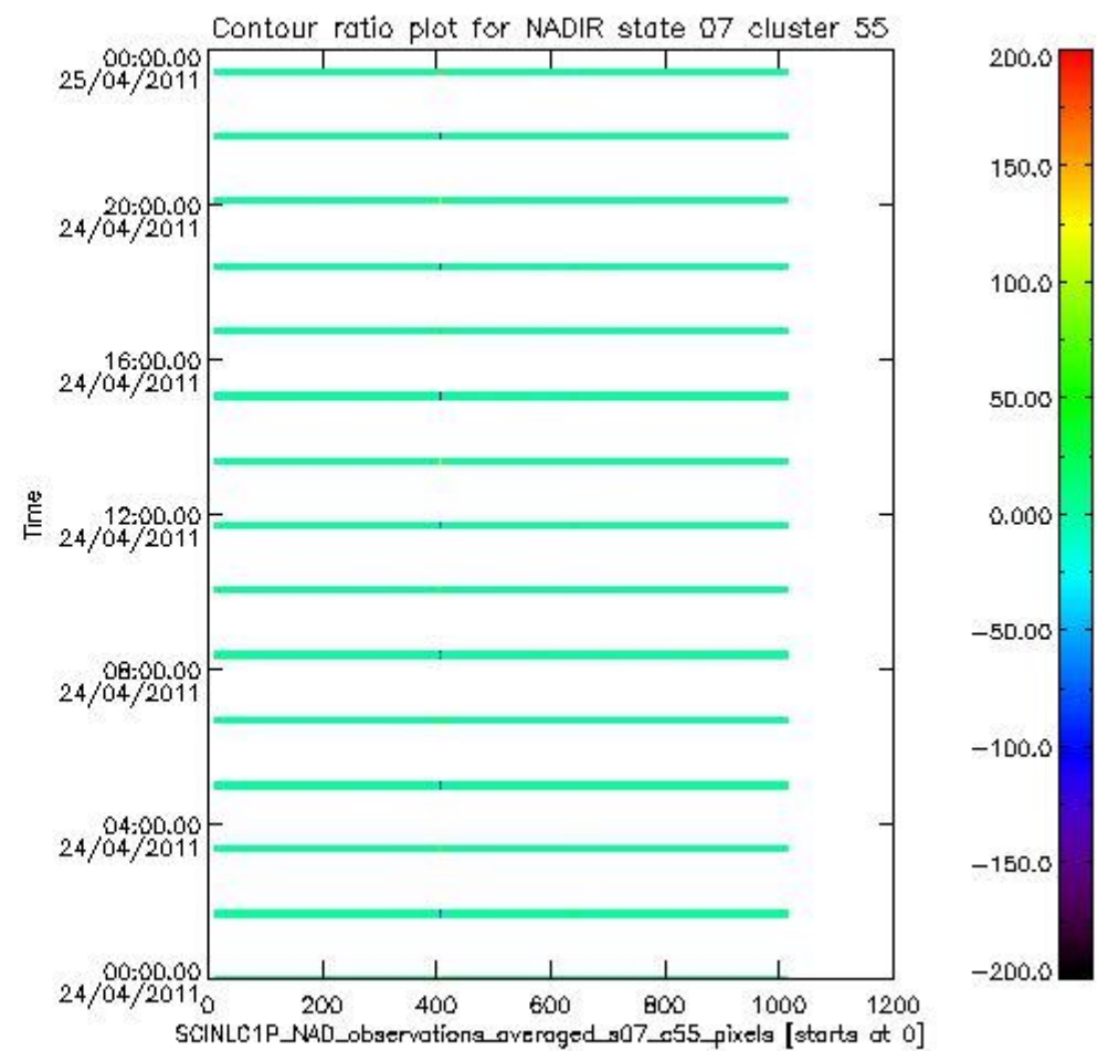
sciamachy_l1b_source_packet_report_SCIA_7_04_U_20110424_9.PNG
