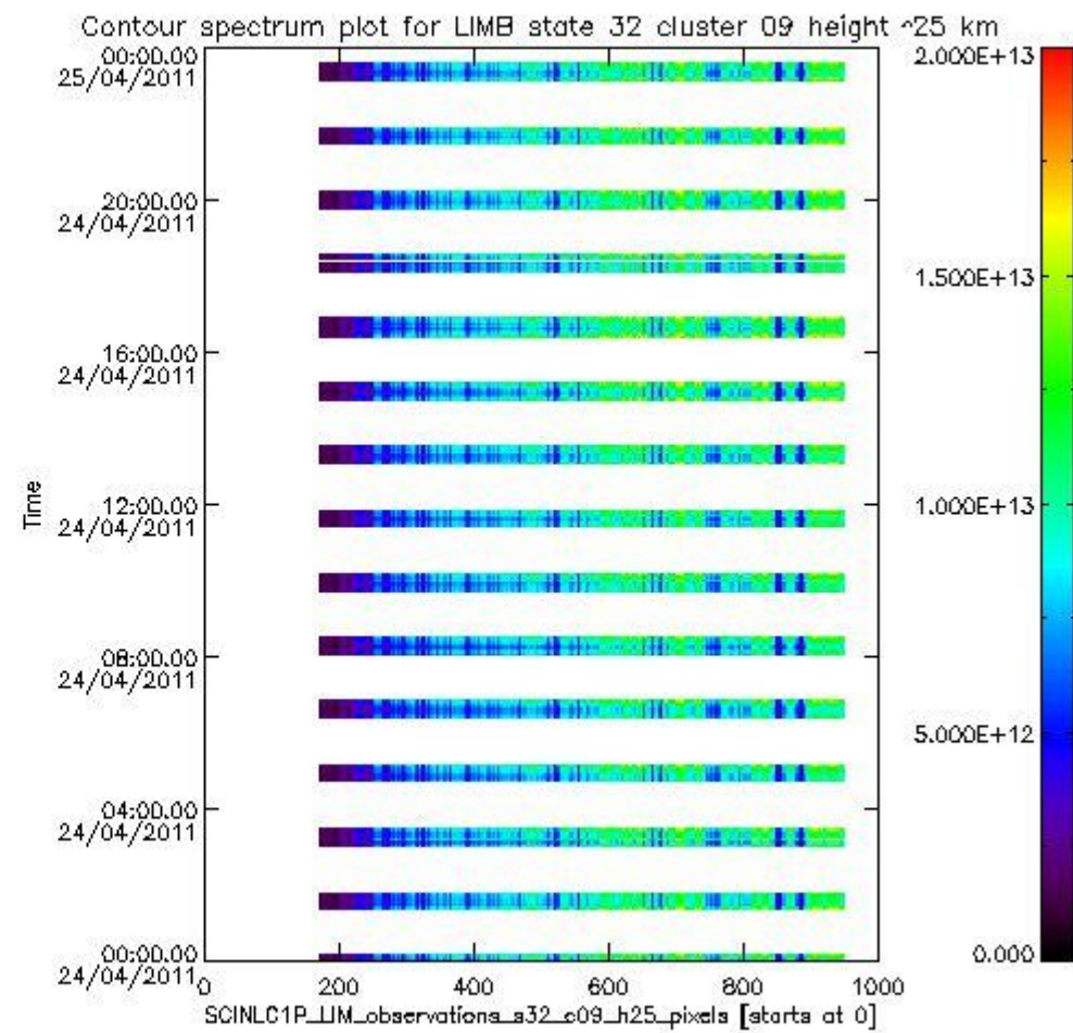
sciamachy_l1b_source_packet_report_SCIA_7_04_U_20110424_14.PNG
