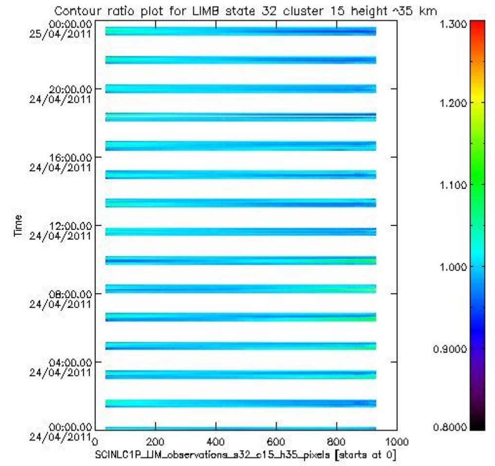
sciamachy_11b_source_packet_report_SCIA_7_04_U_20110424_21.PNG
