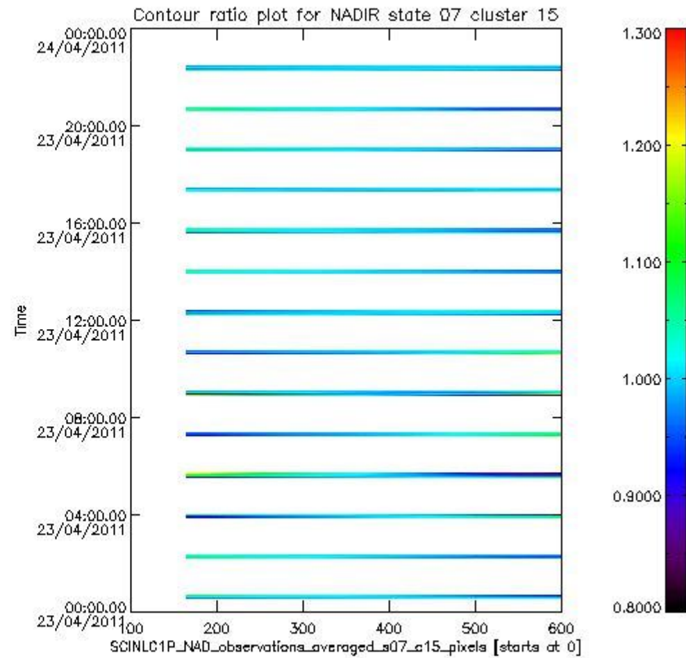
sciamachy_l1b_source_packet_report_SCIA_7_04_U_20110423_5.PNG
