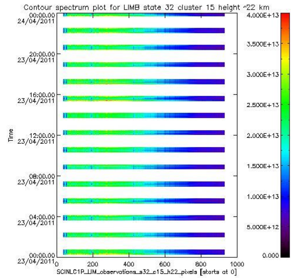
sciamachy_l1b_source_packet_report_SCIA_7_04_U_20110423_16.PNG
