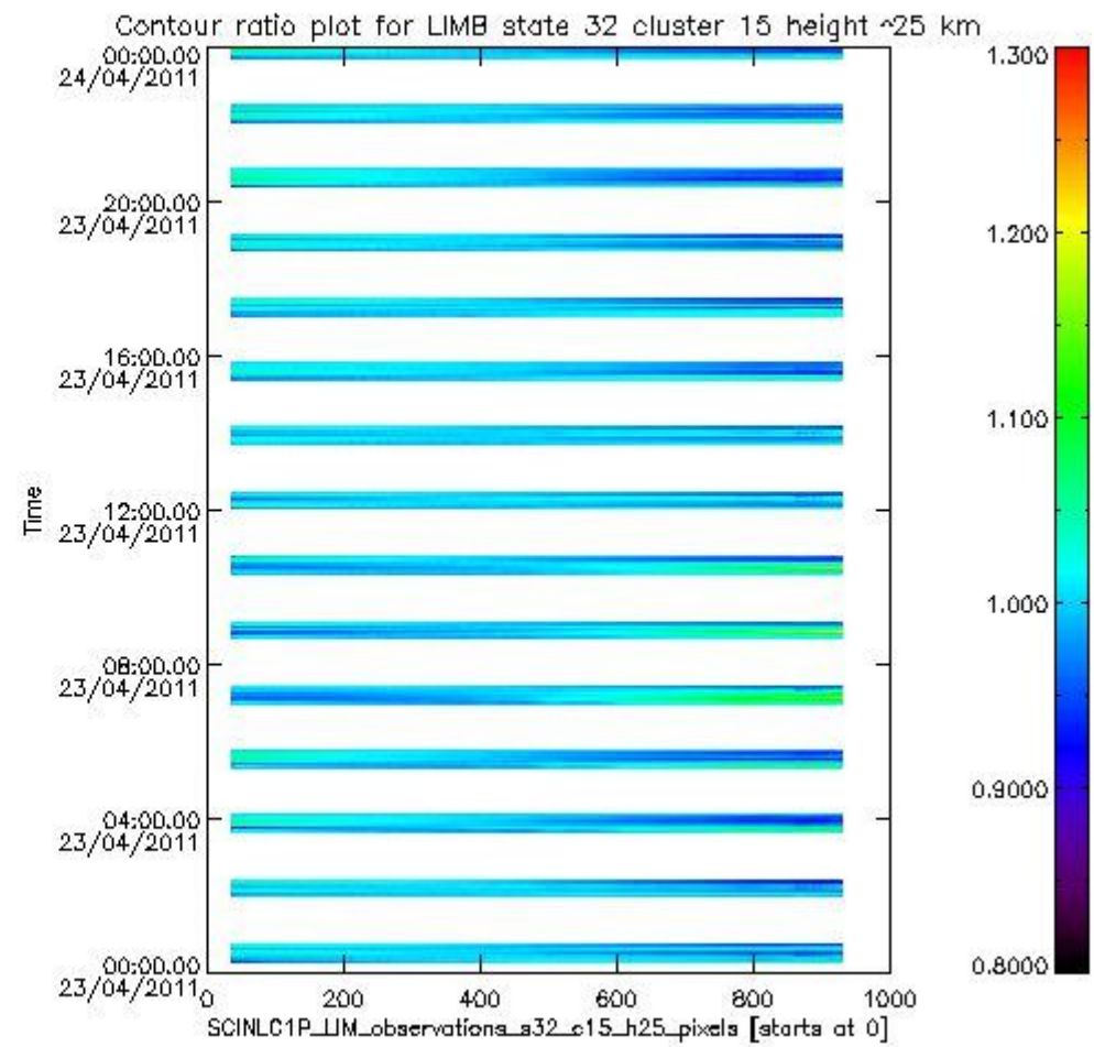
sciamachy_11b_source_packet_report_SCIA_7_04_U_20110423_19.PNG
