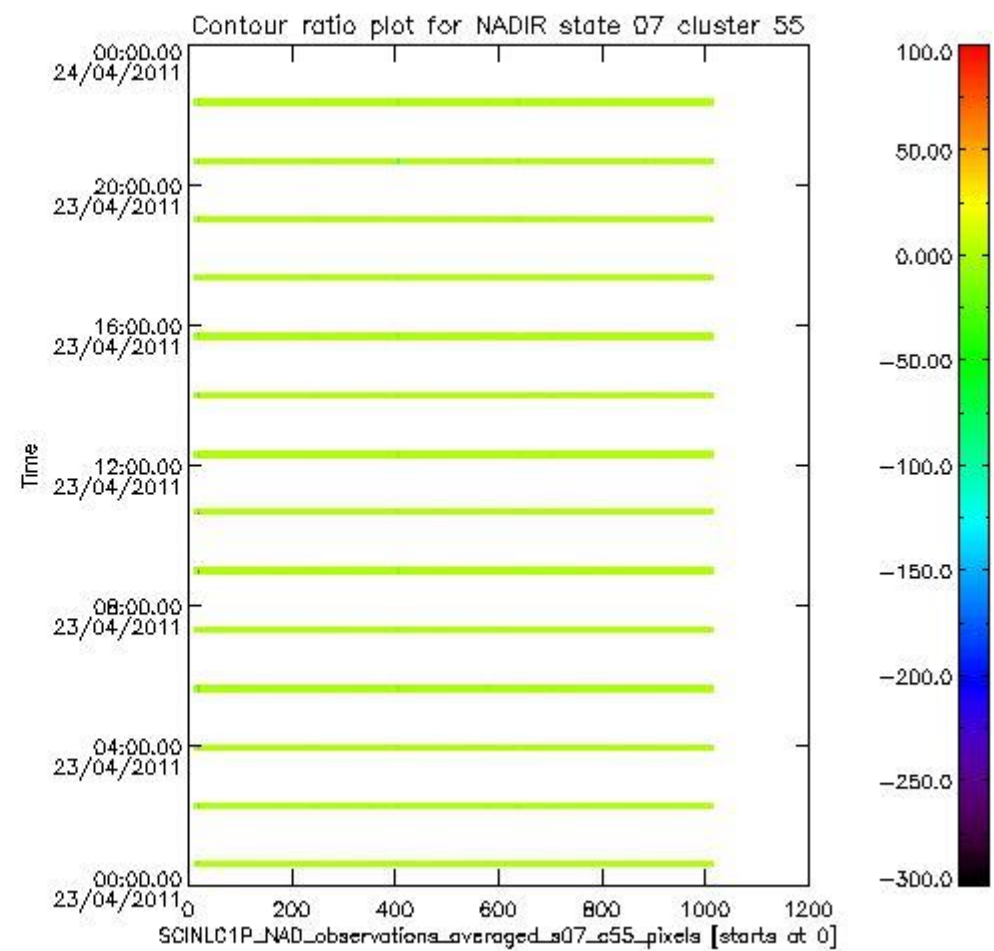
sciamachy_l1b_source_packet_report_SCIA_7_04_U_20110423_9.PNG
