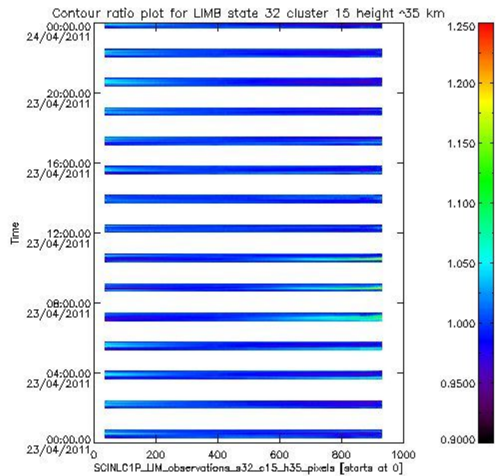
sciamachy_i1b_source_packet_report_SCIA_7_04_U_20110423_21.PNG
