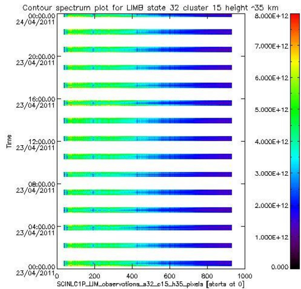
sciamachy_11b_source_packet_report_SCIA_7_04_U_20110423_20.PNG
