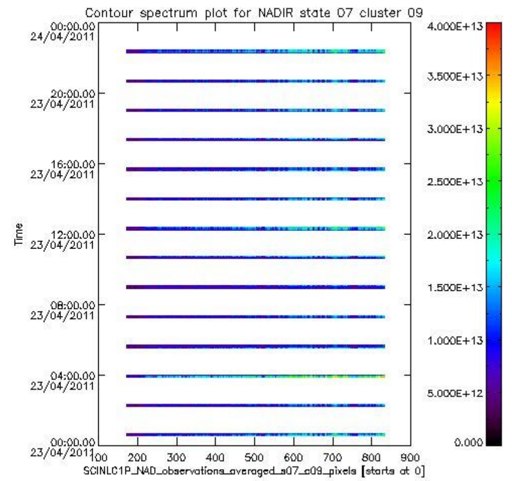
sciamachy_i1b_source_packet_report_SCIA_7_04_U_20110423_2.PNG
