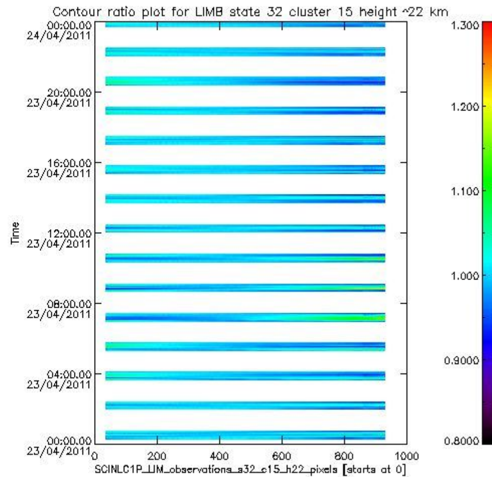
sciamachy_11b_source_packet_report_SCIA_7_04_U_20110423_17.PNG
