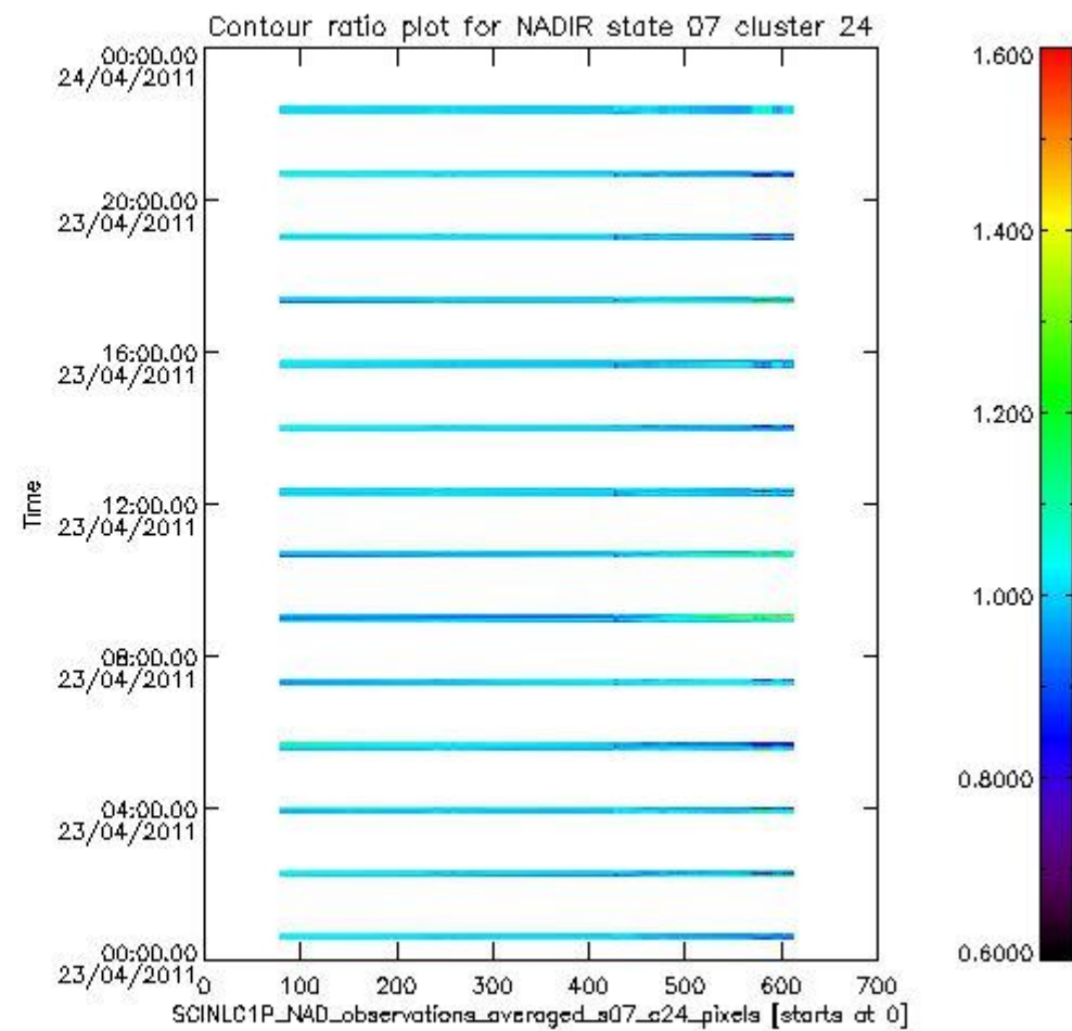
sciamachy_l1b_source_packet_report_SCIA_7_04_U_20110423_7.PNG
