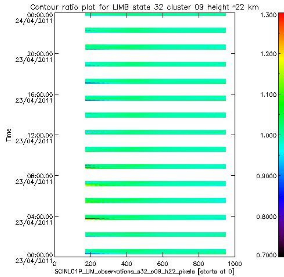
sciamachy_l1b_source_packet_report_SCIA_7_04_U_20110423_13.PNG
