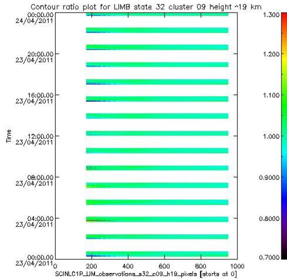
sciamachy_l1b_source_packet_report_SCIA_7_04_U_20110423_11.PNG
