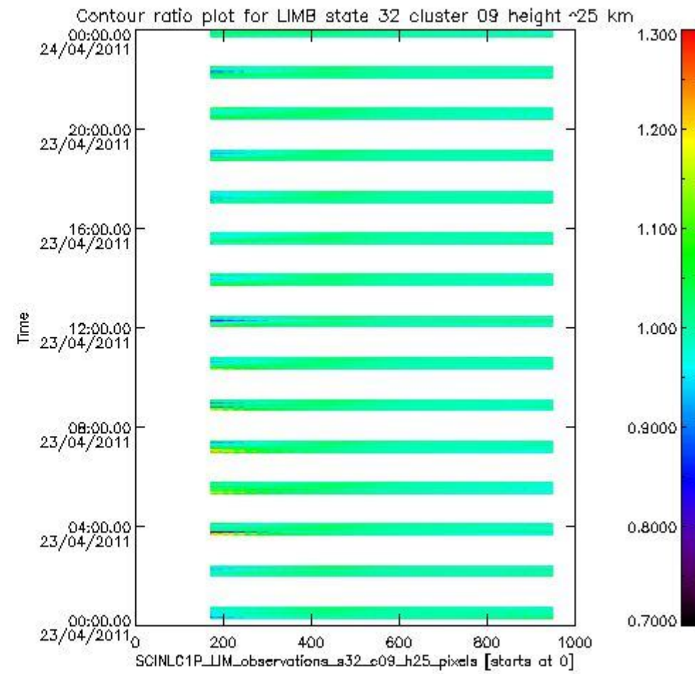
sciamachy_l1b_source_packet_report_SCIA_7_04_U_20110423_15.PNG
