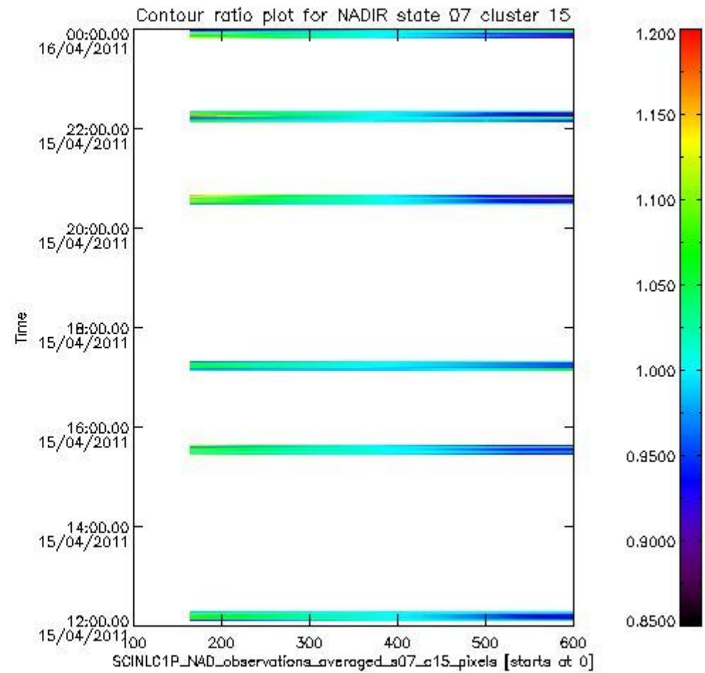
sciamachy_l1b_source_packet_report_SCIA_7_04_U_20110415_5.PNG
