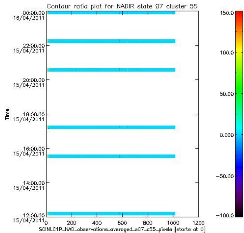
sciamachy_l1b_source_packet_report_SCIA_7_04_U_20110415_9.PNG
