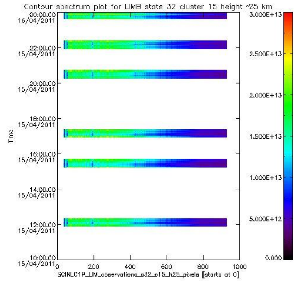
sciamachy_l1b_source_packet_report_SCIA_7_04_U_20110415_18.PNG
