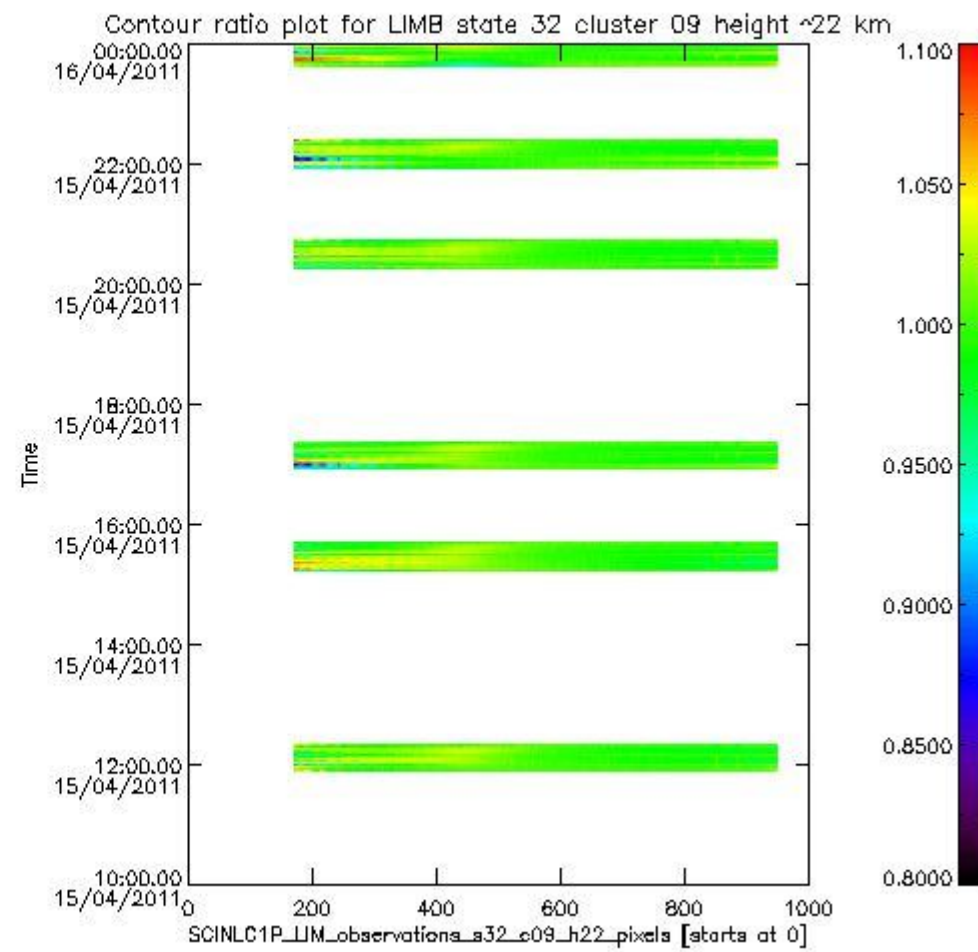
sciamachy_l1b_source_packet_report_SCIA_7_04_U_20110415_13.PNG
