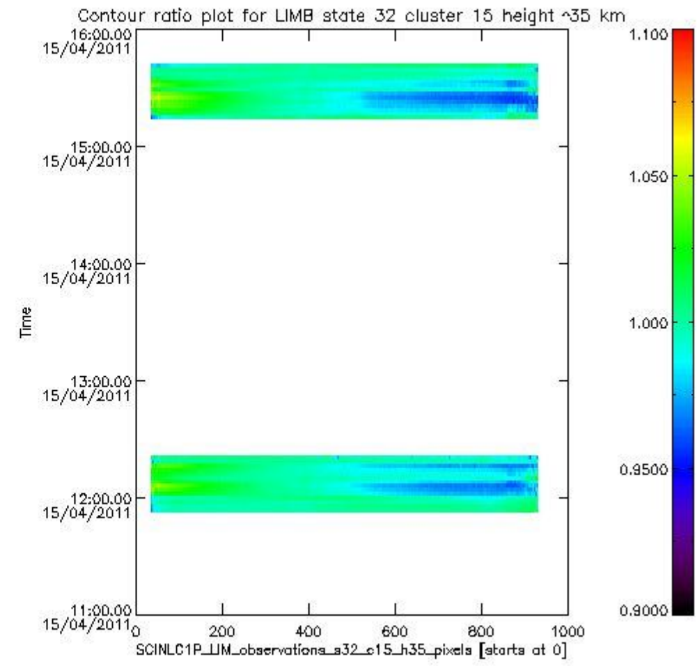
sciamachy_i1b_source_packet_report_SCIA_7_04_U_20110415_21.PNG
