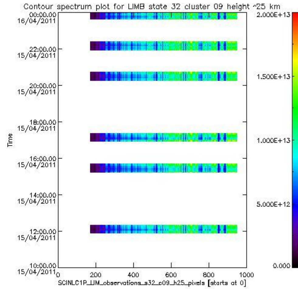
sciamachy_l1b_source_packet_report_SCIA_7_04_U_20110415_14.PNG
