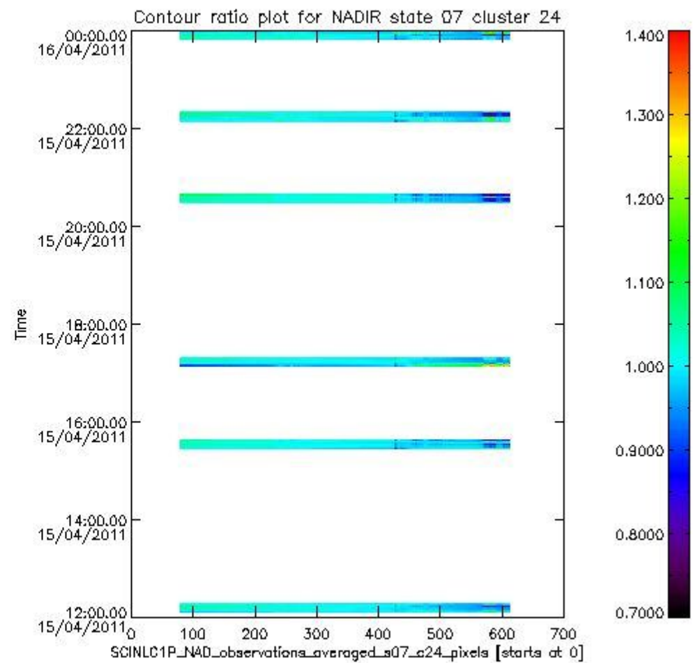
sciamachy_l1b_source_packet_report_SCIA_7_04_U_20110415_7.PNG
