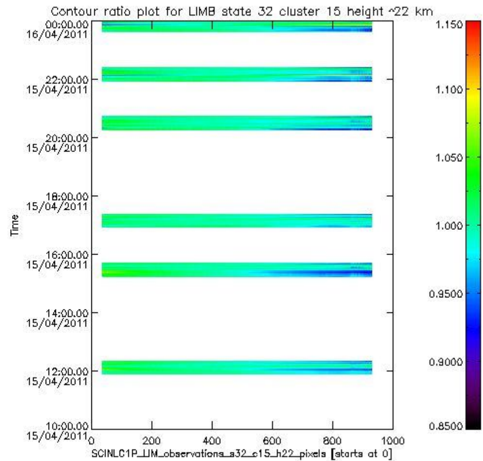
sciamachy_l1b_source_packet_report_SCIA_7_04_U_20110415_17.PNG
