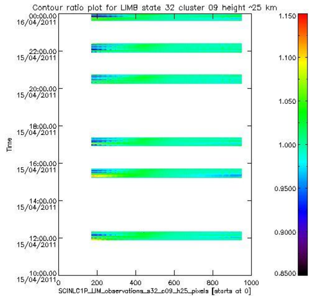
sciamachy_l1b_source_packet_report_SCIA_7_04_U_20110415_15.PNG
