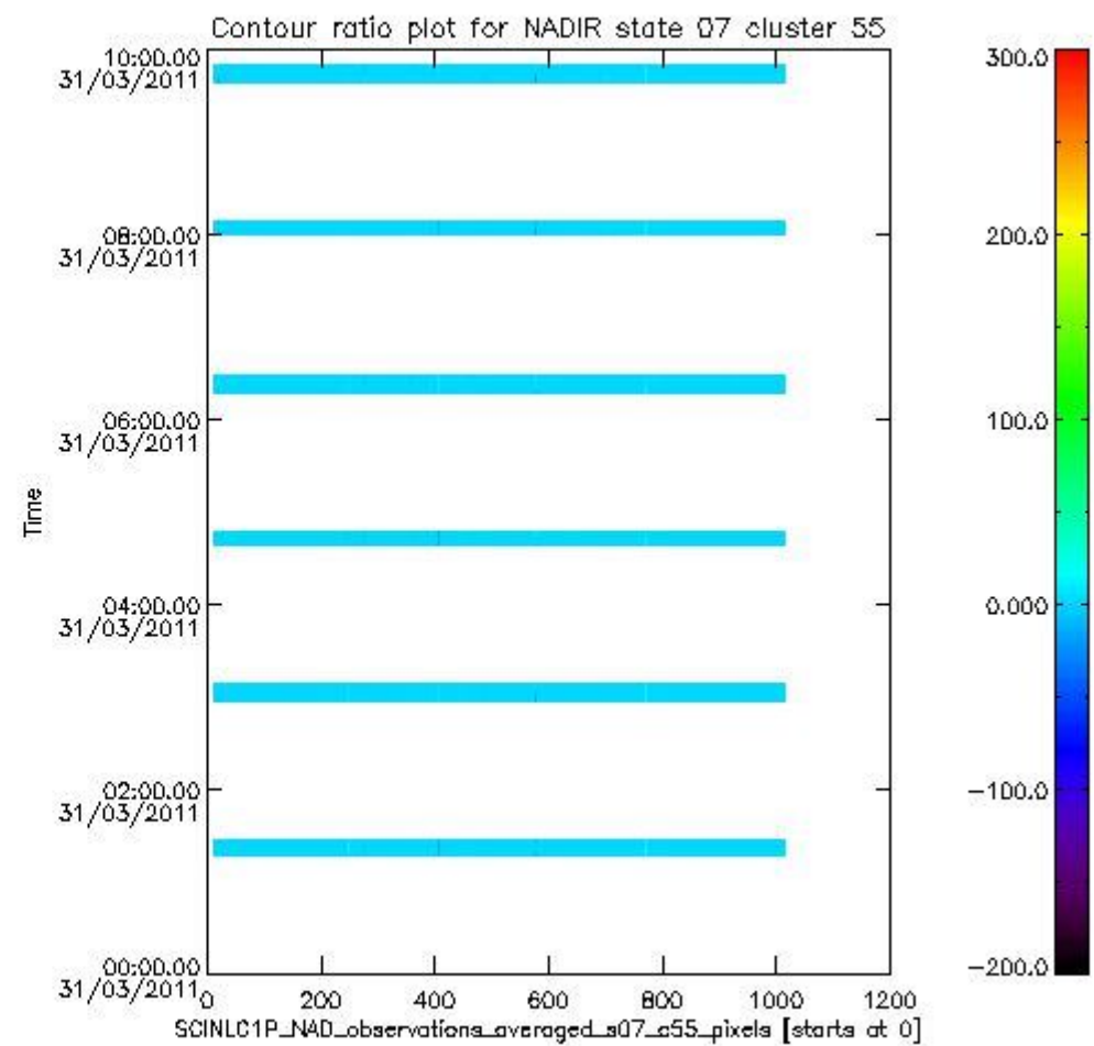
sciamachy_l1b_source_packet_report_SCIA_7_04_U_20110331_9.PNG
