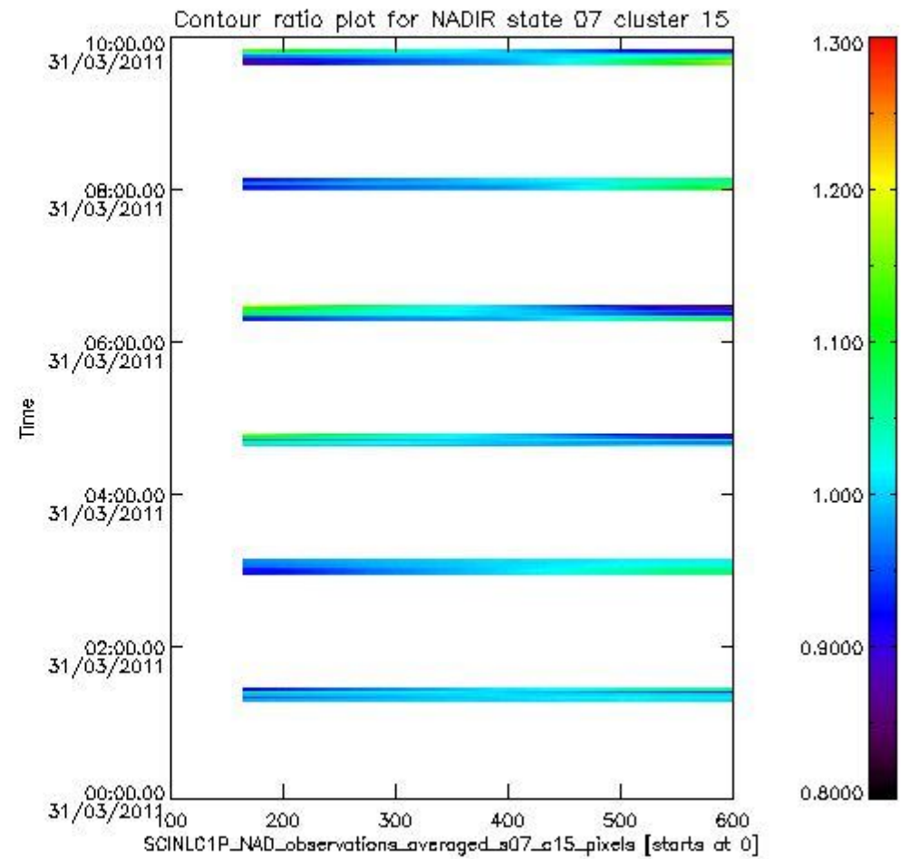
sciamachy_l1b_source_packet_report_SCIA_7_04_U_20110331_5.PNG
