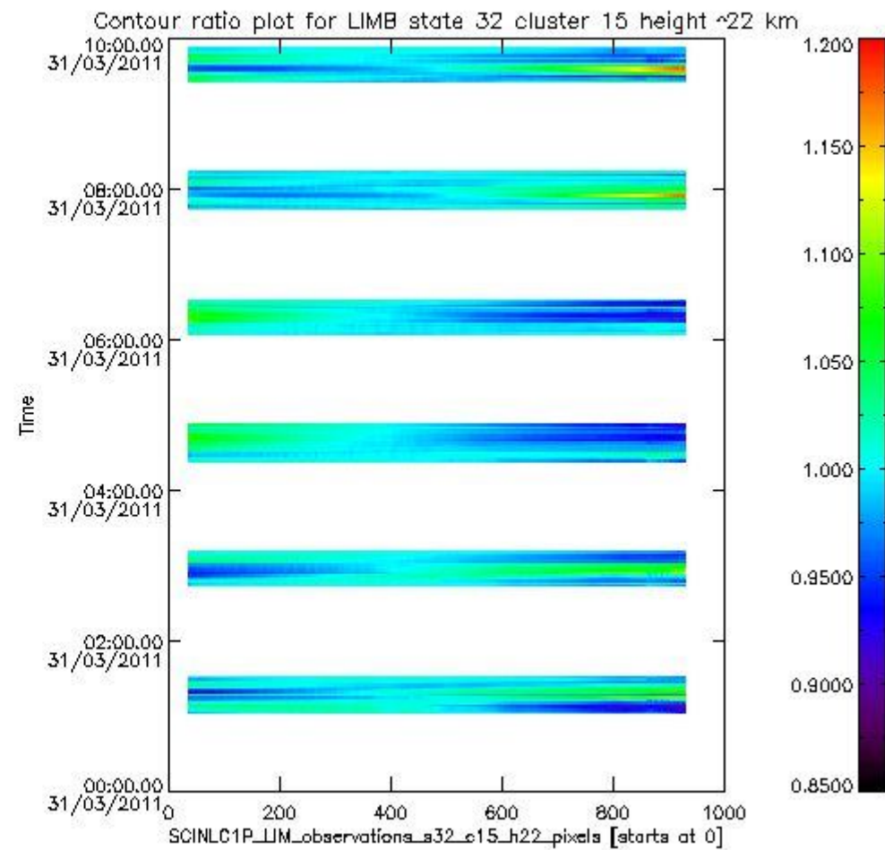
sciamachy_11b_source_packet_report_SCIA_7_04_U_20110331_17.PNG
