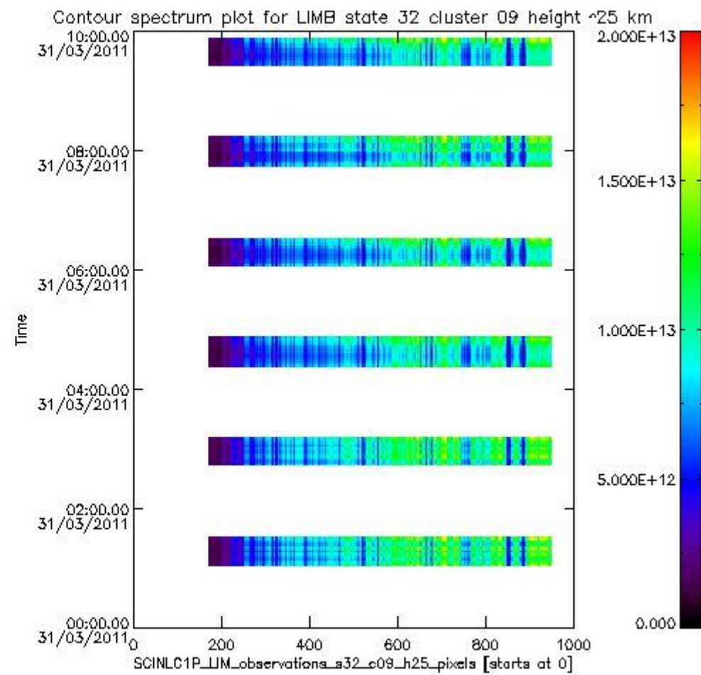
sciamachy_l1b_source_packet_report_SCIA_7_04_U_20110331_14.PNG
