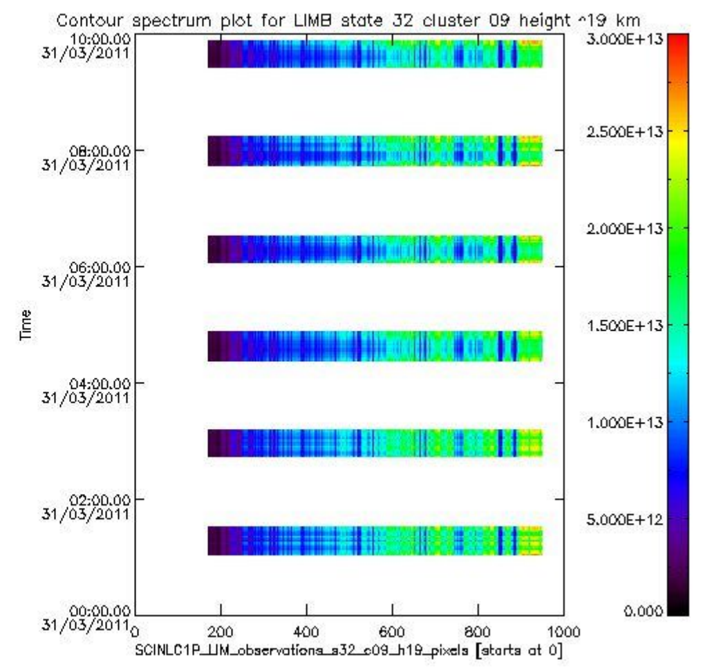
sciamachy_i1b_source_packet_report_SCIA_7_04_U_20110331_10.PNG
