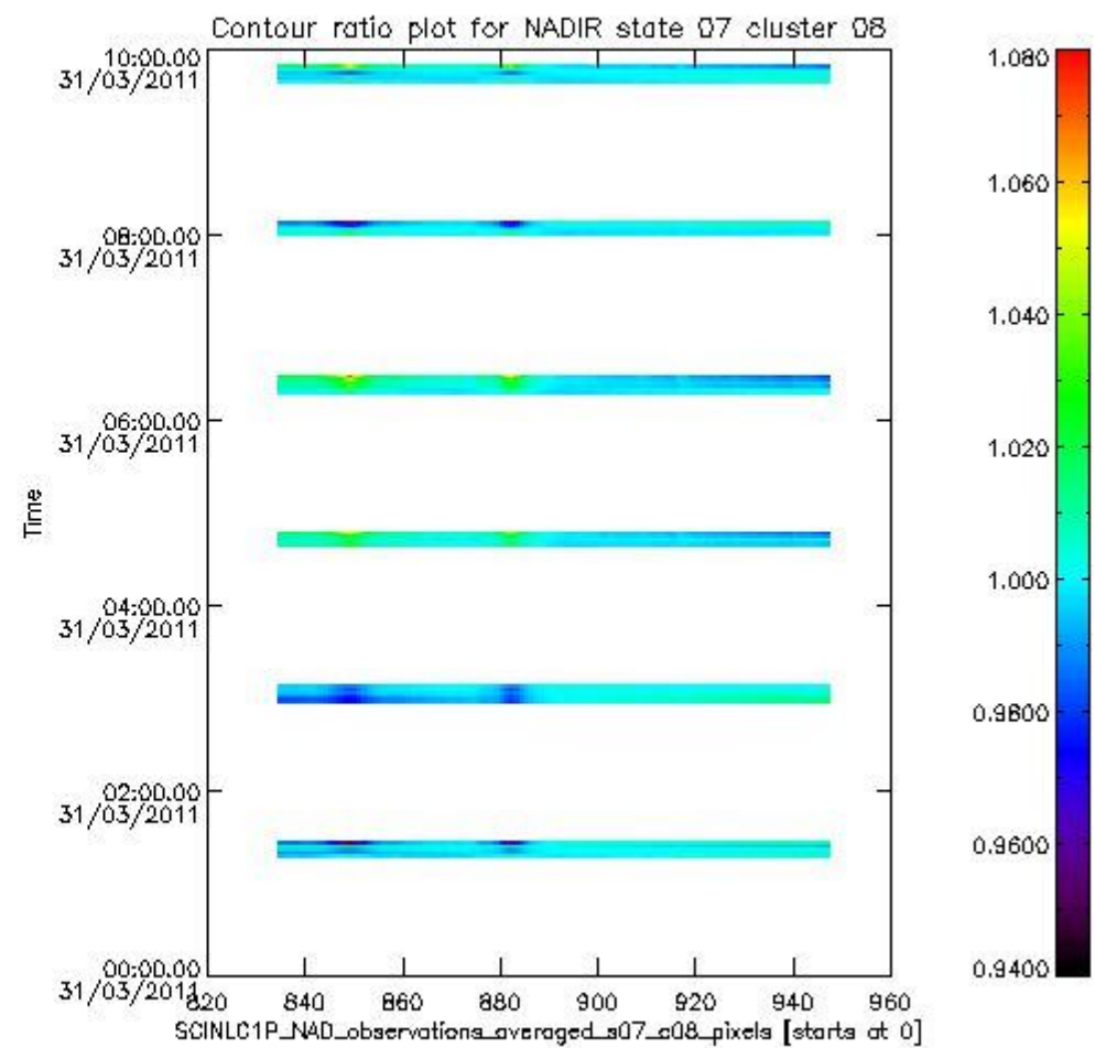
sciamachy_i1b_source_packet_report_SCIA_7_04_U_20110331_1.PNG
