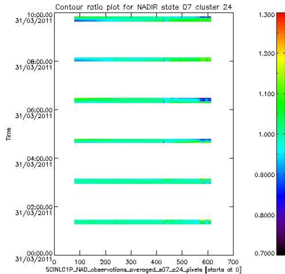
sciamachy_l1b_source_packet_report_SCIA_7_04_U_20110331_7.PNG
