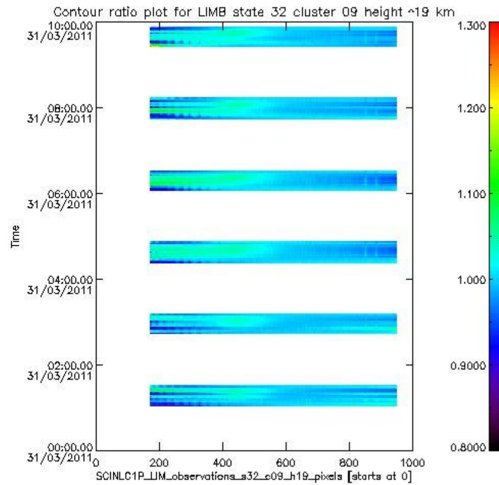
sciamachy_i1b_source_packet_report_SCIA_7_04_U_20110331_11.PNG
