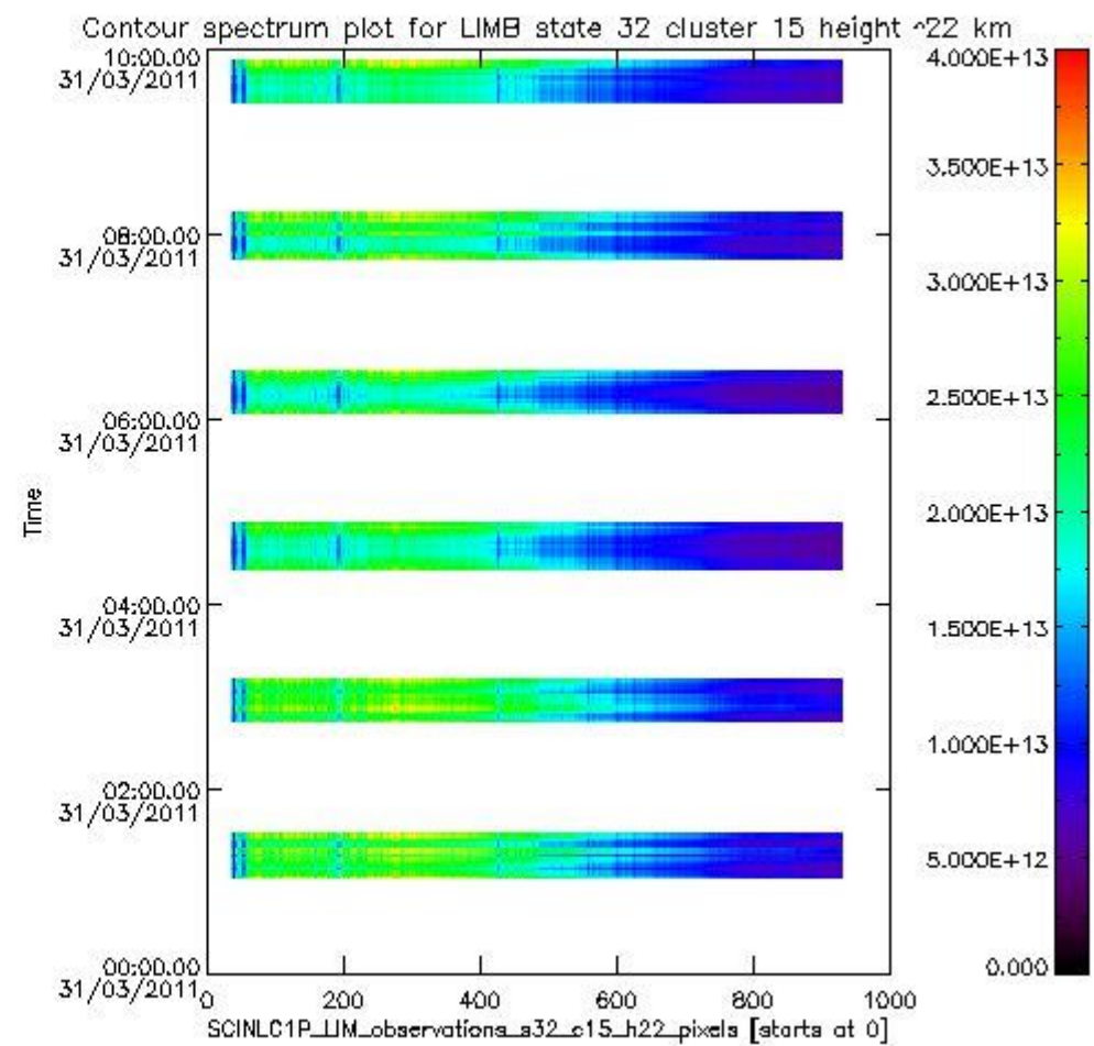
sciamachy_i1b_source_packet_report_SCIA_7_04_U_20110331_16.PNG
