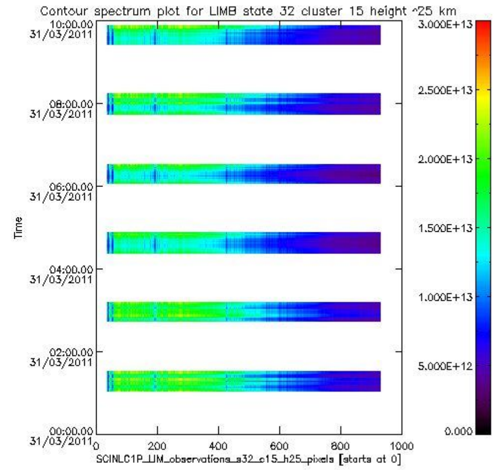
sciamachy_l1b_source_packet_report_SCIA_7_04_U_20110331_18.PNG
