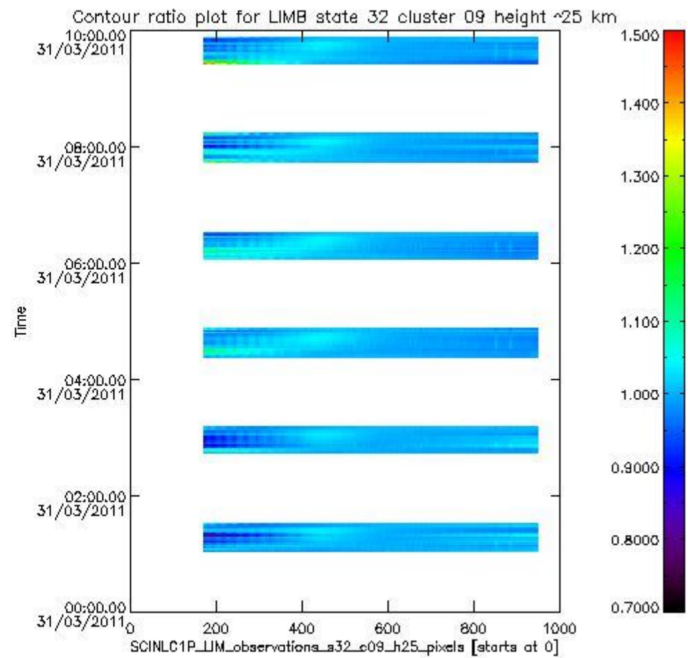
sciamachy_l1b_source_packet_report_SCIA_7_04_U_20110331_15.PNG
