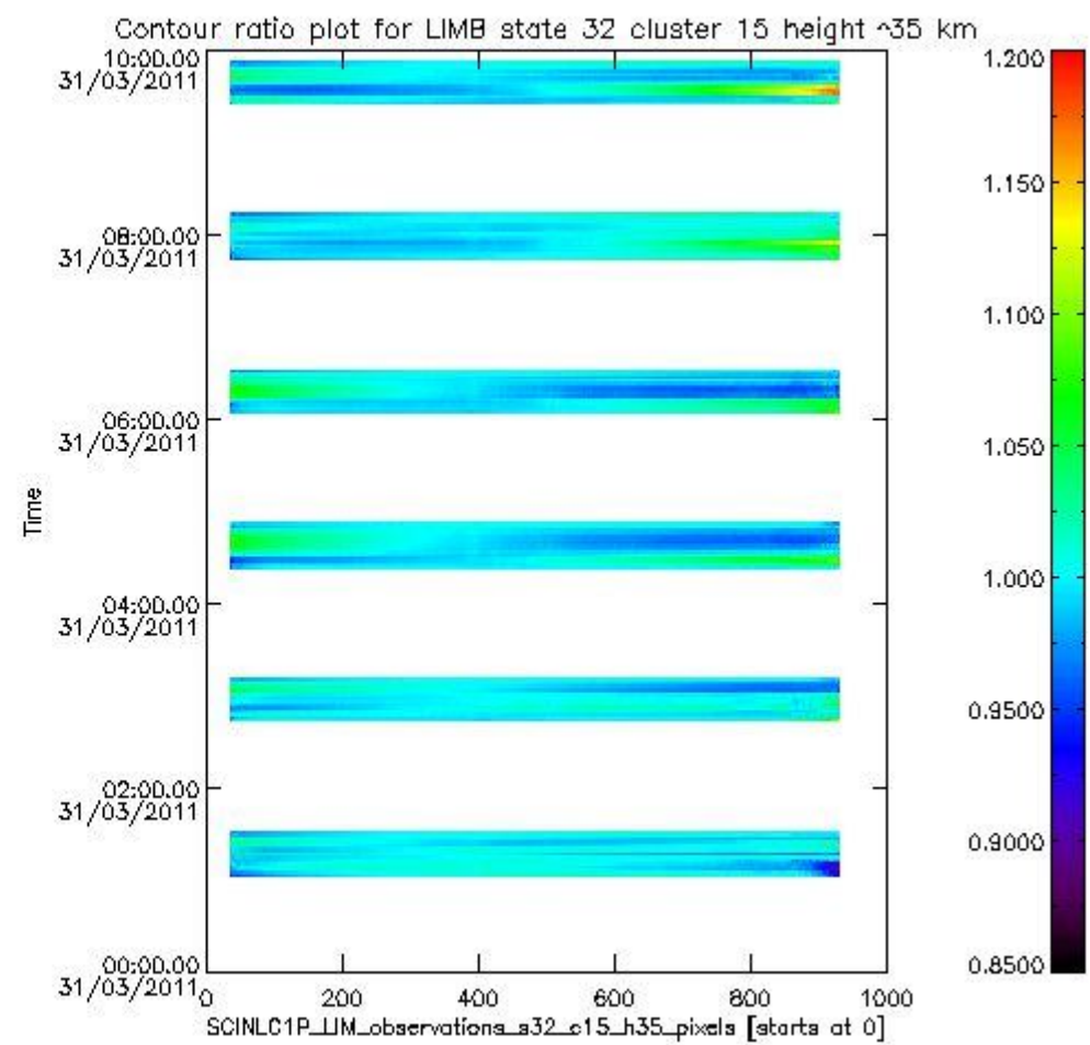
sciamachy_i1b_source_packet_report_SCIA_7_04_U_20110331_21.PNG
