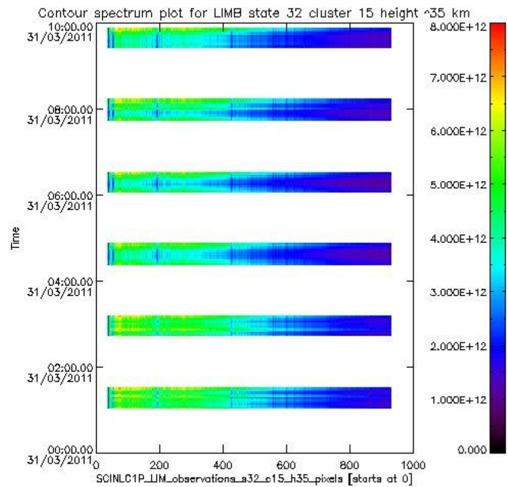
sciamachy_11b_source_packet_report_SCIA_7_04_U_20110331_20.PNG
