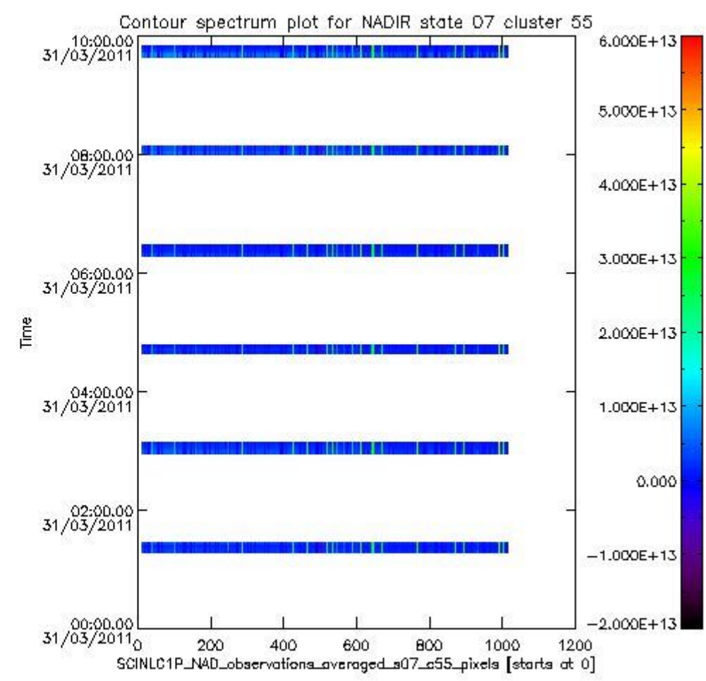
sciamachy_i1b_source_packet_report_SCIA_7_04_U_20110331_8.PNG
