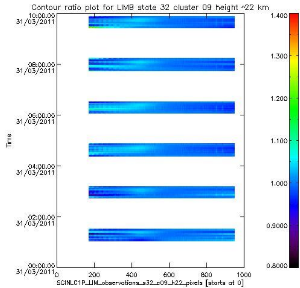
sciamachy_l1b_source_packet_report_SCIA_7_04_U_20110331_13.PNG
