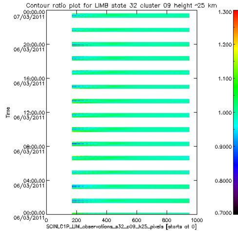
sciamachy_l1b_source_packet_report_SCIA_7_04_U_20110306_15.PNG
