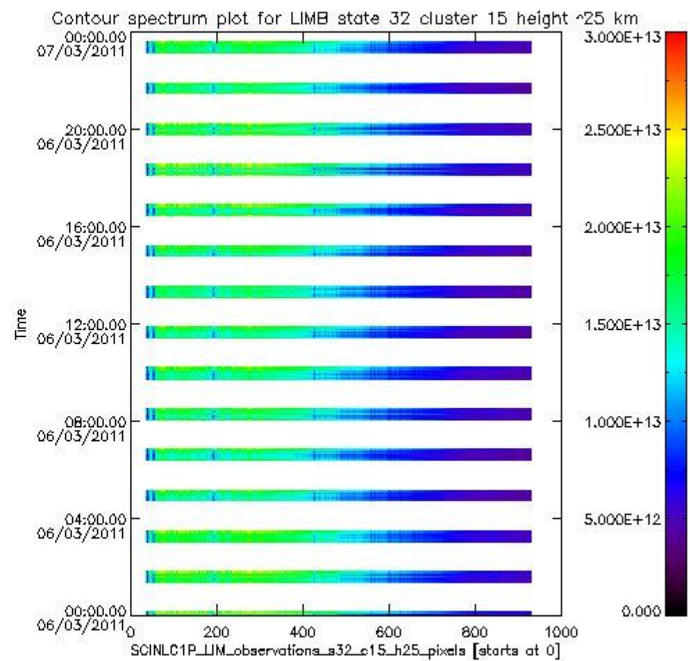
sciamachy_l1b_source_packet_report_SCIA_7_04_U_20110306_18.PNG
