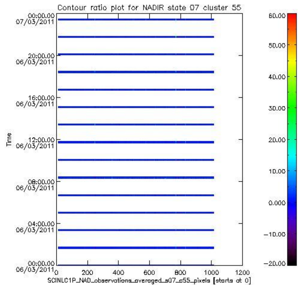
sciamachy_l1b_source_packet_report_SCIA_7_04_U_20110306_9.PNG
