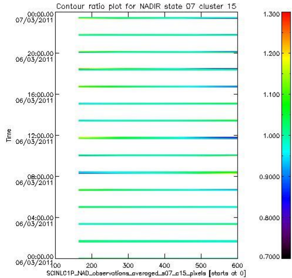
sciamachy_l1b_source_packet_report_SCIA_7_04_U_20110306_5.PNG
