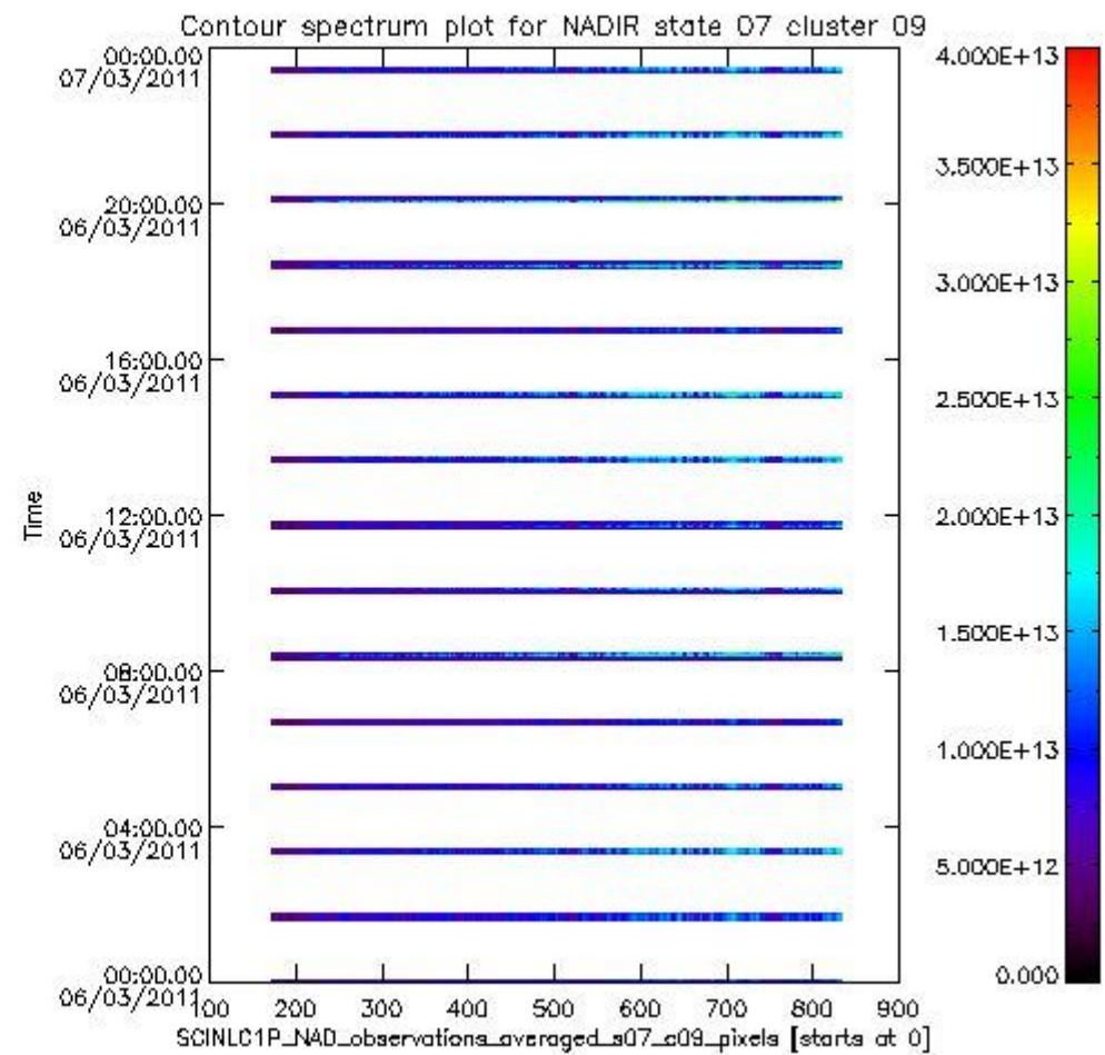
sciamachy_i1b_source_packet_report_SCIA_7_04_U_20110306_2.PNG
