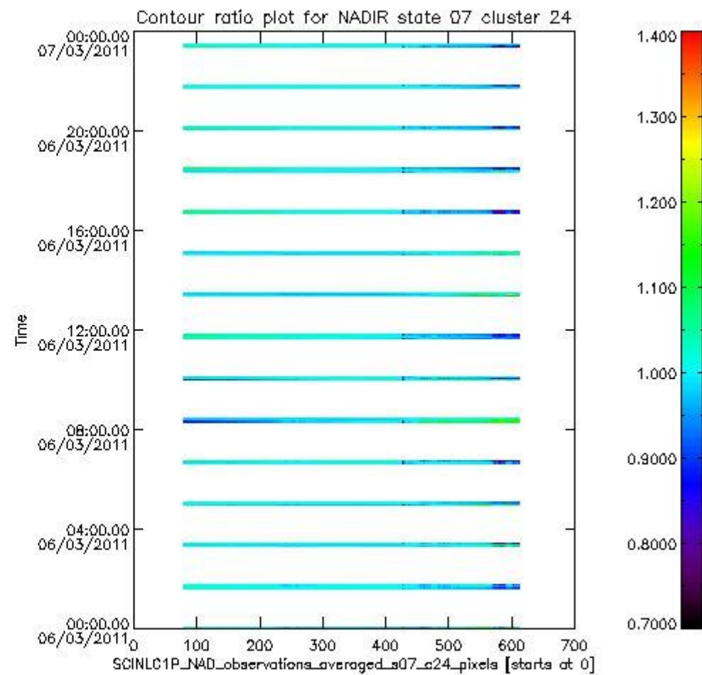
sciamachy_l1b_source_packet_report_SCIA_7_04_U_20110306_7.PNG
