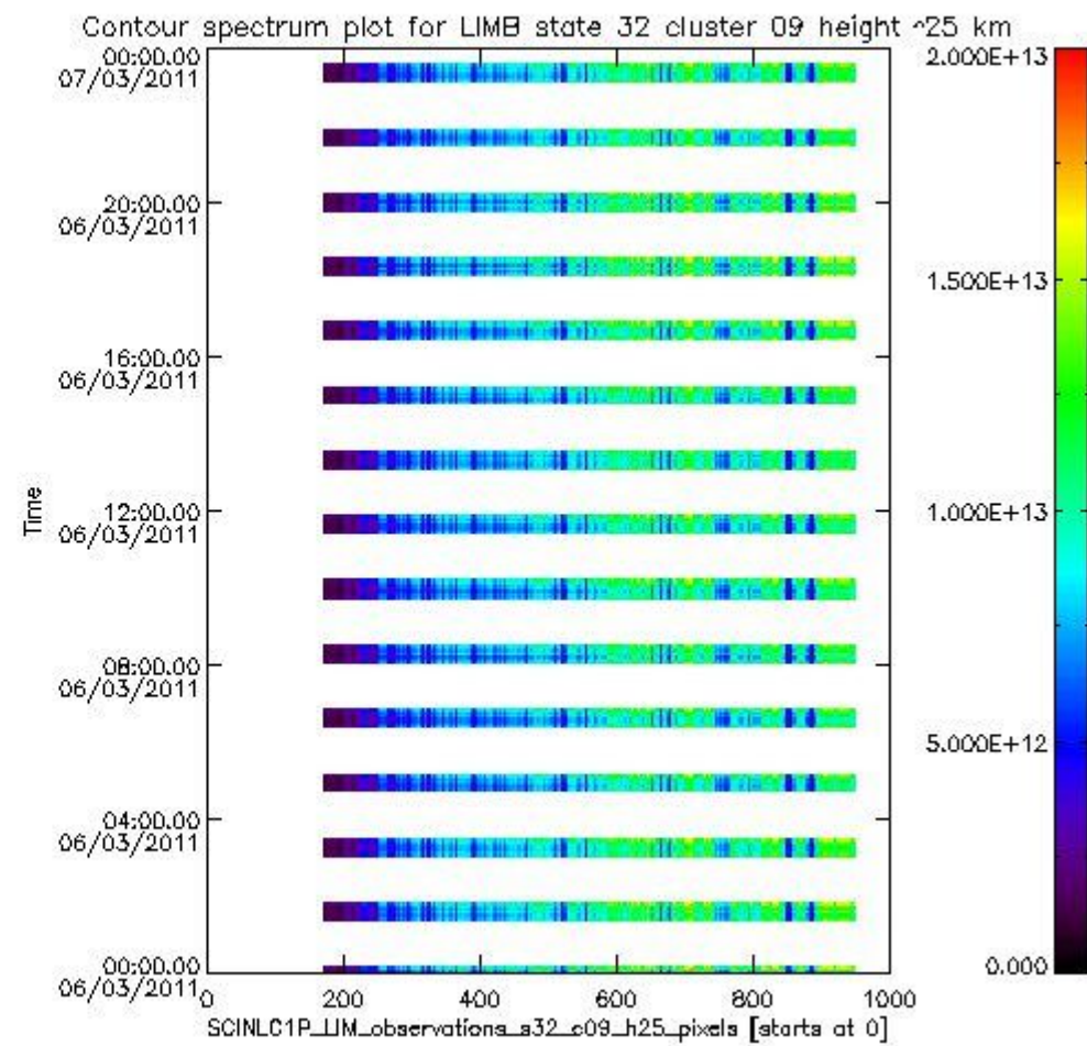
sciamachy_l1b_source_packet_report_SCIA_7_04_U_20110306_14.PNG
