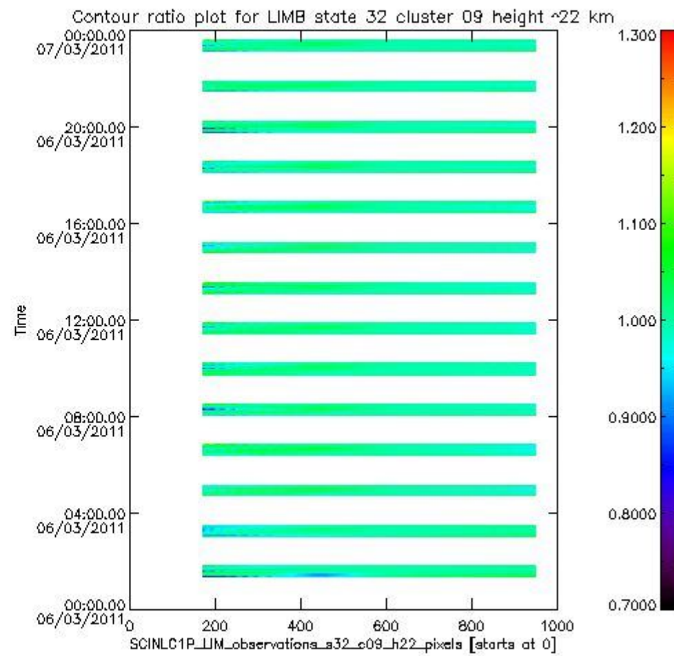
sciamachy_l1b_source_packet_report_SCIA_7_04_U_20110306_13.PNG
