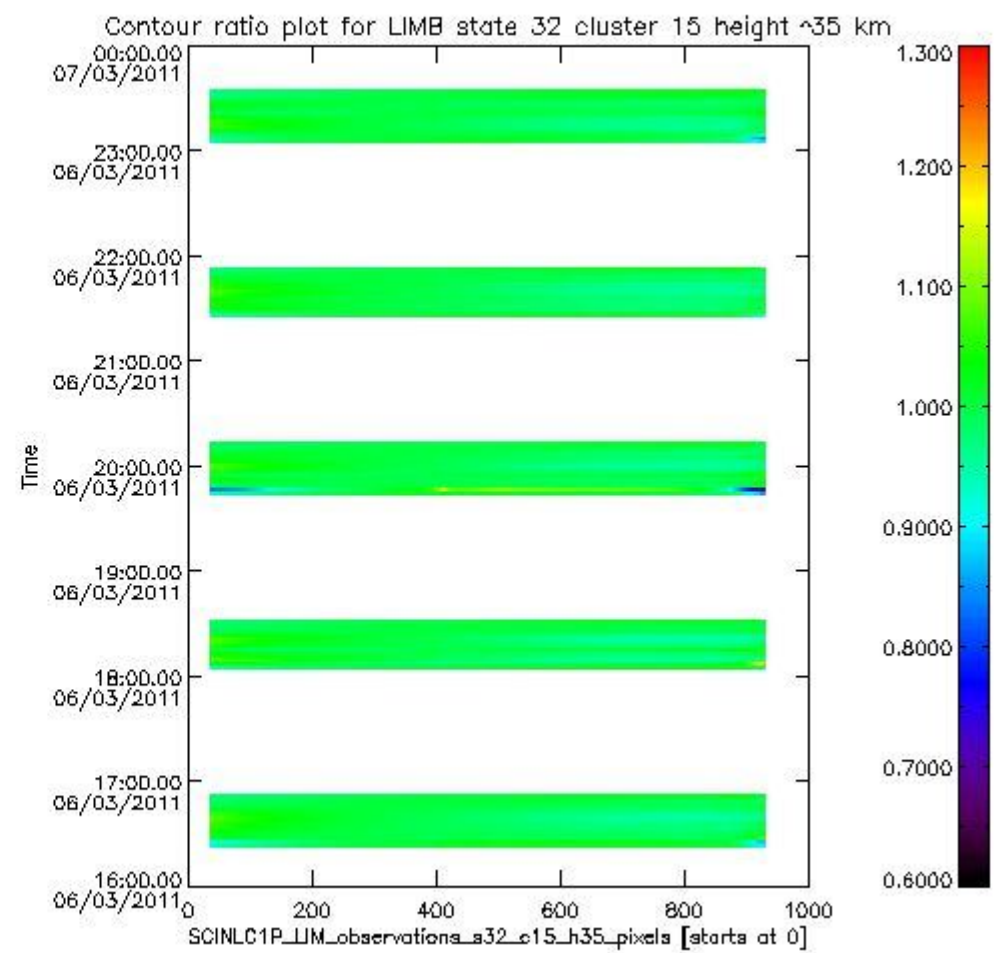
sciamachy_11b_source_packet_report_SCIA_7_04_U_20110306_21.PNG
