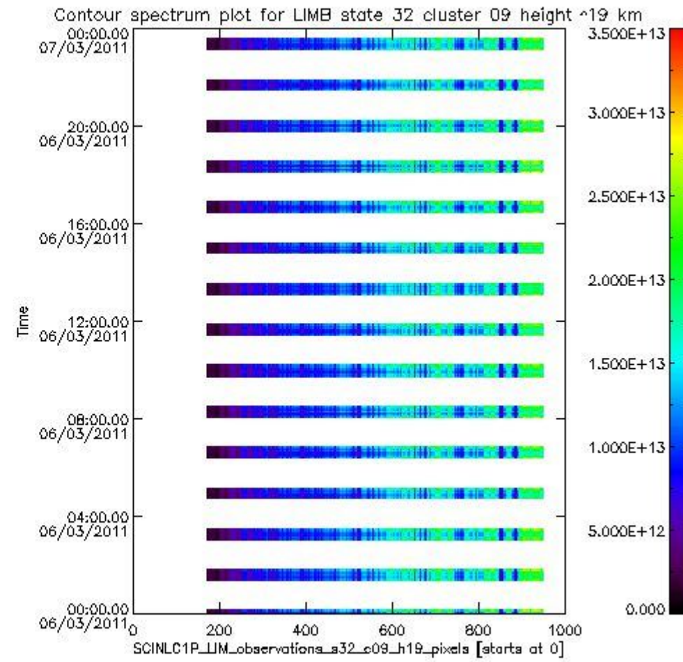
sciamachy_l1b_source_packet_report_SCIA_7_04_U_20110306_10.PNG
