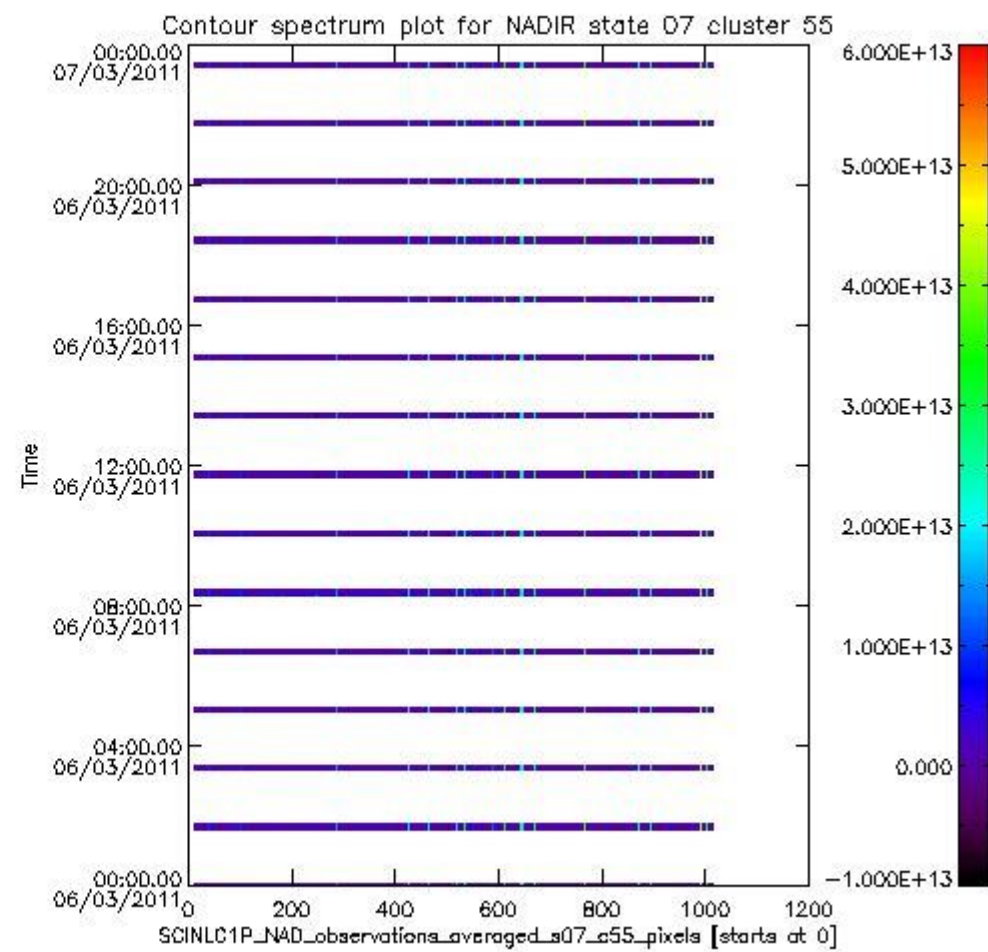
sciamachy_i1b_source_packet_report_SCIA_7_04_U_20110306_8.PNG
