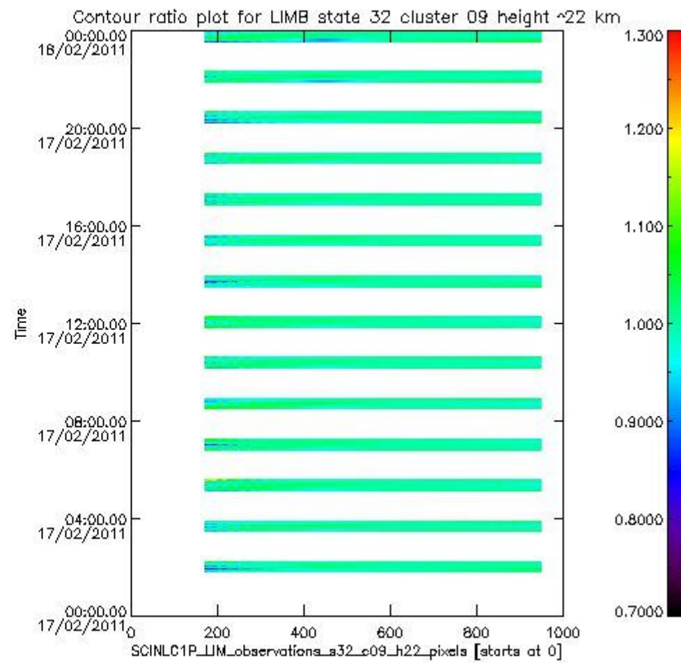
sciamachy_l1b_source_packet_report_SCIA_7_04_U_20110217_13.PNG
