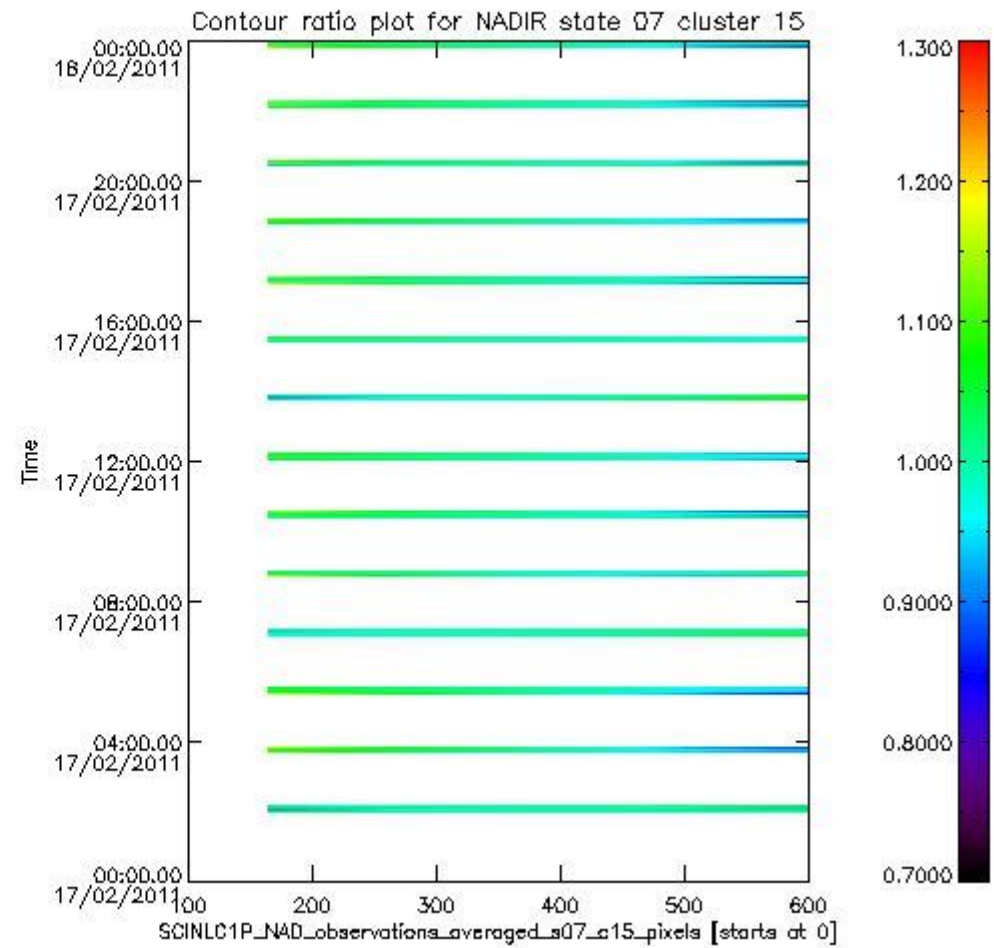
sciamachy_l1b_source_packet_report_SCIA_7_04_U_20110217_5.PNG
