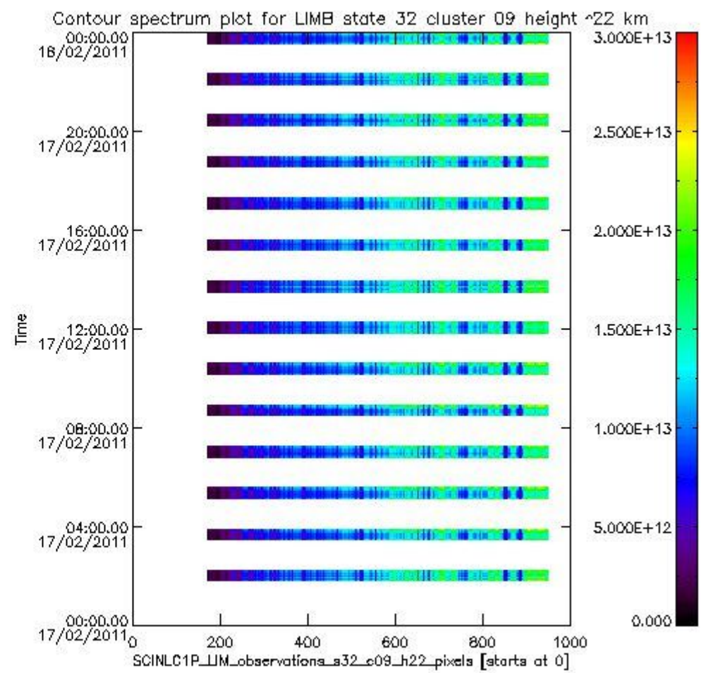
sciamachy_l1b_source_packet_report_SCIA_7_04_U_20110217_12.PNG
