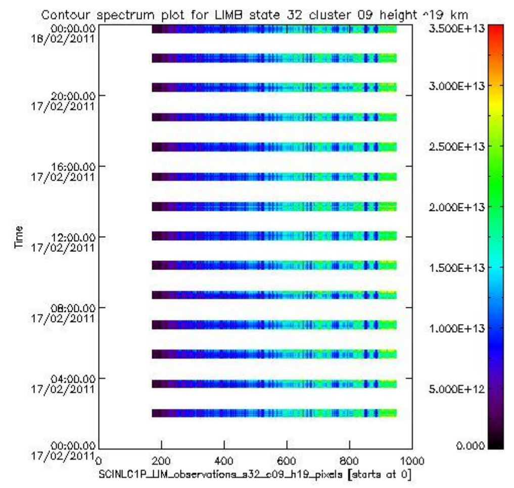
sciamachy_l1b_source_packet_report_SCIA_7_04_U_20110217_10.PNG
