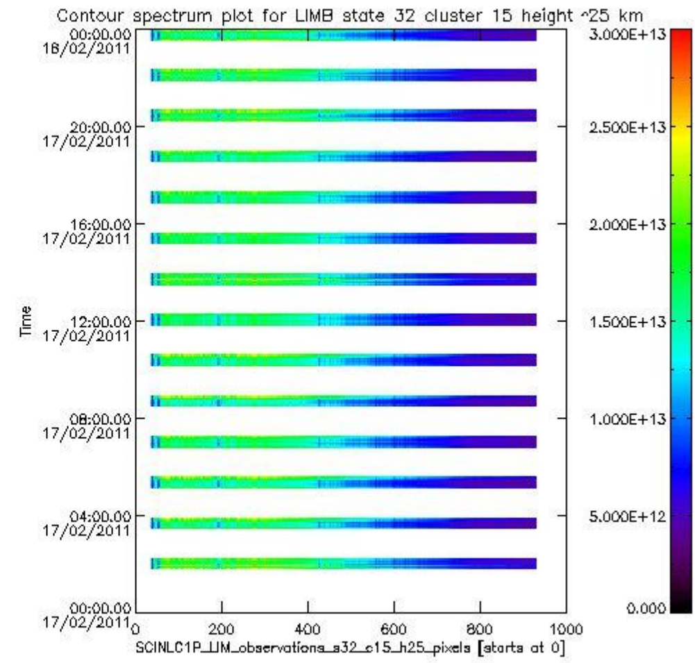
sciamachy_l1b_source_packet_report_SCIA_7_04_U_20110217_18.PNG
