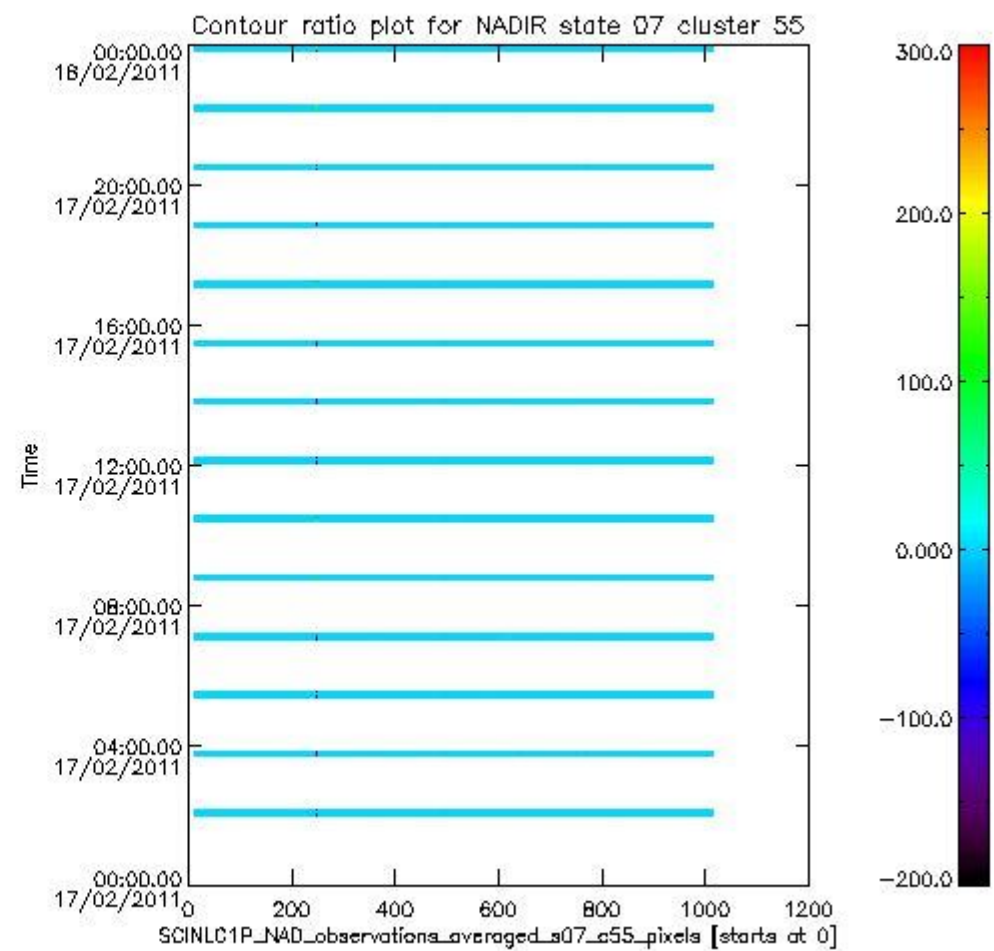
sciamachy_l1b_source_packet_report_SCIA_7_04_U_20110217_9.PNG
