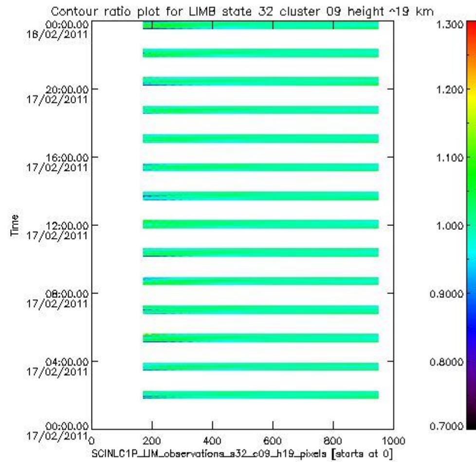
sciamachy_l1b_source_packet_report_SCIA_7_04_U_20110217_11.PNG
