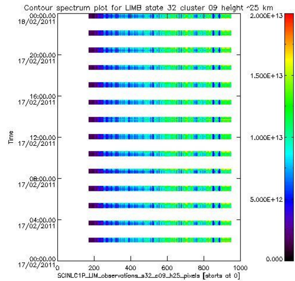
sciamachy_l1b_source_packet_report_SCIA_7_04_U_20110217_14.PNG
