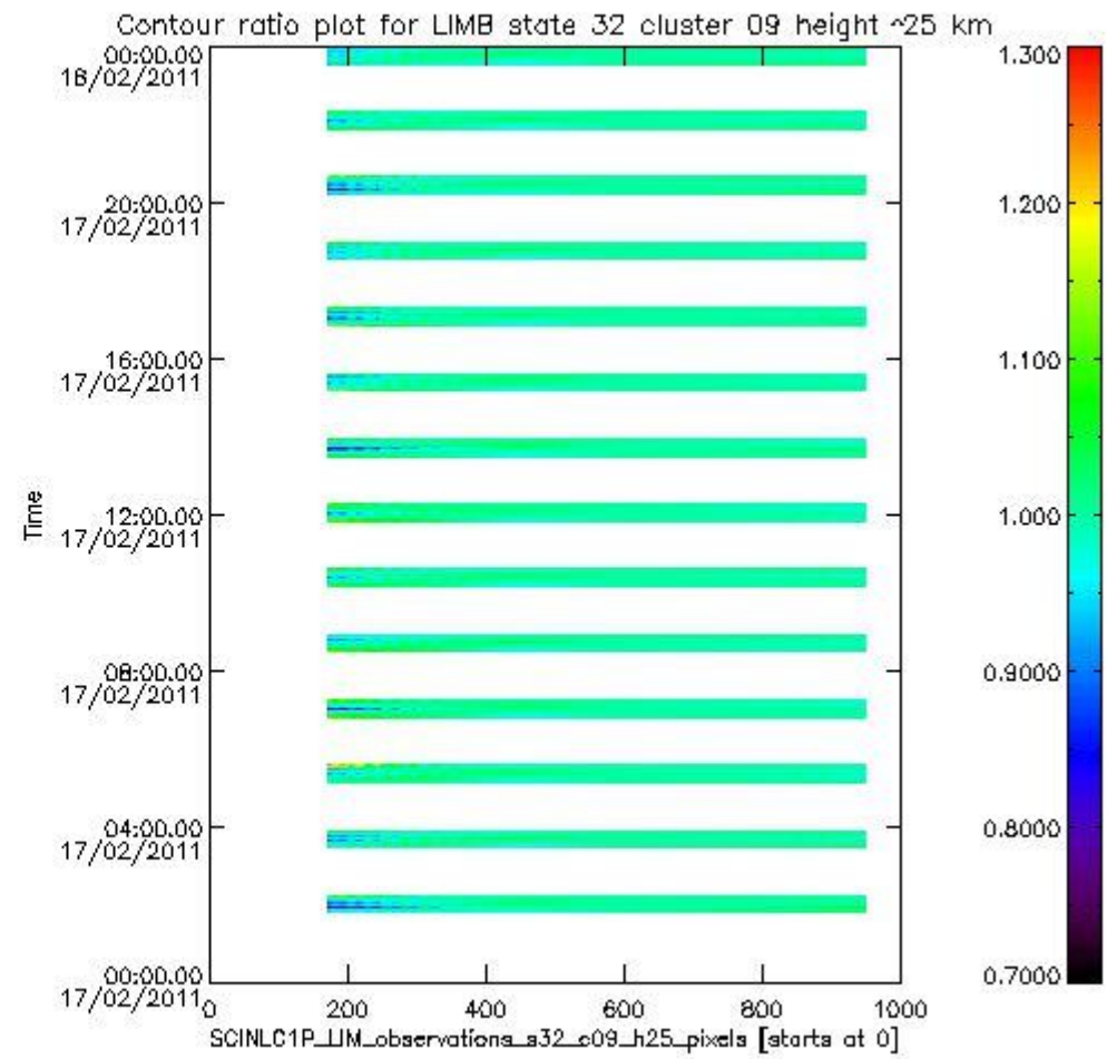
sciamachy_l1b_source_packet_report_SCIA_7_04_U_20110217_15.PNG
