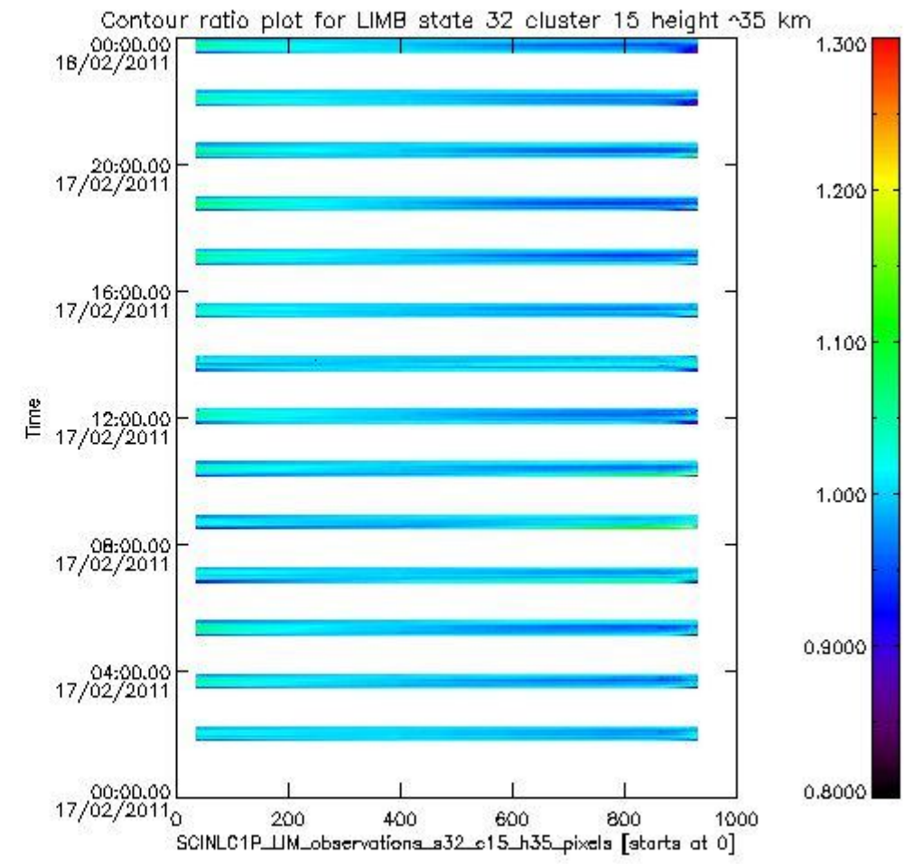
sciamachy_i1b_source_packet_report_SCIA_7_04_U_20110217_21.PNG
