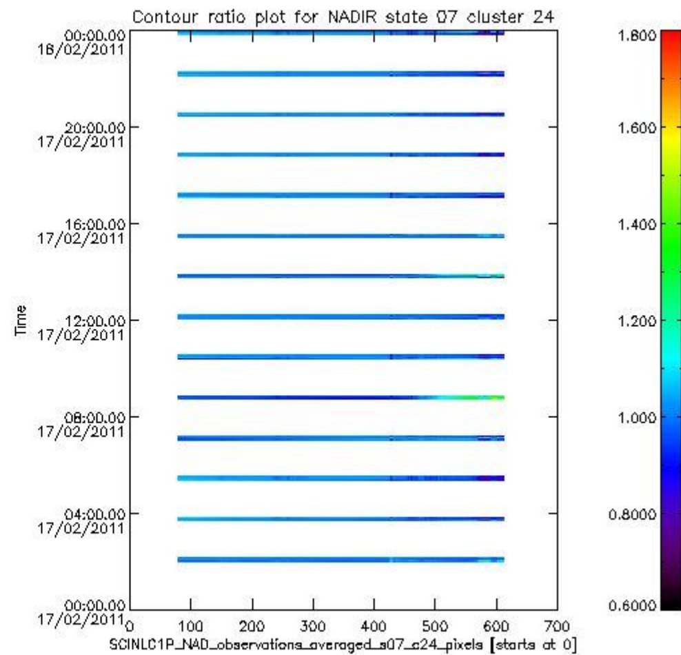
sciamachy_l1b_source_packet_report_SCIA_7_04_U_20110217_7.PNG
