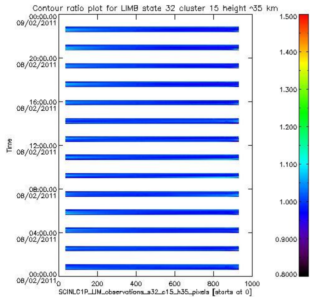
sciamachy_11b_source_packet_report_SCIA_7_04_U_20110208_21.PNG
