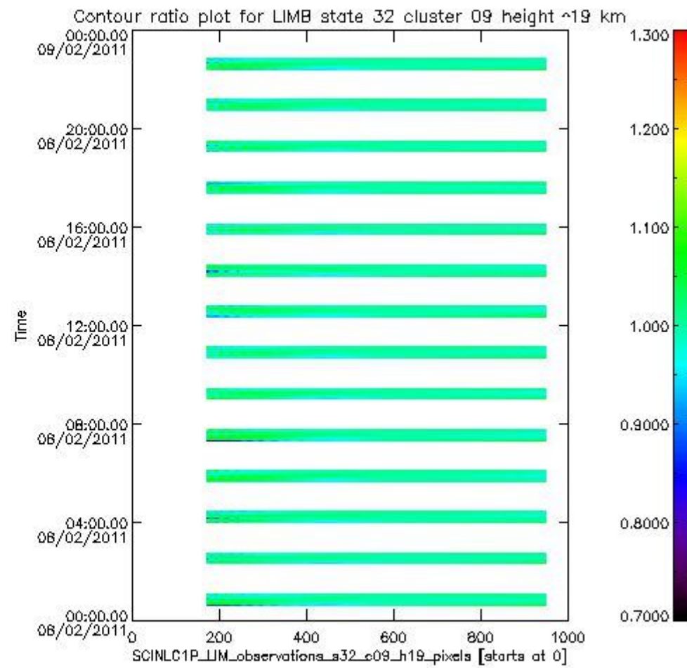
sciamachy_l1b_source_packet_report_SCIA_7_04_U_20110208_11.PNG
