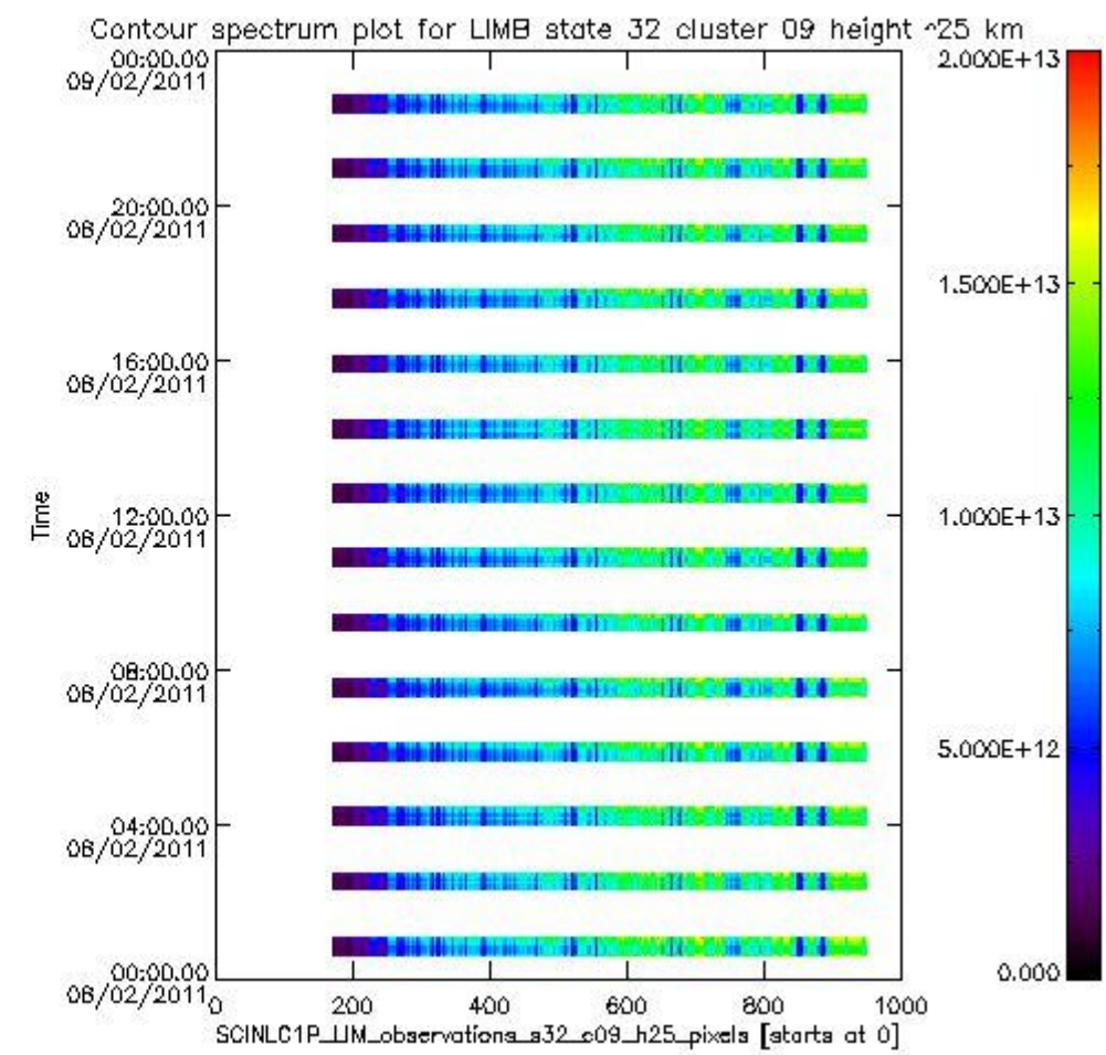
sciamachy_l1b_source_packet_report_SCIA_7_04_U_20110208_14.PNG
