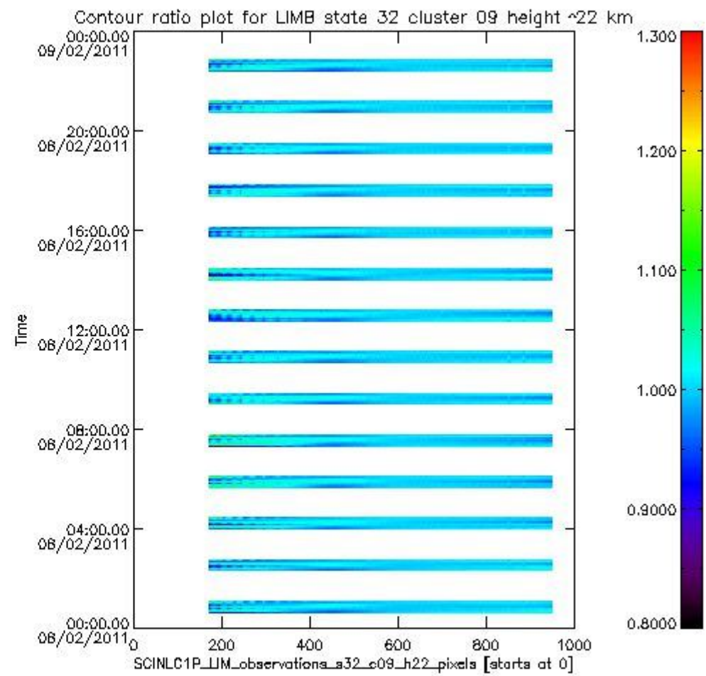
sciamachy_l1b_source_packet_report_SCIA_7_04_U_20110208_13.PNG
