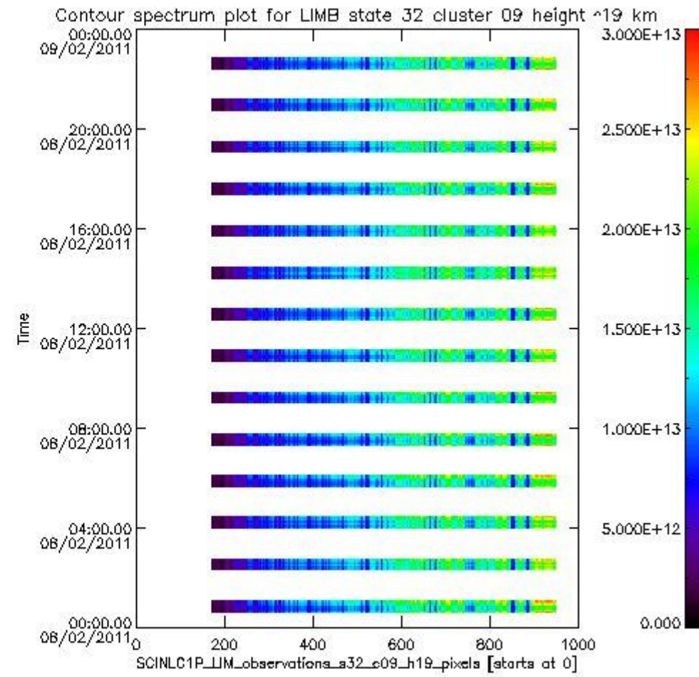
sciamachy_i1b_source_packet_report_SCIA_7_04_U_20110208_10.PNG
