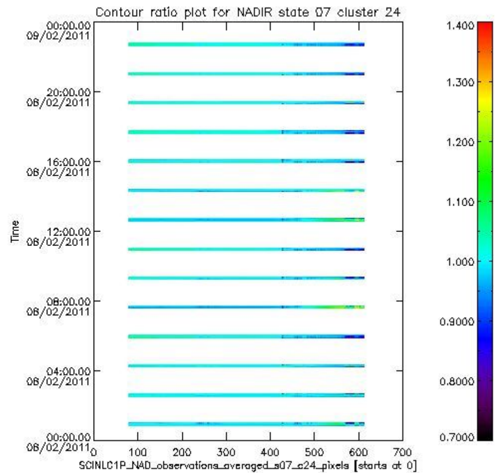
sciamachy_l1b_source_packet_report_SCIA_7_04_U_20110208_7.PNG
