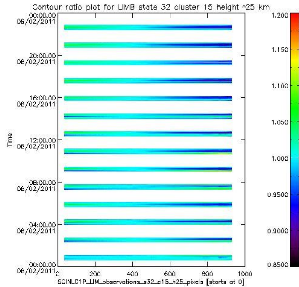
sciamachy_11b_source_packet_report_SCIA_7_04_U_20110208_19.PNG
