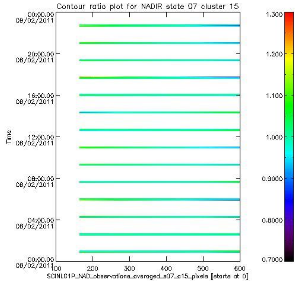
sciamachy_l1b_source_packet_report_SCIA_7_04_U_20110208_5.PNG
