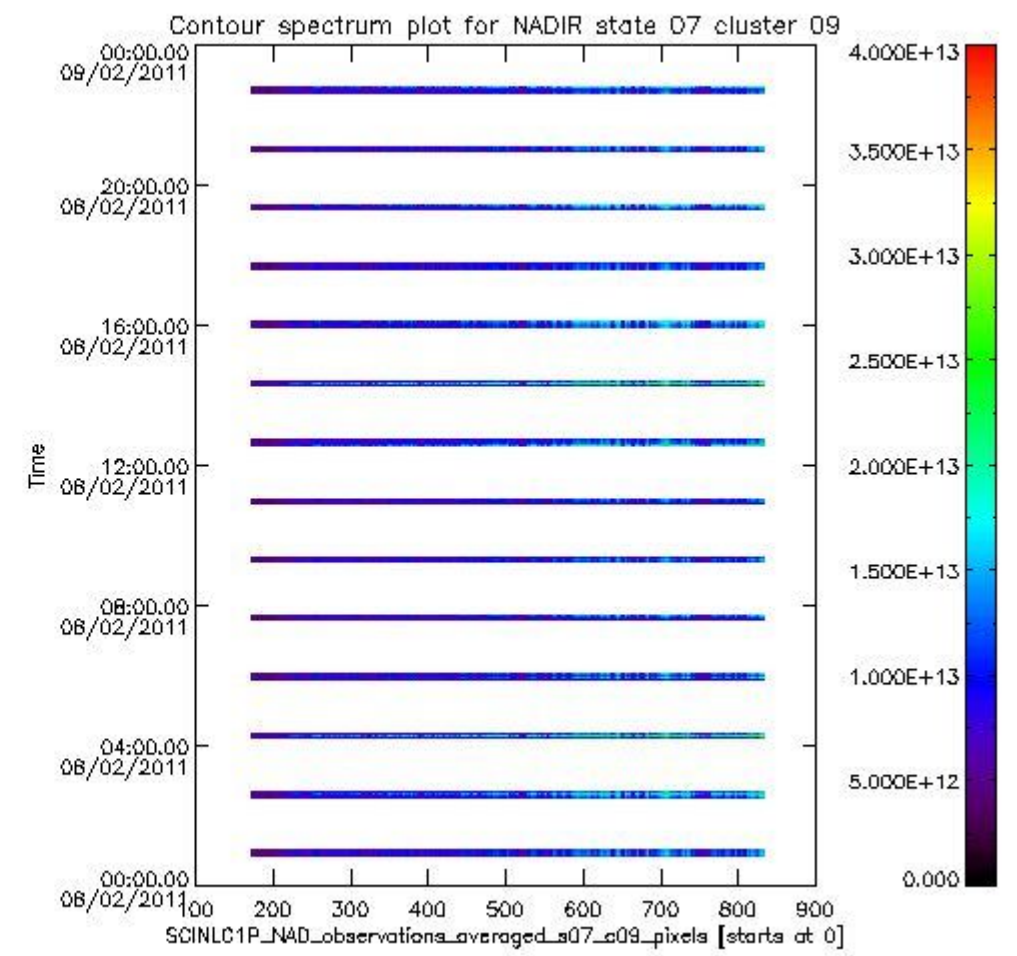
sciamachy_i1b_source_packet_report_SCIA_7_04_U_20110208_2.PNG
