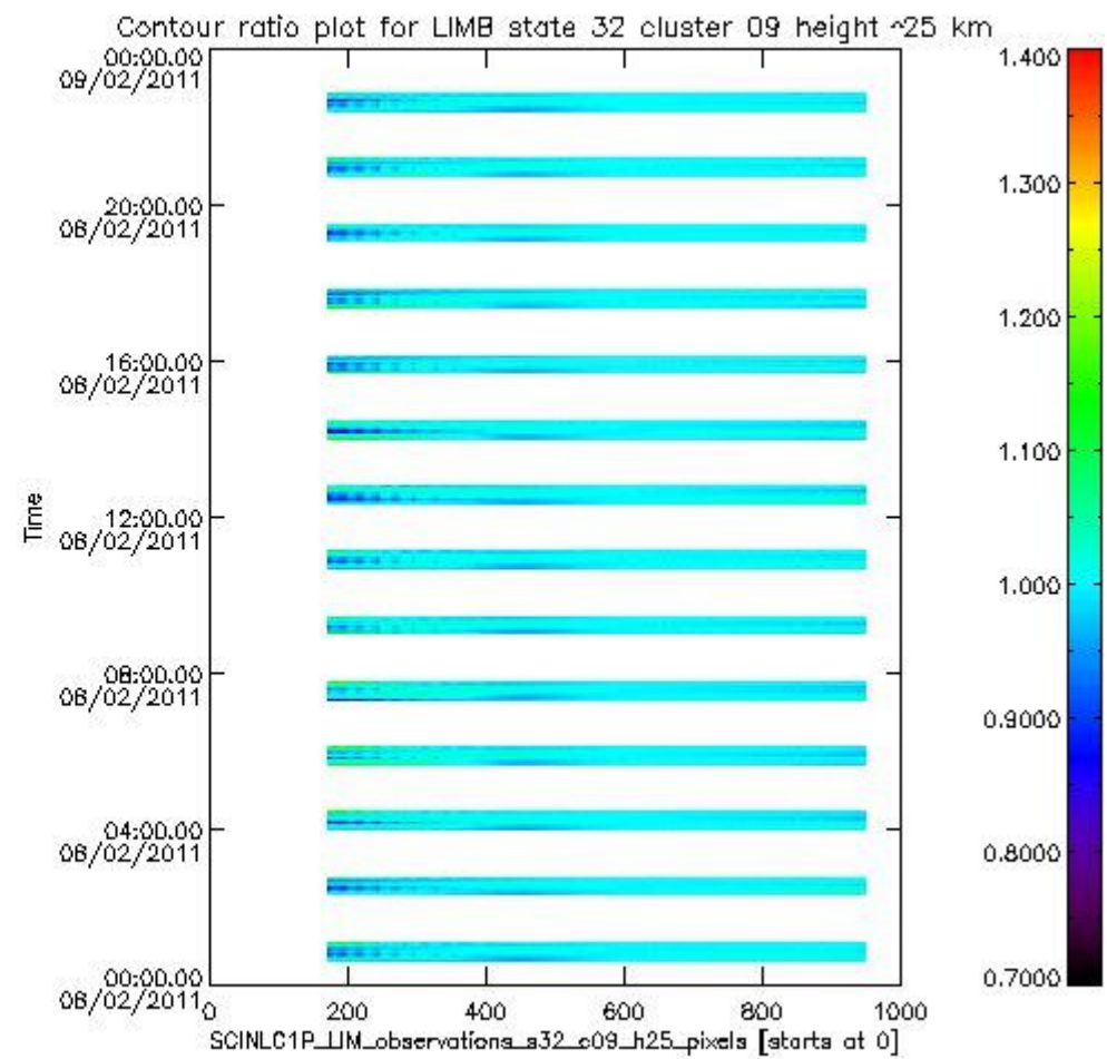
sciamachy_l1b_source_packet_report_SCIA_7_04_U_20110208_15.PNG
