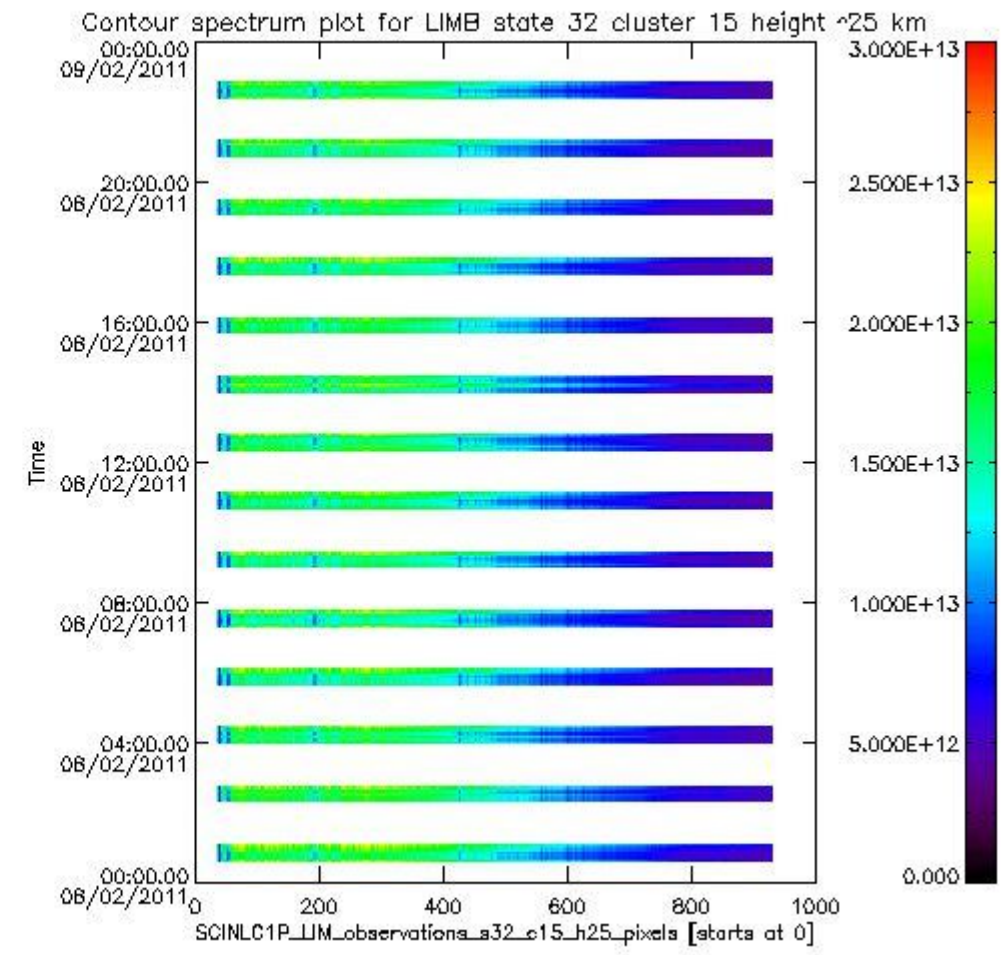
sciamachy_l1b_source_packet_report_SCIA_7_04_U_20110208_18.PNG
