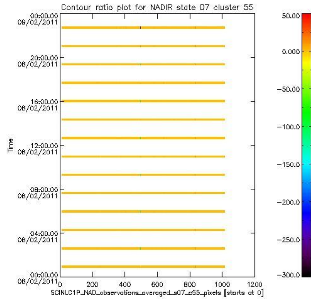
sciamachy_l1b_source_packet_report_SCIA_7_04_U_20110208_9.PNG
