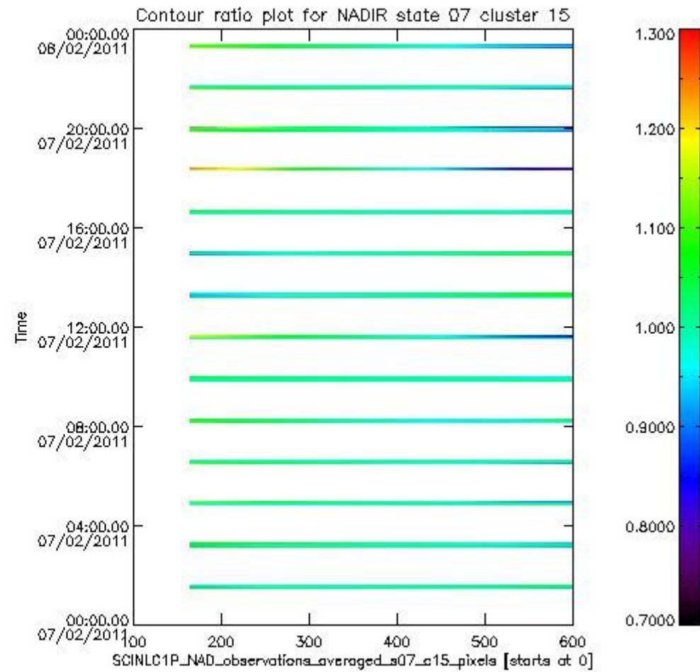
sciamachy_l1b_source_packet_report_SCIA_7_04_U_20110207_5.PNG
