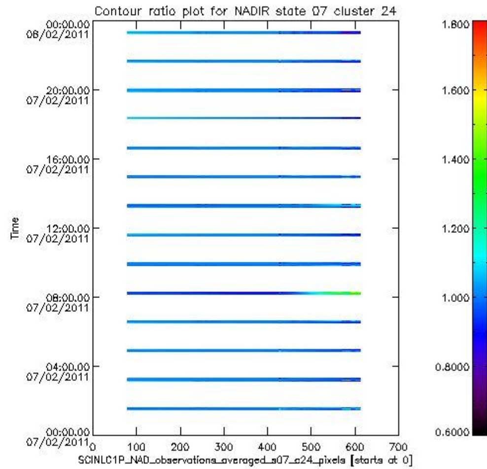
sciamachy_l1b_source_packet_report_SCIA_7_04_U_20110207_7.PNG
