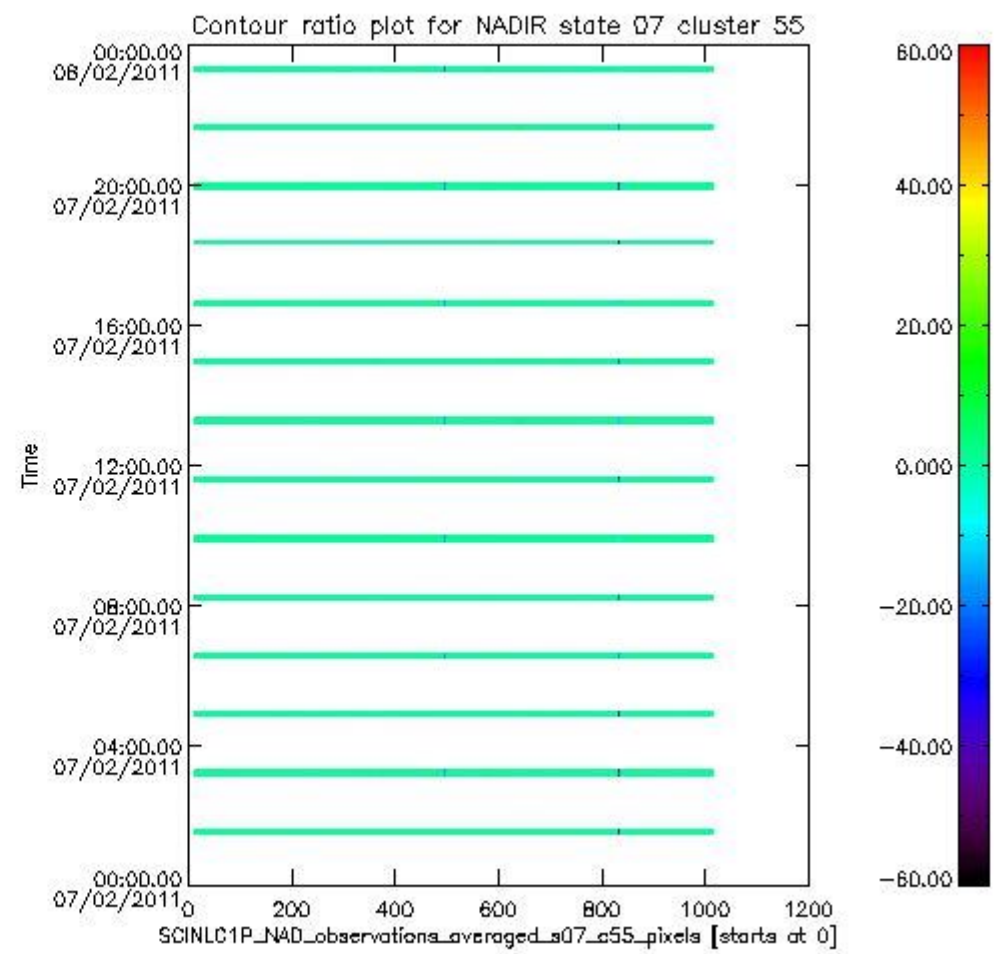
sciamachy_l1b_source_packet_report_SCIA_7_04_U_20110207_9.PNG
