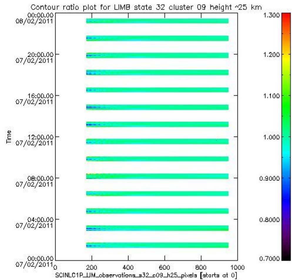
sciamachy_l1b_source_packet_report_SCIA_7_04_U_20110207_15.PNG
