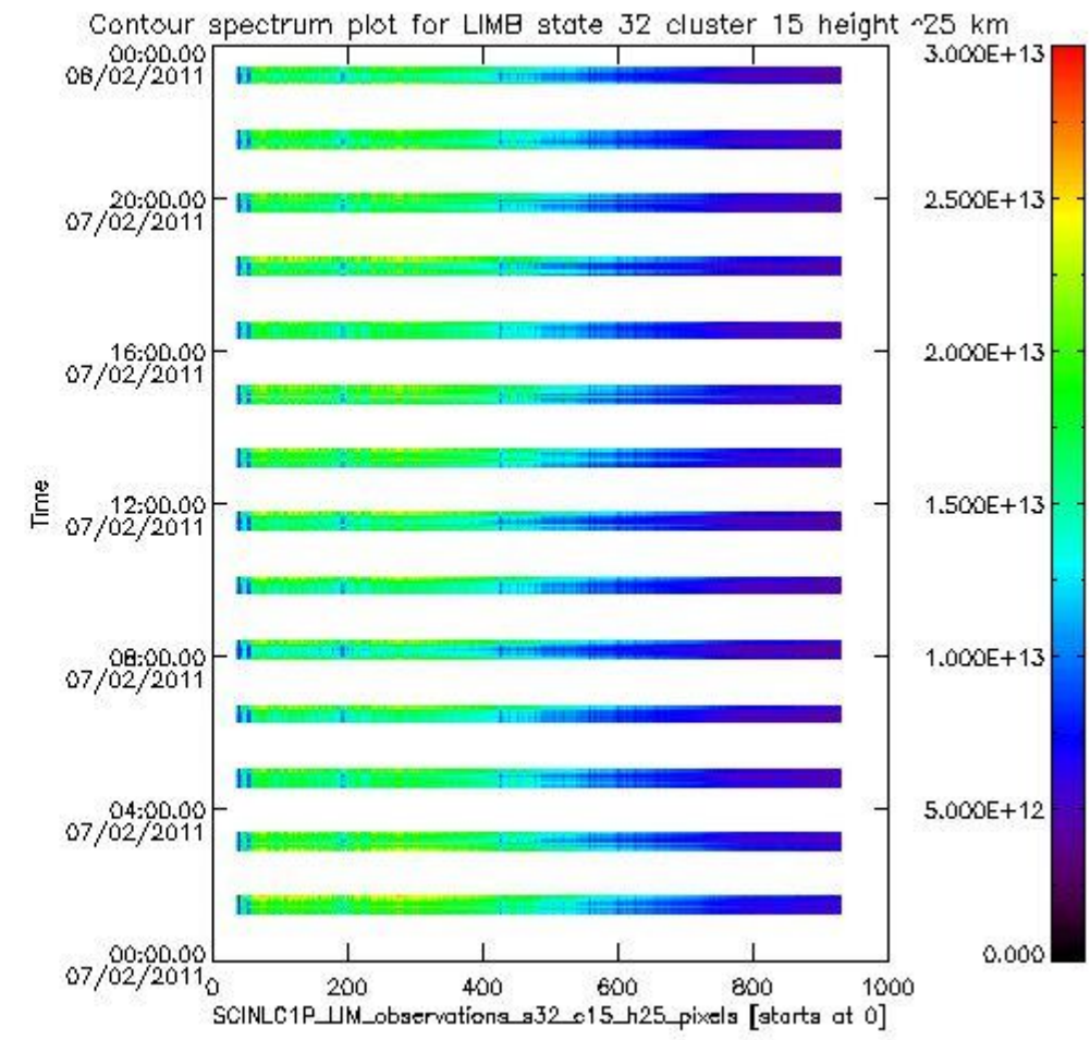
sciamachy_l1b_source_packet_report_SCIA_7_04_U_20110207_18.PNG
