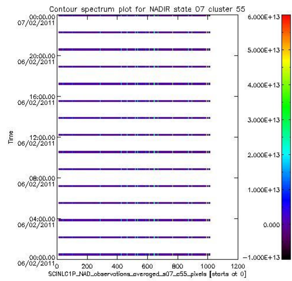
sciamachy_i1b_source_packet_report_SCIA_7_04_U_20110206_8.PNG
