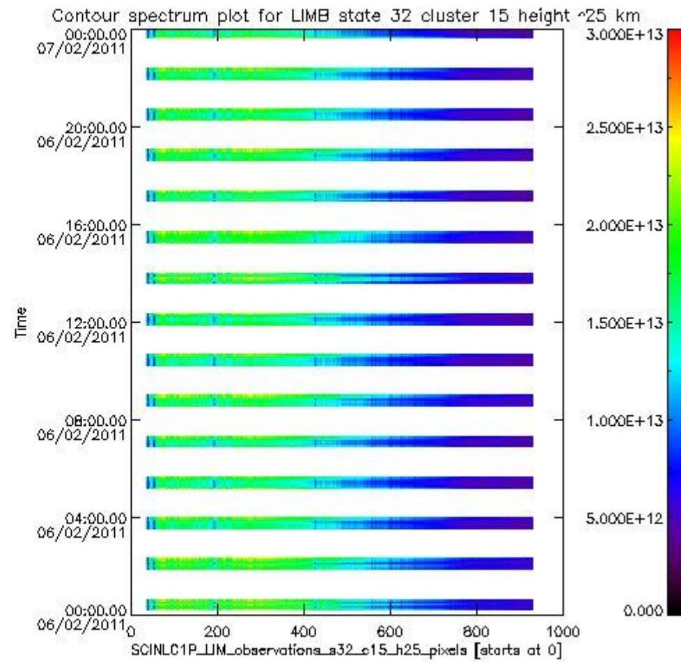
sciamachy_l1b_source_packet_report_SCIA_7_04_U_20110206_18.PNG
