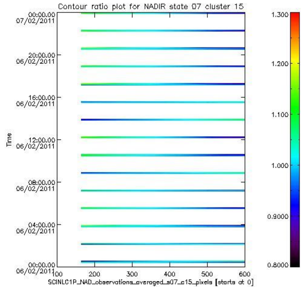
sciamachy_l1b_source_packet_report_SCIA_7_04_U_20110206_5.PNG
