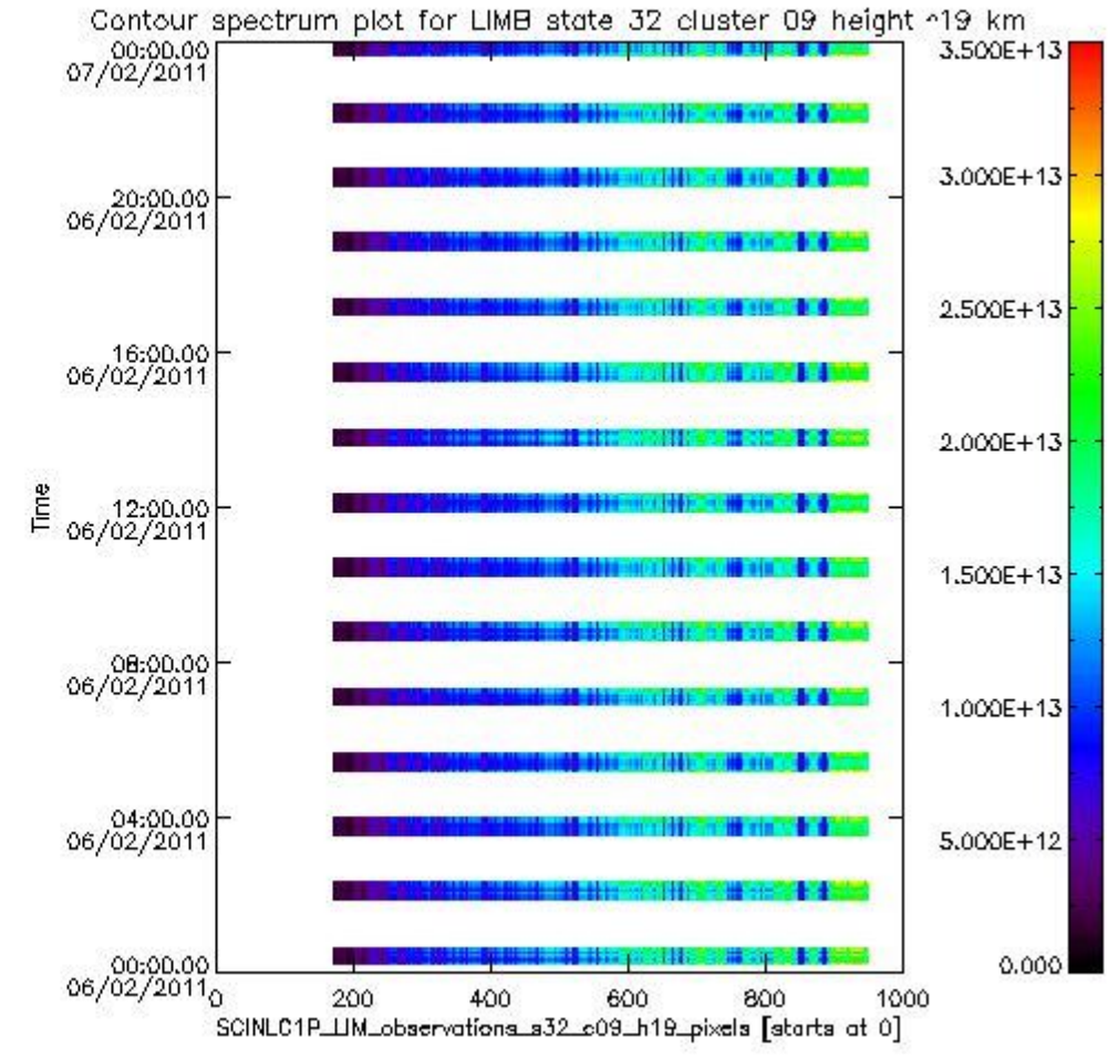
sciamachy_l1b_source_packet_report_SCIA_7_04_U_20110206_10.PNG
