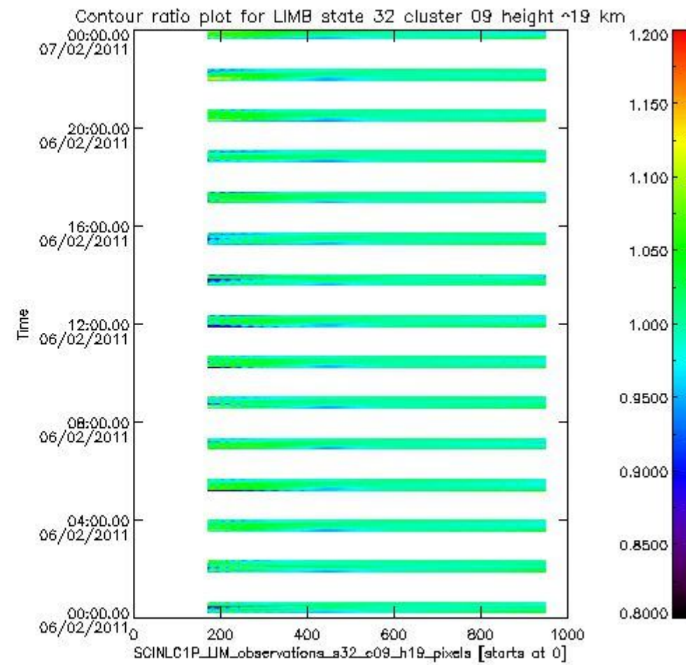
sciamachy_l1b_source_packet_report_SCIA_7_04_U_20110206_11.PNG
