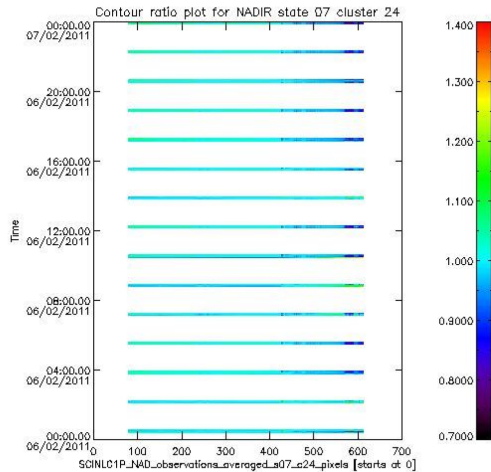
sciamachy_l1b_source_packet_report_SCIA_7_04_U_20110206_7.PNG
