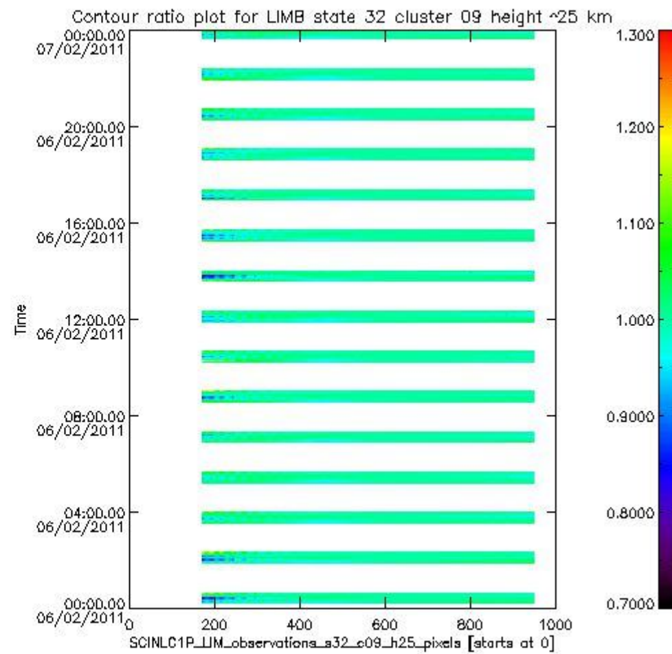
sciamachy_l1b_source_packet_report_SCIA_7_04_U_20110206_15.PNG
