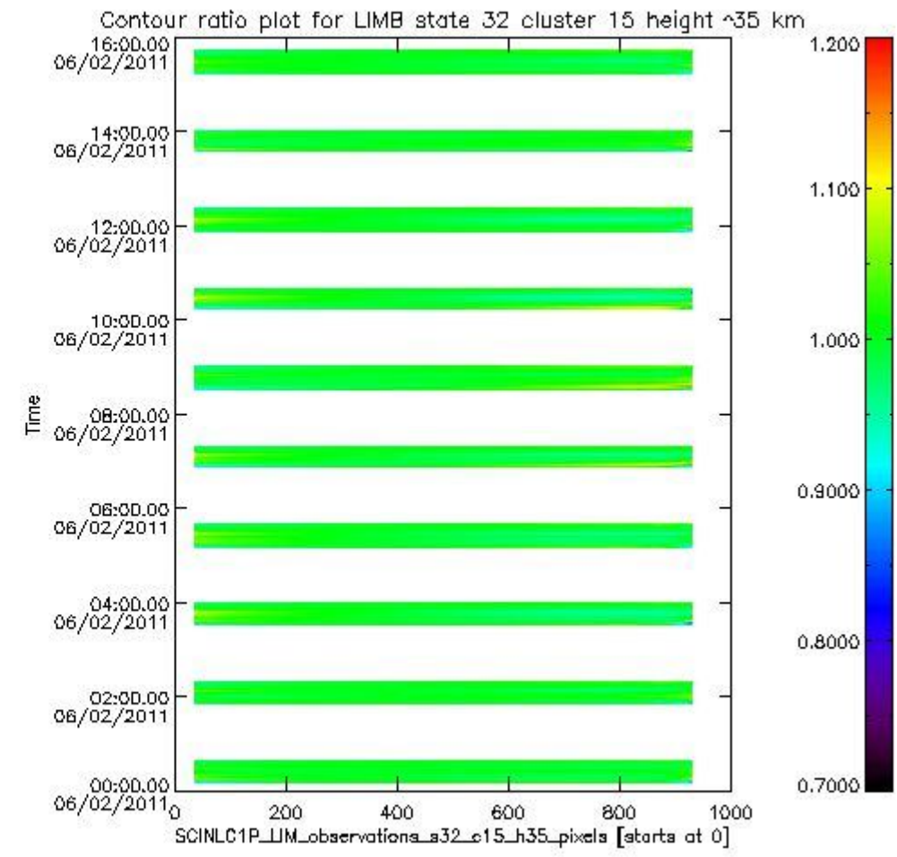
sciamachy_11b_source_packet_report_SCIA_7_04_U_20110206_21.PNG
