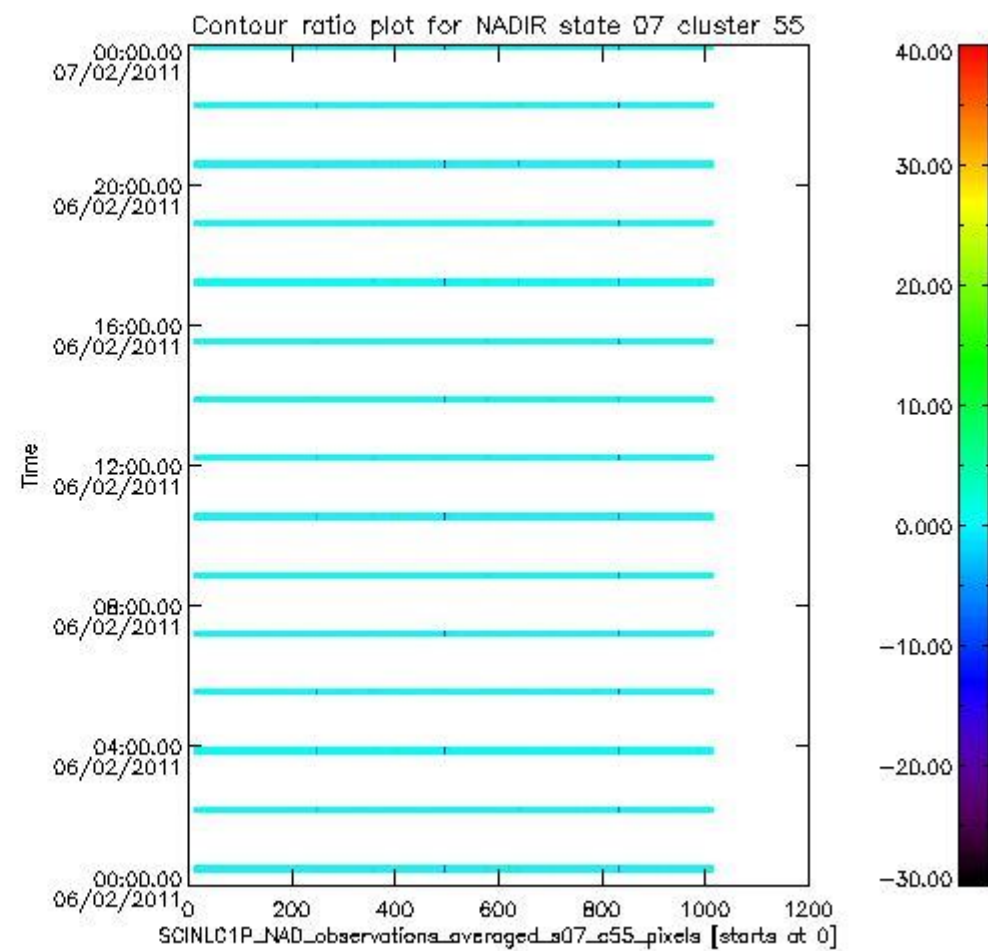
sciamachy_l1b_source_packet_report_SCIA_7_04_U_20110206_9.PNG
