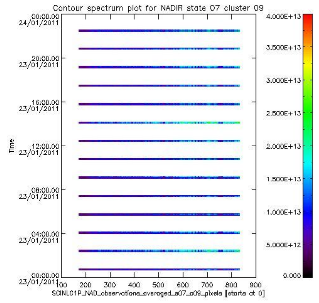
sciamachy_i1b_source_packet_report_SCIA_7_04_U_20110123_2.PNG
