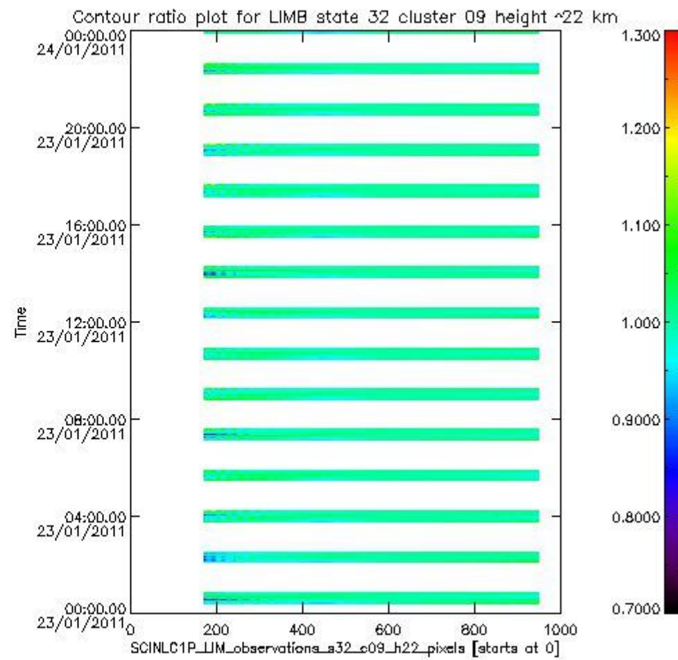
sciamachy_l1b_source_packet_report_SCIA_7_04_U_20110123_13.PNG
