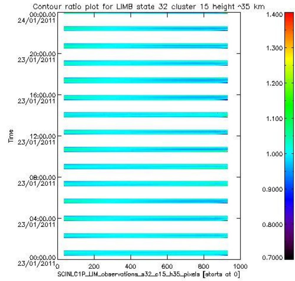
sciamachy_11b_source_packet_report_SCIA_7_04_U_20110123_21.PNG
