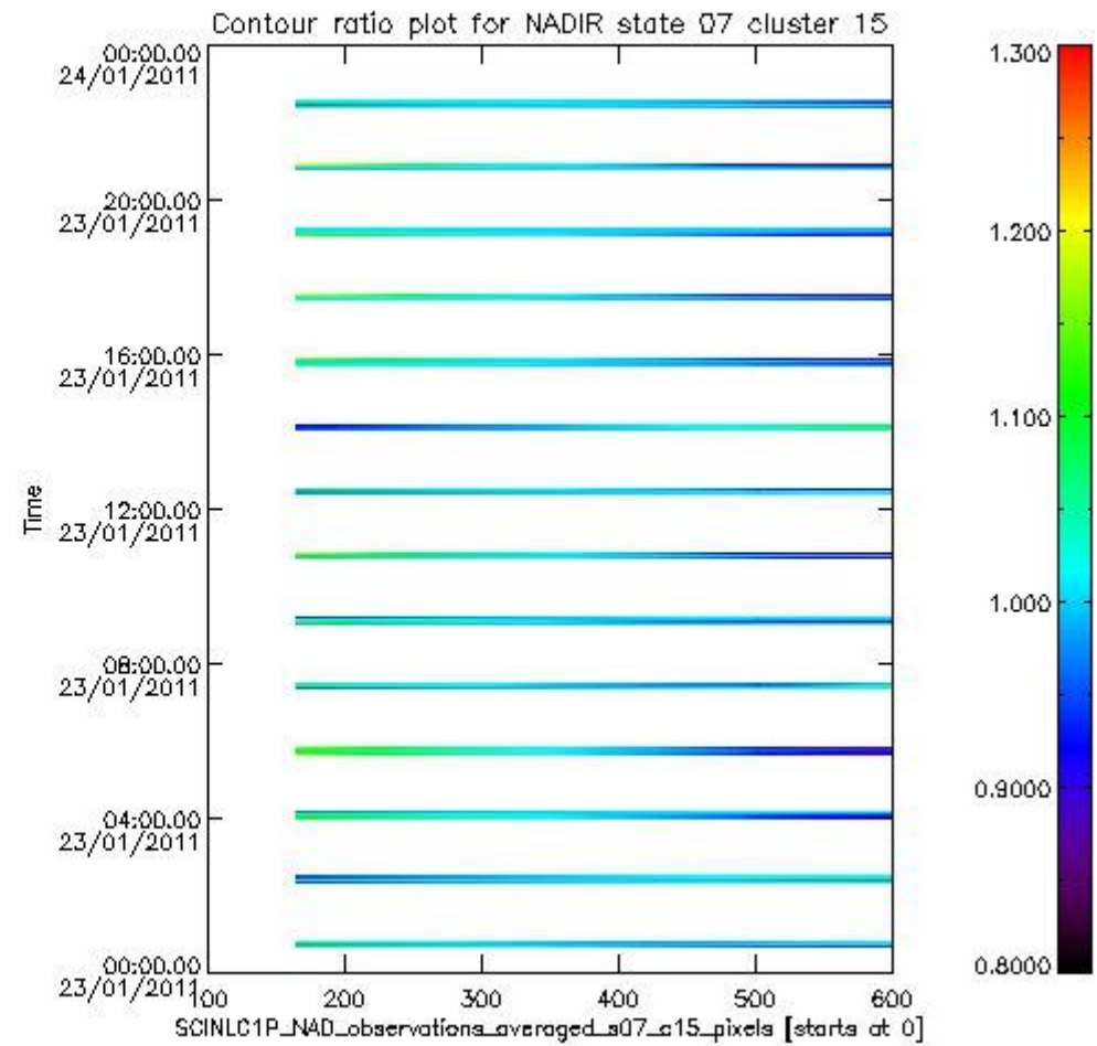
sciamachy_l1b_source_packet_report_SCIA_7_04_U_20110123_5.PNG
