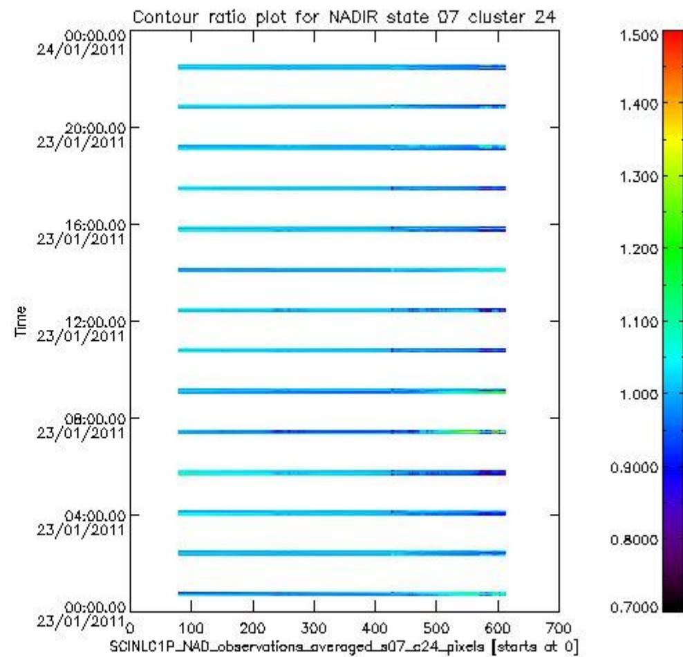
sciamachy_l1b_source_packet_report_SCIA_7_04_U_20110123_7.PNG
