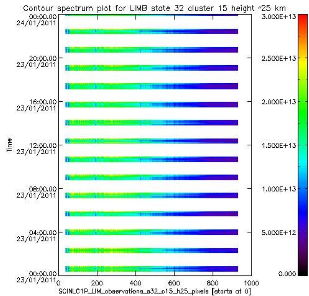
sciamachy_l1b_source_packet_report_SCIA_7_04_U_20110123_18.PNG
