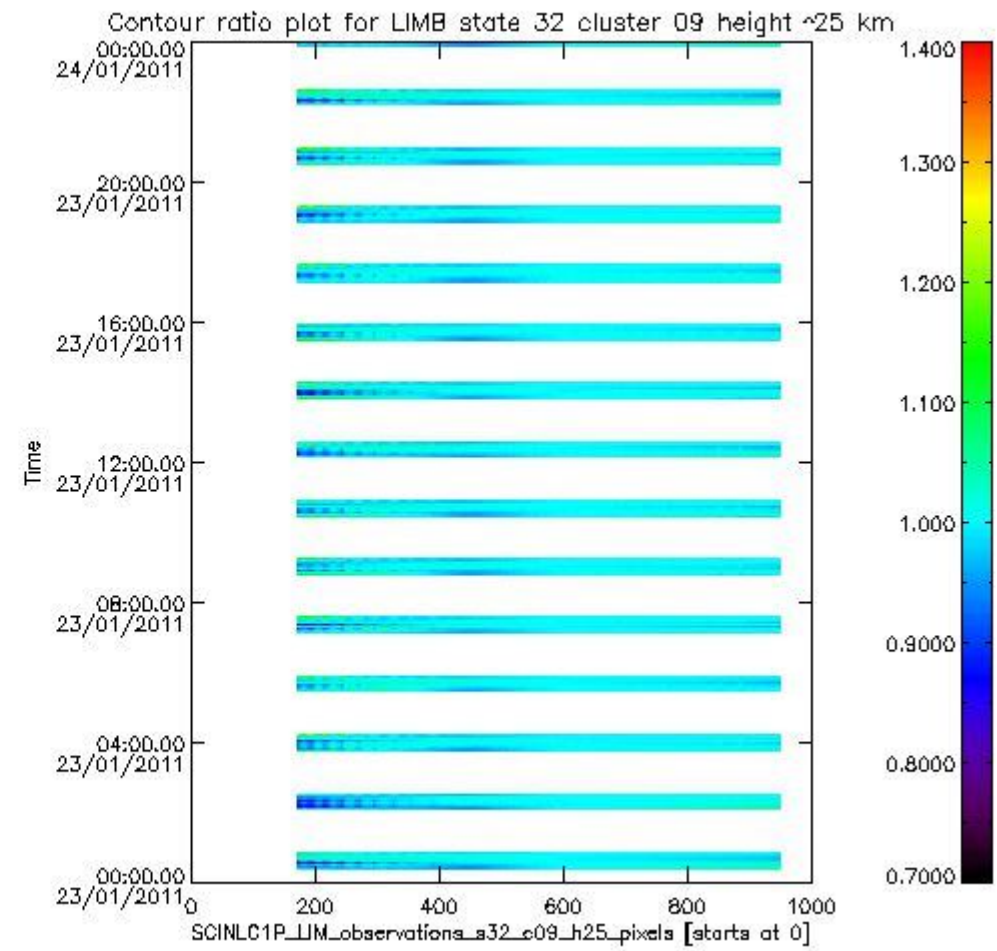
sciamachy_l1b_source_packet_report_SCIA_7_04_U_20110123_15.PNG
