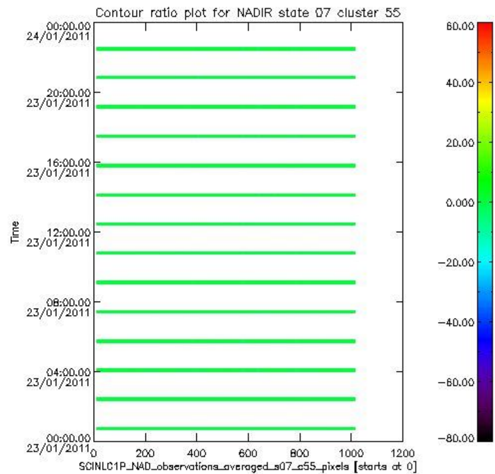
sciamachy_l1b_source_packet_report_SCIA_7_04_U_20110123_9.PNG
