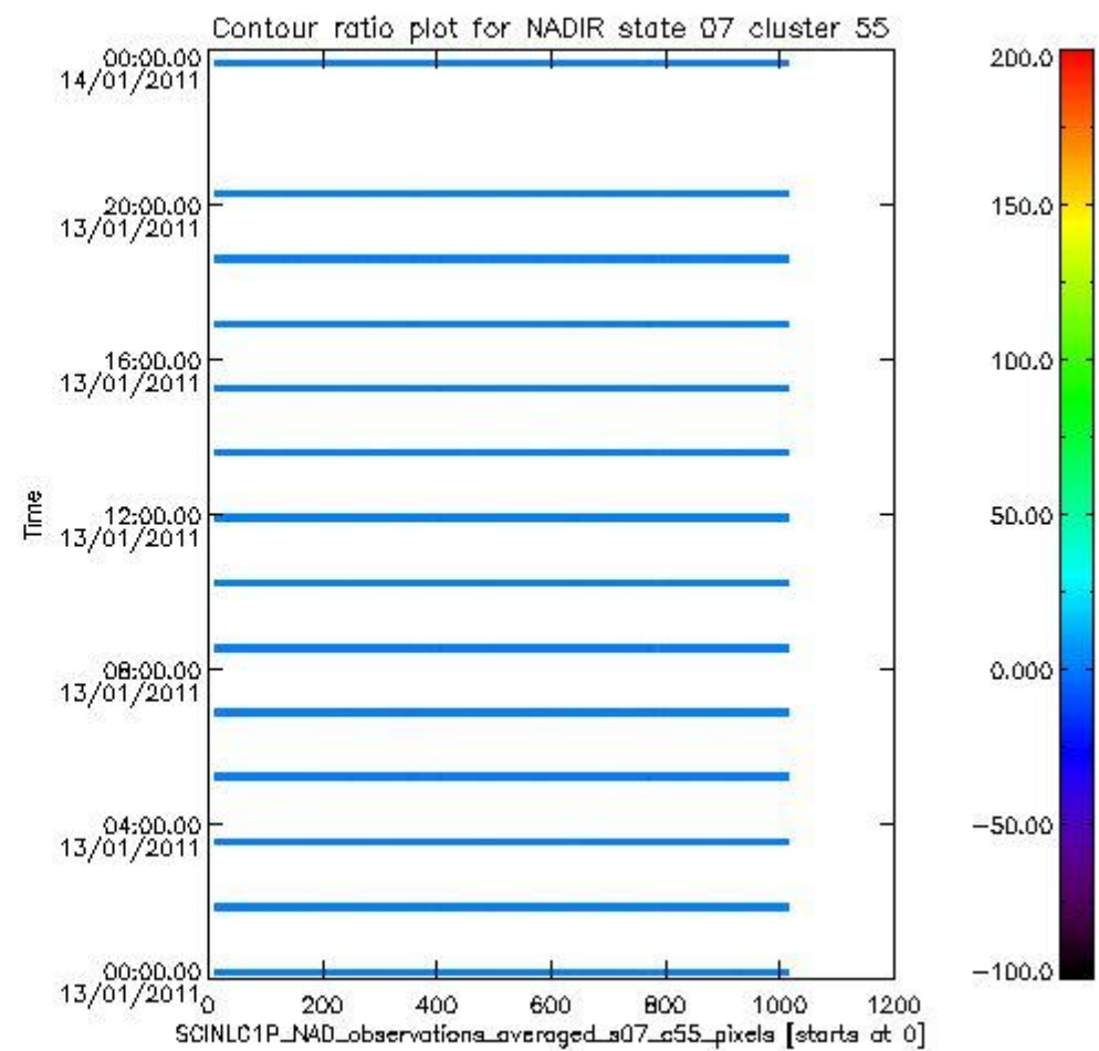
sciamachy_l1b_source_packet_report_SCIA_7_04_U_20110113_9.PNG
