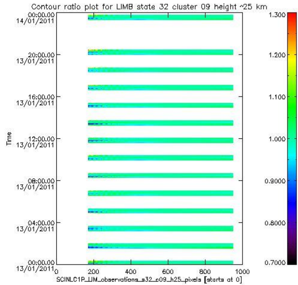
sciamachy_l1b_source_packet_report_SCIA_7_04_U_20110113_15.PNG
