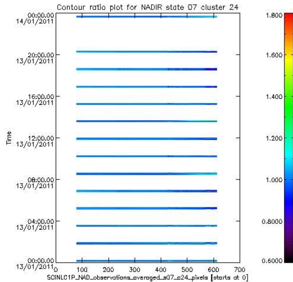
sciamachy_l1b_source_packet_report_SCIA_7_04_U_20110113_7.PNG
