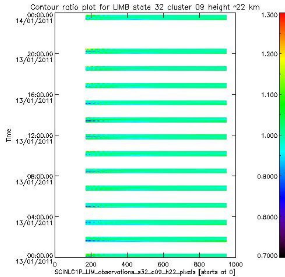
sciamachy_l1b_source_packet_report_SCIA_7_04_U_20110113_13.PNG
