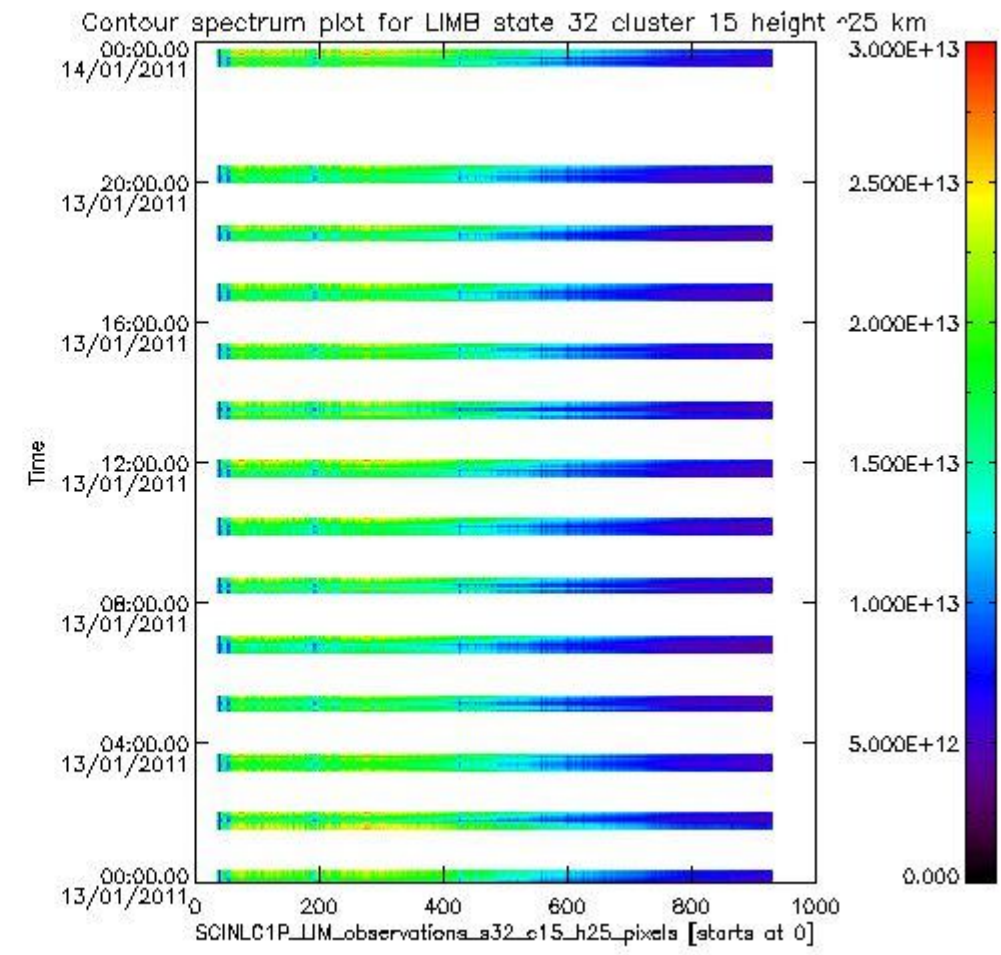
sciamachy_l1b_source_packet_report_SCIA_7_04_U_20110113_18.PNG
