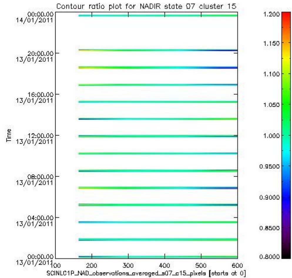
sciamachy_l1b_source_packet_report_SCIA_7_04_U_20110113_5.PNG
