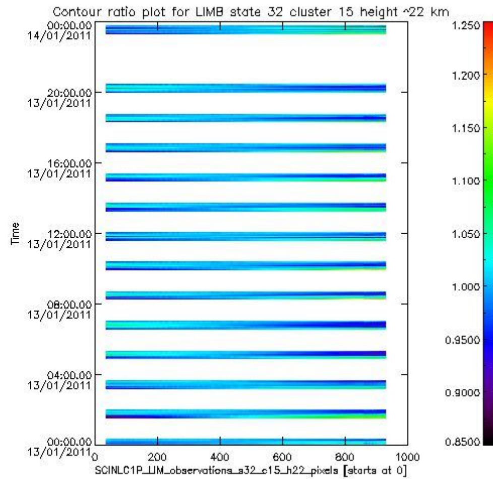
sciamachy_11b_source_packet_report_SCIA_7_04_U_20110113_17.PNG
