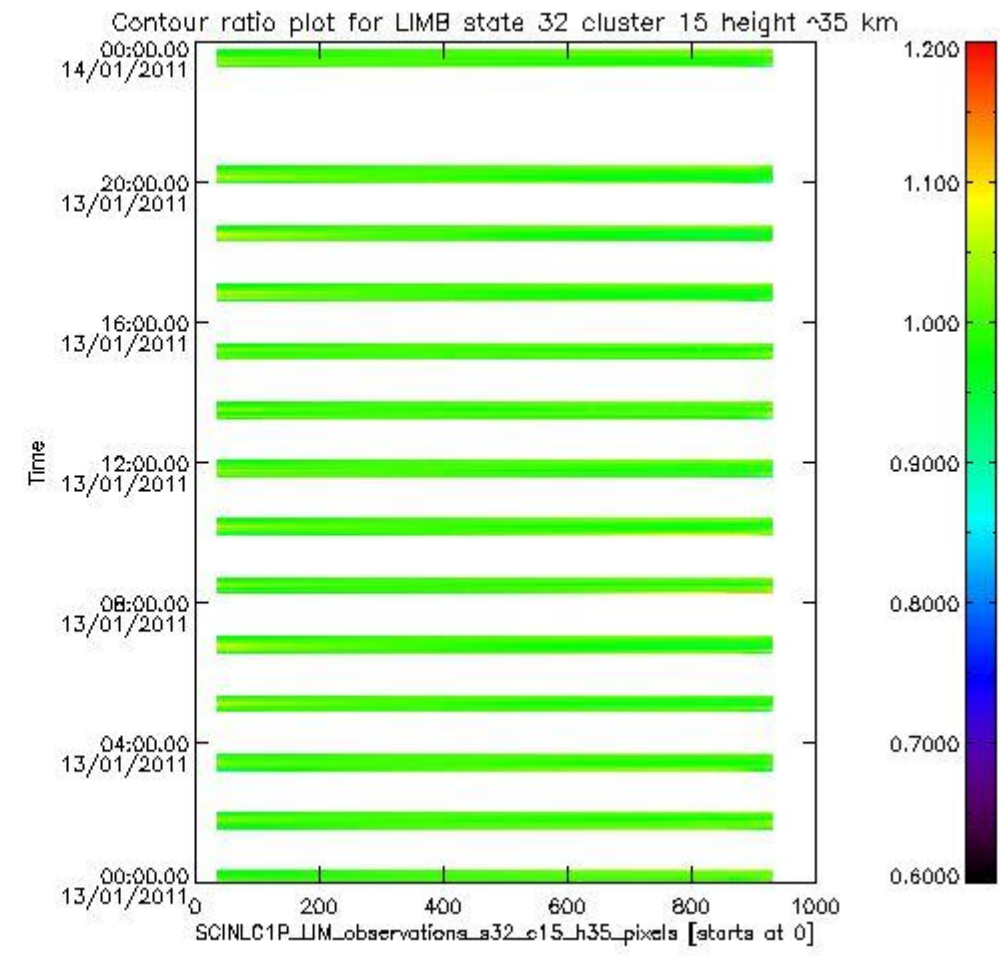
sciamachy_i1b_source_packet_report_SCIA_7_04_U_20110113_21.PNG
