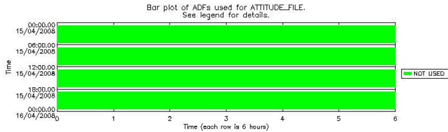
sciamachy_daily_report_level1_SCIA_6_03_N_20080415_50.PNG
