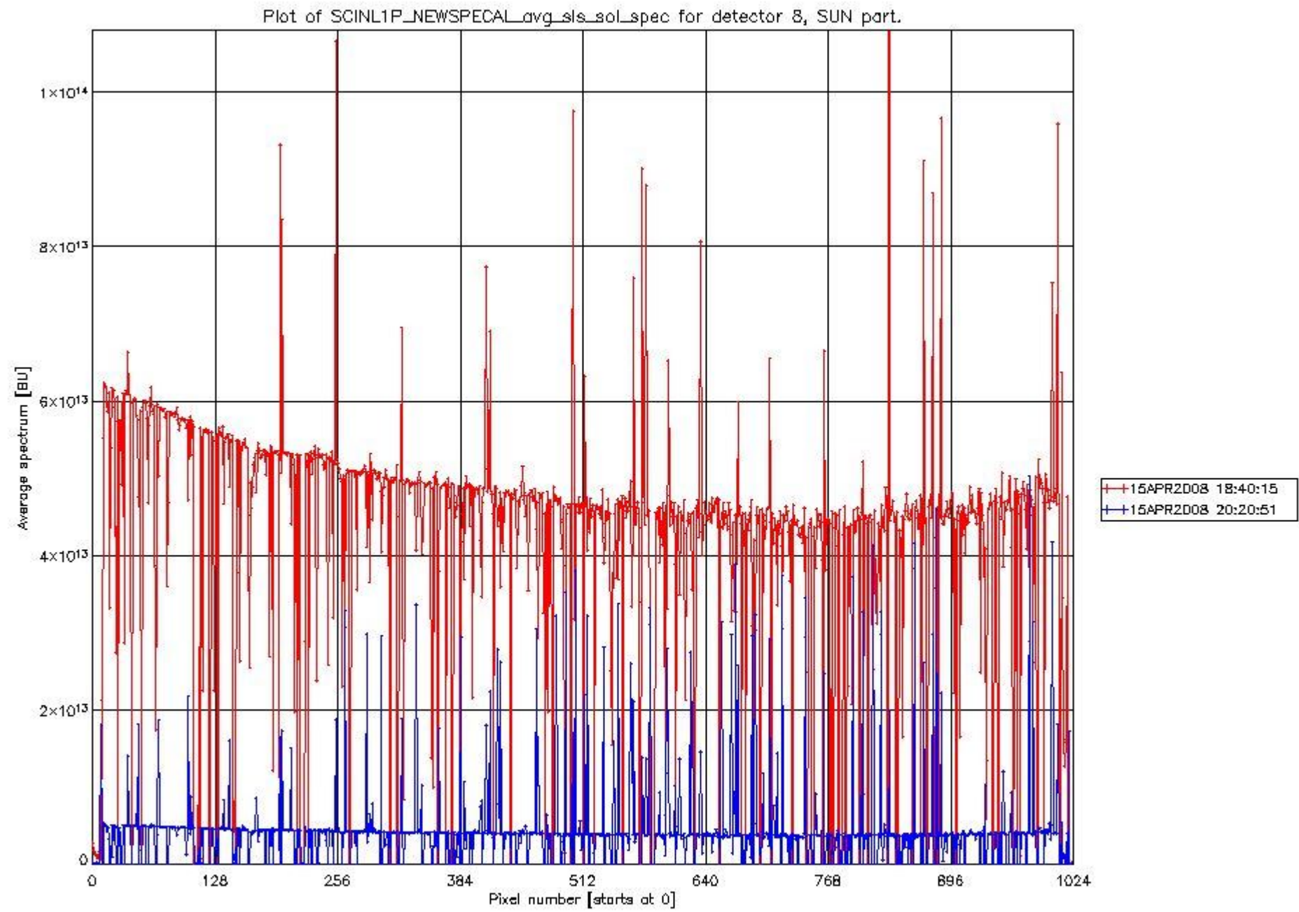
sciamachy_daily_report_level1_SCIA_6_03_N_20080415_30.PNG
