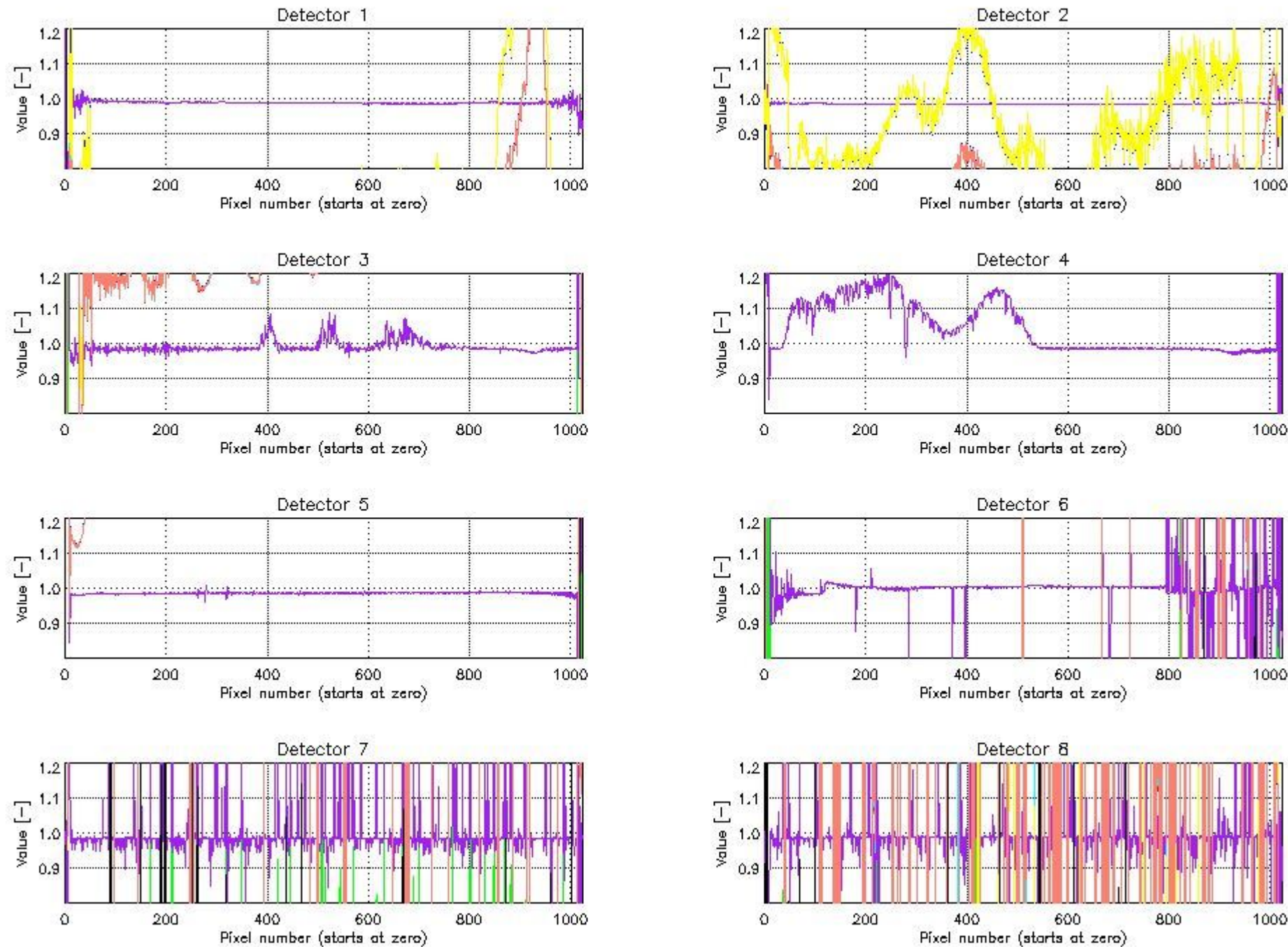
sciamachy_daily_report_level1_SCIA_6_03_N_20080415_41.PNG
