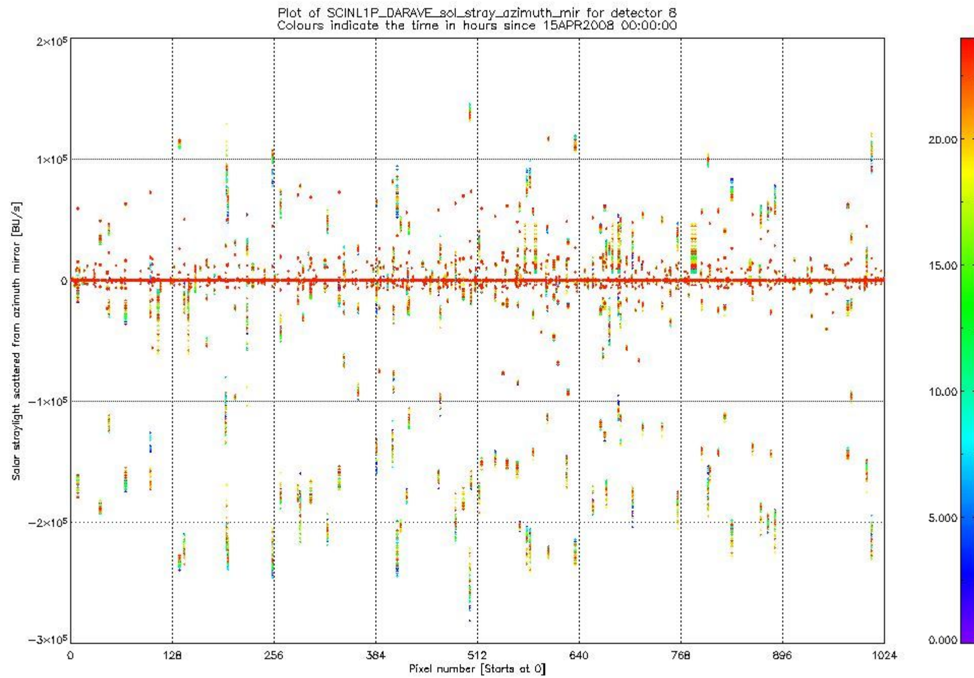
sciamachy_daily_report_level1_SCIA_6_03_N_20080415_17.PNG
