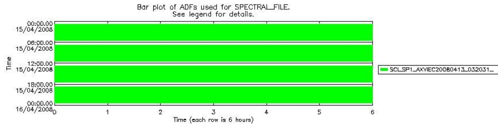
sciamachy_daily_report_level1_SCIA_6_03_N_20080415_44.PNG
