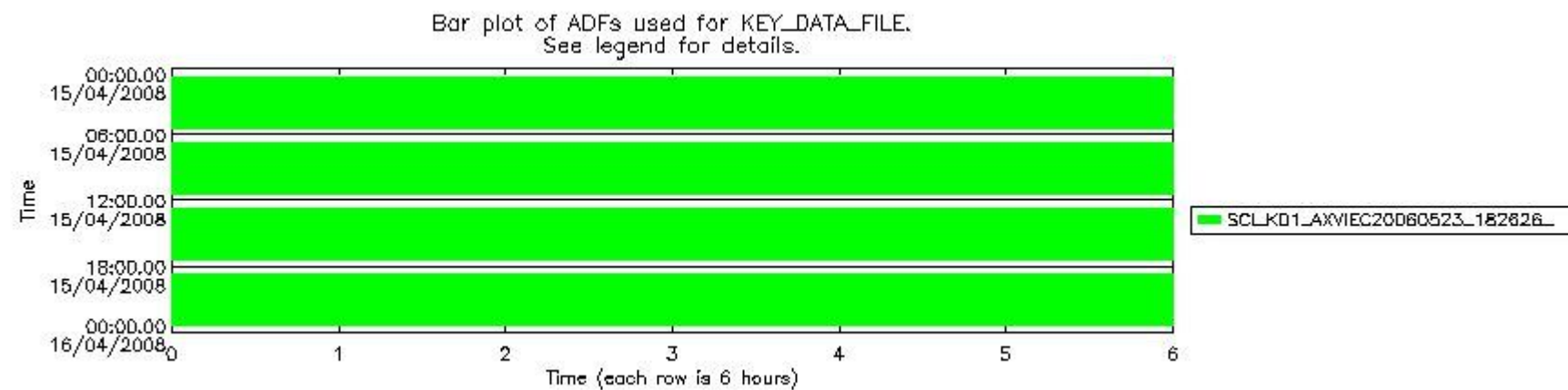
sciamachy_daily_report_level1_SCIA_6_03_N_20080415_45.PNG
