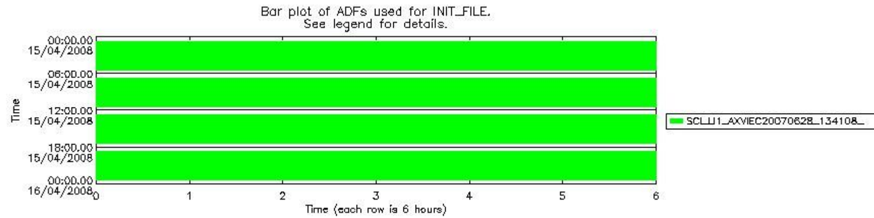
sciamachy_daily_report_level1_SCIA_6_03_N_20080415_48.PNG
