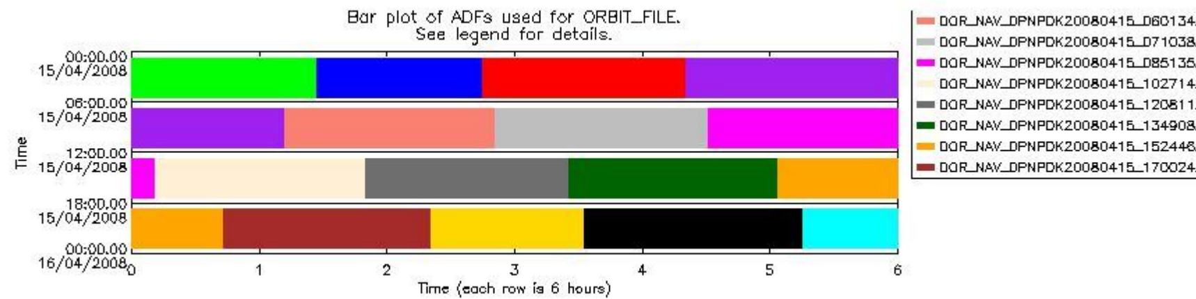
sciamachy_daily_report_level1_SCIA_6_03_N_20080415_49.PNG
