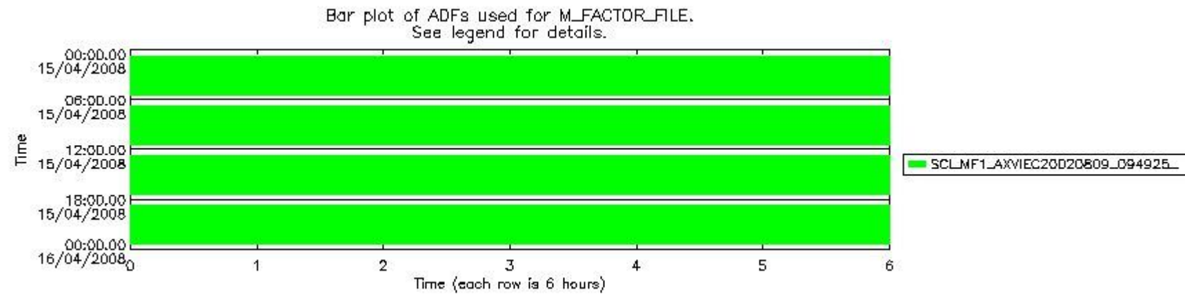
sciamachy_daily_report_level1_SCIA_6_03_N_20080415_47.PNG
