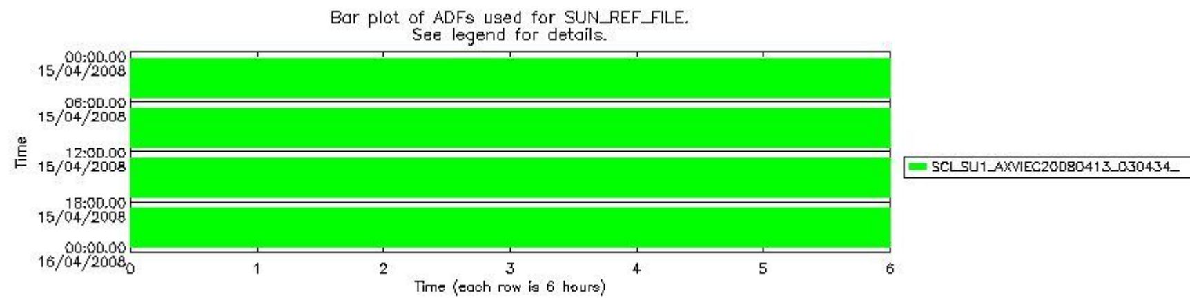
sciamachy_daily_report_level1_SCIA_6_03_N_20080415_45.PNG
