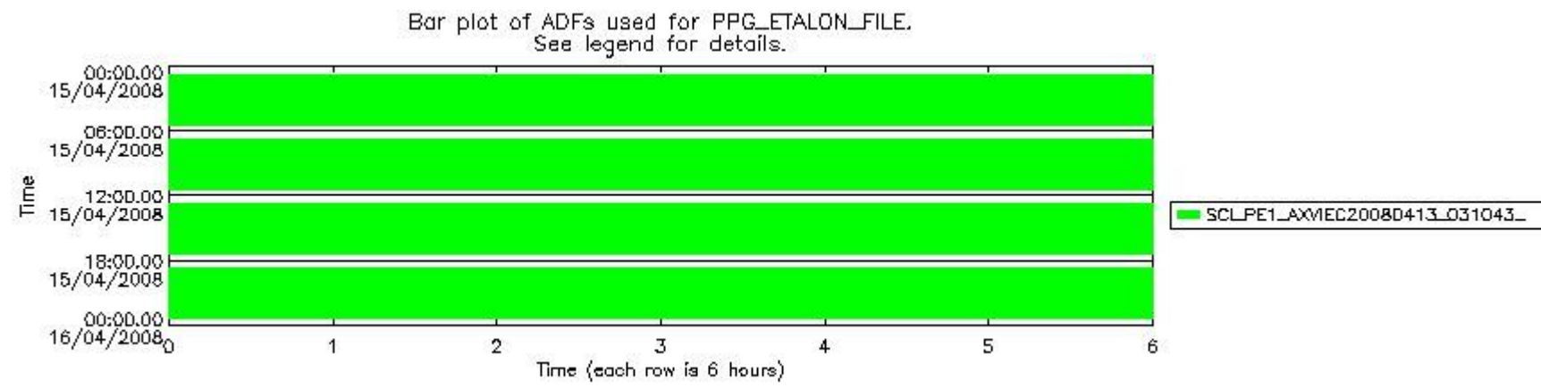
sciamachy_daily_report_level1_SCIA_6_03_N_20080415_43.PNG
