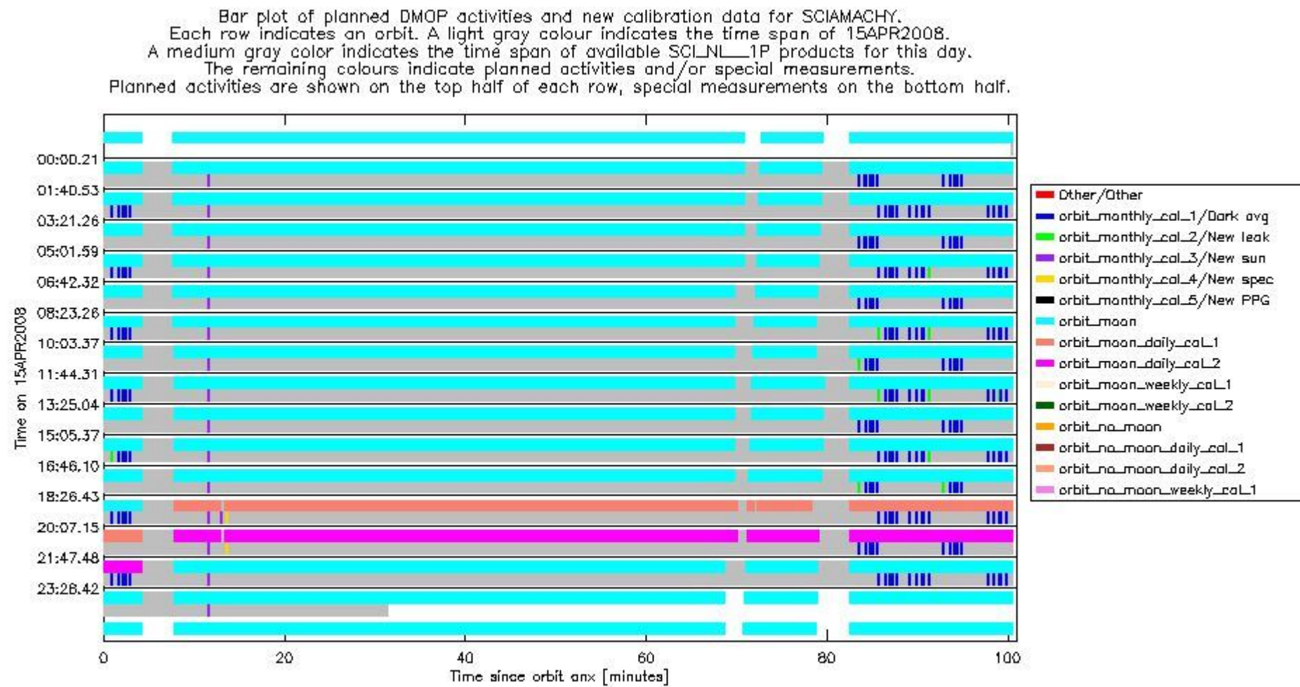
sciamachy_daily_report_level1_SCIA_6_03_N_20080415_51.PNG
