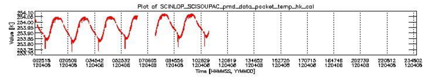
sciamachy_daily_report_level0_KSPT_L0_4504_N_20120408_3.PNG
