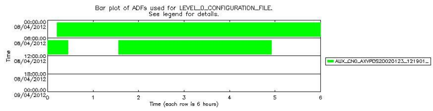
sciamachy_daily_report_level0_KSPT_L0_4504_N_20120408_6.PNG
