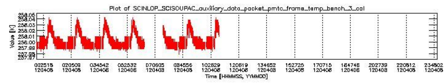
sciamachy_daily_report_level0_KSPT_L0_4504_N_20120408_2.PNG
