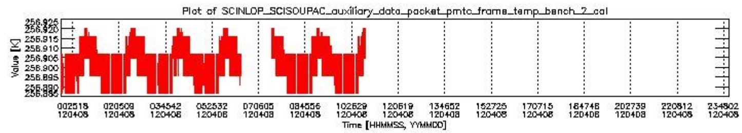
sciamachy_daily_report_level0_KSPT_L0_4504_N_20120408_1.PNG
