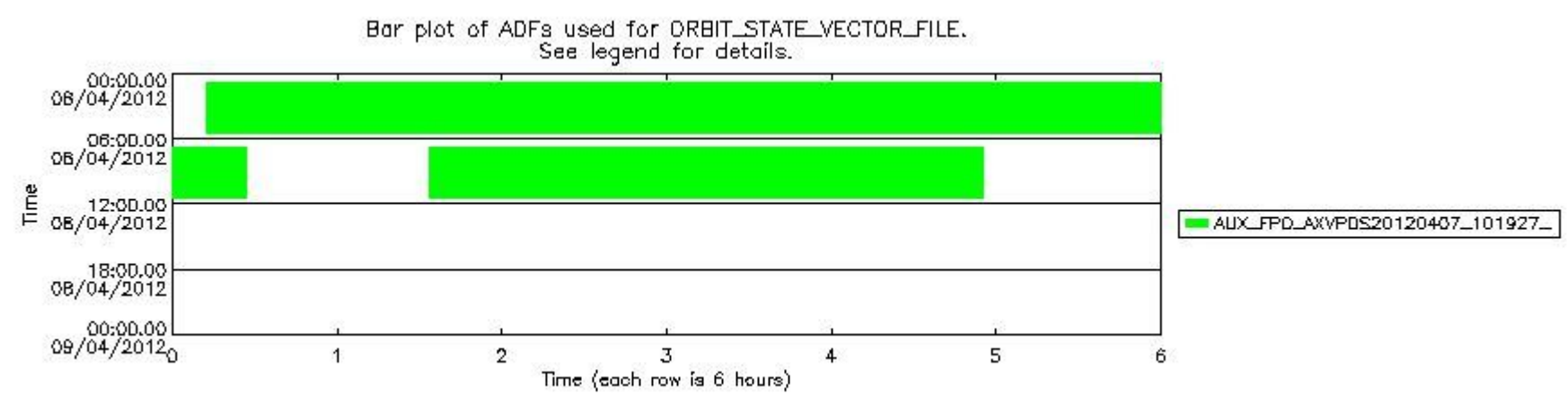
sciamachy_daily_report_level0_KSPT_L0_4504_N_20120408_7.PNG
