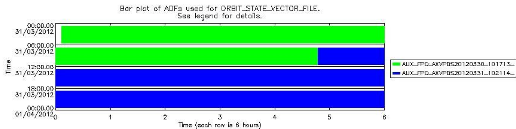
sciamachy_daily_report_level0_KSPT_L0_4504_N_20120331_7.PNG
