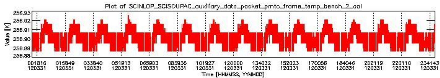
sciamachy_daily_report_level0_KSPT_L0_4504_N_20120331_1.PNG
