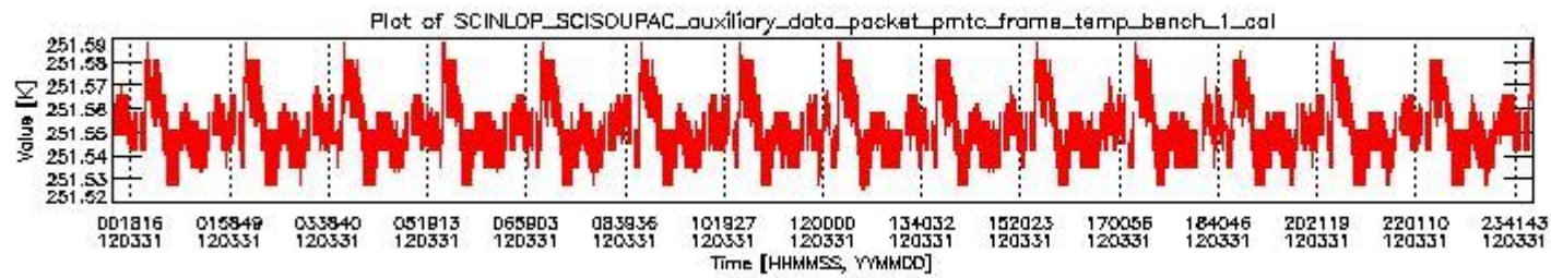
sciamachy_daily_report_level0_KSPT_L0_4504_N_20120331_0.PNG
