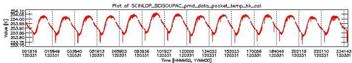
sciamachy_daily_report_level0_KSPT_L0_4504_N_20120331_3.PNG
