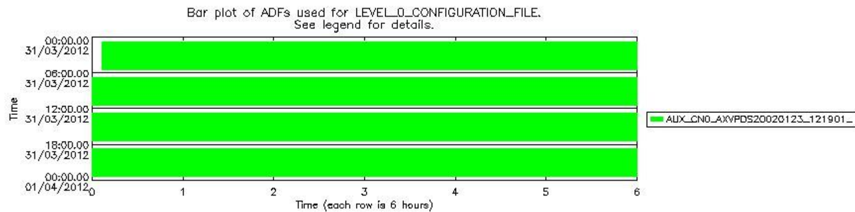
sciamachy_daily_report_level0_KSPT_L0_4504_N_20120331_6.PNG
