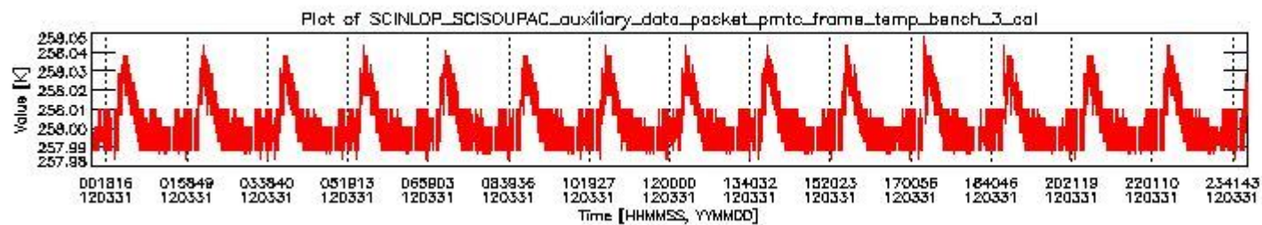
sciamachy_daily_report_level0_KSPT_L0_4504_N_20120331_2.PNG
