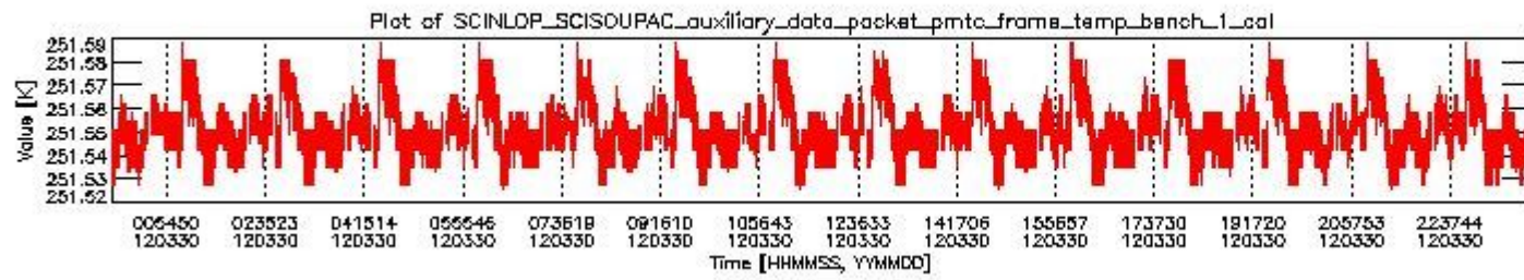
sciamachy_daily_report_level0_KSPT_L0_4504_N_20120330_0.PNG
