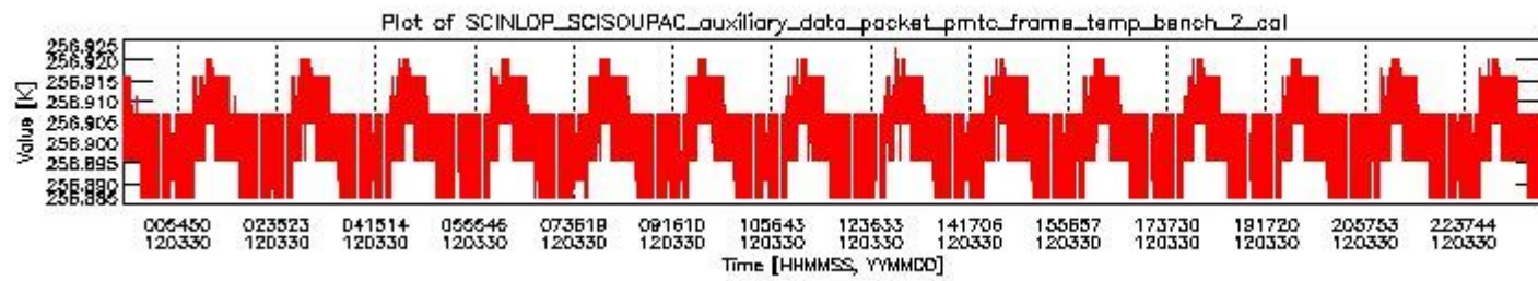
sciamachy_daily_report_level0_KSPT_L0_4504_N_20120330_1.PNG
