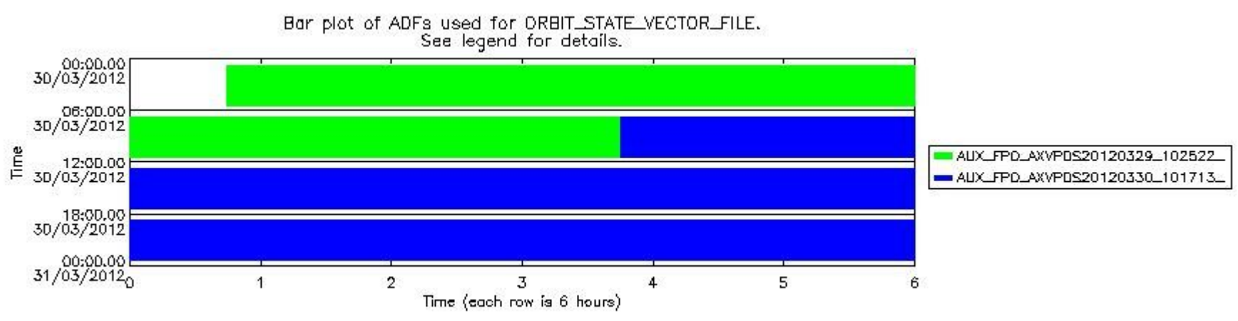
sciamachy_daily_report_level0_KSPT_L0_4504_N_20120330_7.PNG
