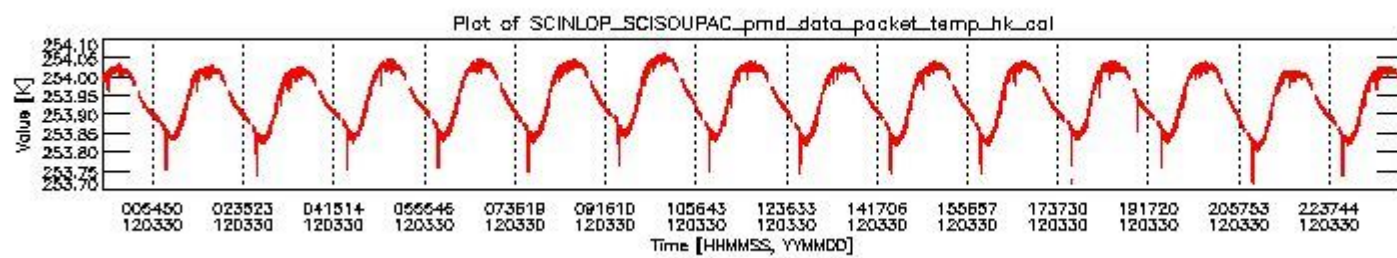
sciamachy_daily_report_level0_KSPT_L0_4504_N_20120330_3.PNG
