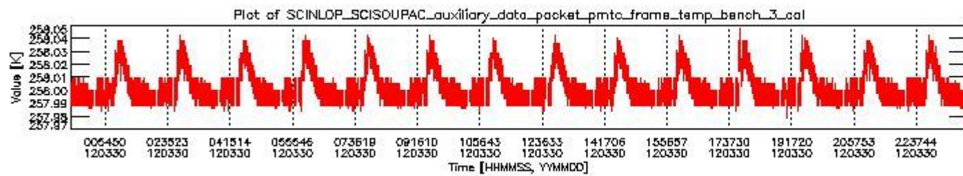
sciamachy_daily_report_level0_KSPT_L0_4504_N_20120330_2.PNG
