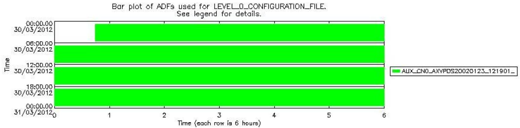
sciamachy_daily_report_level0_KSPT_L0_4504_N_20120330_6.PNG
