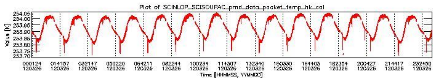
sciamachy_daily_report_level0_KSPT_L0_4504_N_20120326_3.PNG
