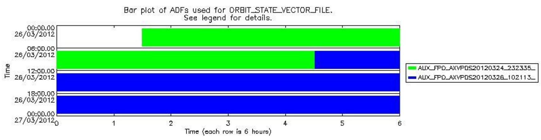
sciamachy_daily_report_level0_KSPT_L0_4504_N_20120326_7.PNG
