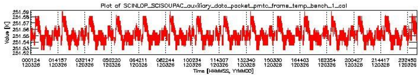
sciamachy_daily_report_level0_KSPT_L0_4504_N_20120326_0.PNG
