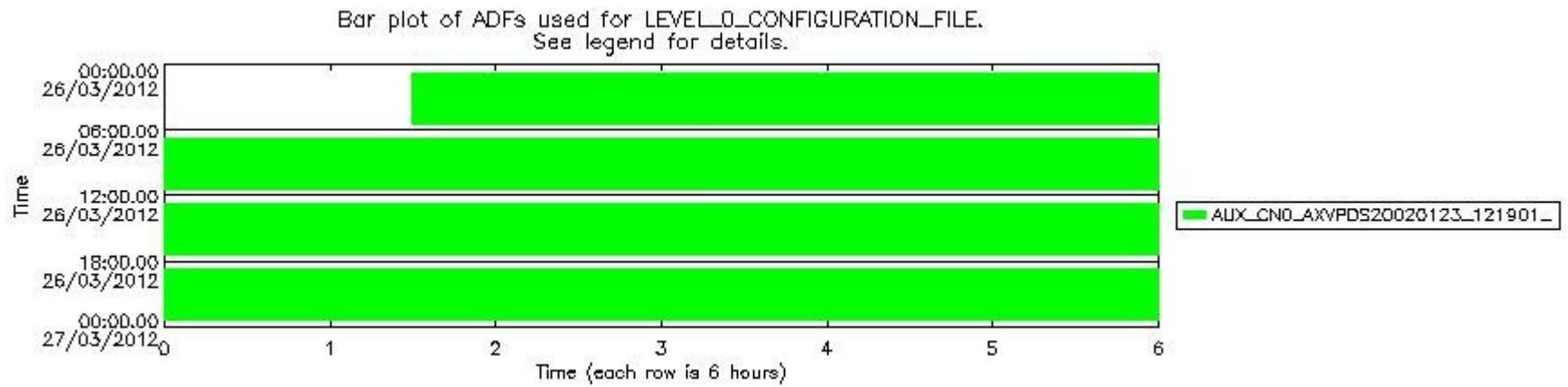
sciamachy_daily_report_level0_KSPT_L0_4504_N_20120326_6.PNG
