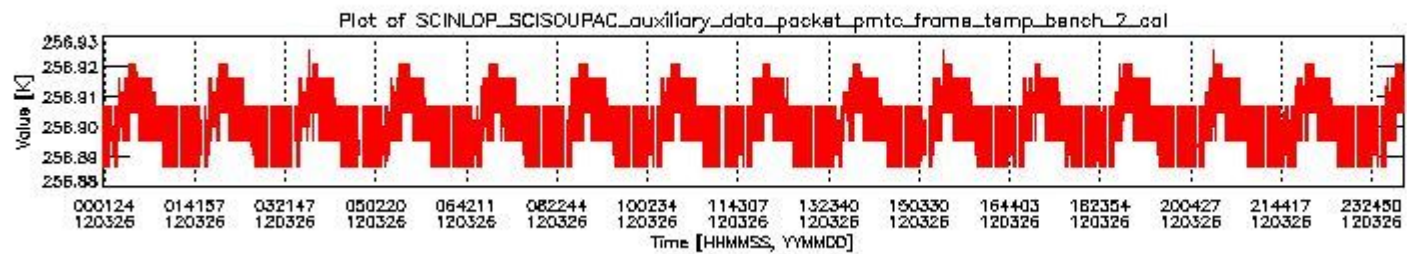
sciamachy_daily_report_level0_KSPT_L0_4504_N_20120326_1.PNG
