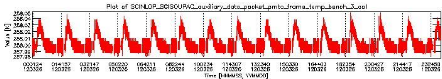
sciamachy_daily_report_level0_KSPT_L0_4504_N_20120326_2.PNG
