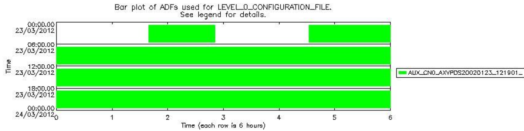
sciamachy_daily_report_level0_KSPT_L0_4504_N_20120323_6.PNG
