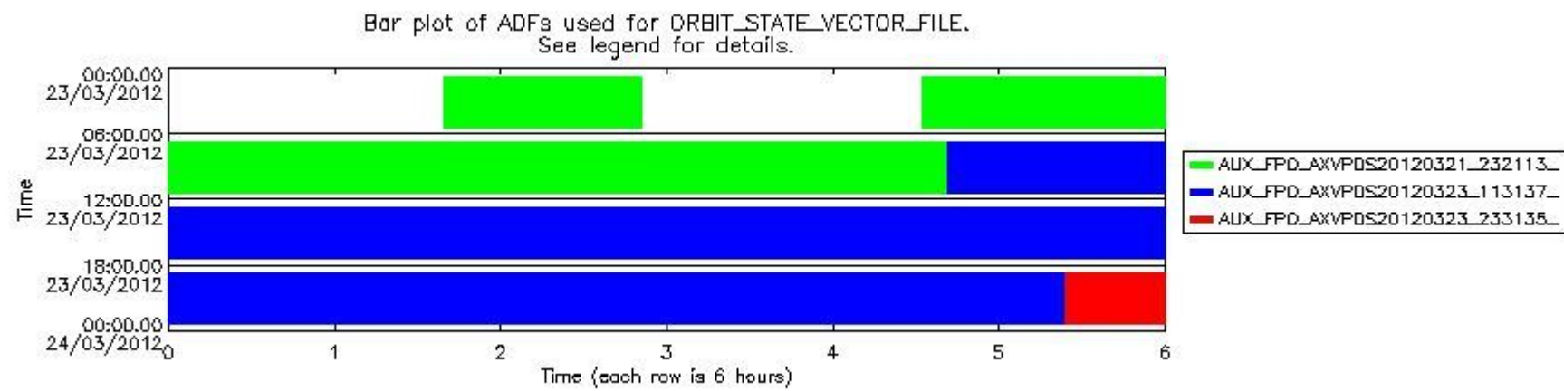
sciamachy_daily_report_level0_KSPT_L0_4504_N_20120323_7.PNG
