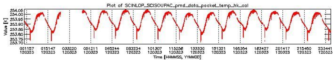
sciamachy_daily_report_level0_KSPT_L0_4504_N_20120323_3.PNG
