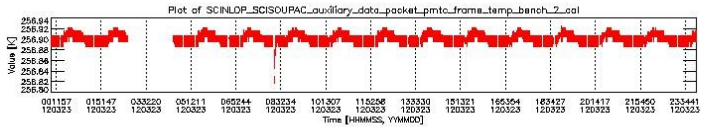
sciamachy_daily_report_level0_KSPT_L0_4504_N_20120323_1.PNG
