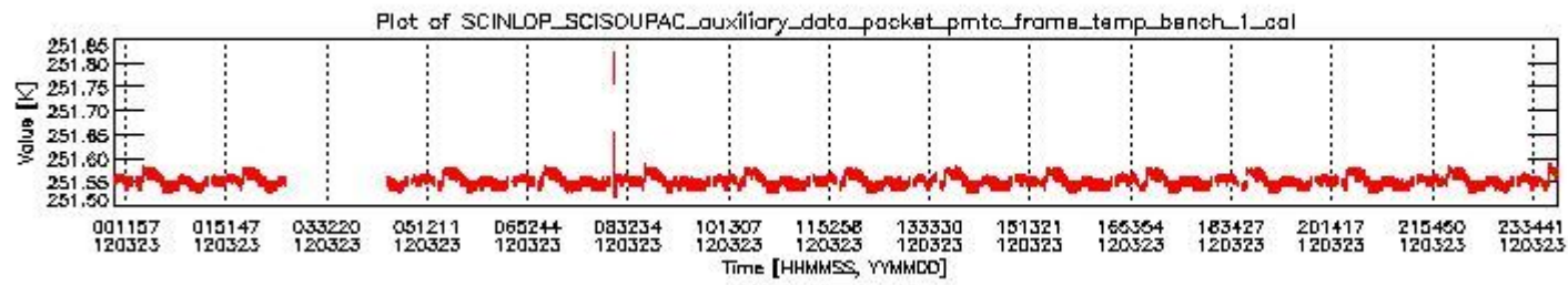
sciamachy_daily_report_level0_KSPT_L0_4504_N_20120323_0.PNG
