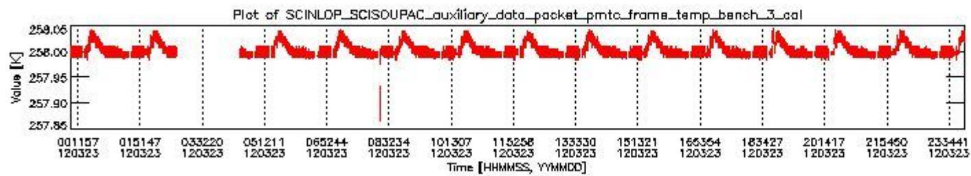
sciamachy_daily_report_level0_KSPT_L0_4504_N_20120323_2.PNG
