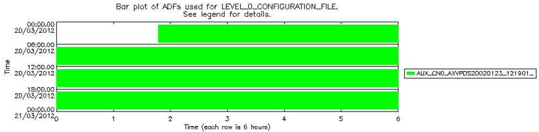
sciamachy_daily_report_level0_KSPT_L0_4504_N_20120320_6.PNG
