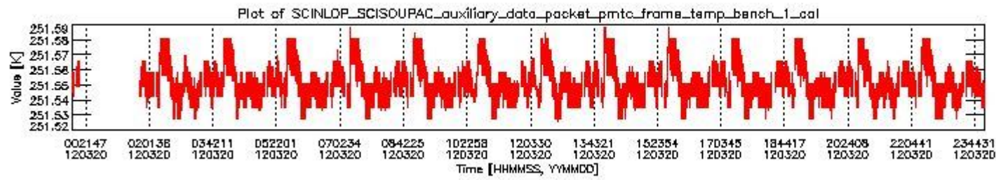
sciamachy_daily_report_level0_KSPT_L0_4504_N_20120320_0.PNG
