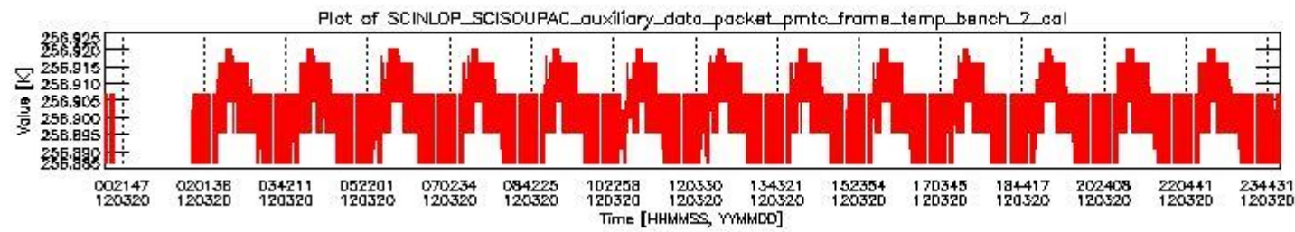
sciamachy_daily_report_level0_KSPT_L0_4504_N_20120320_1.PNG
