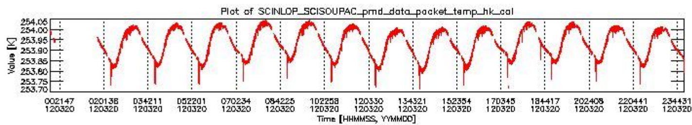
sciamachy_daily_report_level0_KSPT_L0_4504_N_20120320_3.PNG
