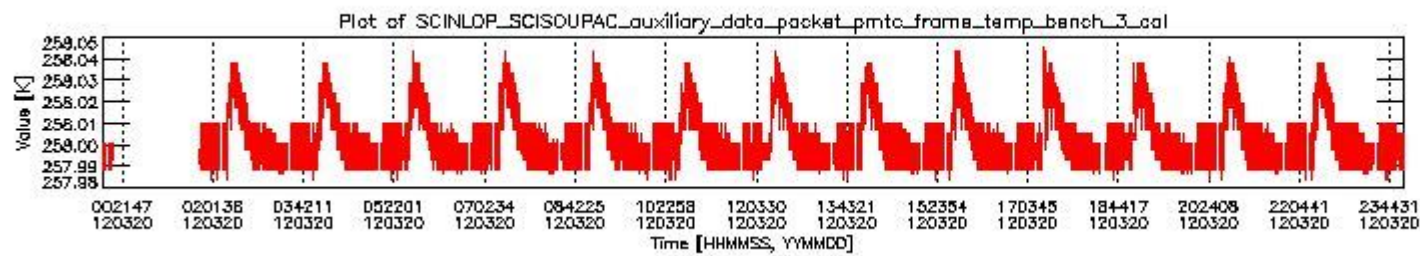
sciamachy_daily_report_level0_KSPT_L0_4504_N_20120320_2.PNG
