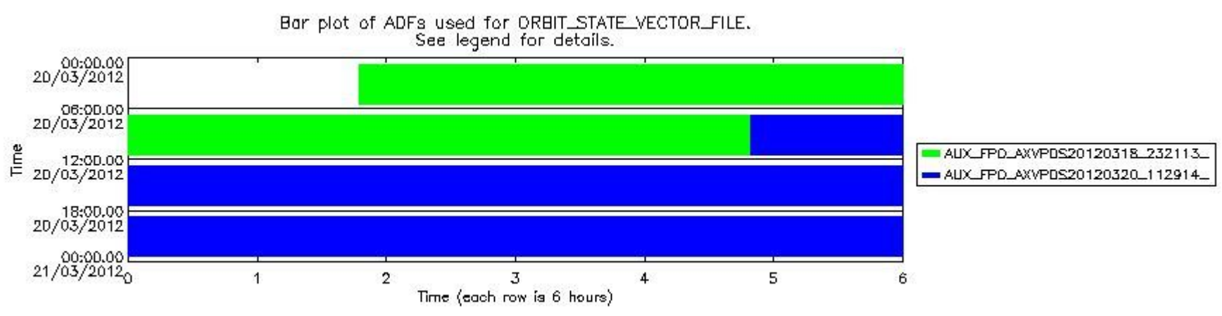
sciamachy_daily_report_level0_KSPT_L0_4504_N_20120320_7.PNG
