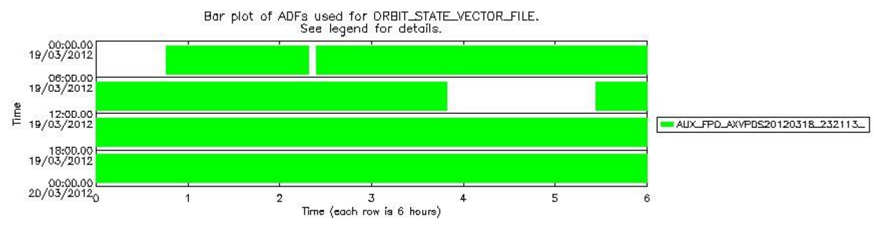
sciamachy_daily_report_level0_KSPT_L0_4504_N_20120319_7.PNG
