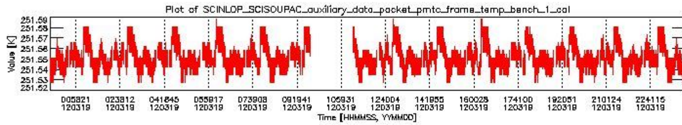
sciamachy_daily_report_level0_KSPT_L0_4504_N_20120319_0.PNG
