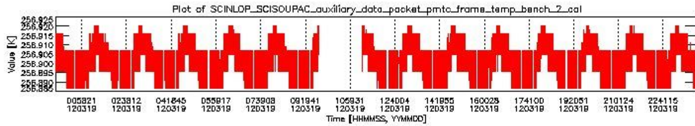
sciamachy_daily_report_level0_KSPT_L0_4504_N_20120319_1.PNG
