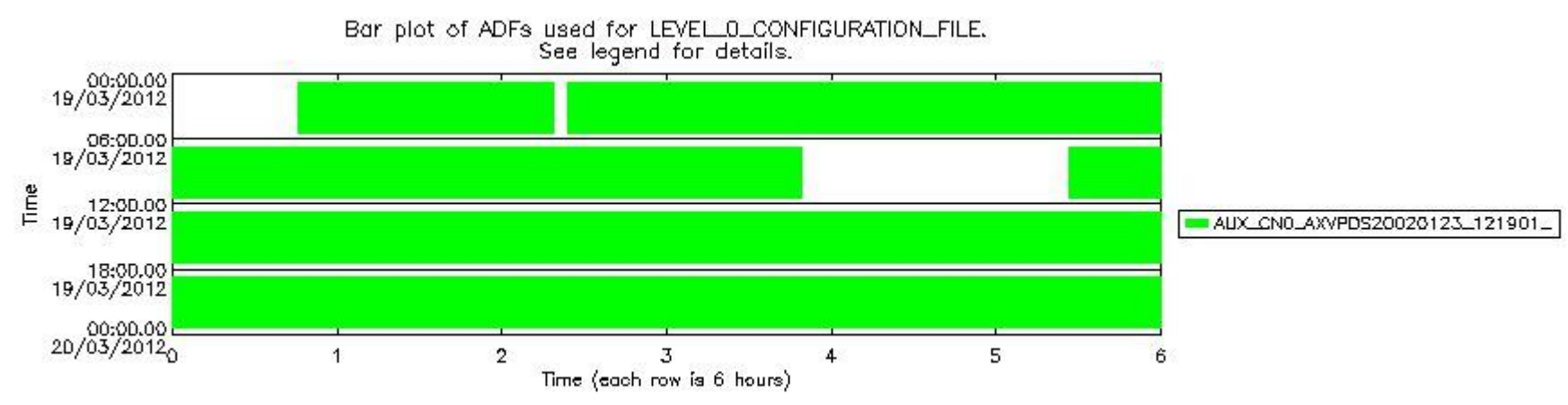
sciamachy_daily_report_level0_KSPT_L0_4504_N_20120319_6.PNG
