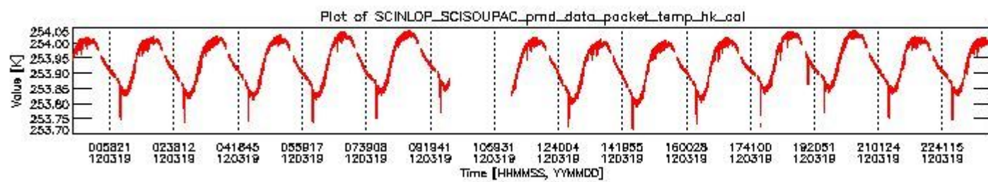
sciamachy_daily_report_level0_KSPT_L0_4504_N_20120319_3.PNG
