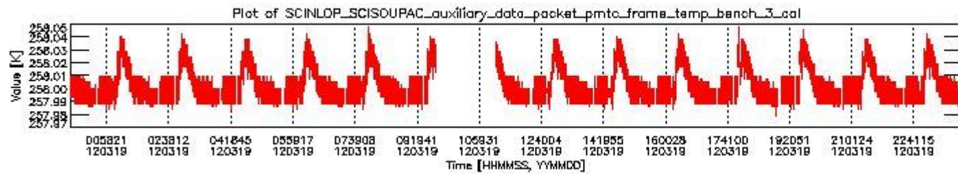
sciamachy_daily_report_level0_KSPT_L0_4504_N_20120319_2.PNG
