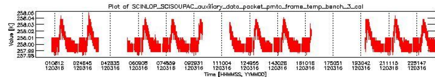
sciamachy_daily_report_level0_KSPT_L0_4504_N_20120316_2.PNG
