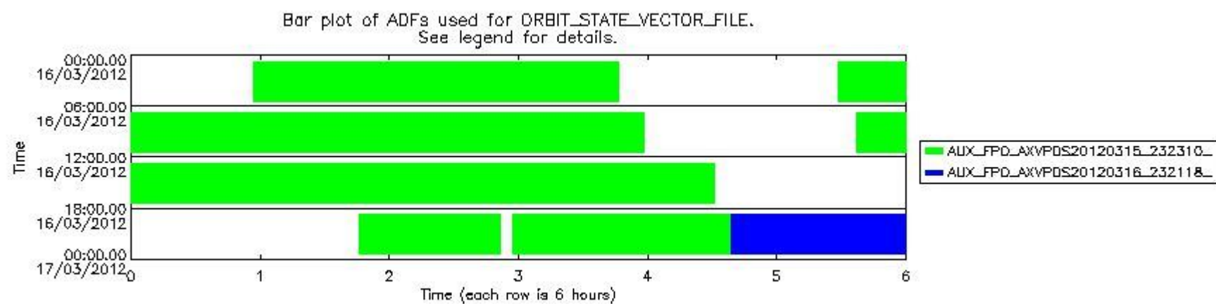
sciamachy_daily_report_level0_KSPT_L0_4504_N_20120316_7.PNG
