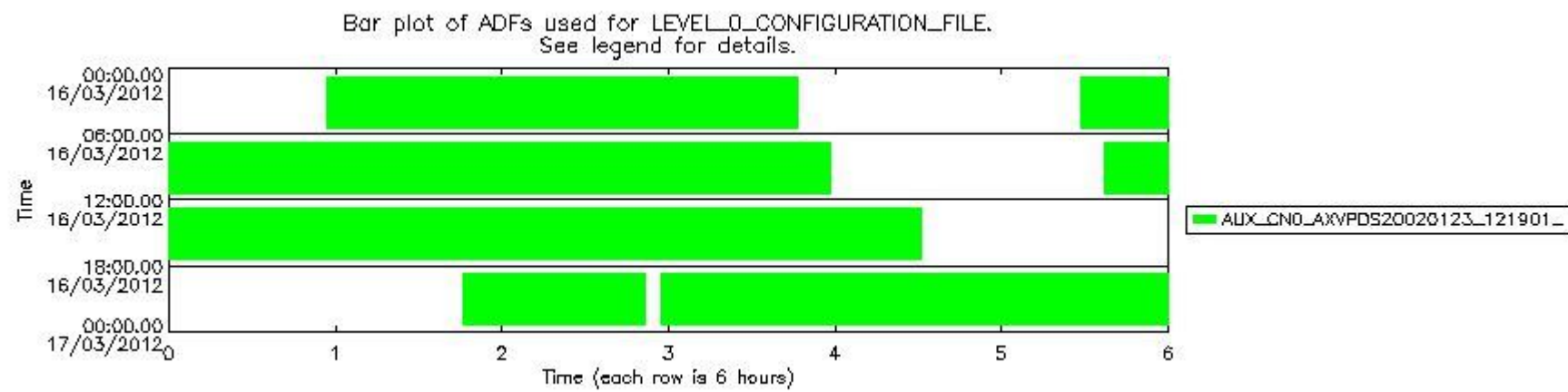
sciamachy_daily_report_level0_KSPT_L0_4504_N_20120316_6.PNG
