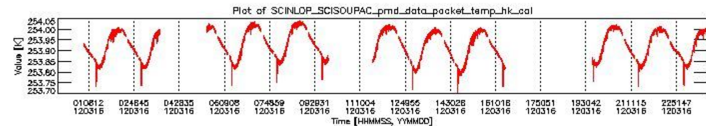
sciamachy_daily_report_level0_KSPT_L0_4504_N_20120316_3.PNG
