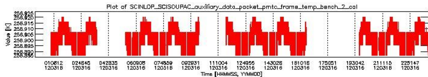
sciamachy_daily_report_level0_KSPT_L0_4504_N_20120316_1.PNG
