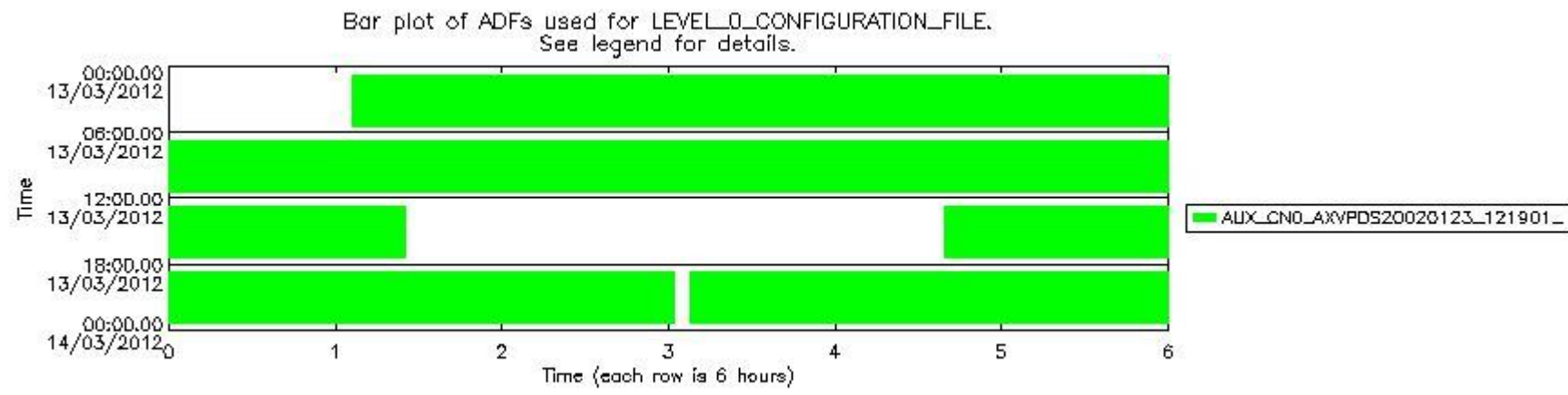
sciamachy_daily_report_level0_KSPT_L0_4504_N_20120313_6.PNG
