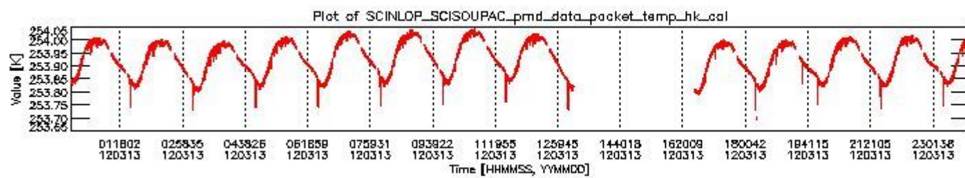
sciamachy_daily_report_level0_KSPT_L0_4504_N_20120313_3.PNG
