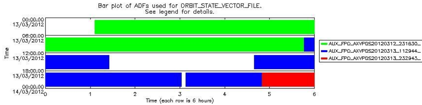
sciamachy_daily_report_level0_KSPT_L0_4504_N_20120313_7.PNG
