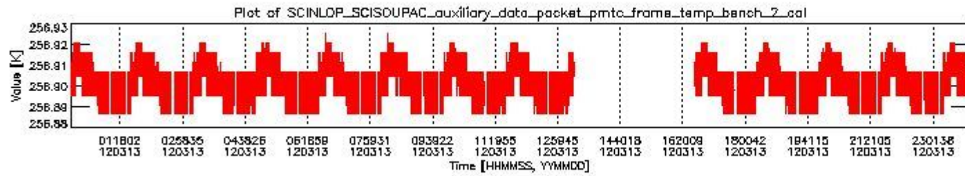
sciamachy_daily_report_level0_KSPT_L0_4504_N_20120313_1.PNG
