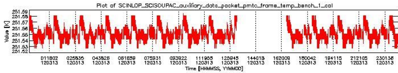
sciamachy_daily_report_level0_KSPT_L0_4504_N_20120313_0.PNG
