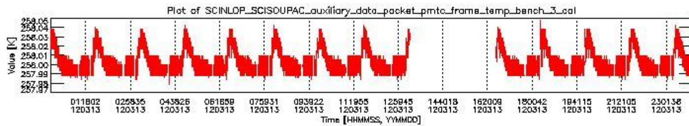
sciamachy_daily_report_level0_KSPT_L0_4504_N_20120313_2.PNG
