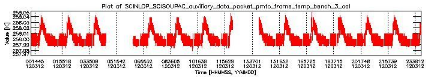
sciamachy_daily_report_level0_KSPT_L0_4504_N_20120312_2.PNG
