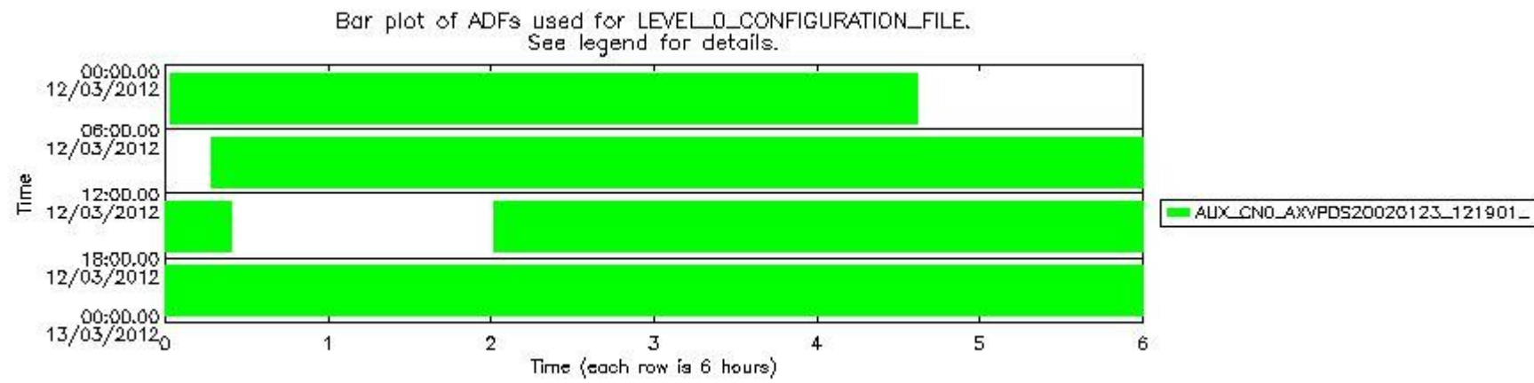
sciamachy_daily_report_level0_KSPT_L0_4504_N_20120312_6.PNG
