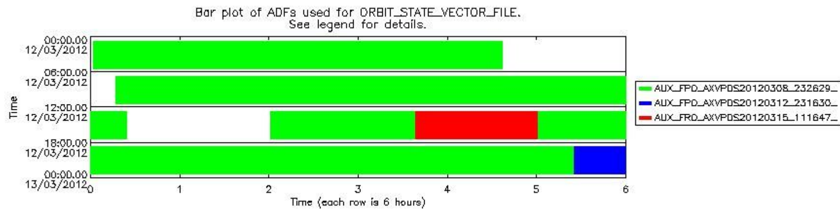
sciamachy_daily_report_level0_KSPT_L0_4504_N_20120312_7.PNG
