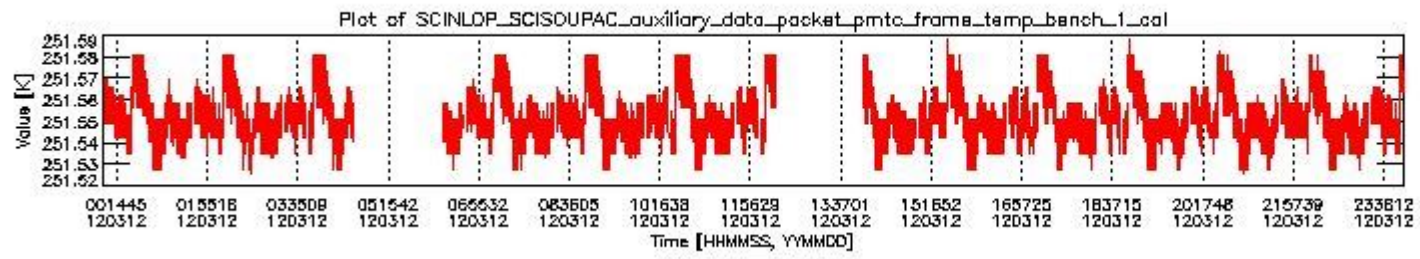
sciamachy_daily_report_level0_KSPT_L0_4504_N_20120312_0.PNG
