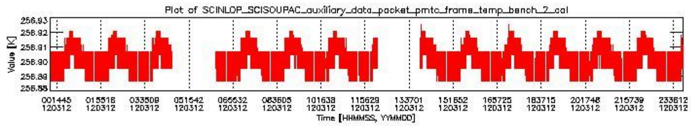
sciamachy_daily_report_level0_KSPT_L0_4504_N_20120312_1.PNG
