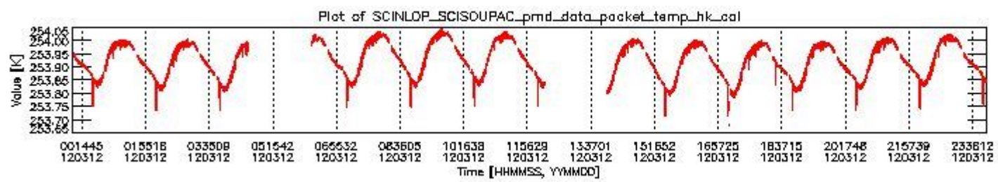
sciamachy_daily_report_level0_KSPT_L0_4504_N_20120312_3.PNG
