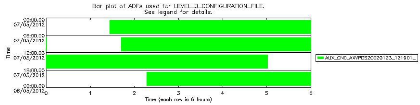
sciamachy_daily_report_level0_KSPT_L0_4504_N_20120307_6.PNG
