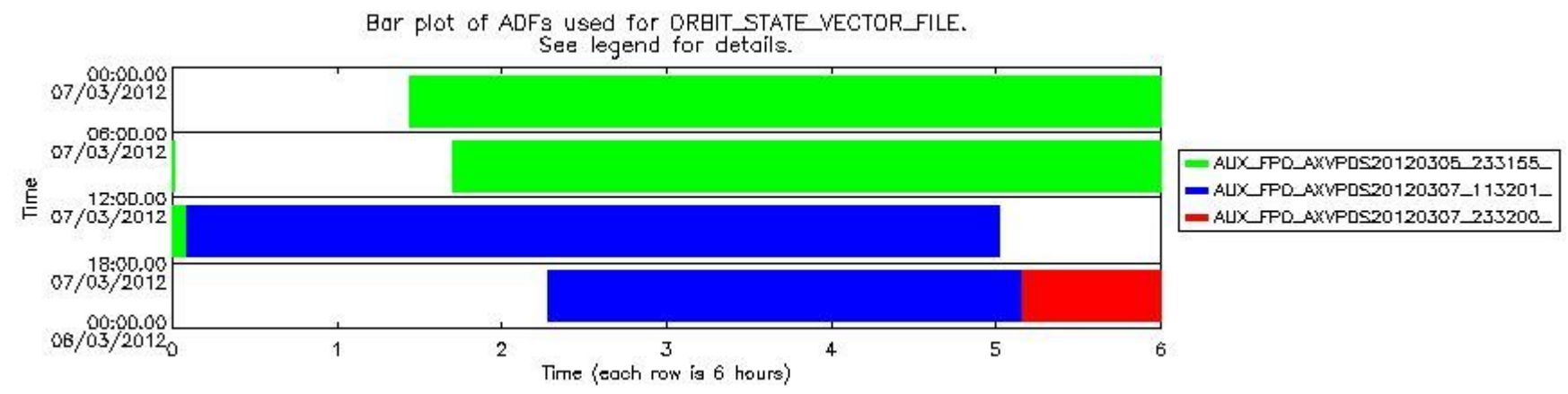
sciamachy_daily_report_level0_KSPT_L0_4504_N_20120307_7.PNG
