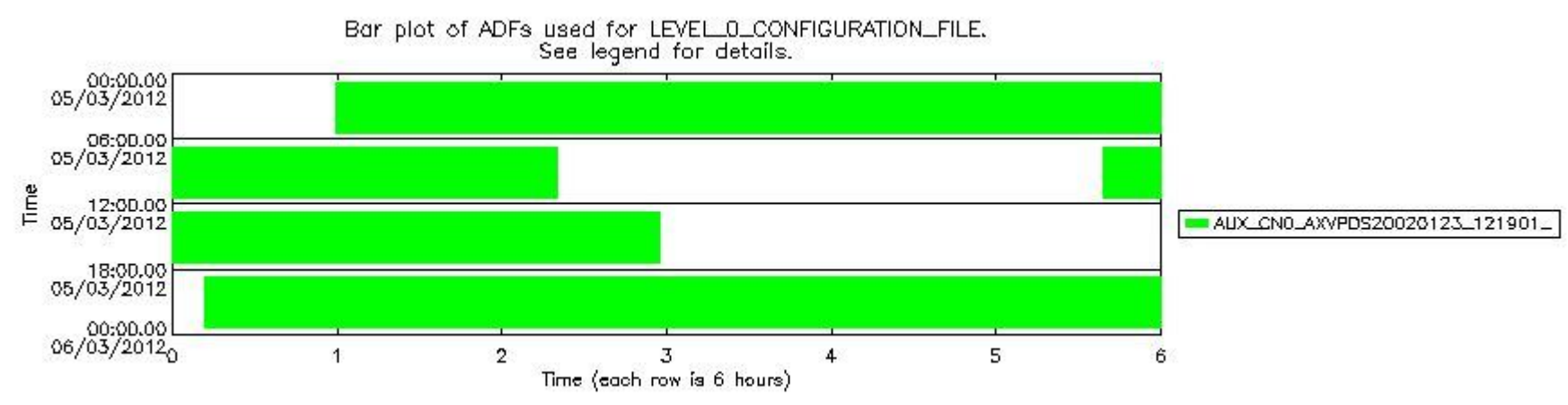
sciamachy_daily_report_level0_KSPT_L0_4504_N_20120305_6.PNG
