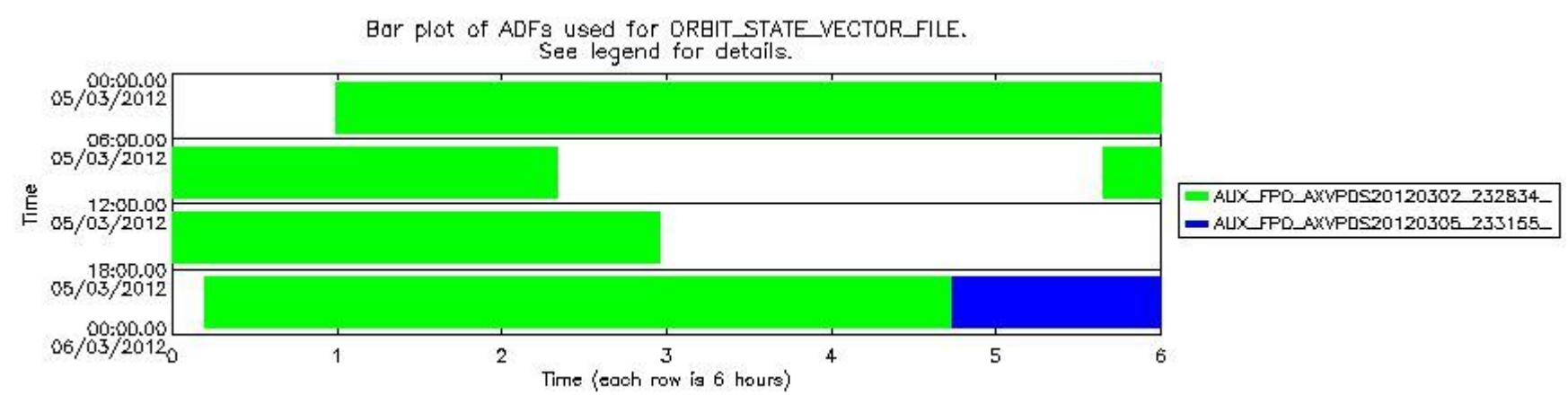
sciamachy_daily_report_level0_KSPT_L0_4504_N_20120305_7.PNG
