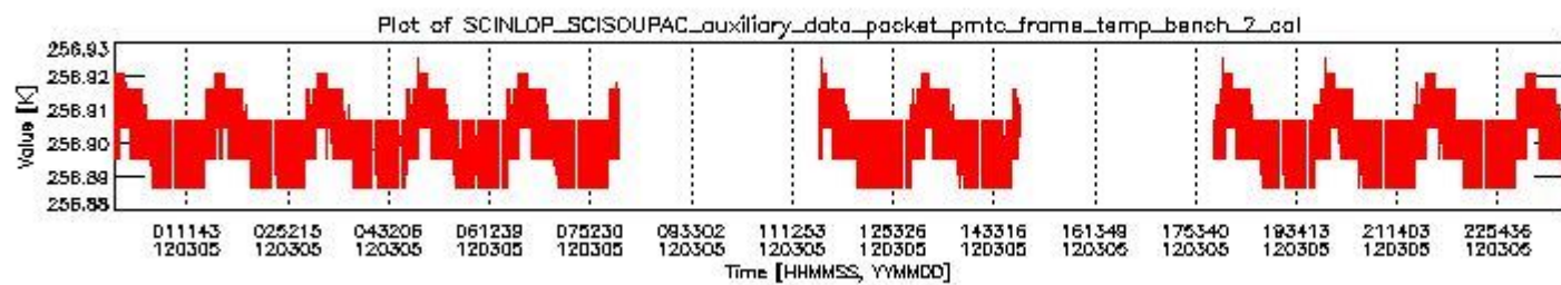
sciamachy_daily_report_level0_KSPT_L0_4504_N_20120305_1.PNG
