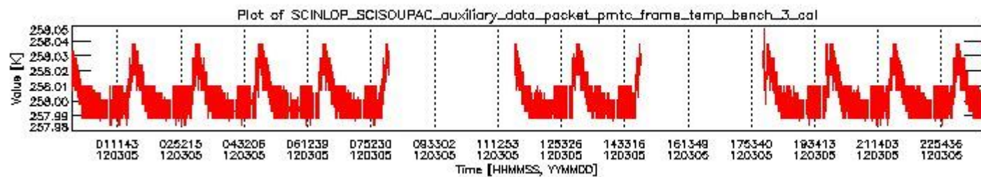
sciamachy_daily_report_level0_KSPT_L0_4504_N_20120305_2.PNG
