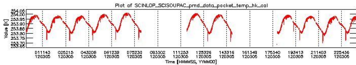
sciamachy_daily_report_level0_KSPT_L0_4504_N_20120305_3.PNG
