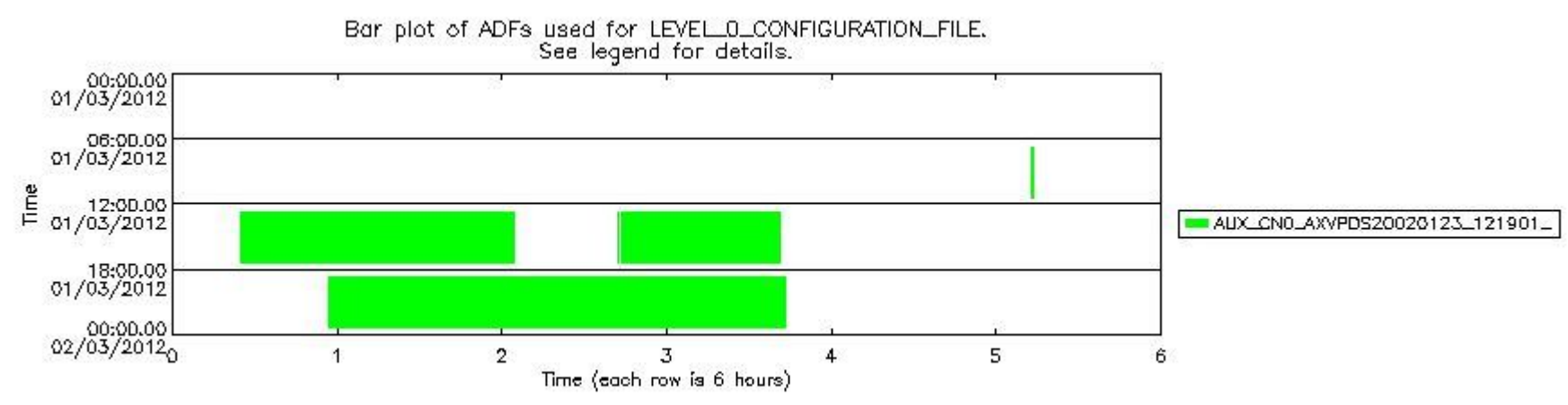
sciamachy_daily_report_level0_KSPT_L0_4504_N_20120301_6.PNG
