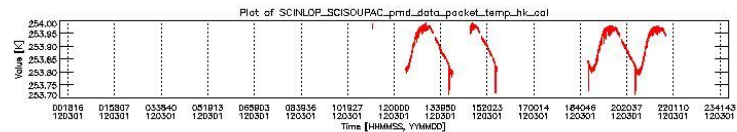
sciamachy_daily_report_level0_KSPT_L0_4504_N_20120301_3.PNG
