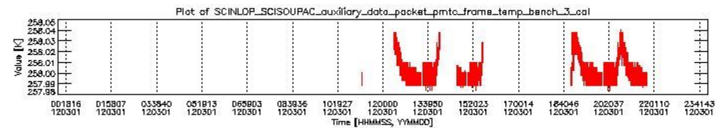
sciamachy_daily_report_level0_KSPT_L0_4504_N_20120301_2.PNG
