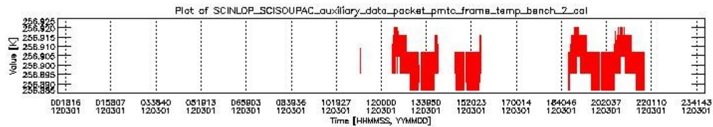
sciamachy_daily_report_level0_KSPT_L0_4504_N_20120301_1.PNG
