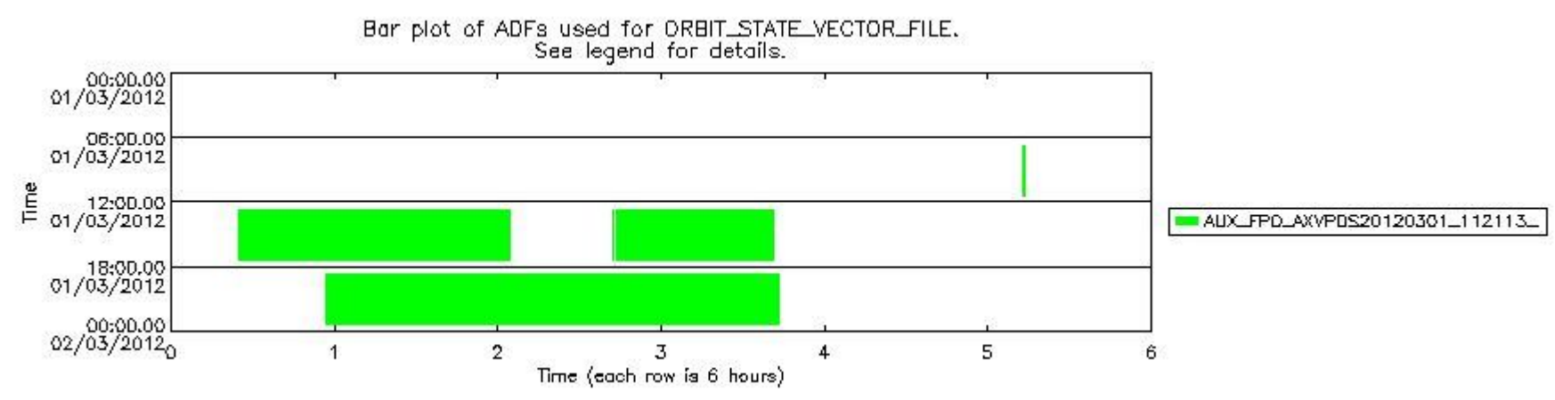
sciamachy_daily_report_level0_KSPT_L0_4504_N_20120301_7.PNG
