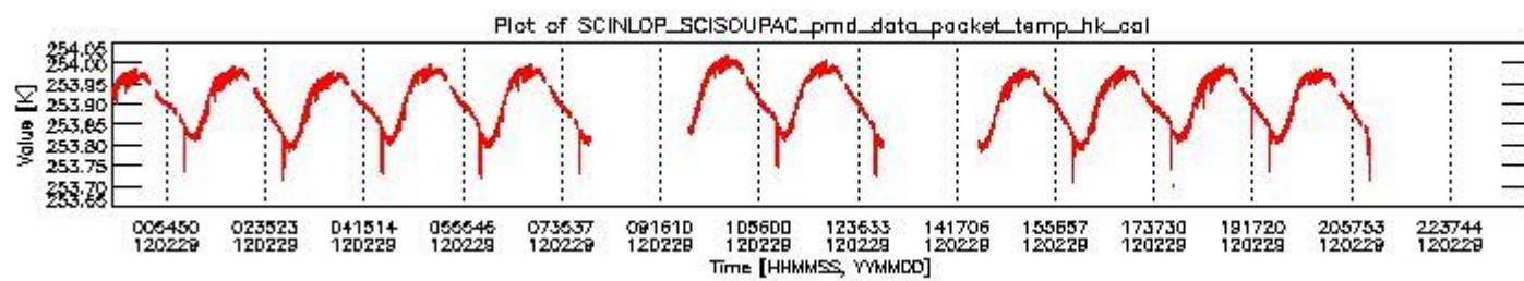
sciamachy_daily_report_level0_KSPT_L0_4504_N_20120229_3.PNG
