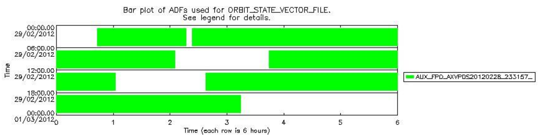
sciamachy_daily_report_level0_KSPT_L0_4504_N_20120229_7.PNG
