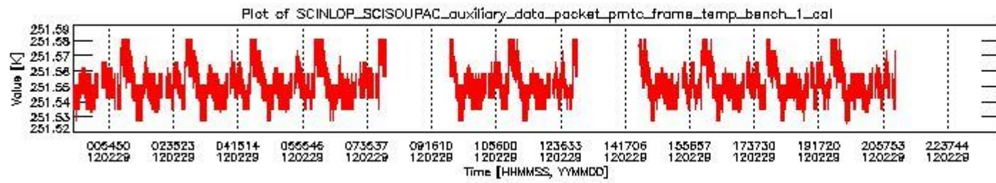
sciamachy_daily_report_level0_KSPT_L0_4504_N_20120229_0.PNG
