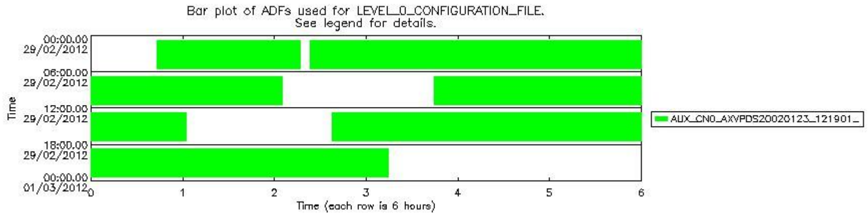
sciamachy_daily_report_level0_KSPT_L0_4504_N_20120229_6.PNG
