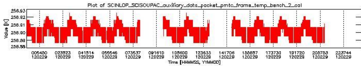
sciamachy_daily_report_level0_KSPT_L0_4504_N_20120229_1.PNG
