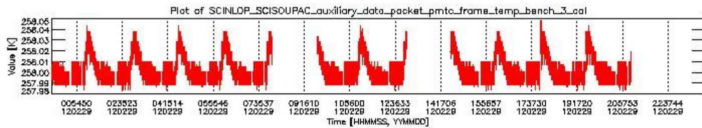
sciamachy_daily_report_level0_KSPT_L0_4504_N_20120229_2.PNG
