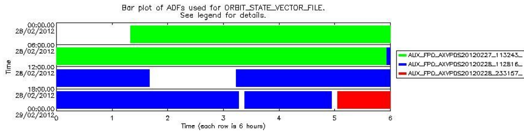
sciamachy_daily_report_level0_KSPT_L0_4504_N_20120228_7.PNG
