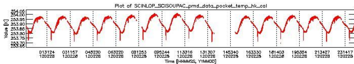
sciamachy_daily_report_level0_KSPT_L0_4504_N_20120228_3.PNG
