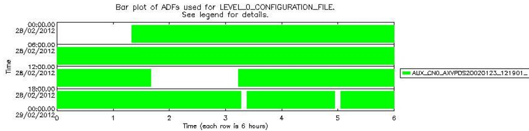
sciamachy_daily_report_level0_KSPT_L0_4504_N_20120228_6.PNG
