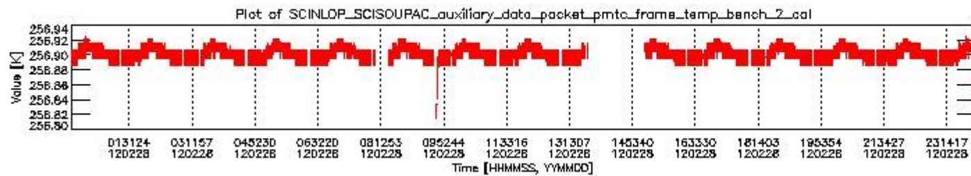
sciamachy_daily_report_level0_KSPT_L0_4504_N_20120228_1.PNG
