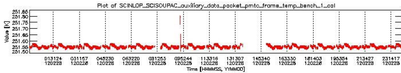
sciamachy_daily_report_level0_KSPT_L0_4504_N_20120228_0.PNG
