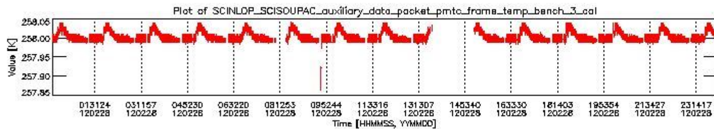
sciamachy_daily_report_level0_KSPT_L0_4504_N_20120228_2.PNG
